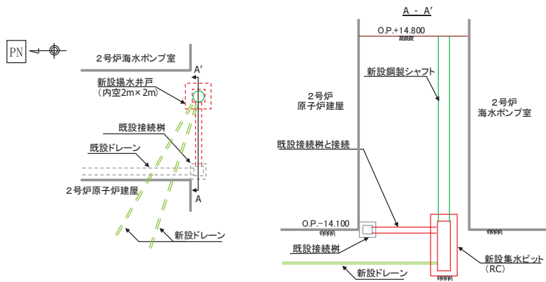
(平面図) (断面図) 補足 8-1 図 新設揚水井戸の構造・配置例
