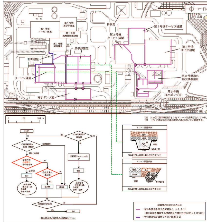
図 5-6 管の耐震性・透水層の連続性の観点からの整理結果 (Step③・⑤)
