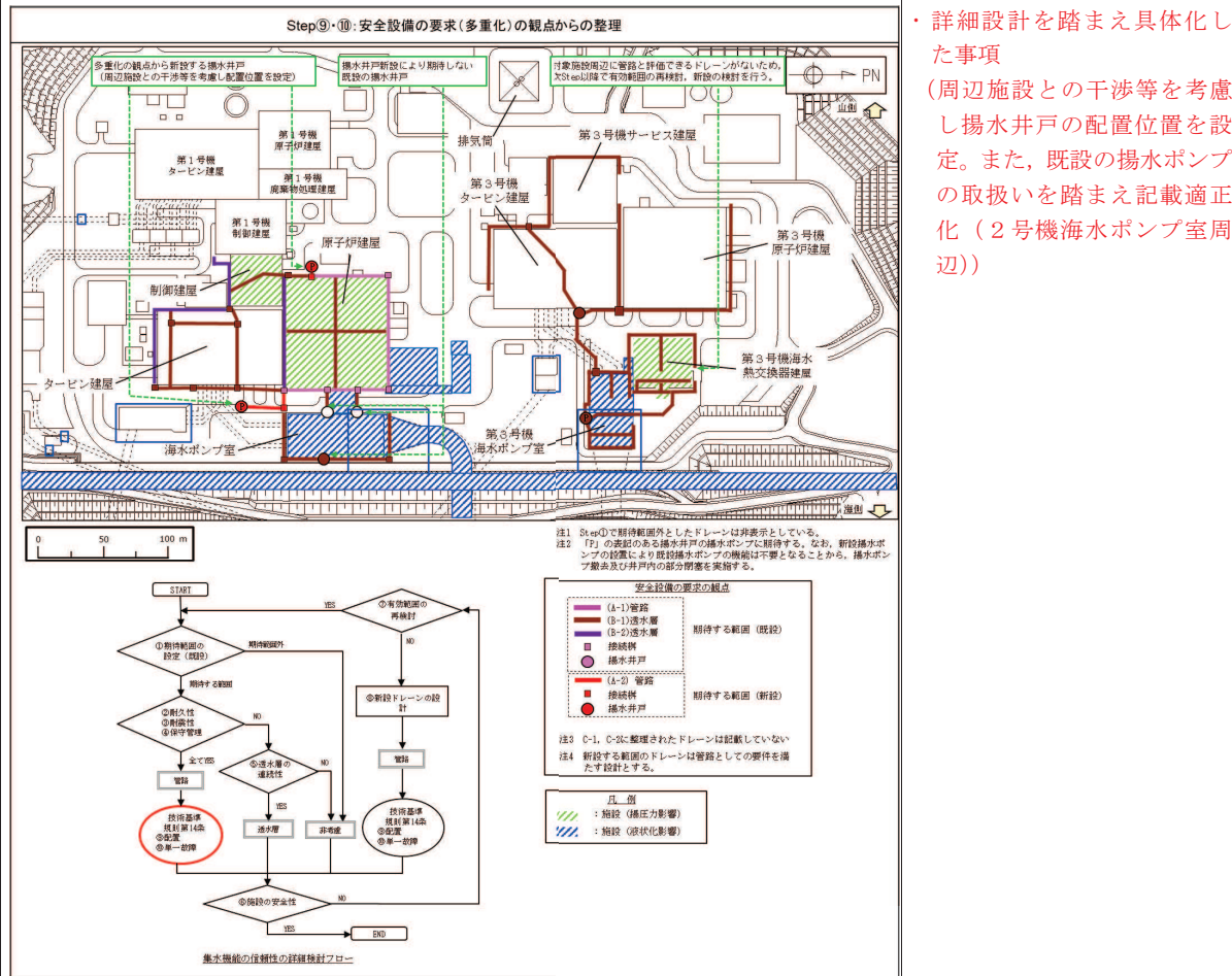
図5-8 安全設備の要求の観点からの整理結果 (Step⑨・⑩)
