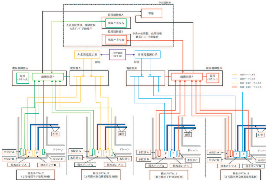
図 4-3 系統構成図
