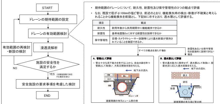
添付 2-2 図 集水機能の検討フロー
