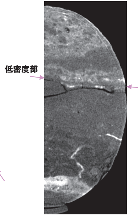
2.5cm 走向方向断面
