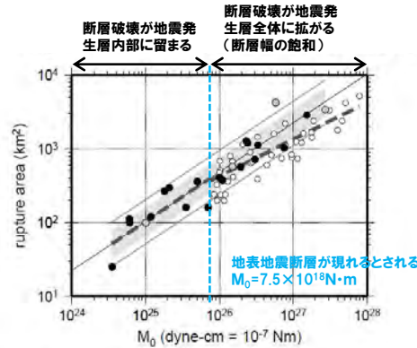
図 8 震源特性化の手続き-その1:巨視的断層パラメータの設定。 Step 1は断層長さLを定義, Step 2は断層長さLと断層幅Wの関係(太点線), Step 3は断層面積( S=LW )と地震モーメント M_0 の関係(太点線)を与える。この結果, シナリオ地震の地震モーメントが与えられる。
