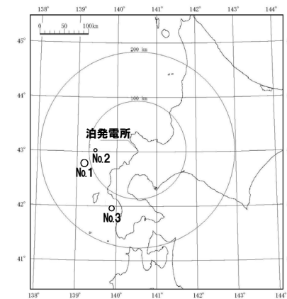
震央分布図
