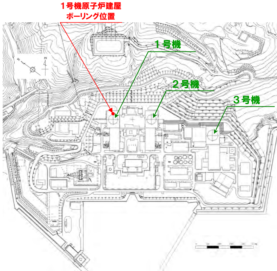
ボーリング位置図
