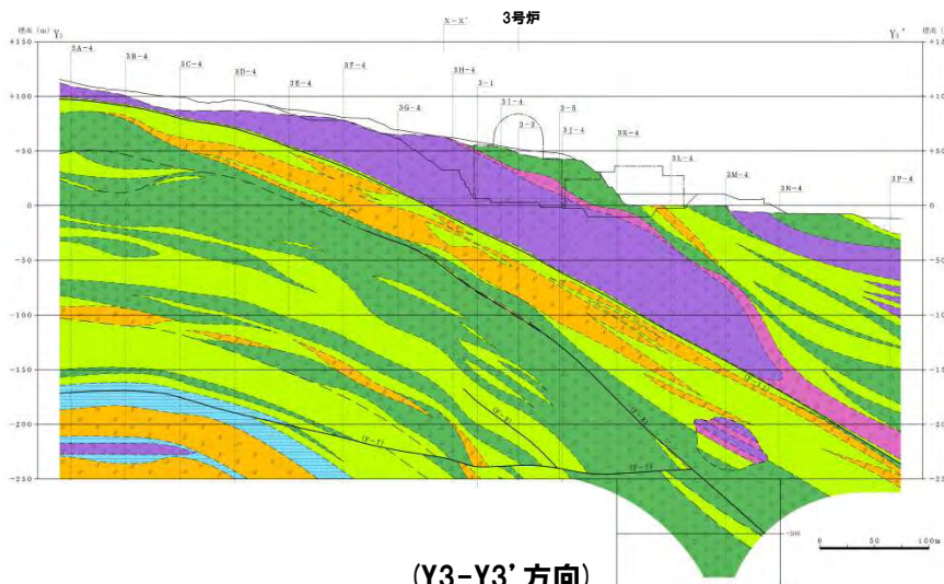
地質断面図 (Y-Y' 方向)
