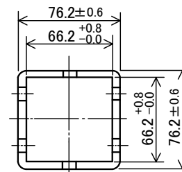
断面 CC
