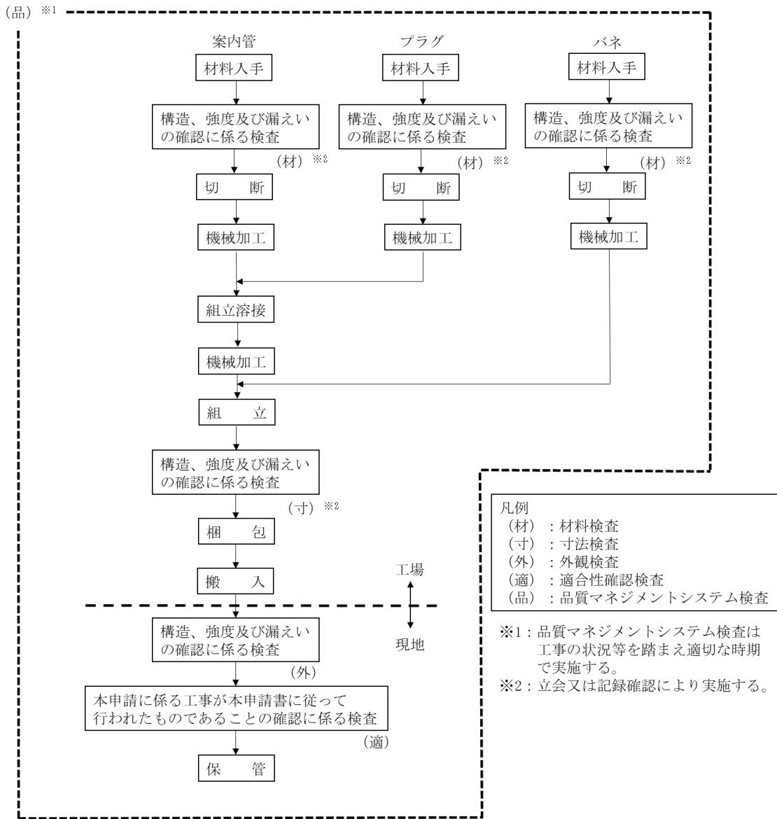
図-2 製作及び工事のフロー
