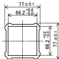
断面 B1 B1
