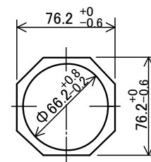
断面 EE
