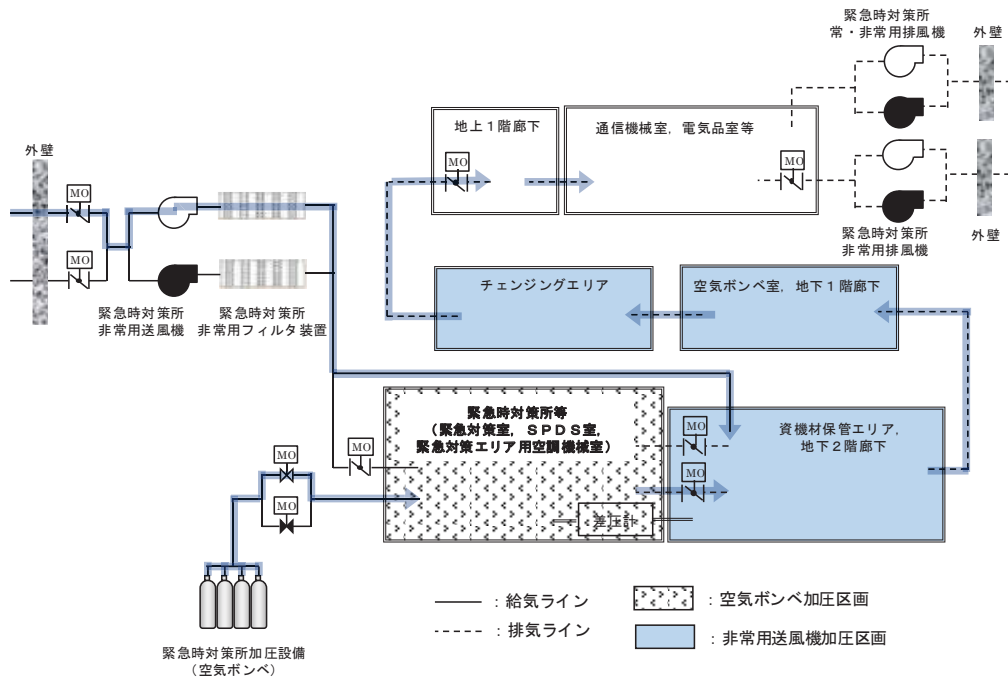
図3-4 放射性雲通過時の緊急時対策所換気空調系等概要図
