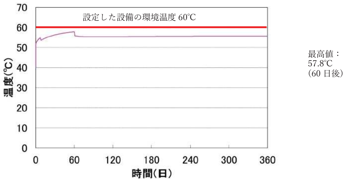
図3-1 HPCWポンプ室の室温評価結果
