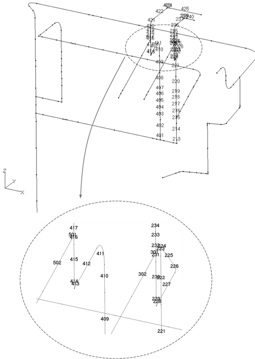
第 3.96 図 貫通部配管 P106(CV 内)の解析モデル図(要素番号 3)
