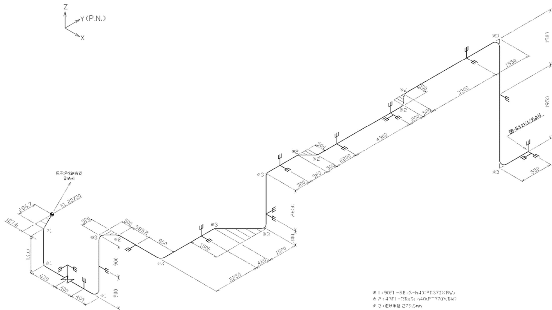
第 3.114 図 貫通部配管 P112(CV 外)のアイソメ図 2
