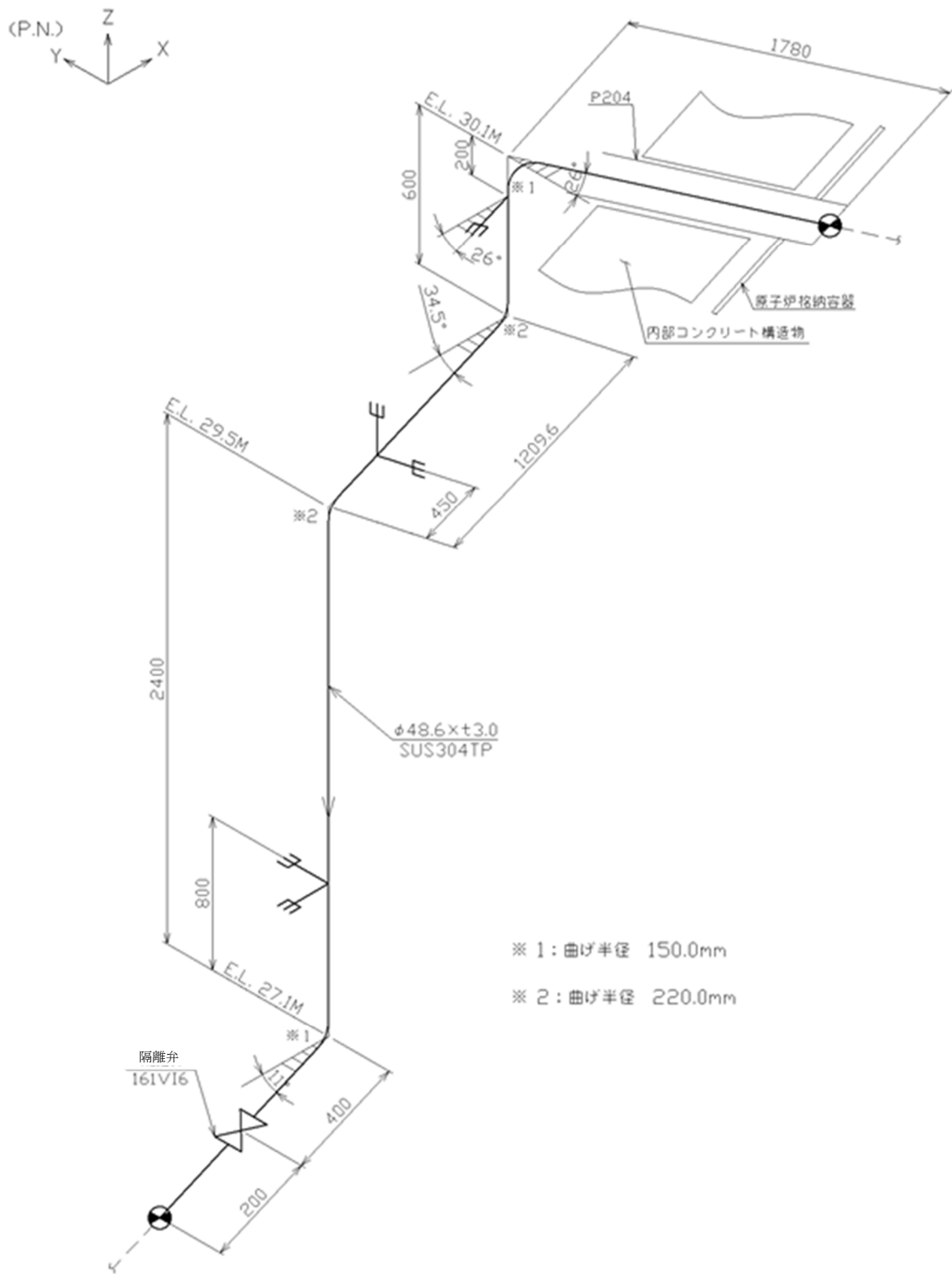
第 3.55 図 貫通部配管 P204(CV 内)のアイソメ図
