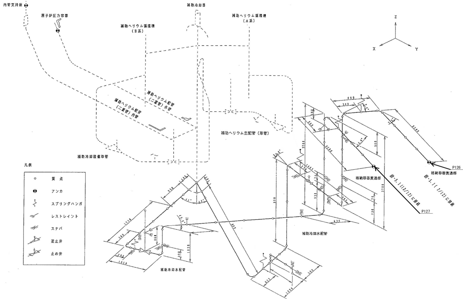
第 3.154 図 貫通部配管 P126 (CV 内) のアイソメ図
