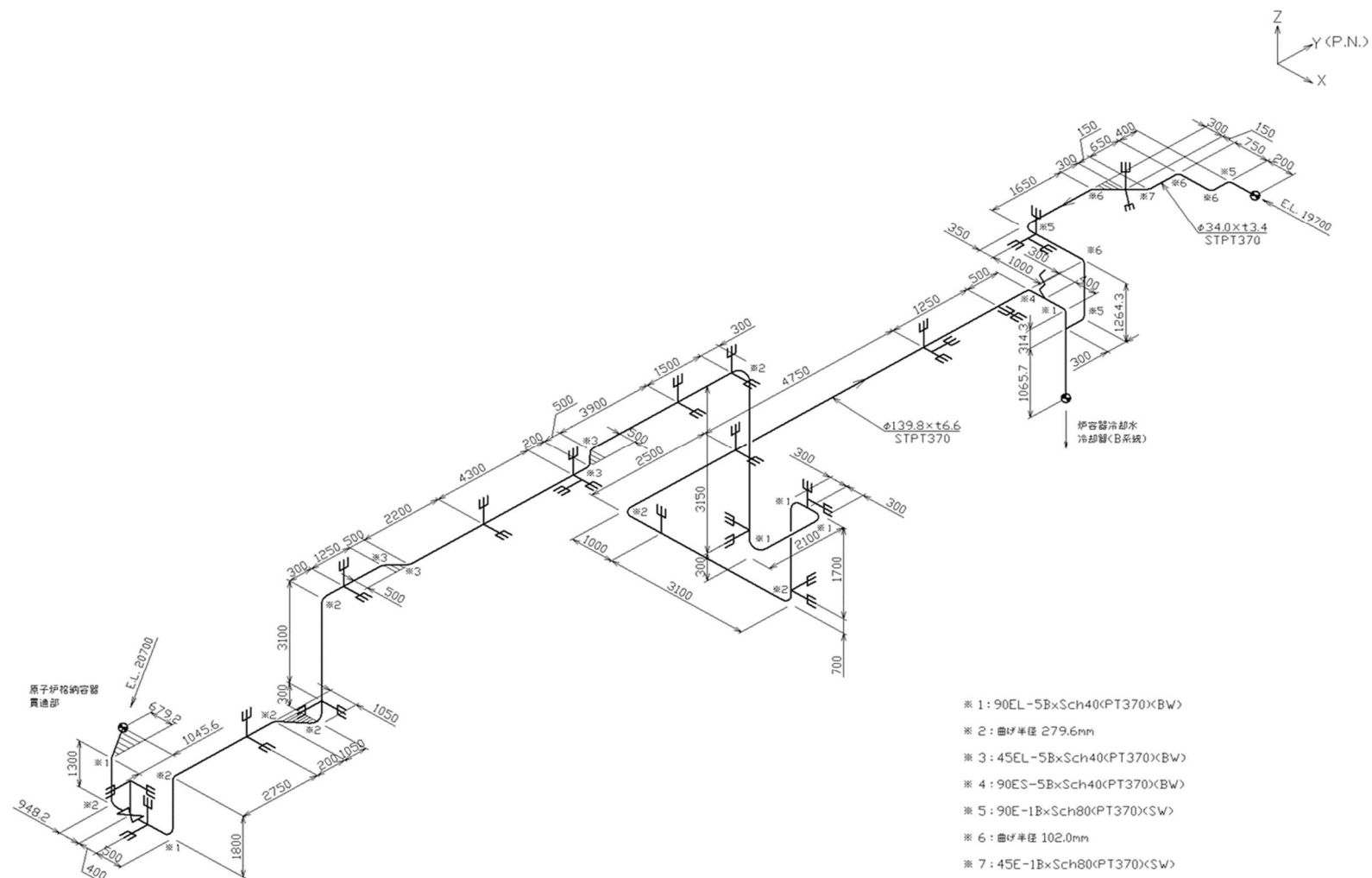
第 3.97 図 貫通部配管 P111 (CV 外) のアイソメ図
