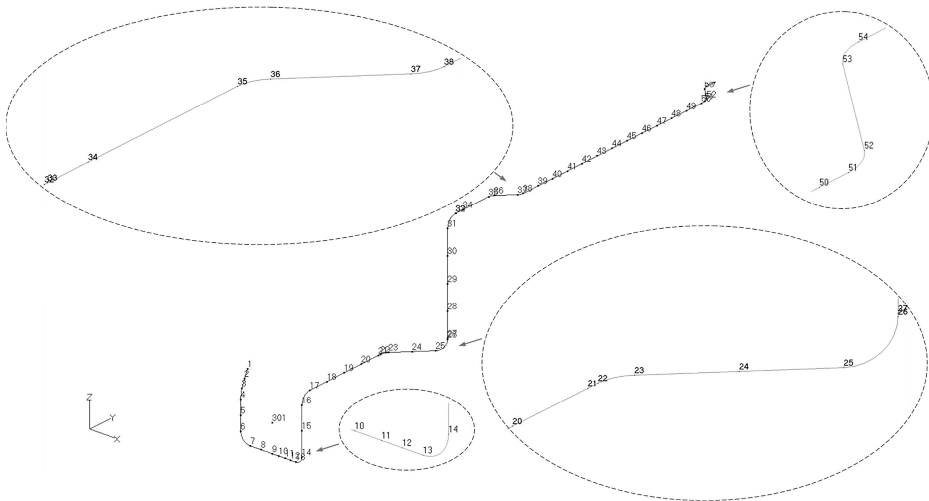
第 3.99 図 貫通部配管 P111 (CV 外) の解析モデル図 (節点番号 1)
