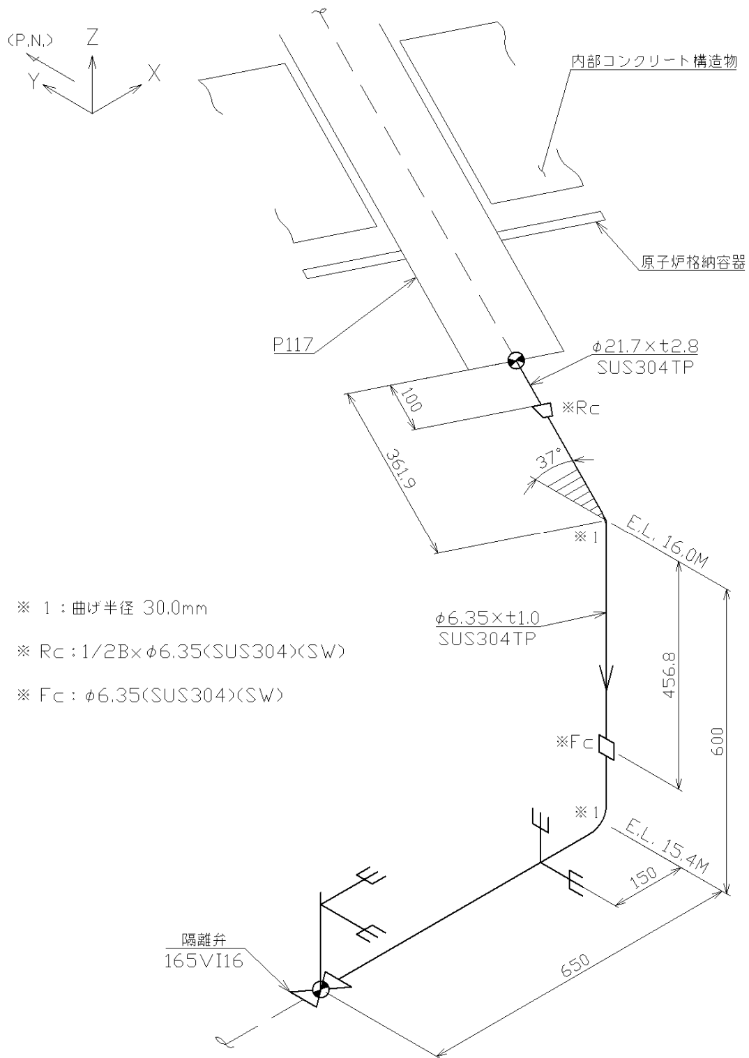
第 3.27 図 貫通部配管 P117 (CV 外) のアイソメ図
