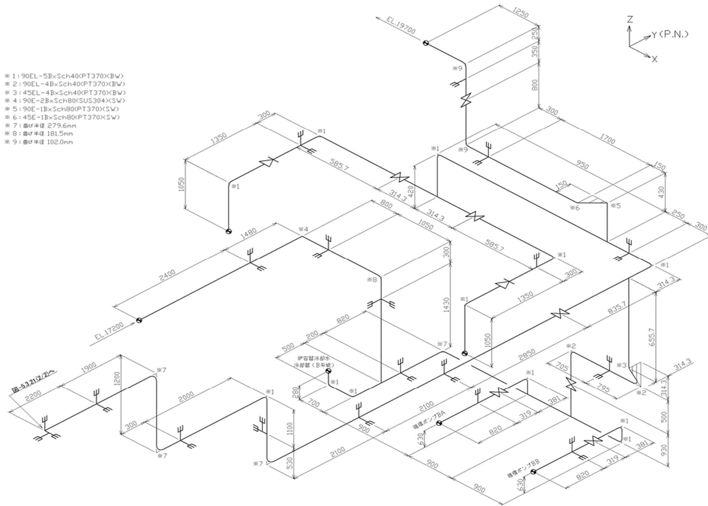
第 3.113 図 貫通部配管 P112(CV 外)のアイソメ図 1
