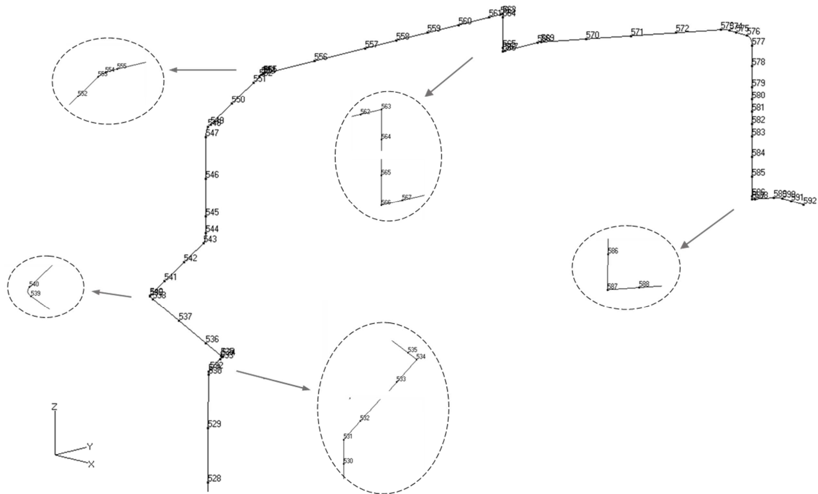
第 3.126 図 貫通部配管 P112 (CV 内) の解析モデル図 (節点番号 3)
