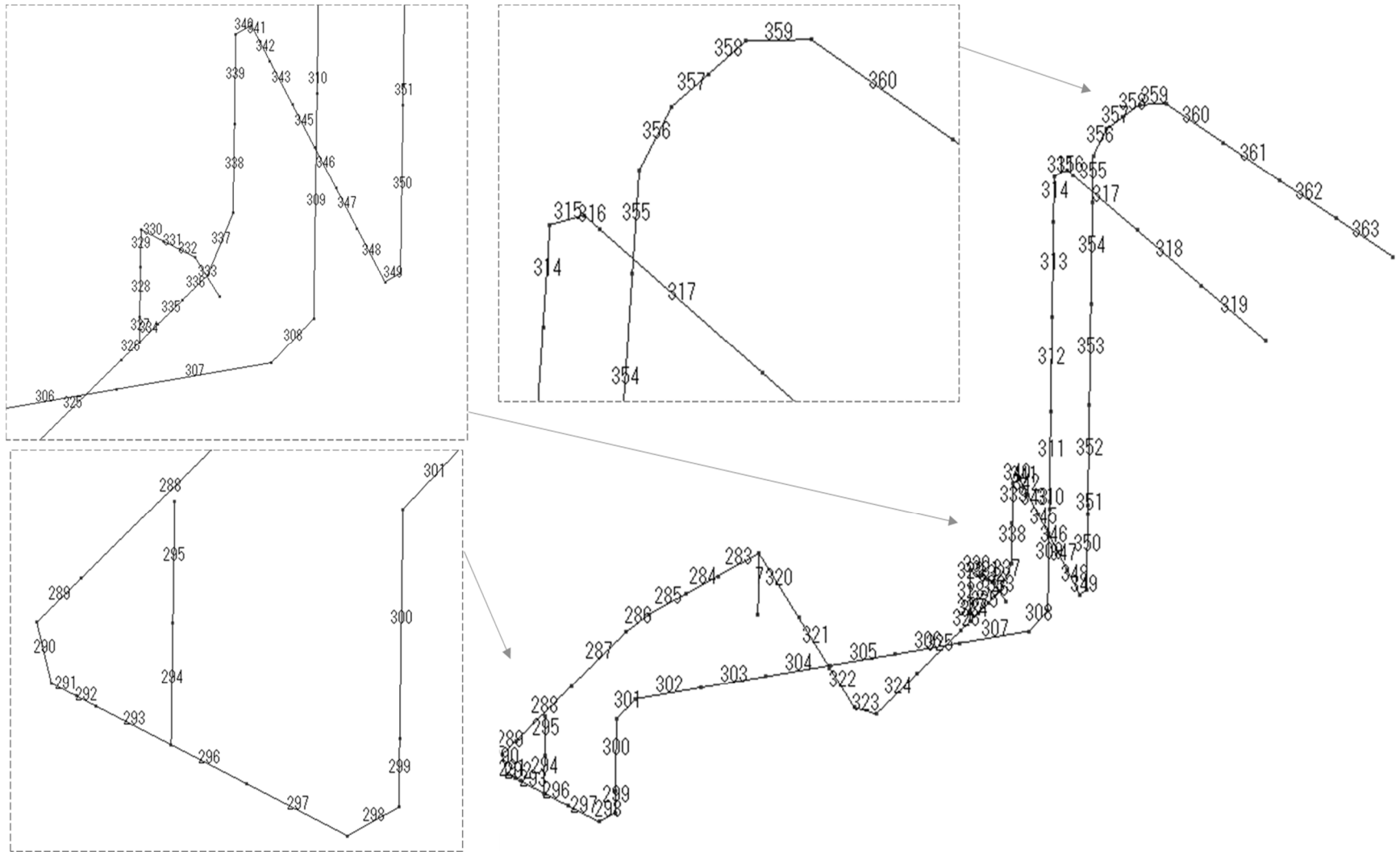
第 3.156 図 貫通部配管 P126(CV 内)の解析モデル図(要素番号)
