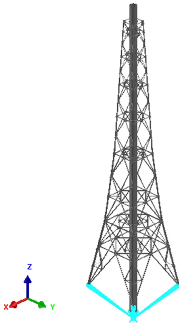
第 3.1 図 H T T R 排気筒メッシュモデル
