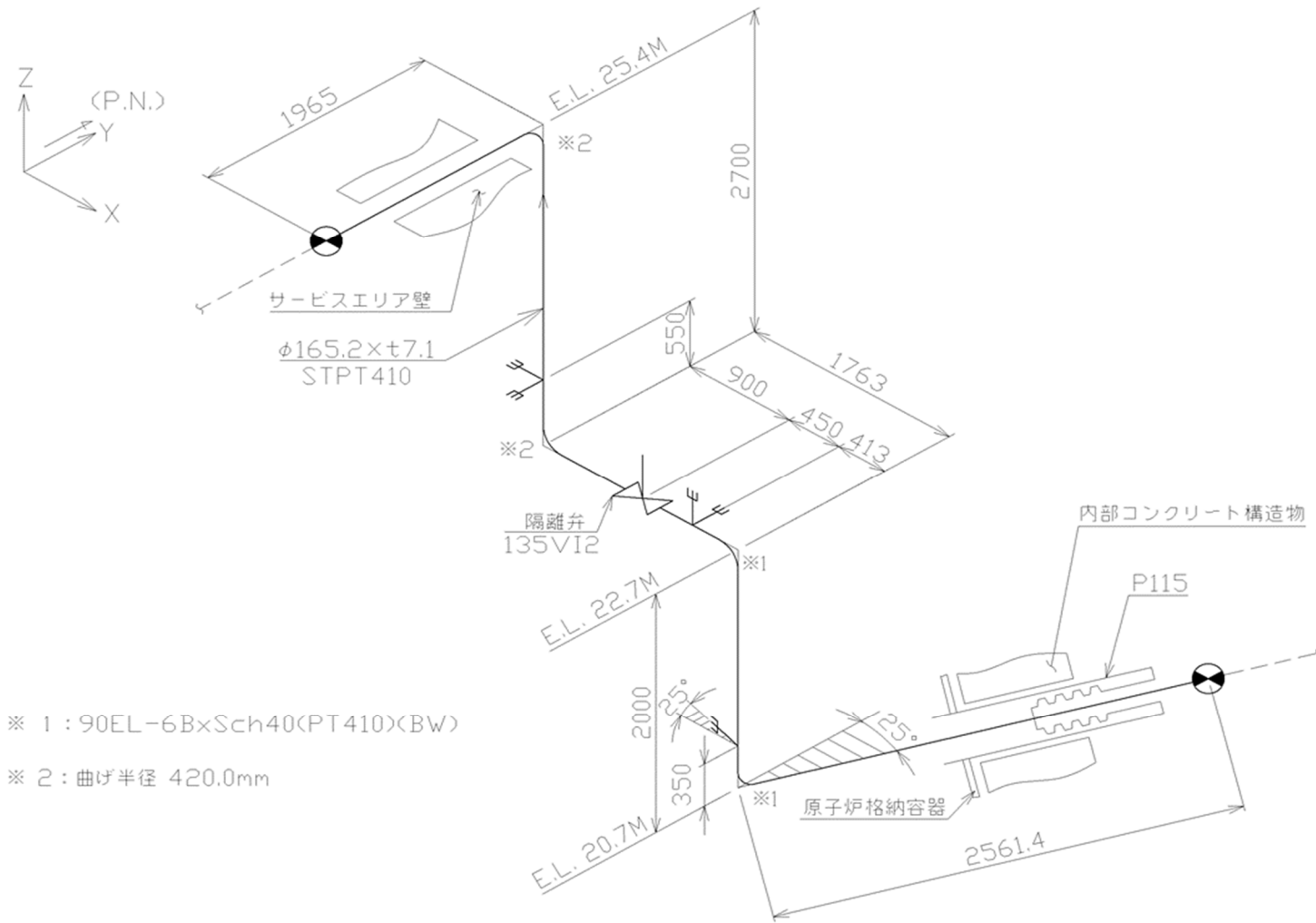
第 3. 131 図 貫通部配管 P115(CV 外) のアイソメ図
