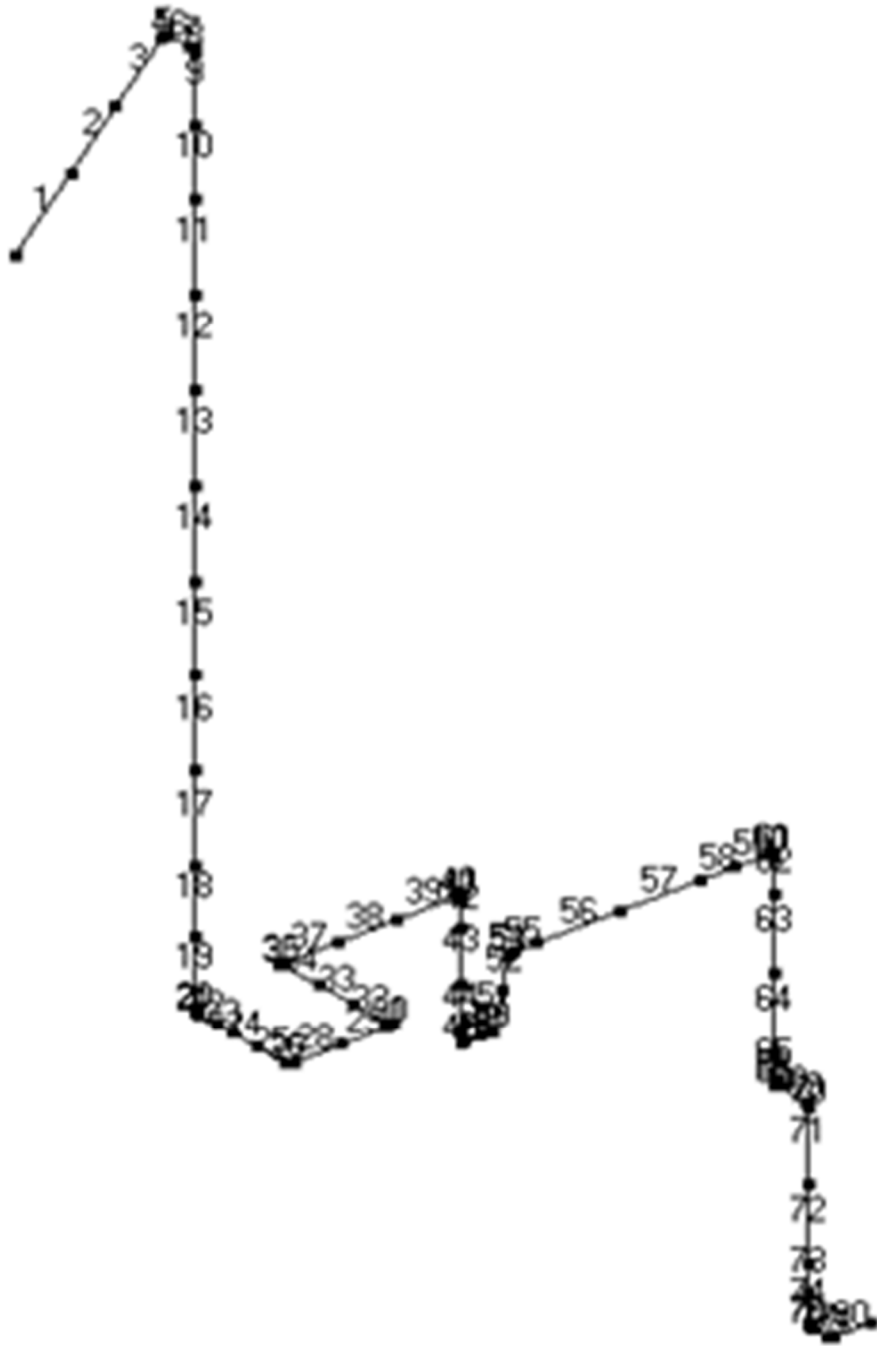
第 3.14 図 貫通部配管 P108 (CV 外) の解析モデル図 (要素番号)
