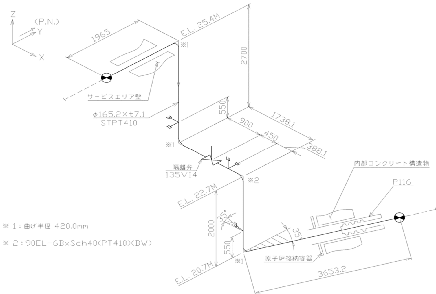
第 3.134 図 貫通部配管 P116(CV 外)のアイソメ図
