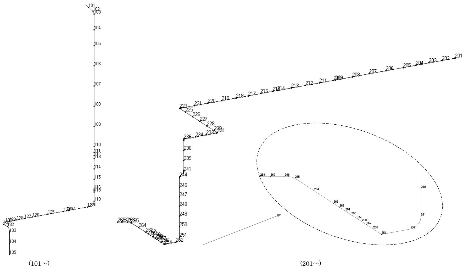
第 3.61 図 貫通部配管 P102(CV 外)の解析モデル図(節点番号 2)
