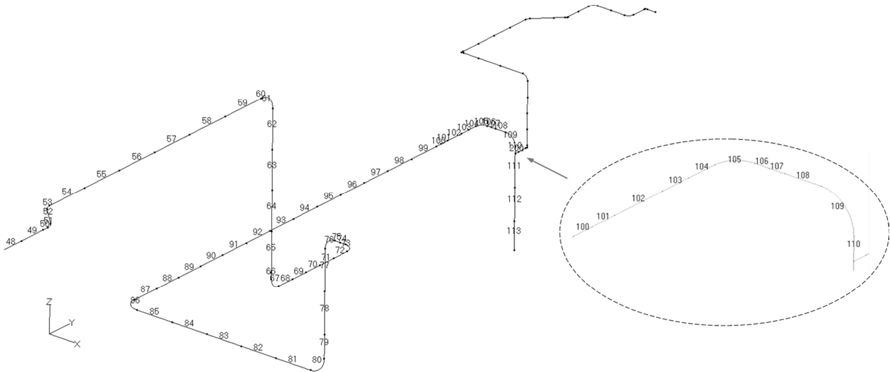
第 3.102 図 貫通部配管 P111 (CV 外) の解析モデル図 (要素番号 2)
