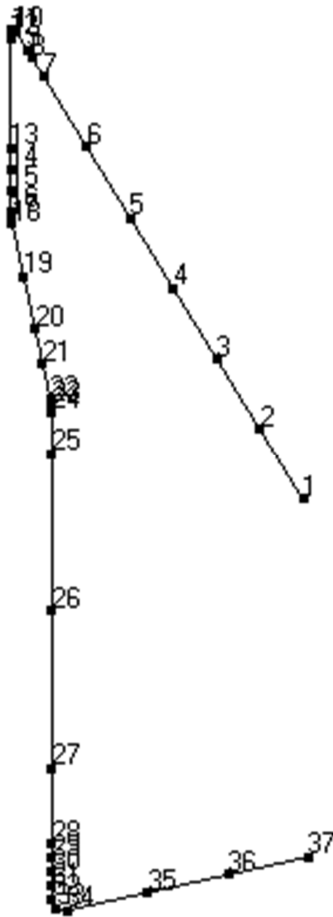
第 3.37 図 貫通部配管 P118 その 1(CV 内)の解析モデル図(節点番号)
