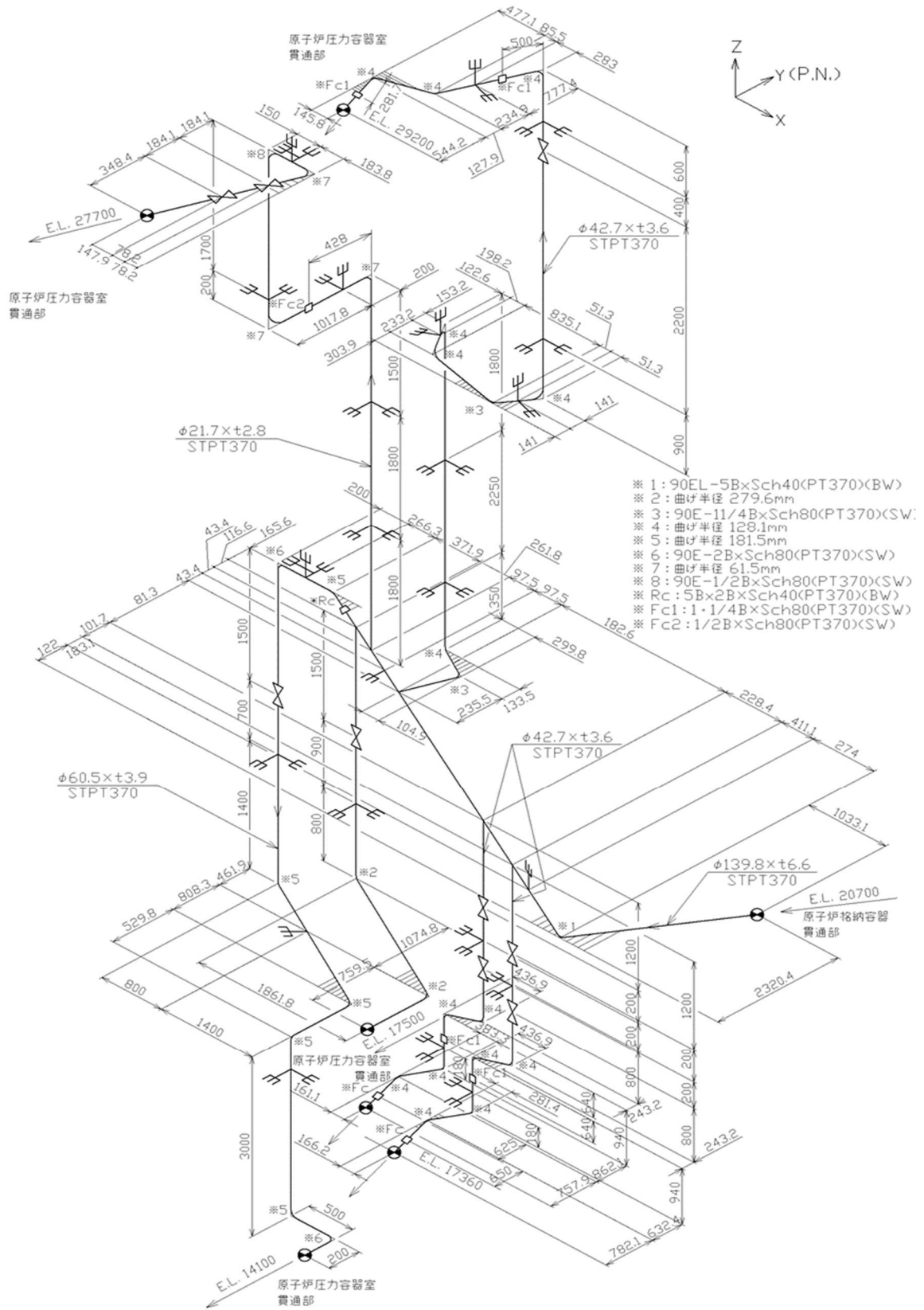
第 3.80 図 貫通部配管 P105(CV 内)のアイソメ図
