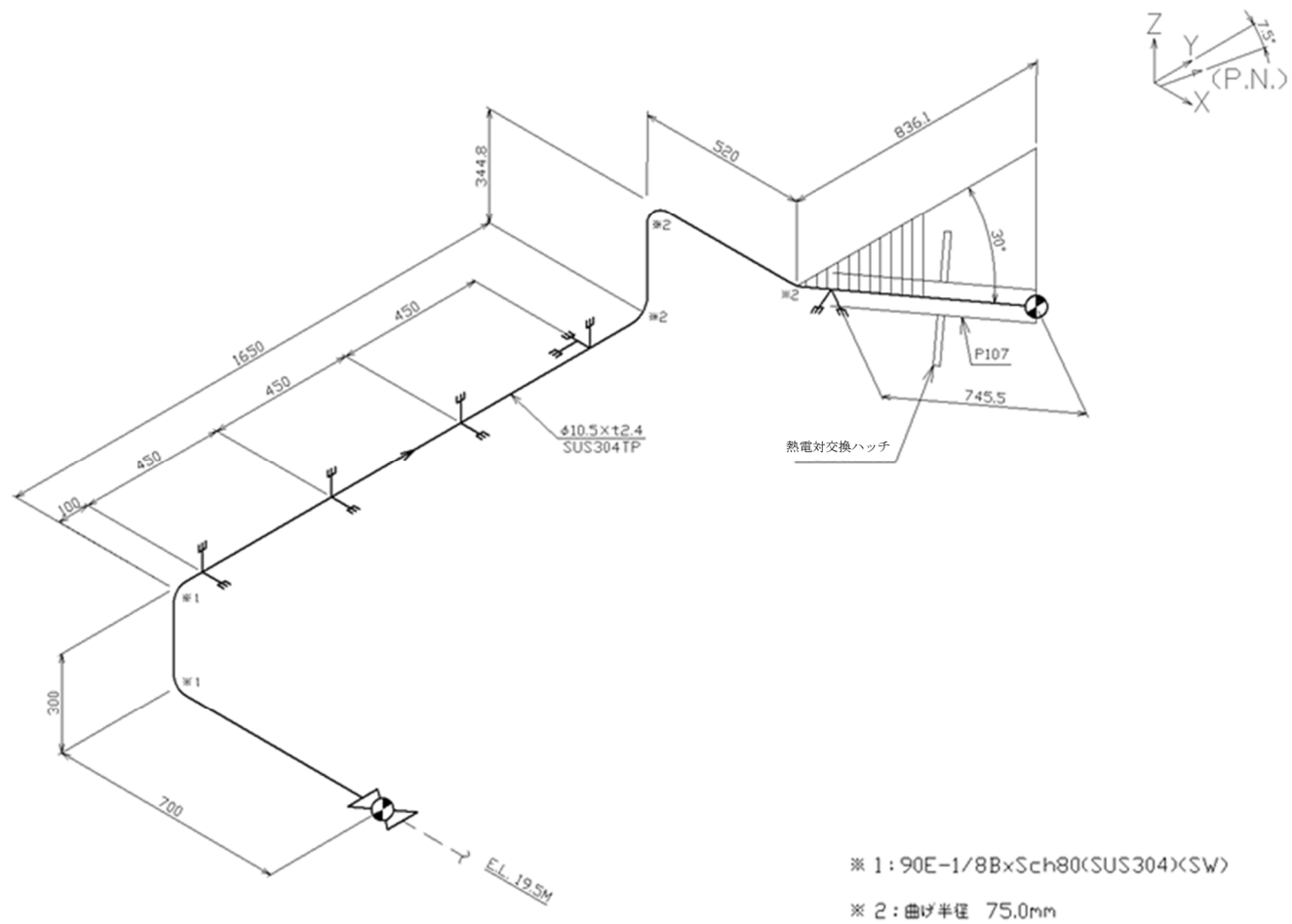
第 3.9 図 貫通部配管 P107 (CV 内) のアイソメ図
