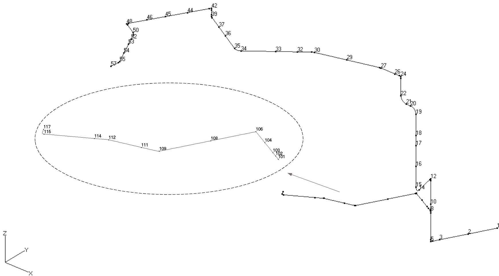
第 3.64 図 貫通部配管 P102 (CV 内) の解析モデル図 (節点番号)
