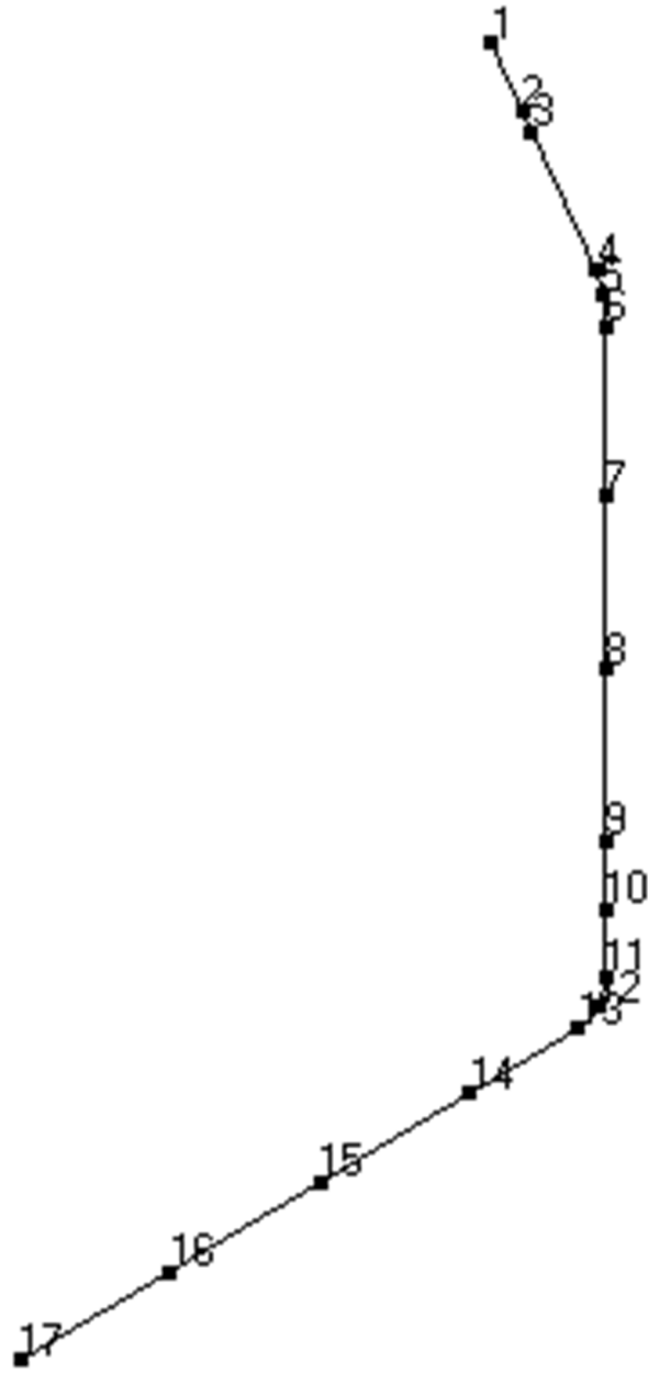
第 3.28 図 貫通部配管 P117 (CV 外) の解析モデル図 (節点番号)
