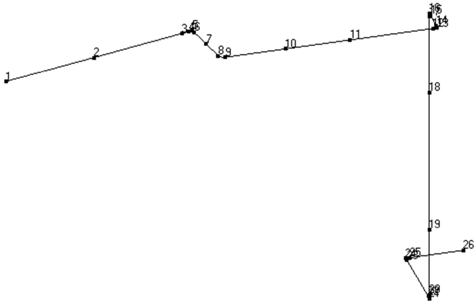
第 3.129 図 貫通部配管 P114(CV 内)の解析モデル図(節点番号)
