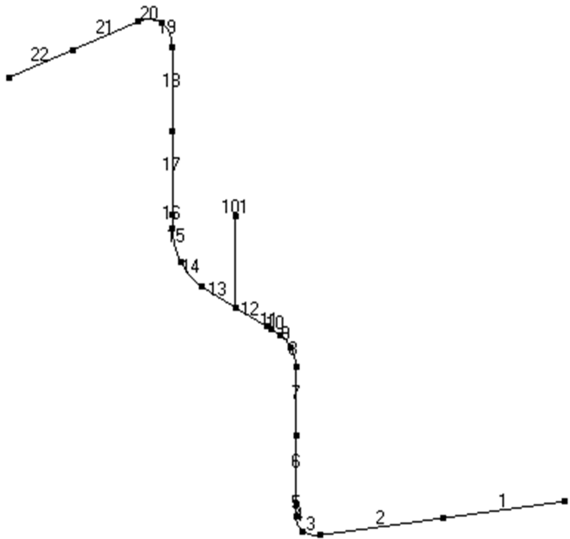
第 3. 133 図 貫通部配管 P115 (CV 外) の解析モデル図 (要素番号)
