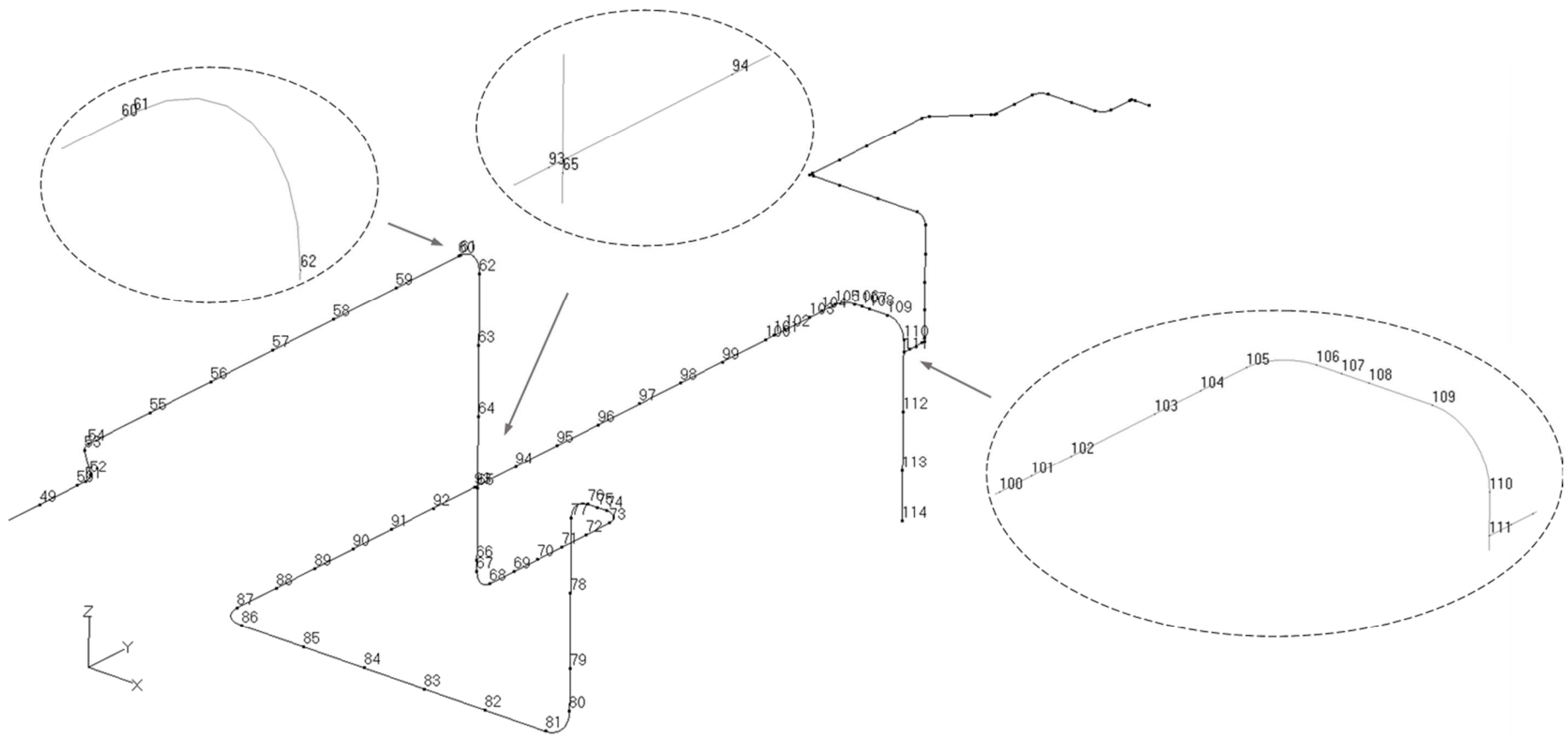
第 3.101 図 貫通部配管 P111 (CV 外) の解析モデル図 (節点番号 2)
