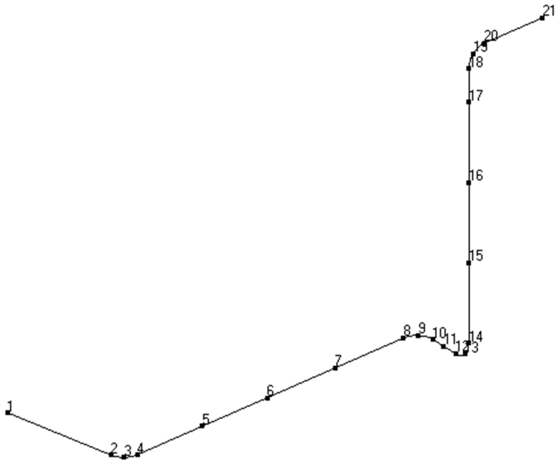
第 3.170 図 貫通部配管 P206 (CV 外) の解析モデル図 (節点番号)
