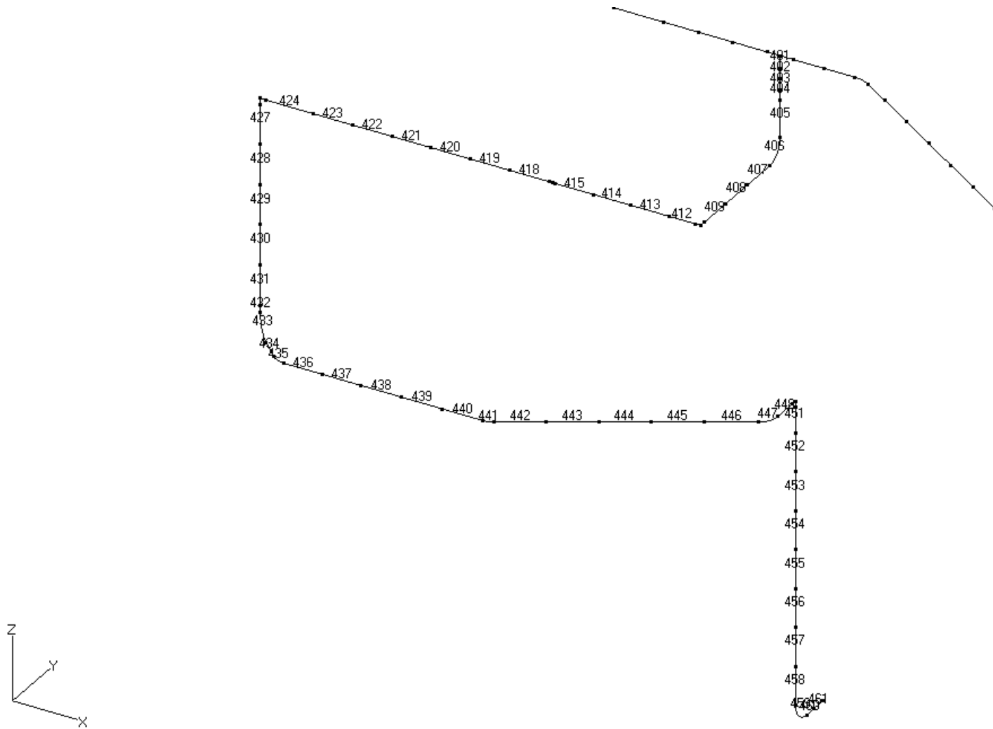
第 3.110 図 貫通部配管 P111 (CV 内) の解析モデル図 (要素番号 2)
