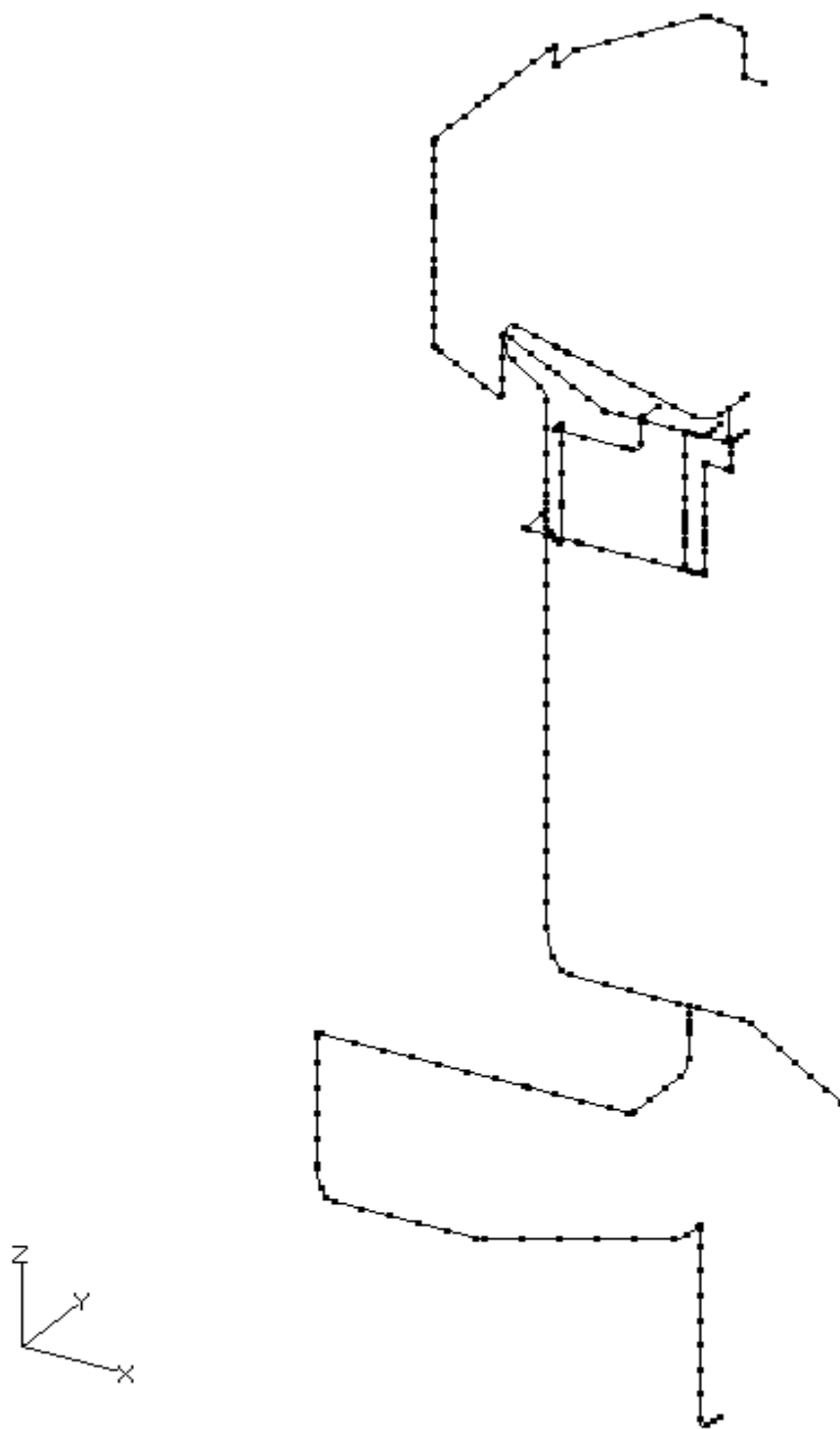
第 3.106 図 貫通部配管 P111(CV 内)の解析モデル図(全体)
