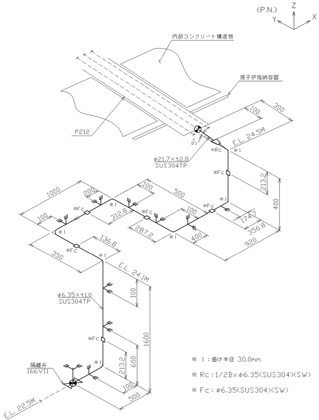
第 3.183 図 貫通部配管 P212 その 1 (CV 外) のアイソメ図
