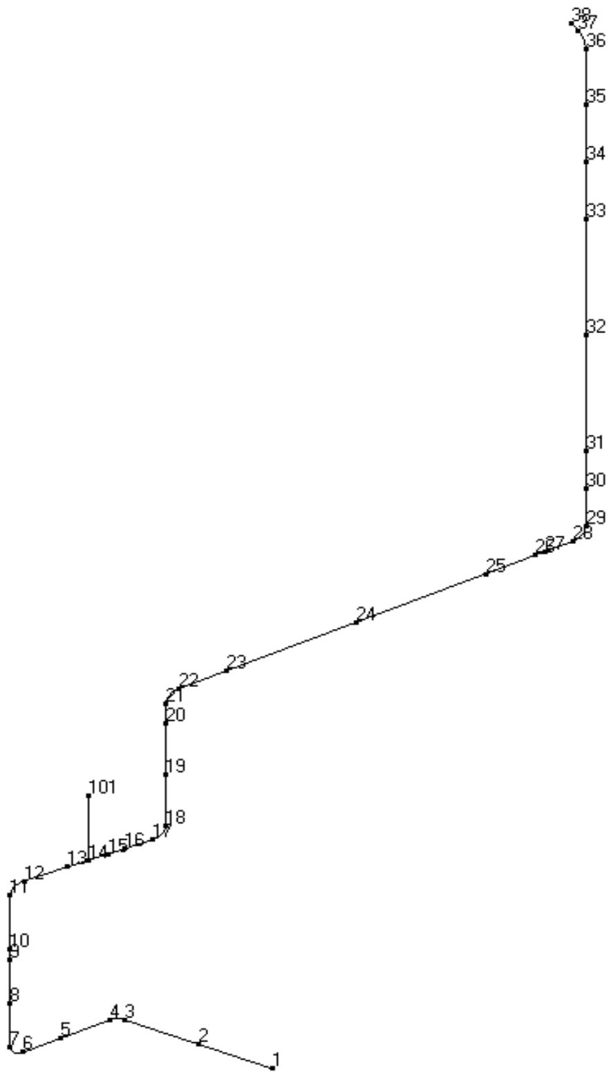
第 3.152 図 貫通部配管 P126 (CV 外) の解析モデル図 (節点番号)
