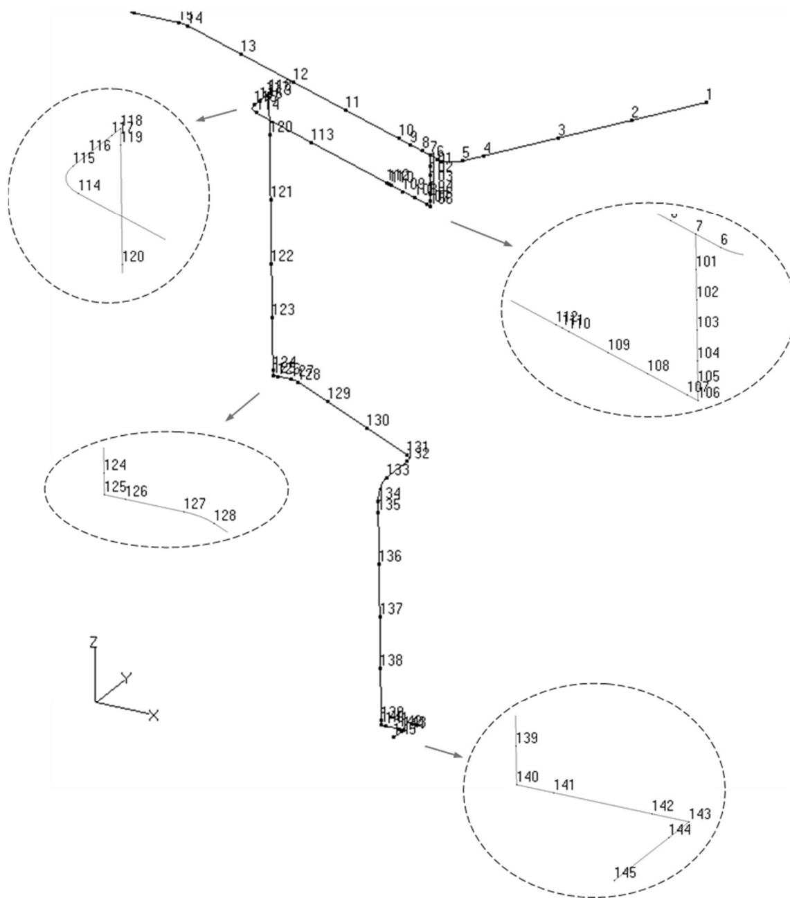
第 3.91 図 貫通部配管 P106(CV 内)の解析モデル図(節点番号 1)
