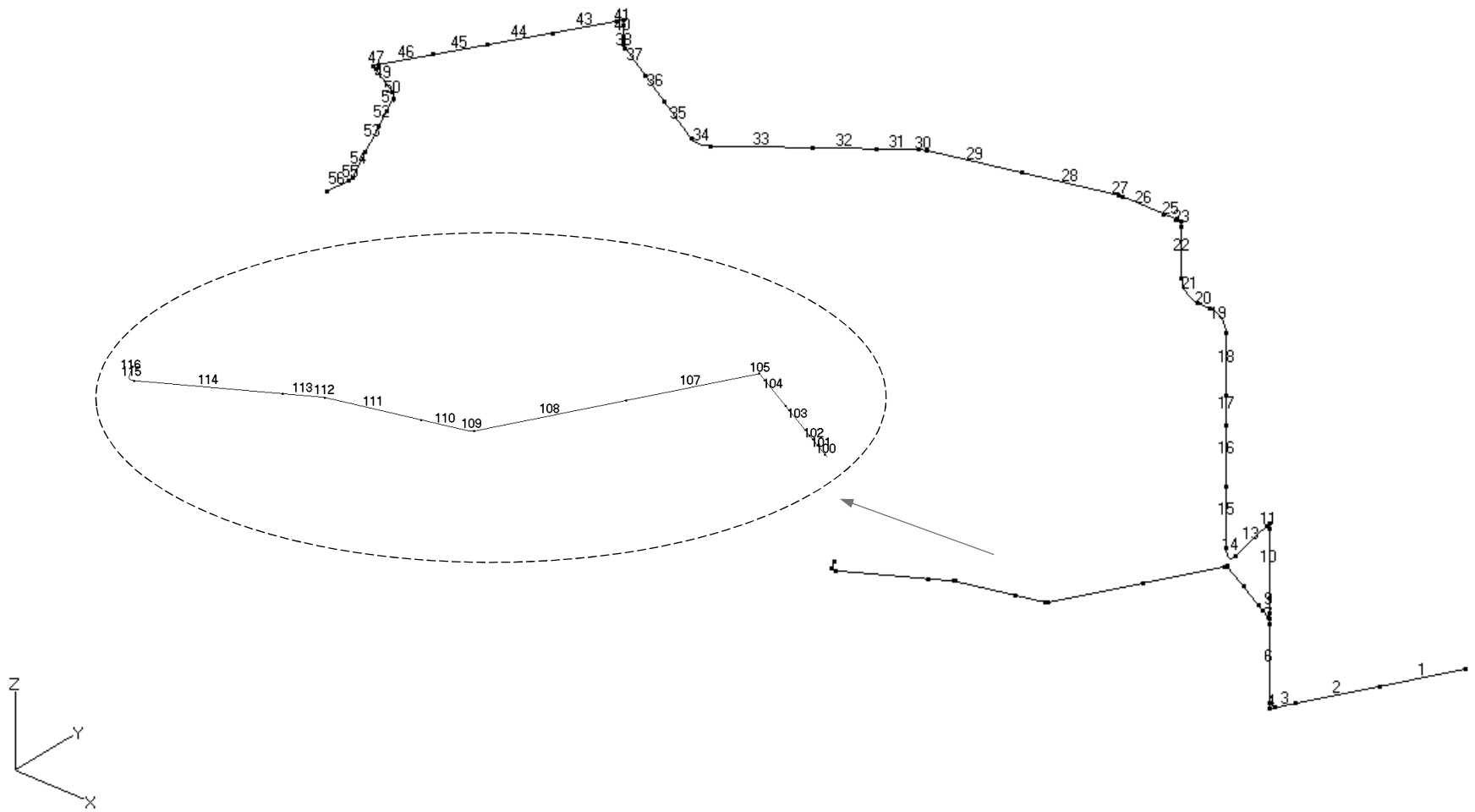
第 3. 65 図 貫通部配管 P102 (CV 内) の解析モデル図 (要素番号)
