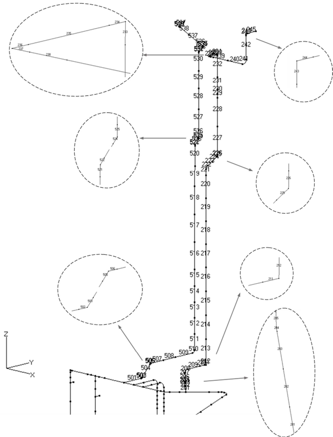
第 3.125 図 貫通部配管 P112(CV 内)の解析モデル図(要素番号 2)
