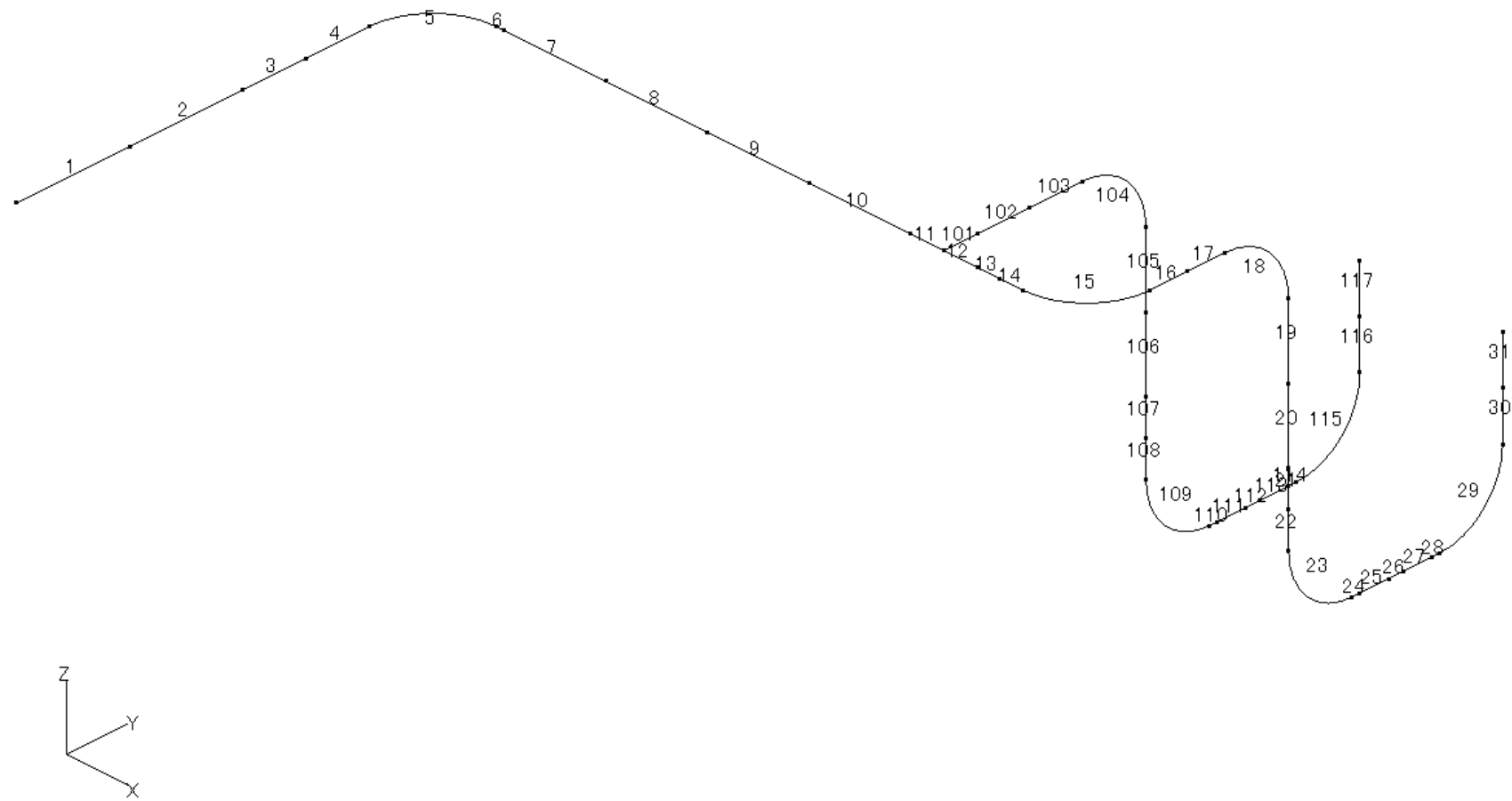
第 3.206 図 非常用空気浄化設備主ダクトの解析モデル図(要素番号)
