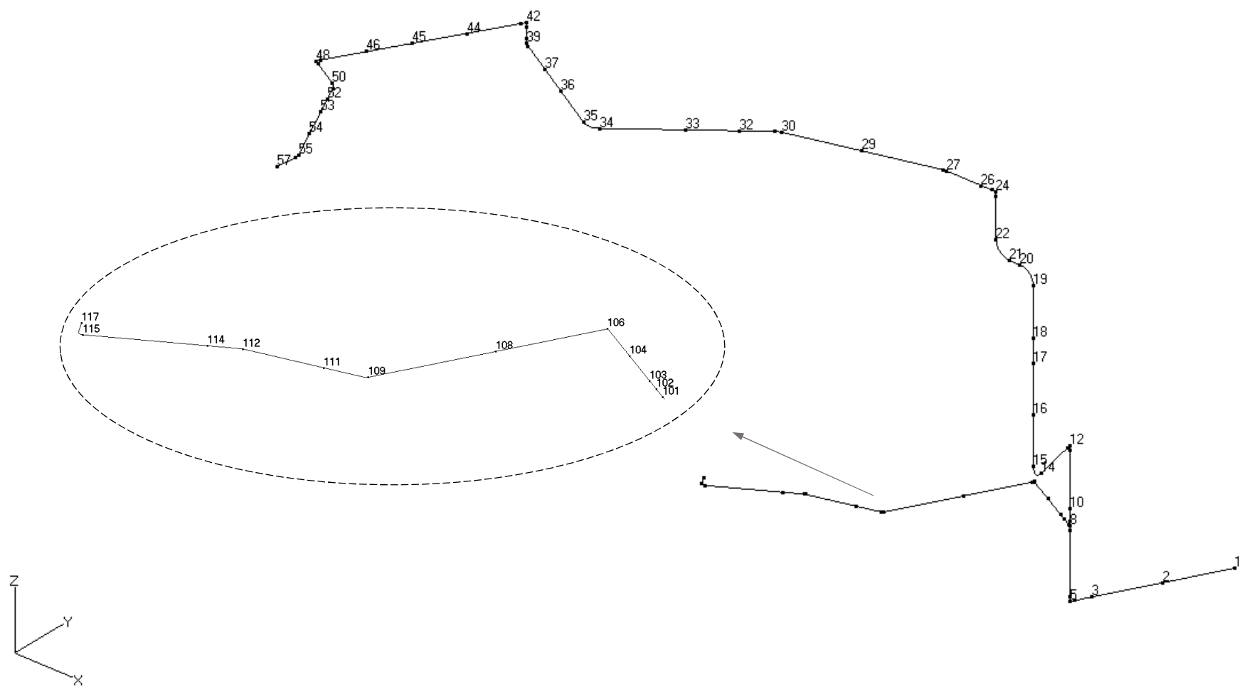
第 3.72 図 貫通部配管 P103 (CV 内) の解析モデル図 (節点番号)
