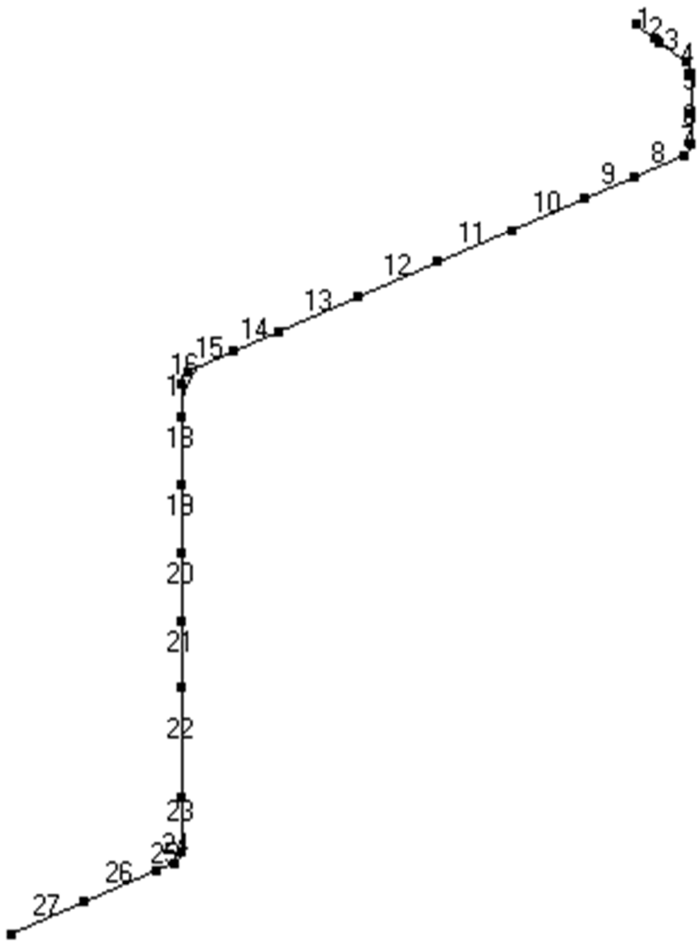
第 3.188 図 貫通部配管 P212 その 3(CV 外)の解析モデル図(要素番号)
