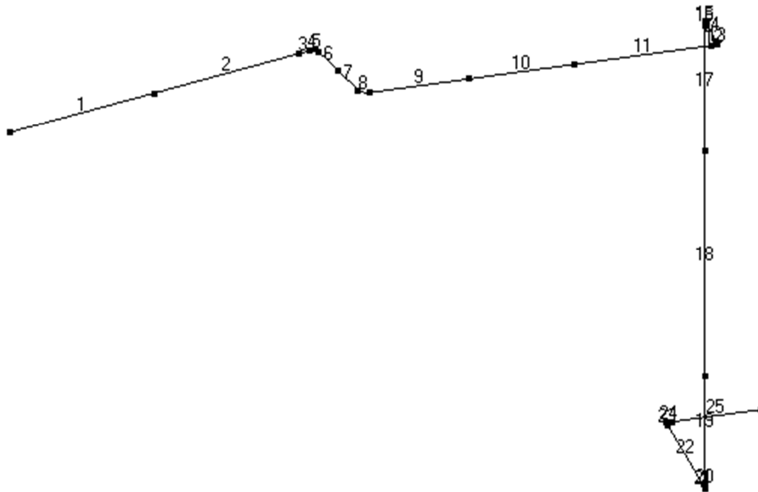
第 3.130 図 貫通部配管 P114(CV 内)の解析モデル図(要素番号)
