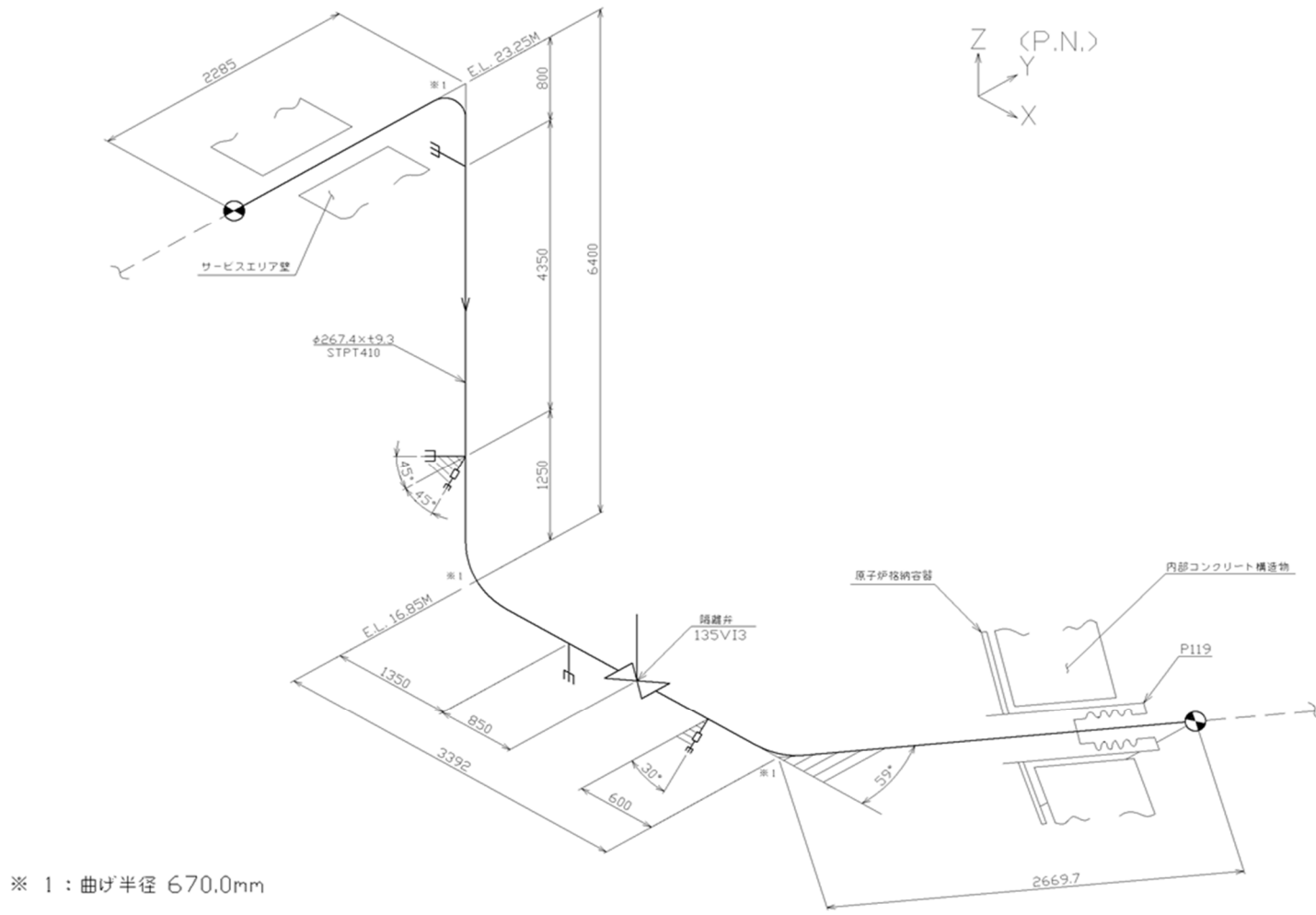
第 3.137 図 貫通部配管 P119(CV 外)のアイソメ図
