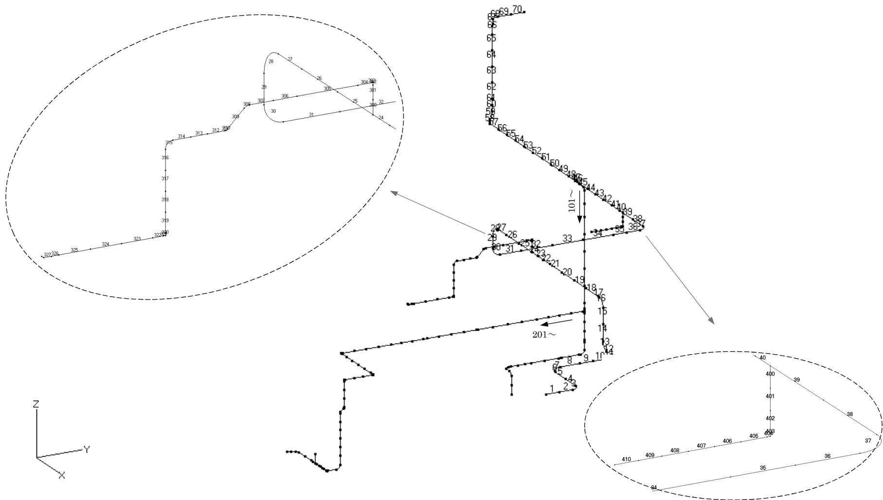
第 3.60 図 貫通部配管 P102(CV 外)の解析モデル図(要素番号 1)
