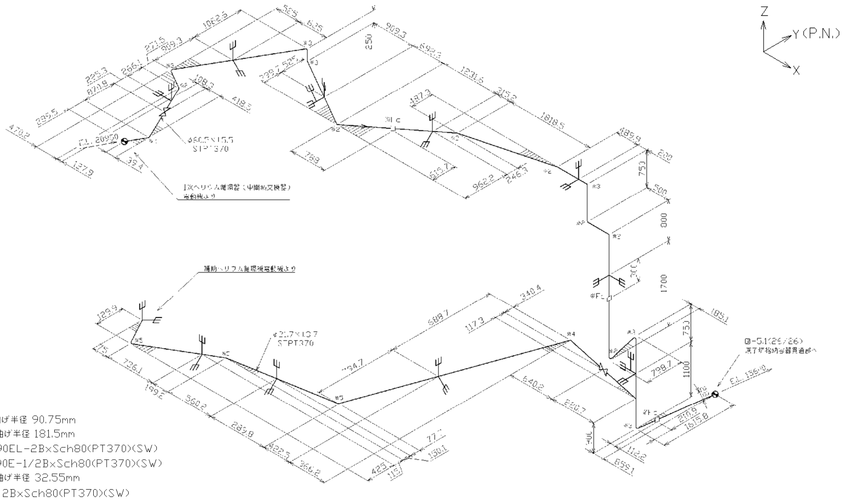
第 3.63 図 貫通部配管 P102(CV 内)のアイソメ図
