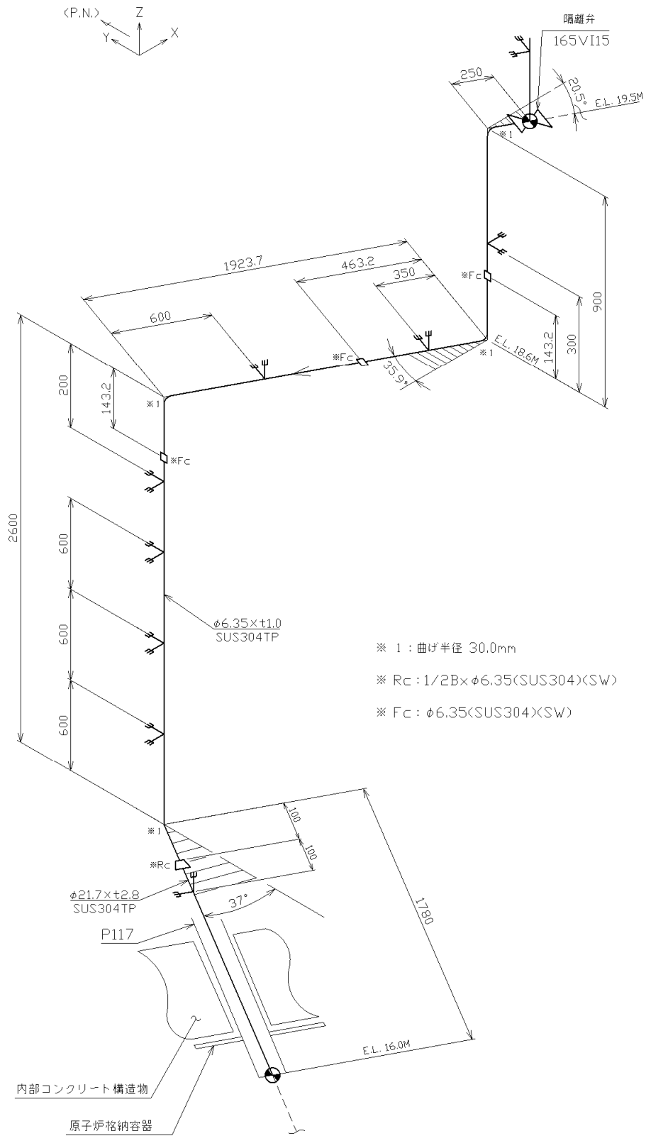
第 3.30 図 貫通部配管 P117(CV 内)のアイソメ図
