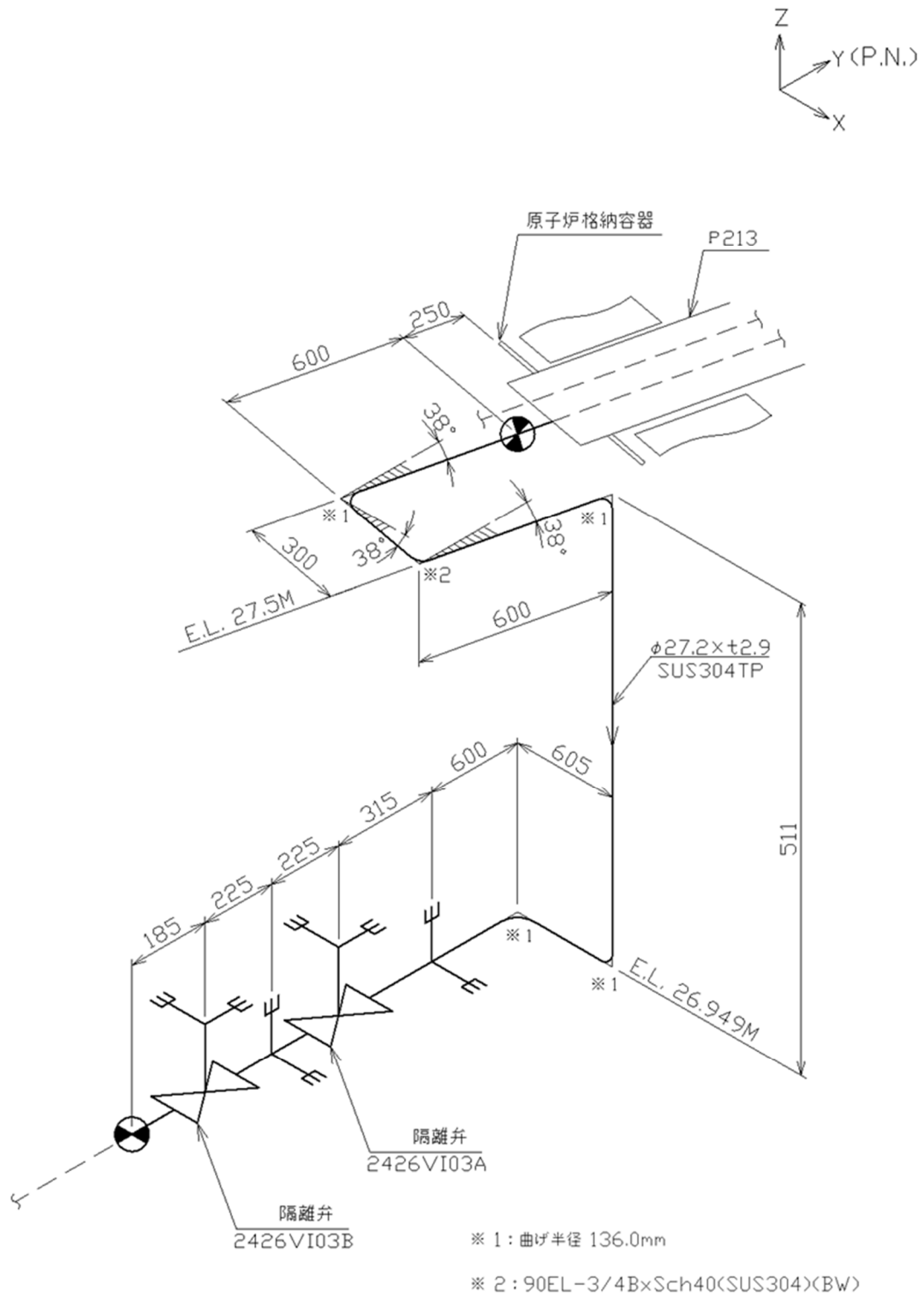
第 3.189 図 貫通部配管 P213 その 1 (CV 外) のアイソメ図
