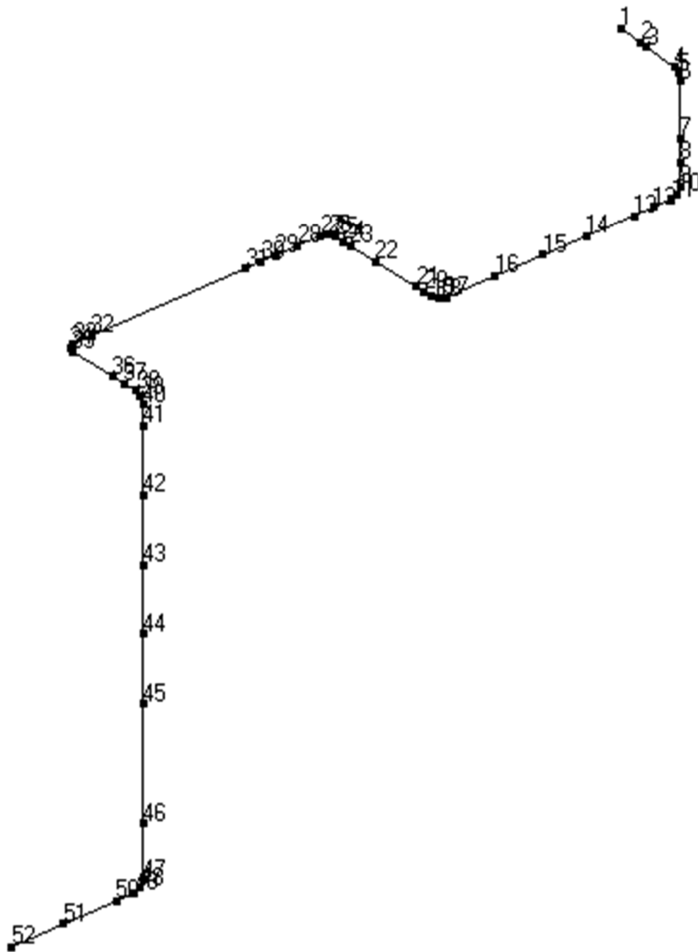
第 3.184 図 貫通部配管 P212 その 1(CV 外)の解析モデル図(節点番号)
