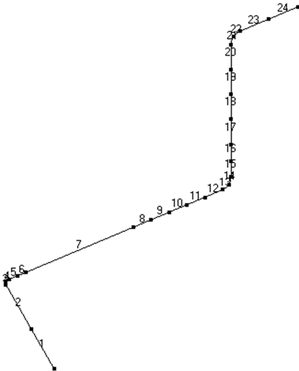
第 3.76 図 貫通部配管 P104 (CV 外) の解析モデル図 (要素番号)
