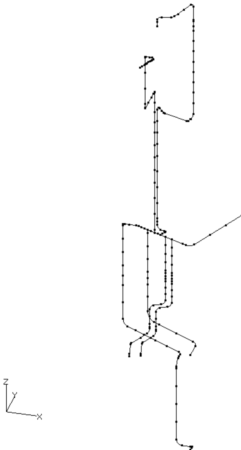
第 3.81 図 貫通部配管 P105 (CV 内) の解析モデル図 (全体)
