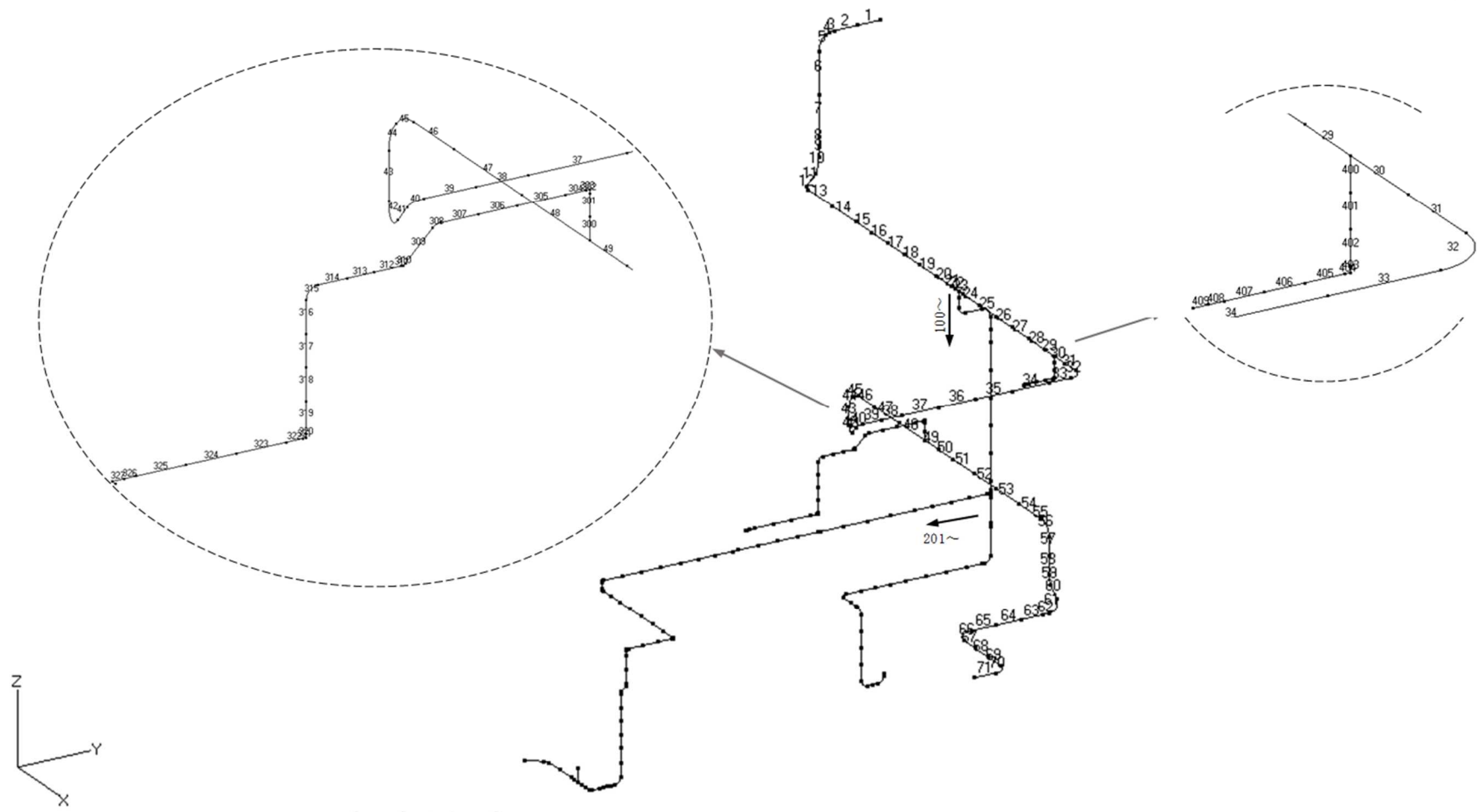
第 3.68 図 貫通部配管 P103(CV 外)の解析モデル図(要素番号 1)
