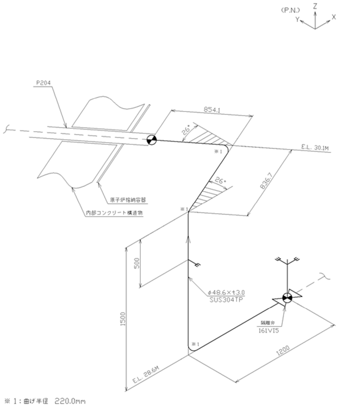
第 3.53 図 貫通部配管 P204(CV 外)のアイソメ図
