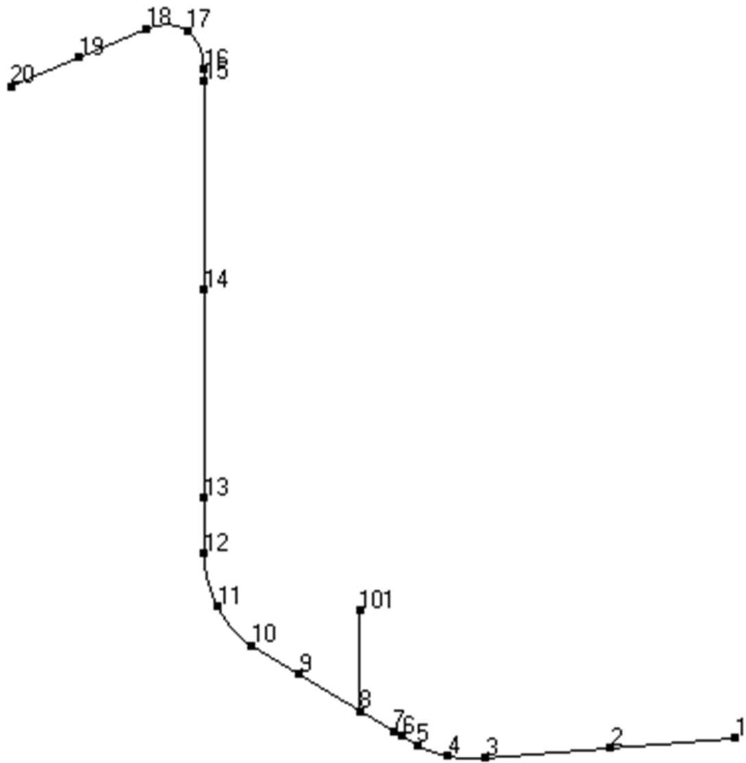
第 3. 138 図 貫通部配管 P119 (CV 外) の解析モデル図 (節点番号)
