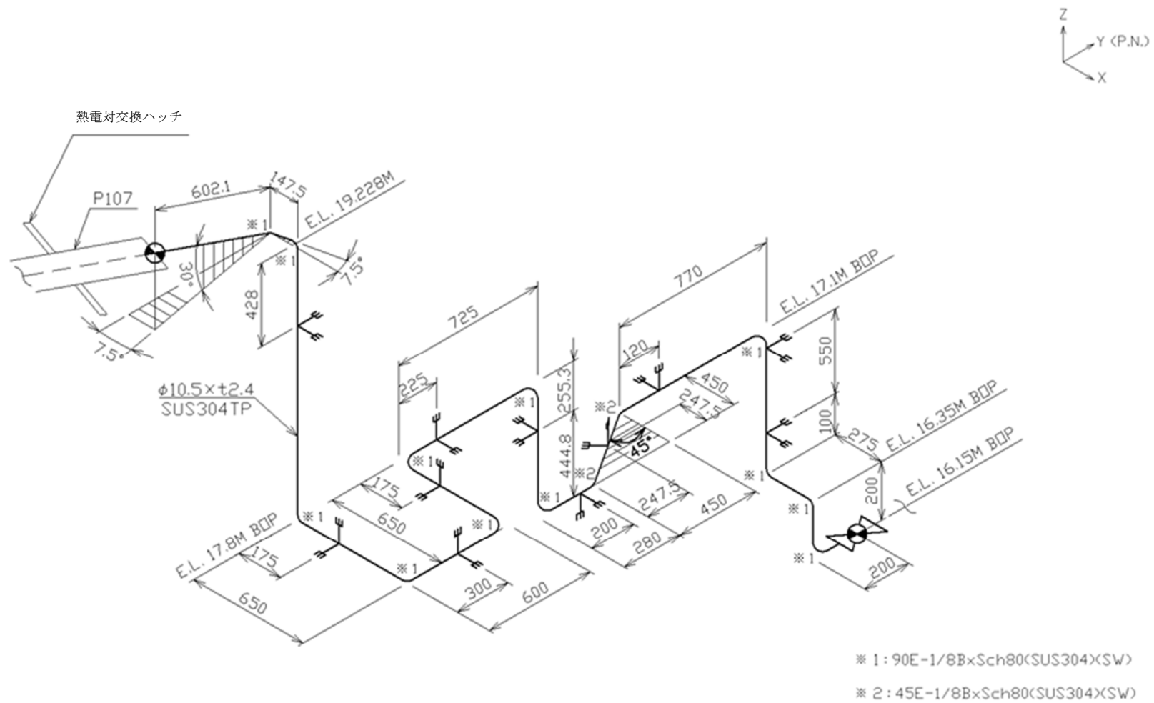
第 3.6 図 貫通部配管 P107 (CV 外) のアイソメ図
