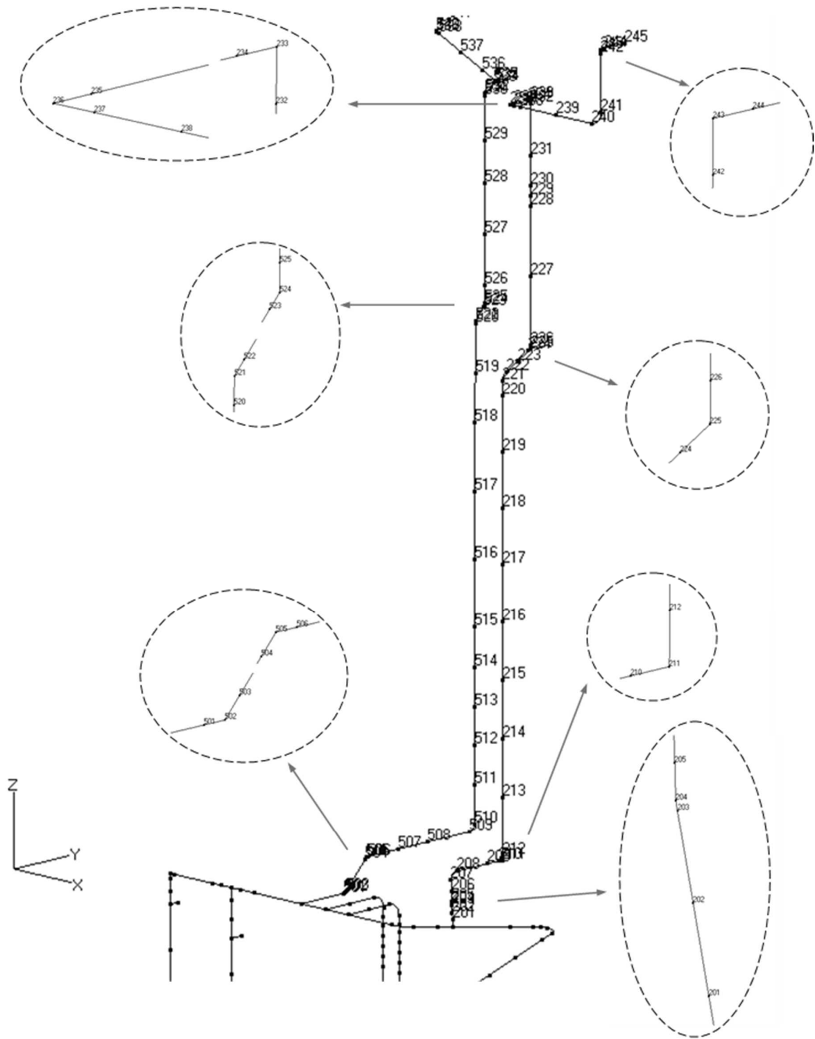
第 3.124 図 貫通部配管 P112(CV 内)の解析モデル図(節点番号 2)
