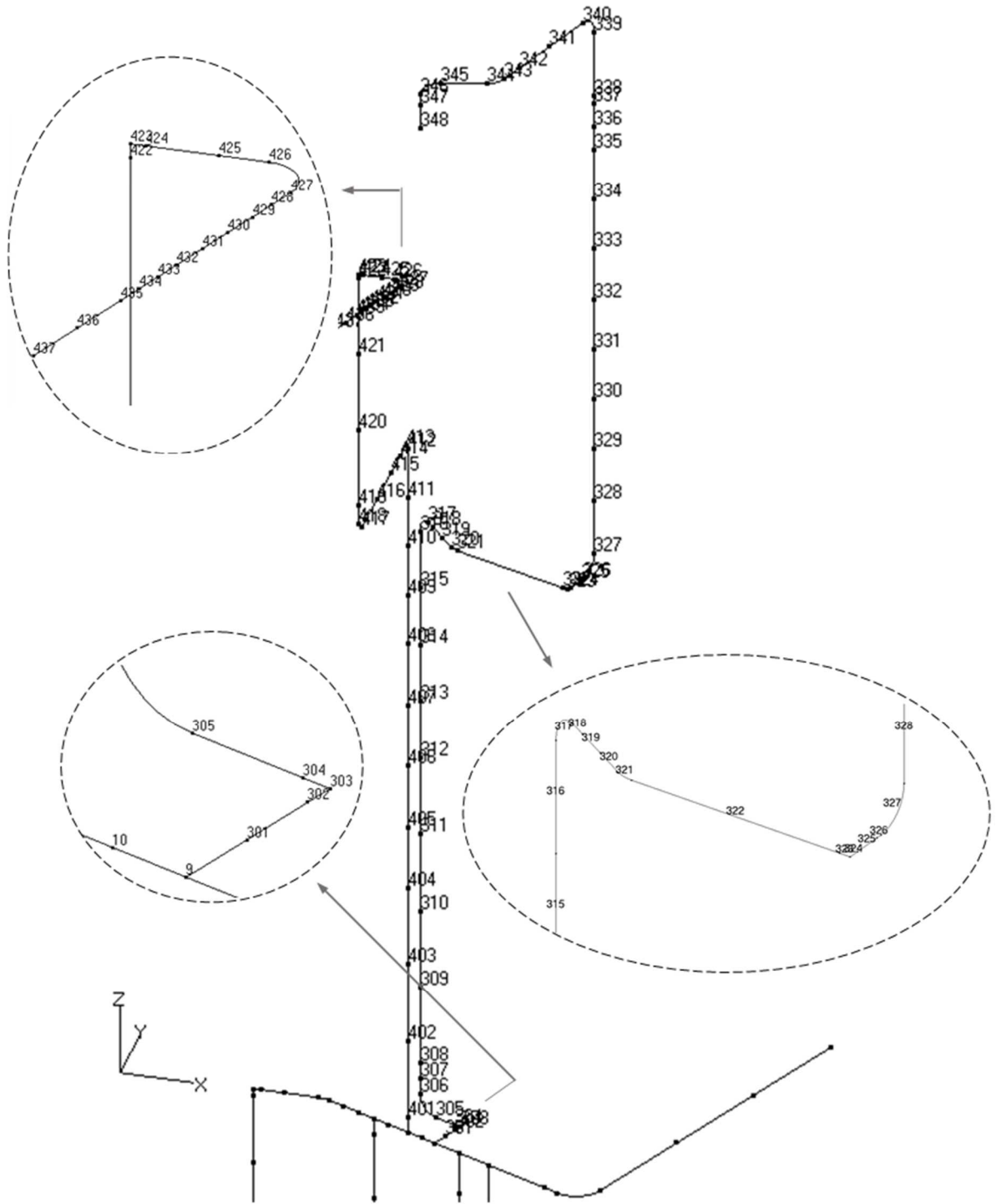
第 3.84 図 貫通部配管 P105(CV 内)の解析モデル図(節点番号 2)
