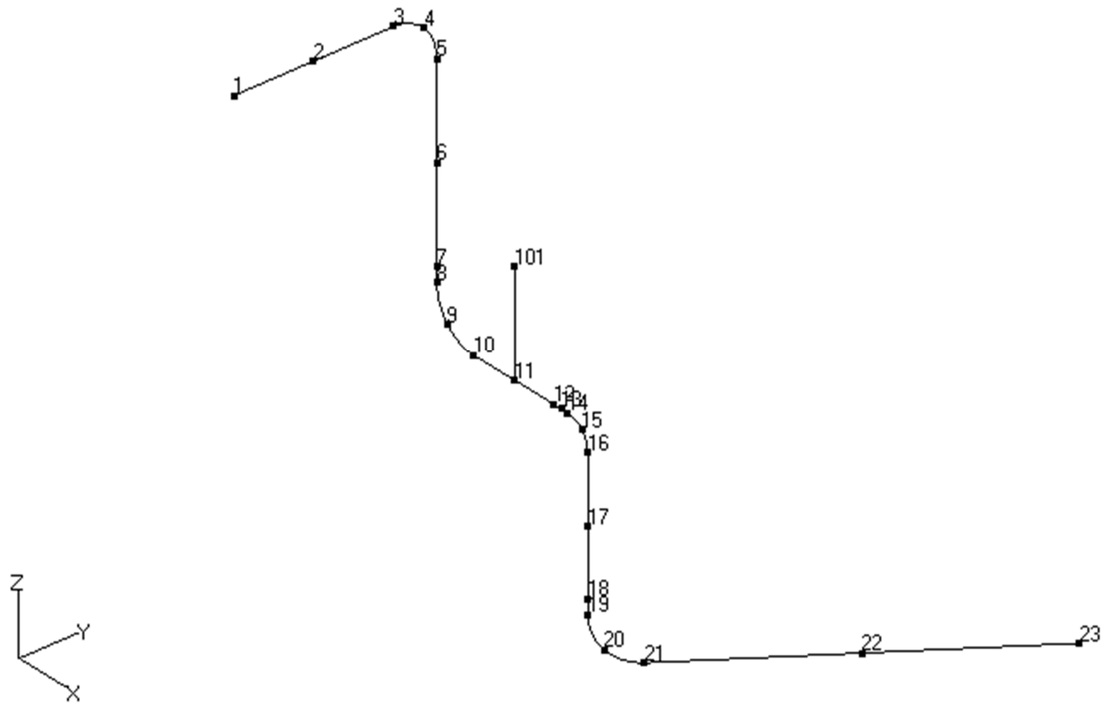
第 3.135 図 貫通部配管 P116(CV 外)の解析モデル図(節点番号)
