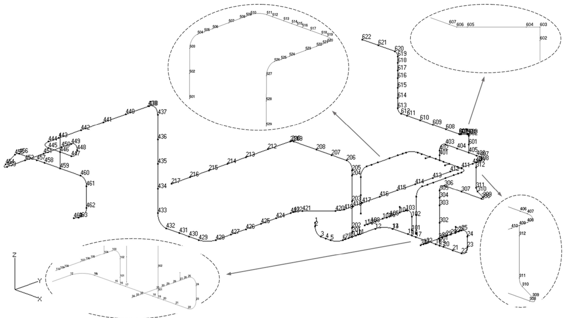
第 3.78 図 貫通部配管 P105(CV 外)の解析モデル図(節点番号)
