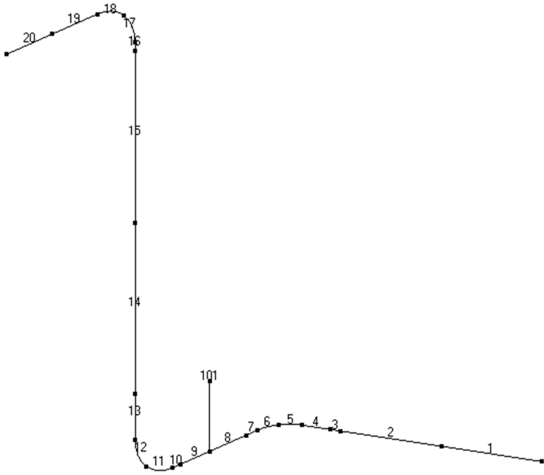
第 3. 142 図 貫通部配管 P120 (CV 外) の解析モデル図 (要素番号)
