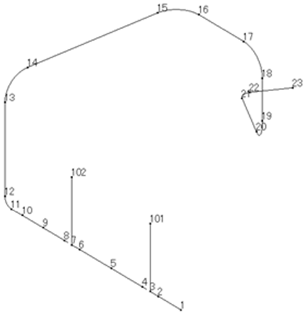
第 3.178 図 貫通部配管 P211 その 1 (CV 外) の解析モデル図 (節点番号)
