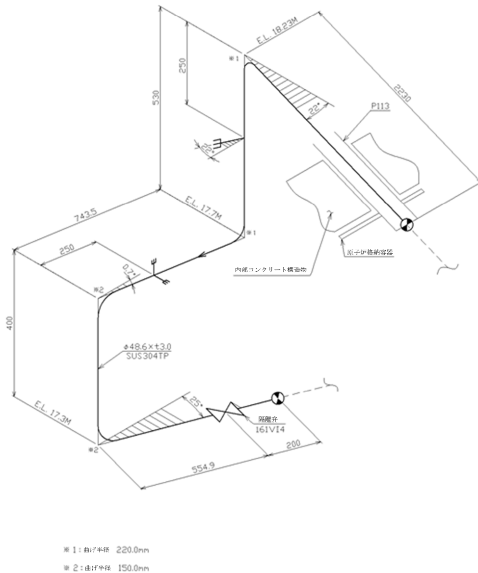
第 3.25 図 貫通部配管 P113(CV 内)のアイソメ図
