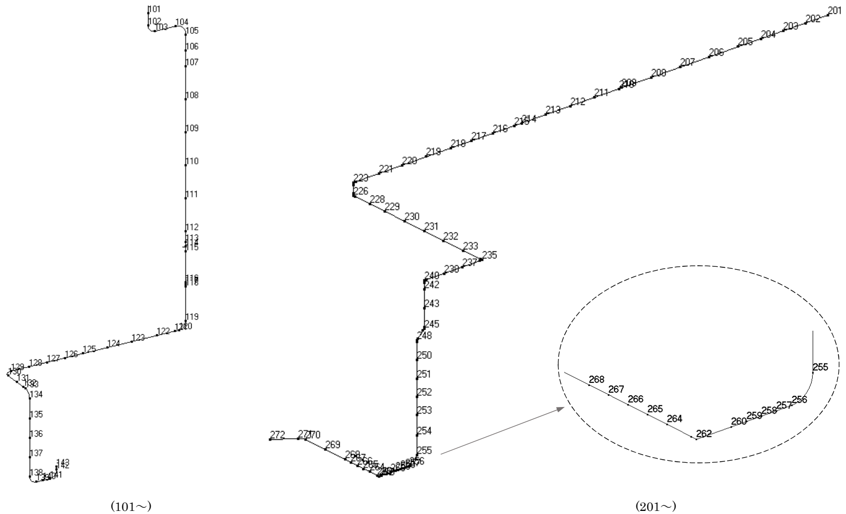
第 3.69 図 貫通部配管 P103(CV 外)の解析モデル図(節点番号 2)
