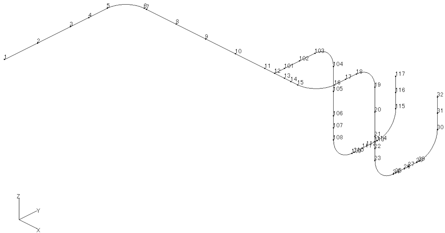
第 3.205 図 非常用空気浄化設備主ダクトの解析モデル図(節点番号)
