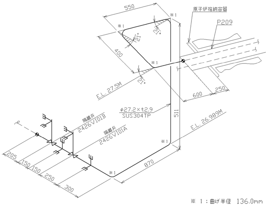
第 3.175 図 貫通部配管 P209 その 1 (CV 外) のアイソメ図
