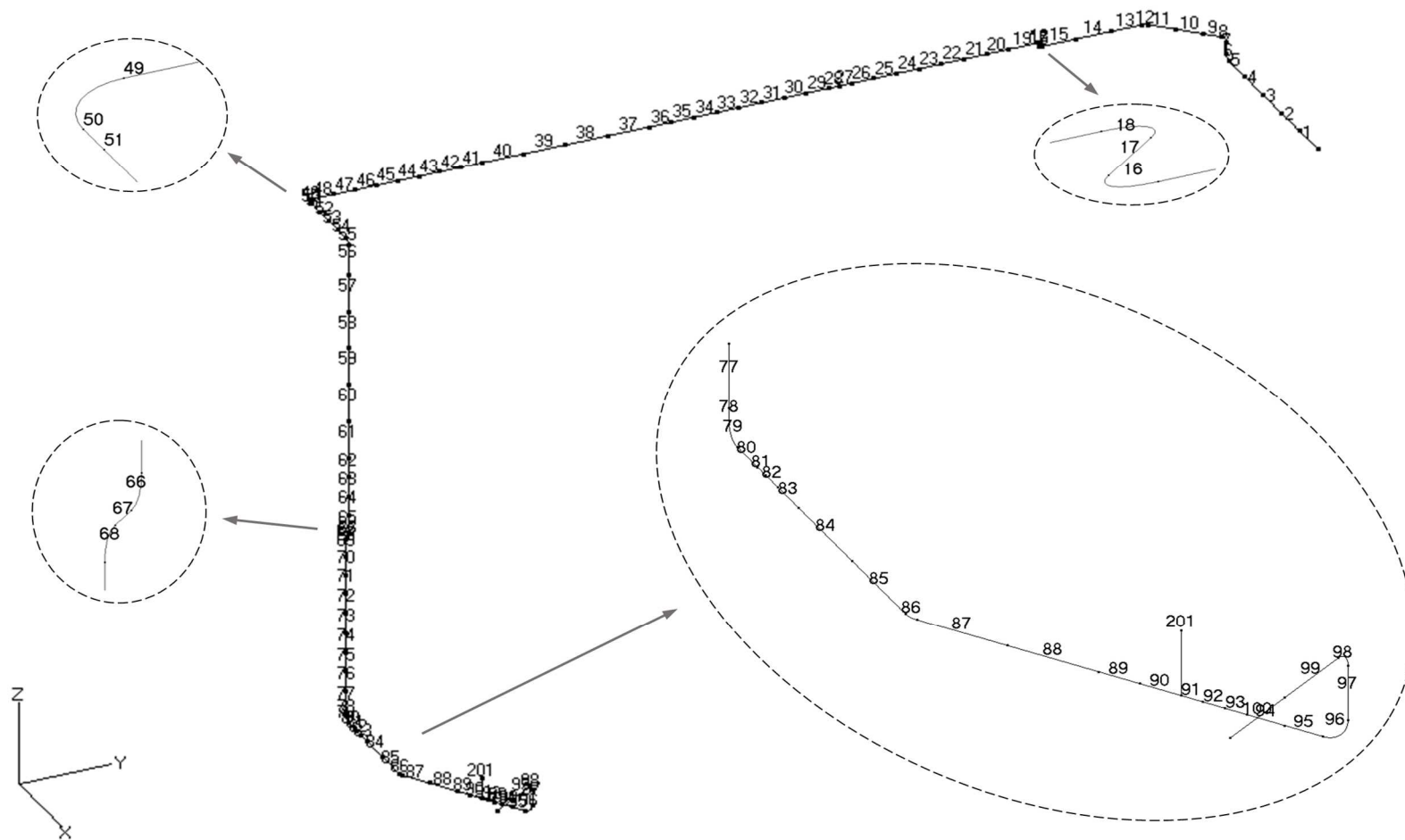
第 3.148 図 貫通部配管 P125(CV 外)の解析モデル図(要素番号)
