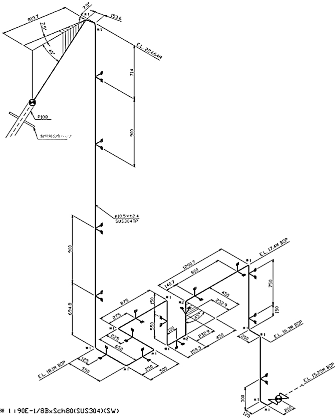
第 3.12 図 貫通部配管 P108(CV 外)のアイソメ図
