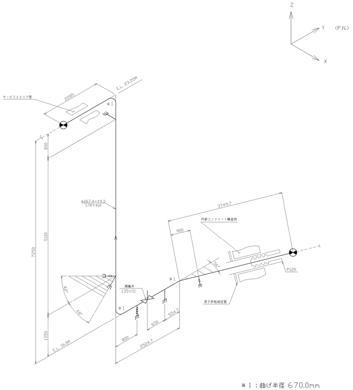
第 3.140 図 貫通部配管 P120 (CV 外) のアイソメ図
