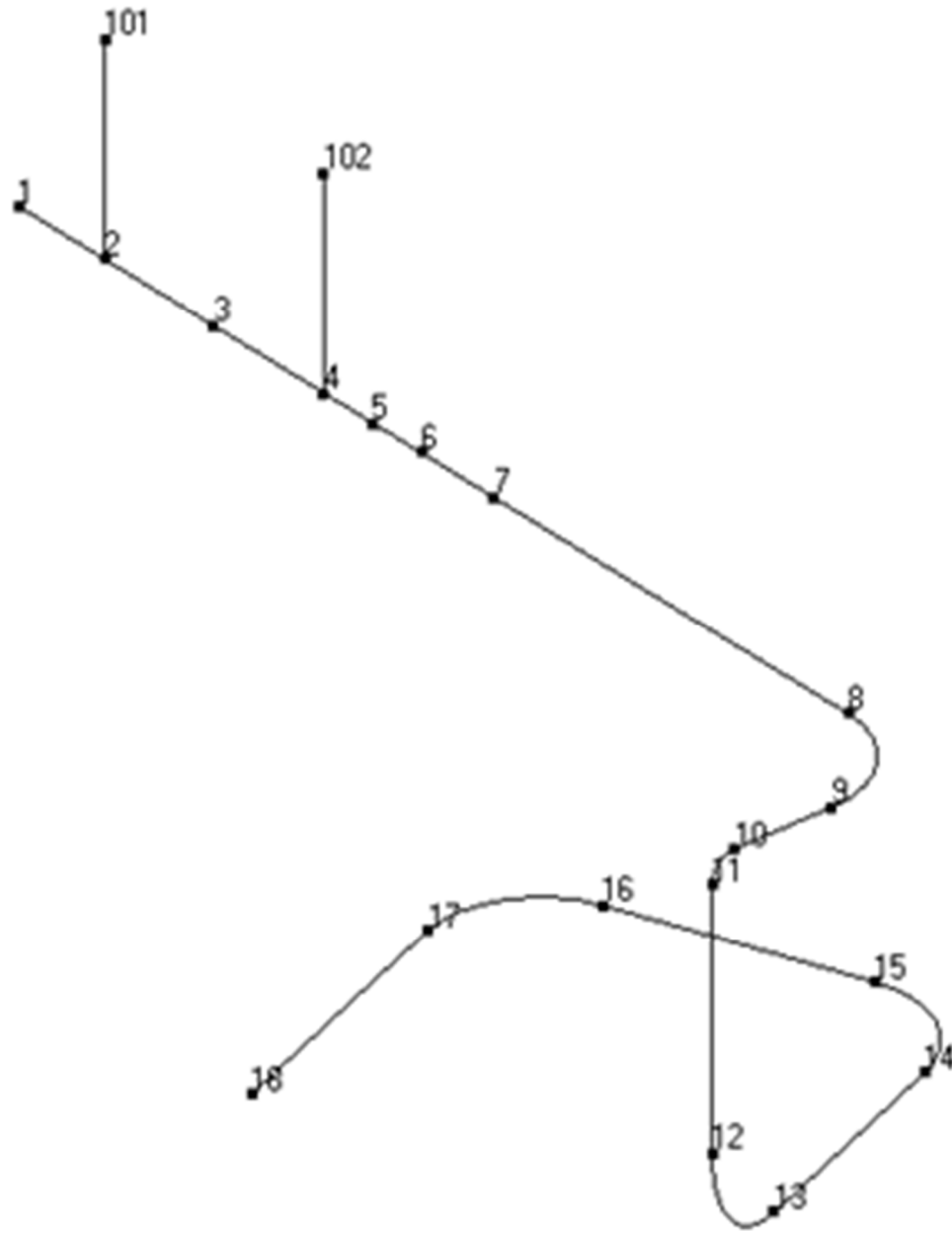
第 3. 202 図 貫通部配管 P225 (CV 外) の解析モデル図 (節点番号)
