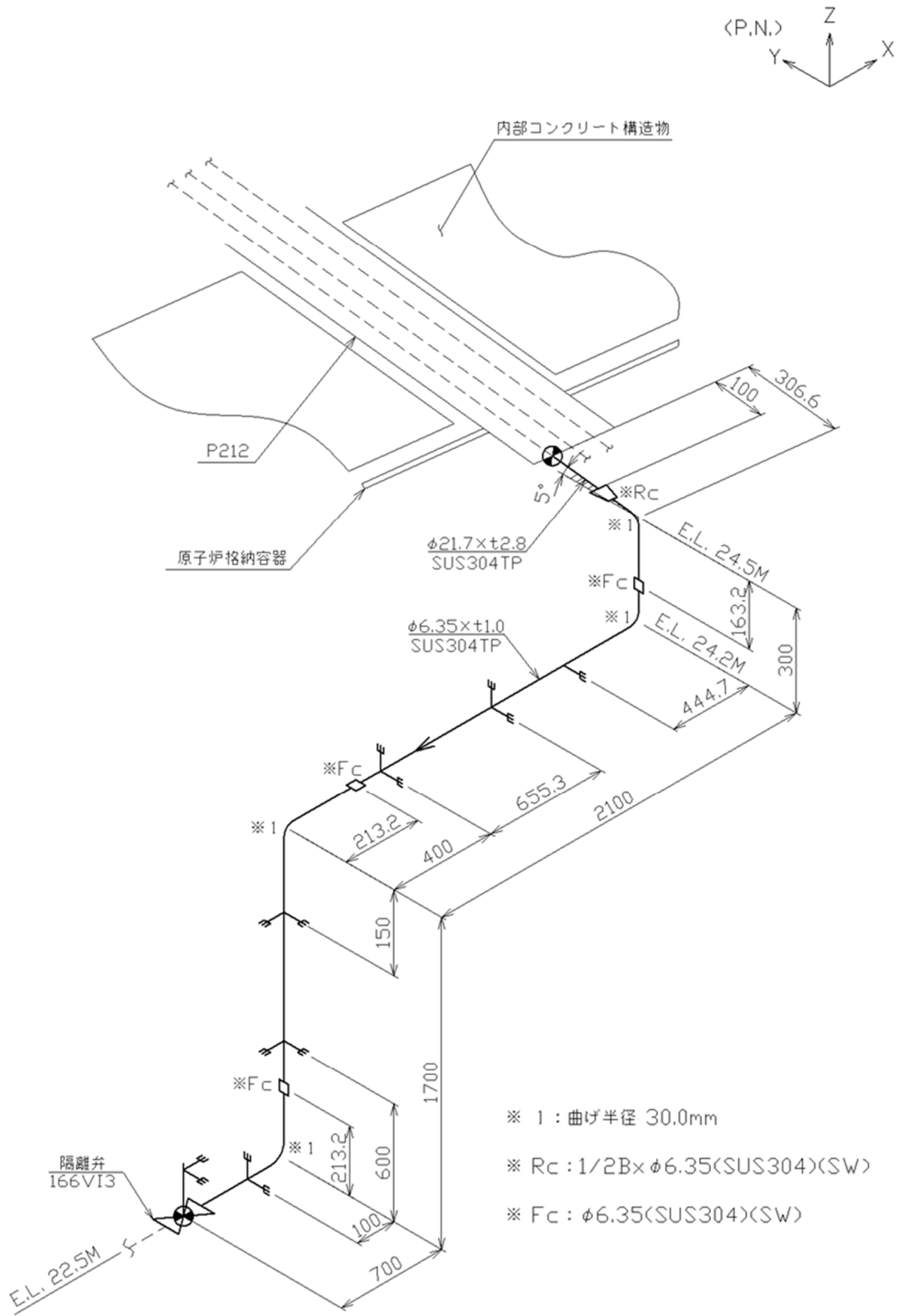
第 3.186 図 貫通部配管 P212 その 3(CV 外)のアイソメ図
