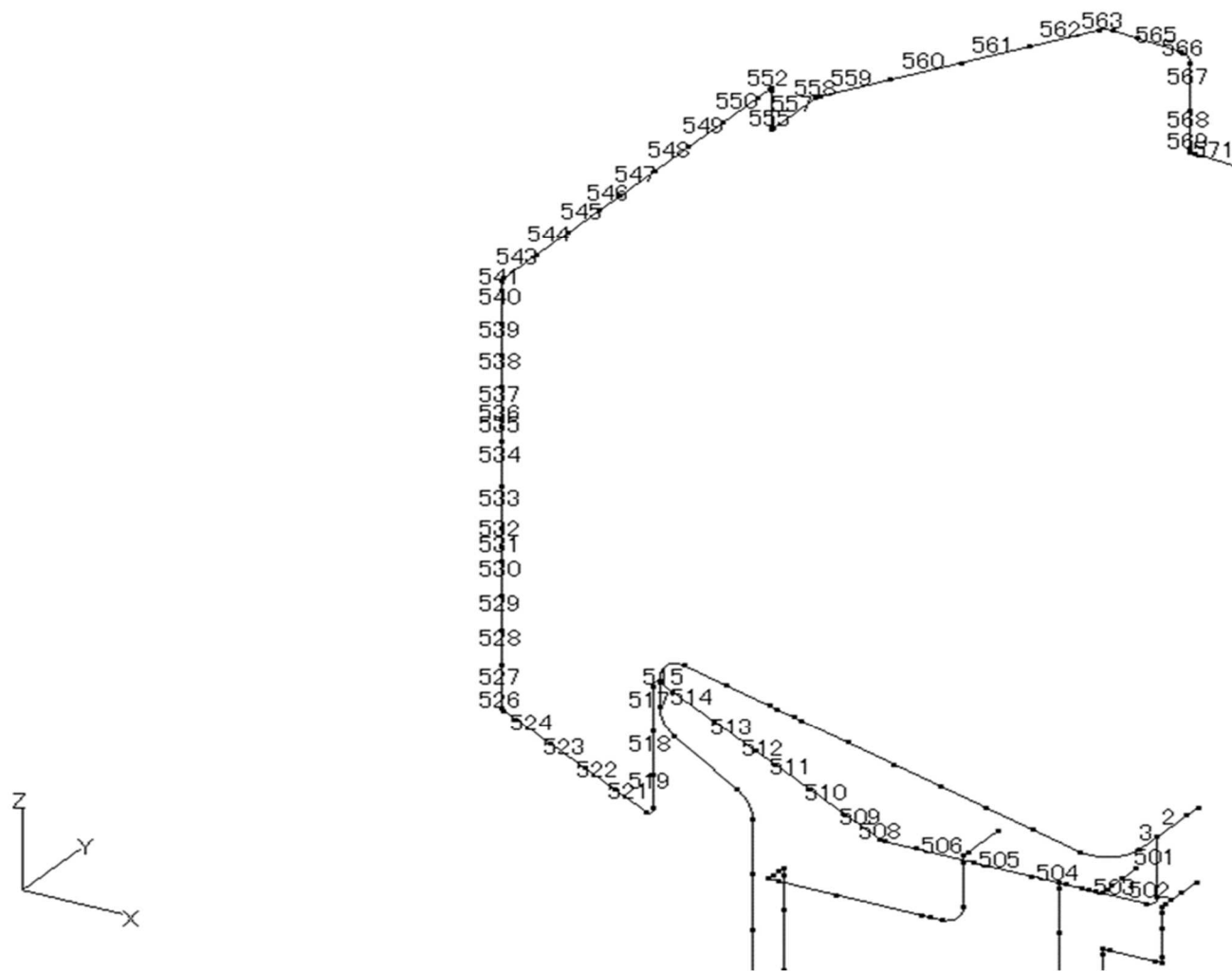
第 3.112 図 貫通部配管 P111 (CV 内) の解析モデル図 (要素番号 3)
