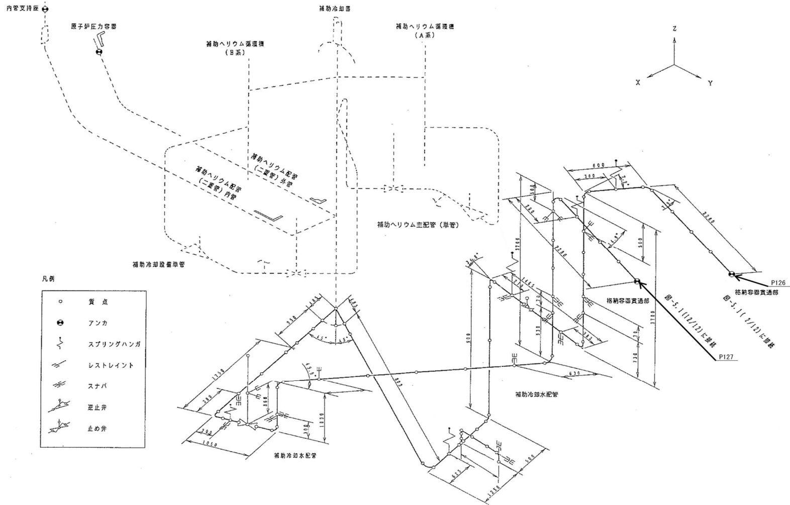
第 3.160 図 貫通部配管 P127(CV 内)のアイソメ図
