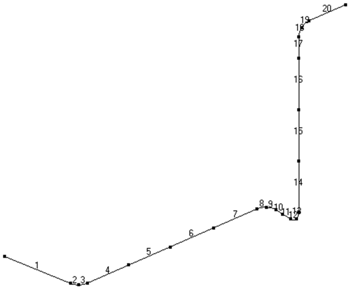
第 3.171 図 貫通部配管 P206 (CV 外) の解析モデル図 (要素番号)
