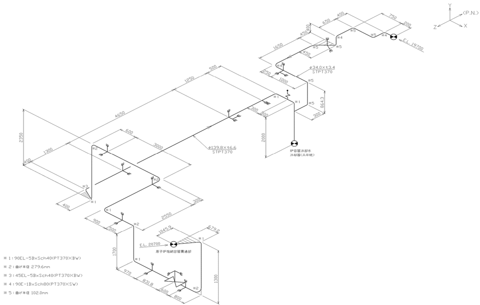
第 3.86 図 貫通部配管 P106(CV 外)のアイソメ図
