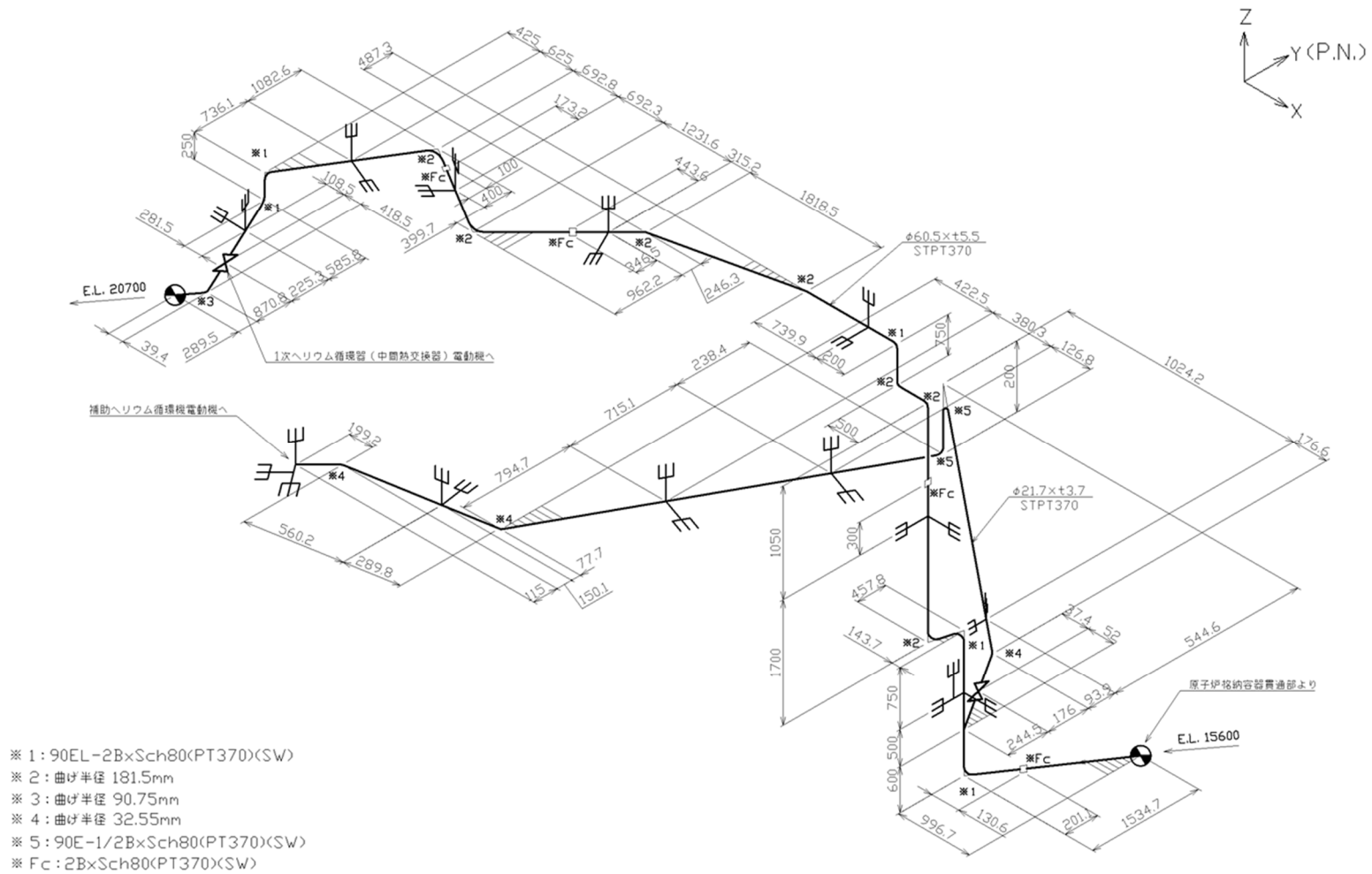
第 3.71 図 貫通部配管 P103(CV 内)のアイソメ図
