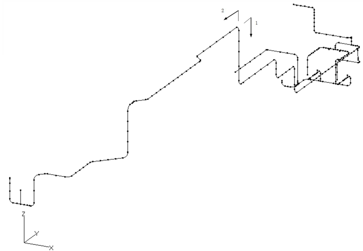
第 3.115 図 貫通部配管 P112(CV 外)の解析モデル図(全体)
