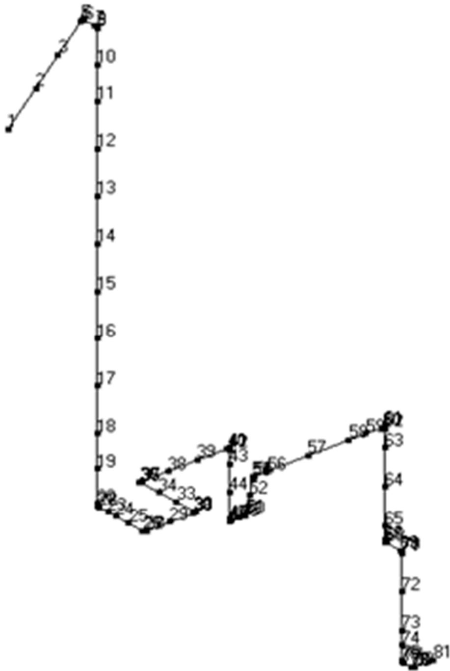
第 3.13 図 貫通部配管 P108 (CV 外) の解析モデル図 (節点番号)
