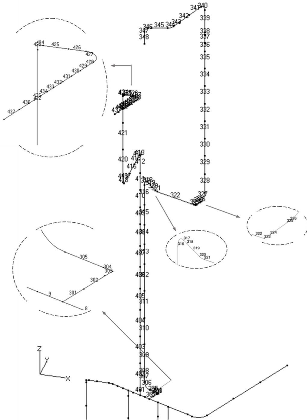
第 3.85 図 貫通部配管 P105(CV 内)の解析モデル図(要素番号 2)
