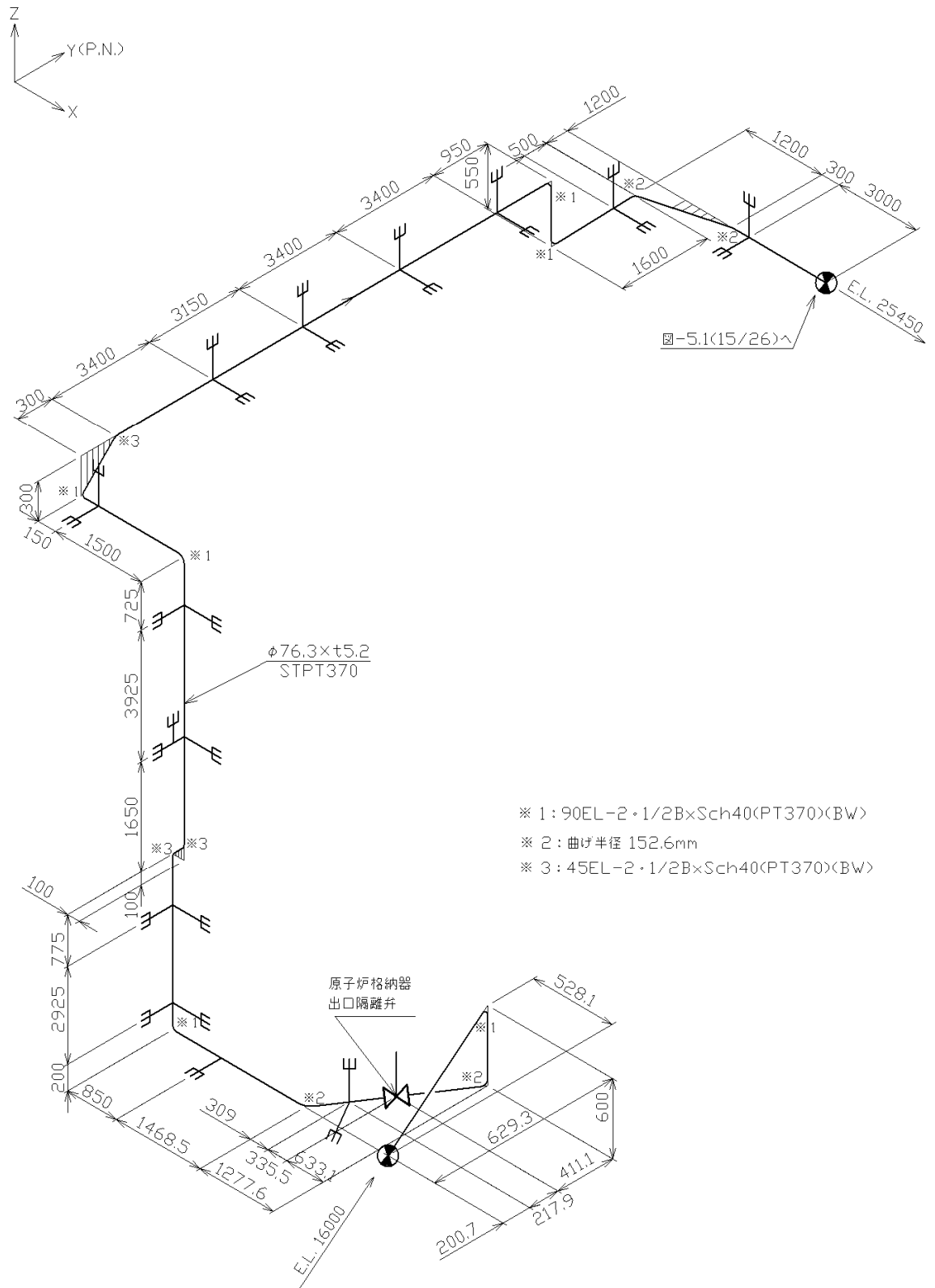
第 3.143 図 貫通部配管 P124(CV 外)のアイソメ図
