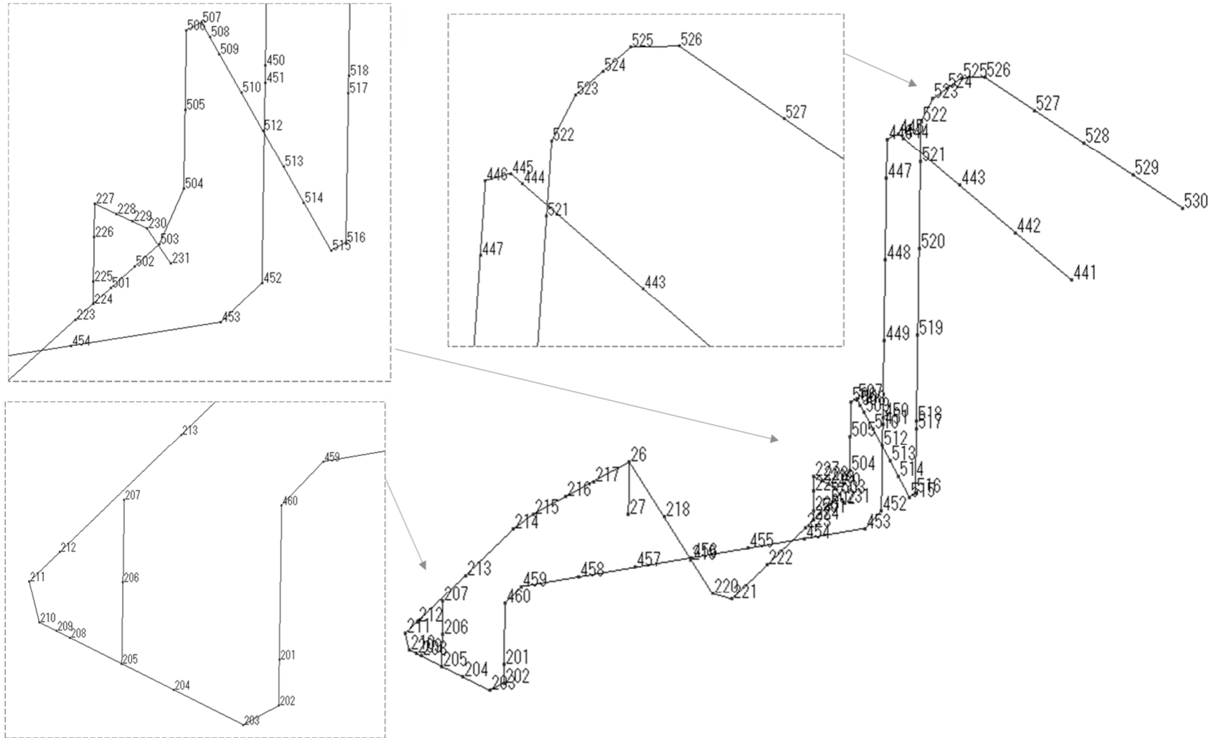
第 3.161 図 貫通部配管 P127(CV 内)の解析モデル図(節点番号)
