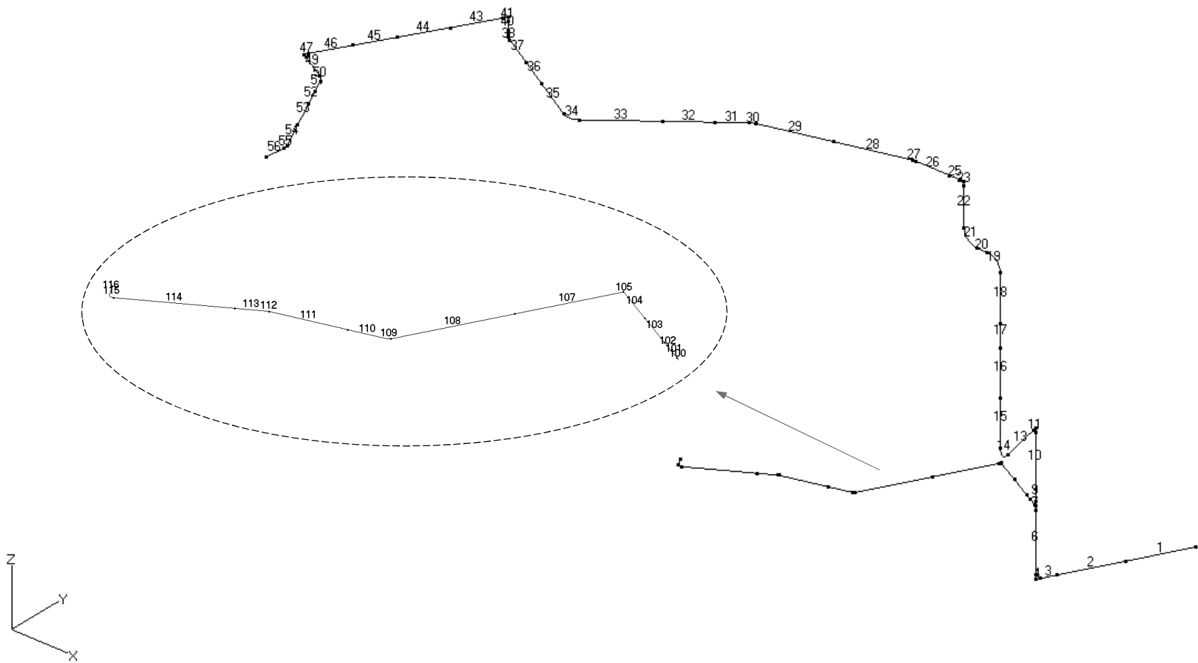
第 3.73 図 貫通部配管 P103 (CV 内) の解析モデル図 (要素番号)
