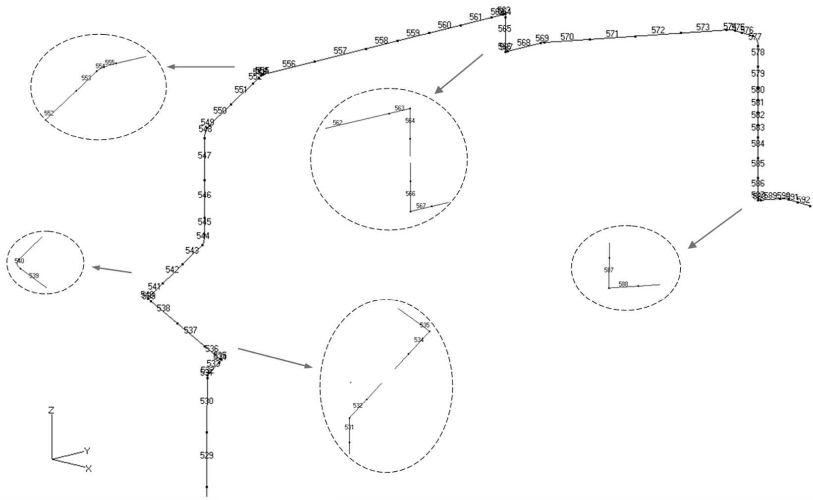
第 3.127 図 貫通部配管 P112 (CV 内) の解析モデル図 (要素番号 3)
