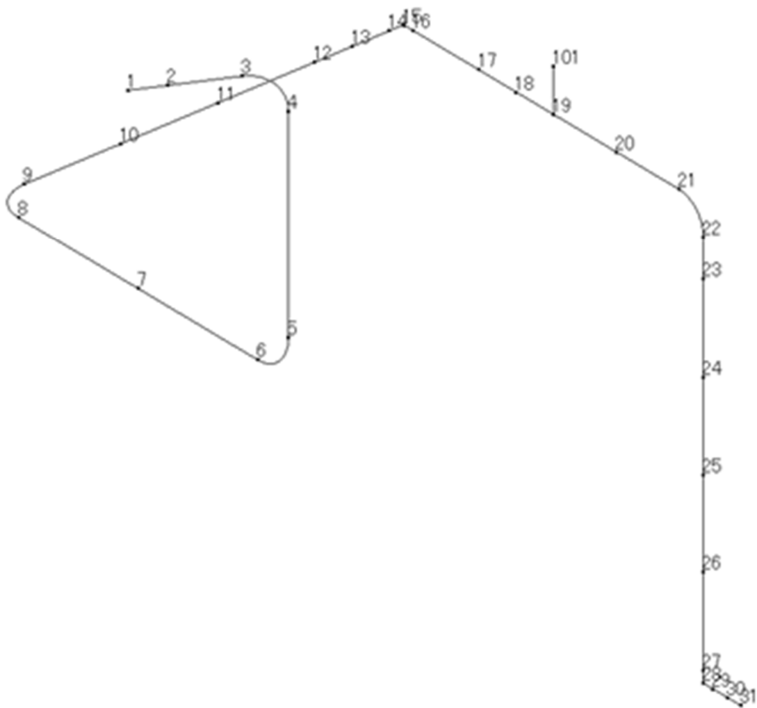
第 3.164 図 貫通部配管 P201 (CV 外) の解析モデル図 (節点番号)
