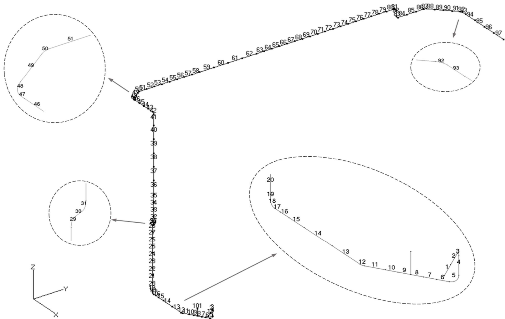
第 3.145 図 貫通部配管 P124(CV 外)の解析モデル図(要素番号)
