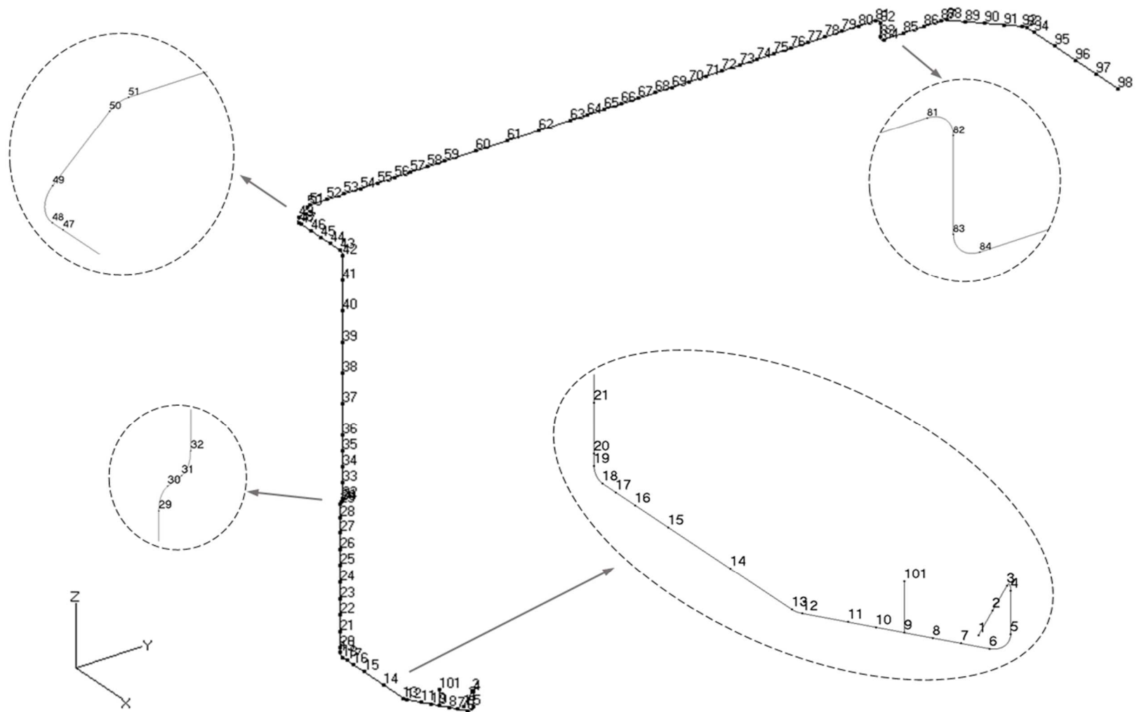
第 3.144 図 貫通部配管 P124(CV 外)の解析モデル図(節点番号)
