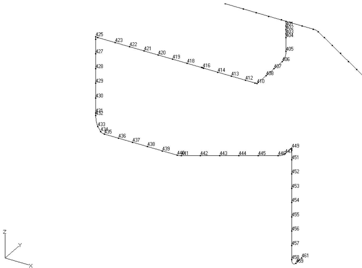
第 3.109 図 貫通部配管 P111 (CV 内) の解析モデル図 (節点番号 2)
