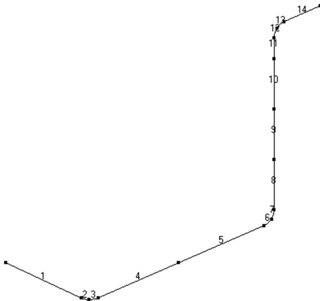
第 3.174 図 貫通部配管 P207 (CV 外) の解析モデル図 (要素番号)
