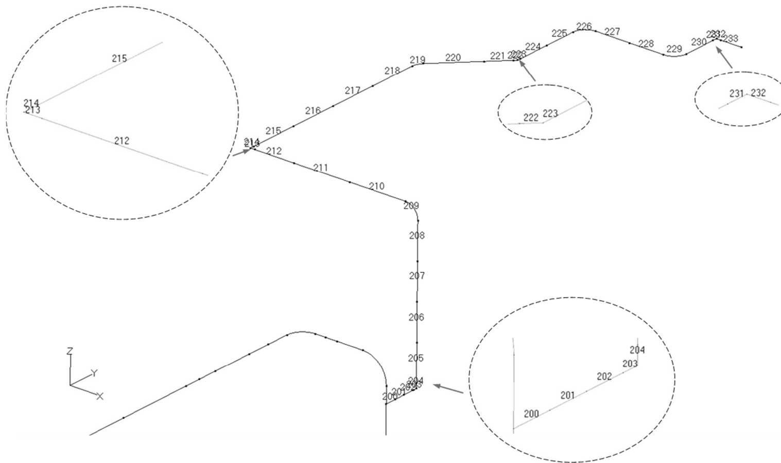
第 3.104 図 貫通部配管 P111 (CV 外) の解析モデル図 (要素番号 3)
