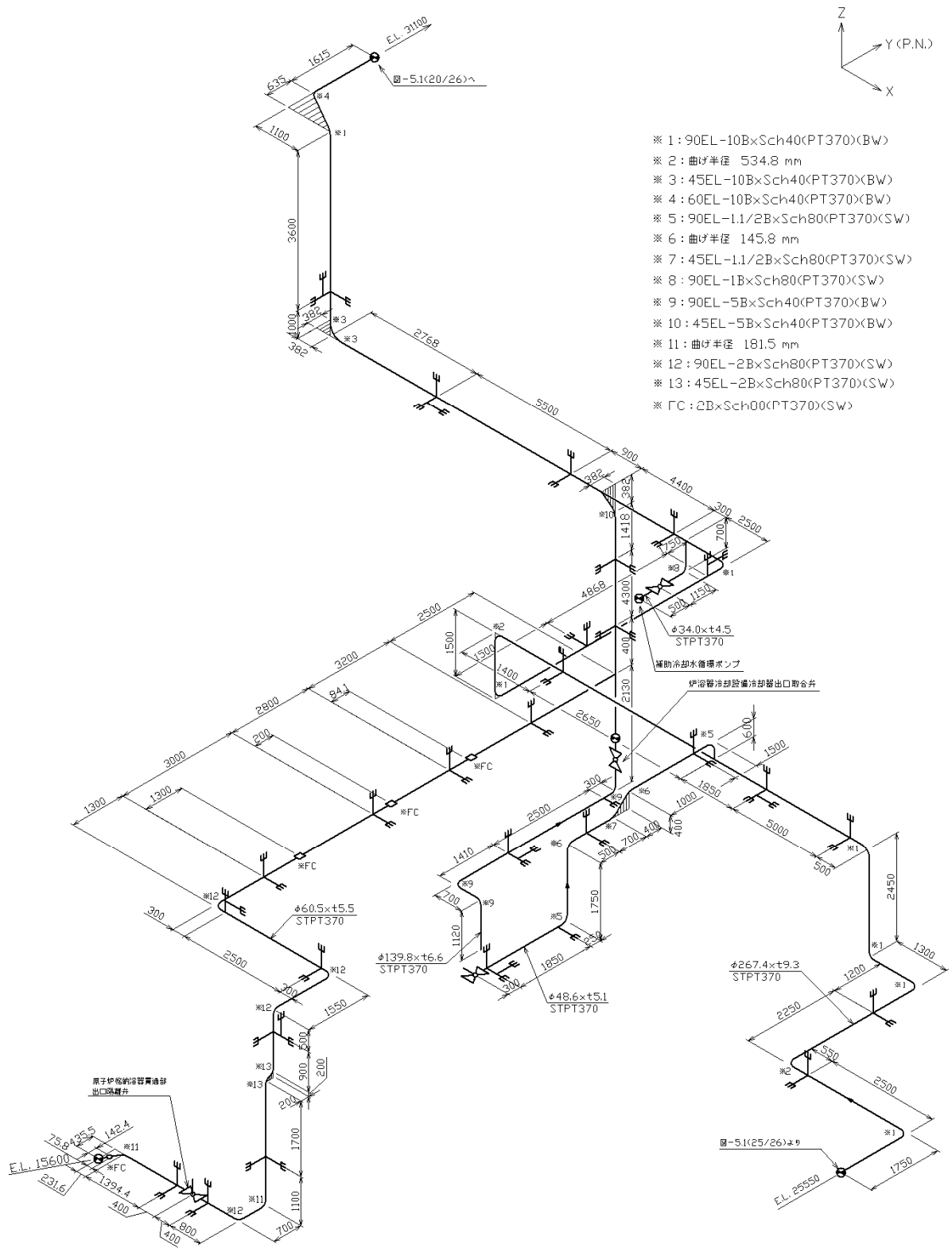
第 3.58 図 貫通部配管 P102(CV 外)のアイソメ図
