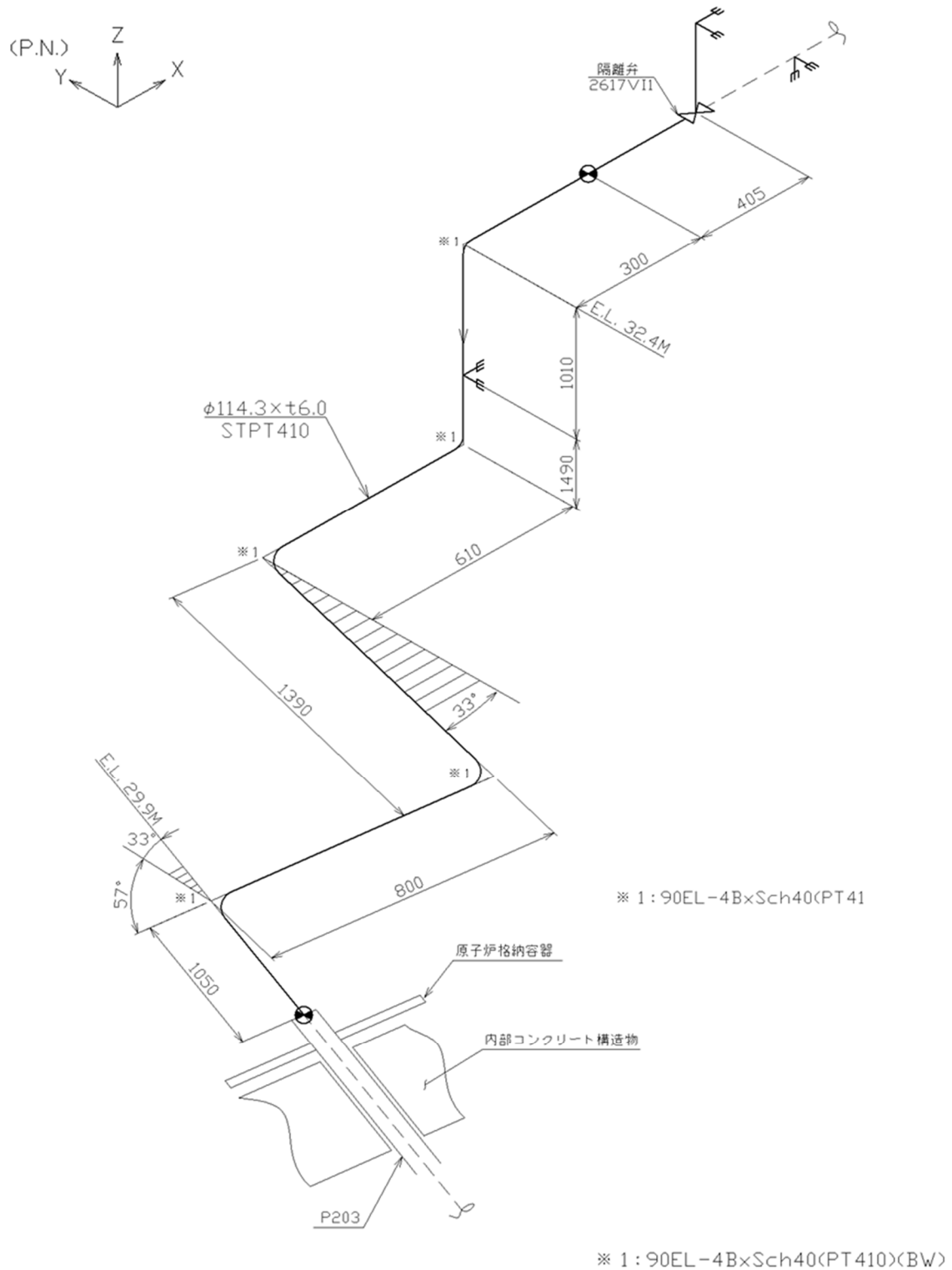
第 3.166 図 貫通部配管 P203 (CV 外) のアイソメ図
