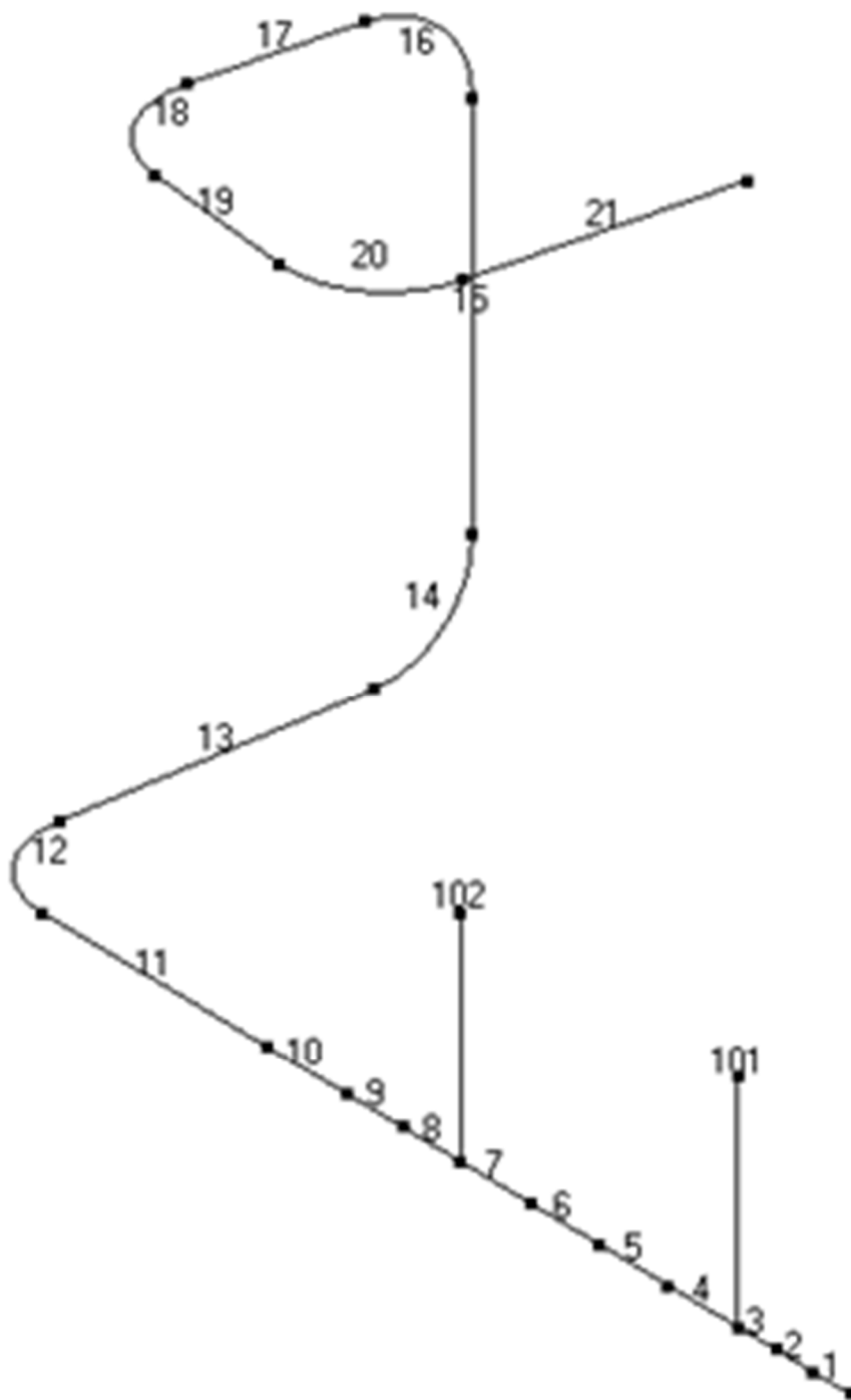
第 3.200 図 貫通部配管 P219 (CV 外) の解析モデル図 (要素番号)
