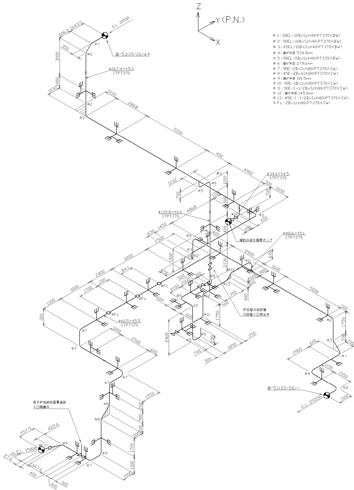
第 3.66 図 貫通部配管 P103(CV 外)のアイソメ図
