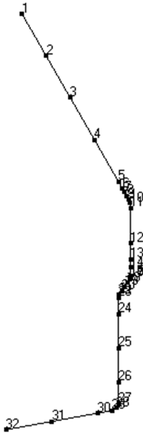
第 3.4 図 貫通部配管 P101 (CV 内) の解析モデル図 (節点番号)
