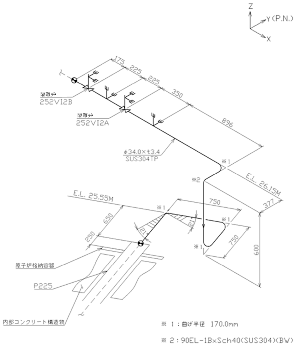
第 3.201 図 貫通部配管 P225 (CV 外) のアイソメ図
