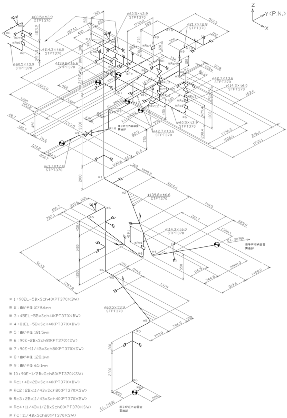
第 3.89 図 貫通部配管 P106(CV 内)のアイソメ図
