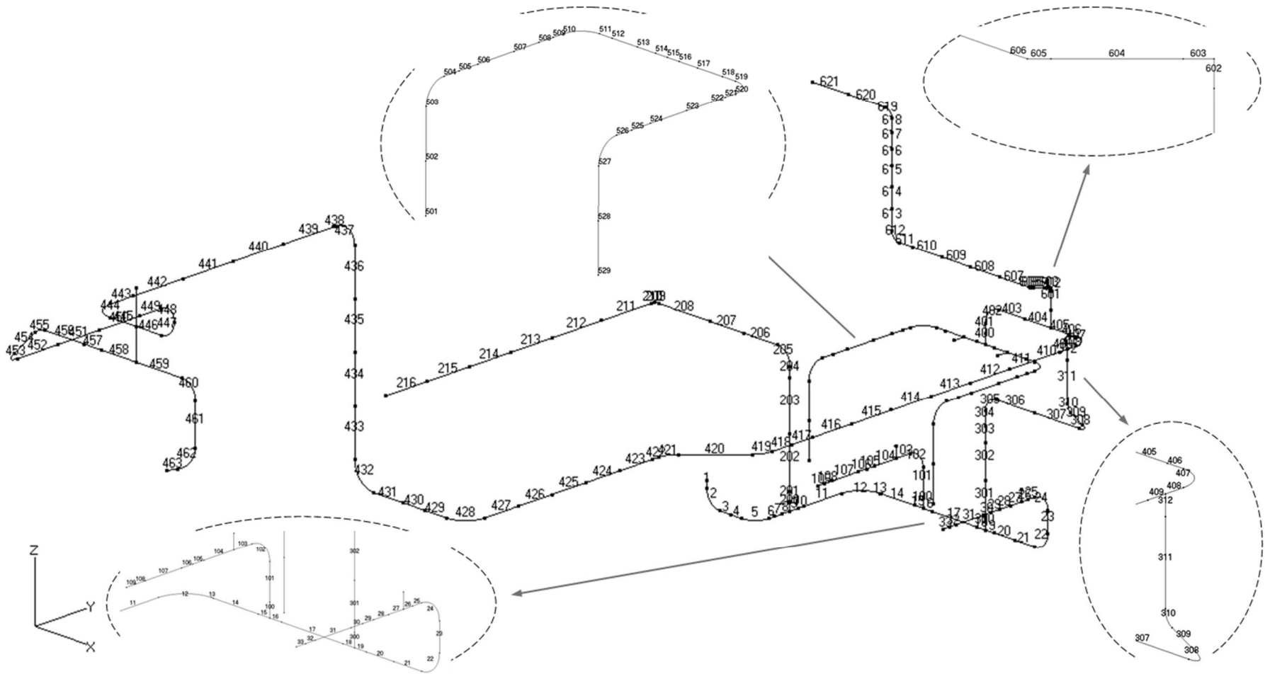
第 3.79 図 貫通部配管 P105 (CV 外) の解析モデル図 (要素番号)
