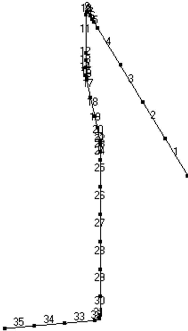
第 3.44 図 貫通部配管 P118 その 2(CV 内)の解析モデル図(要素番号)
