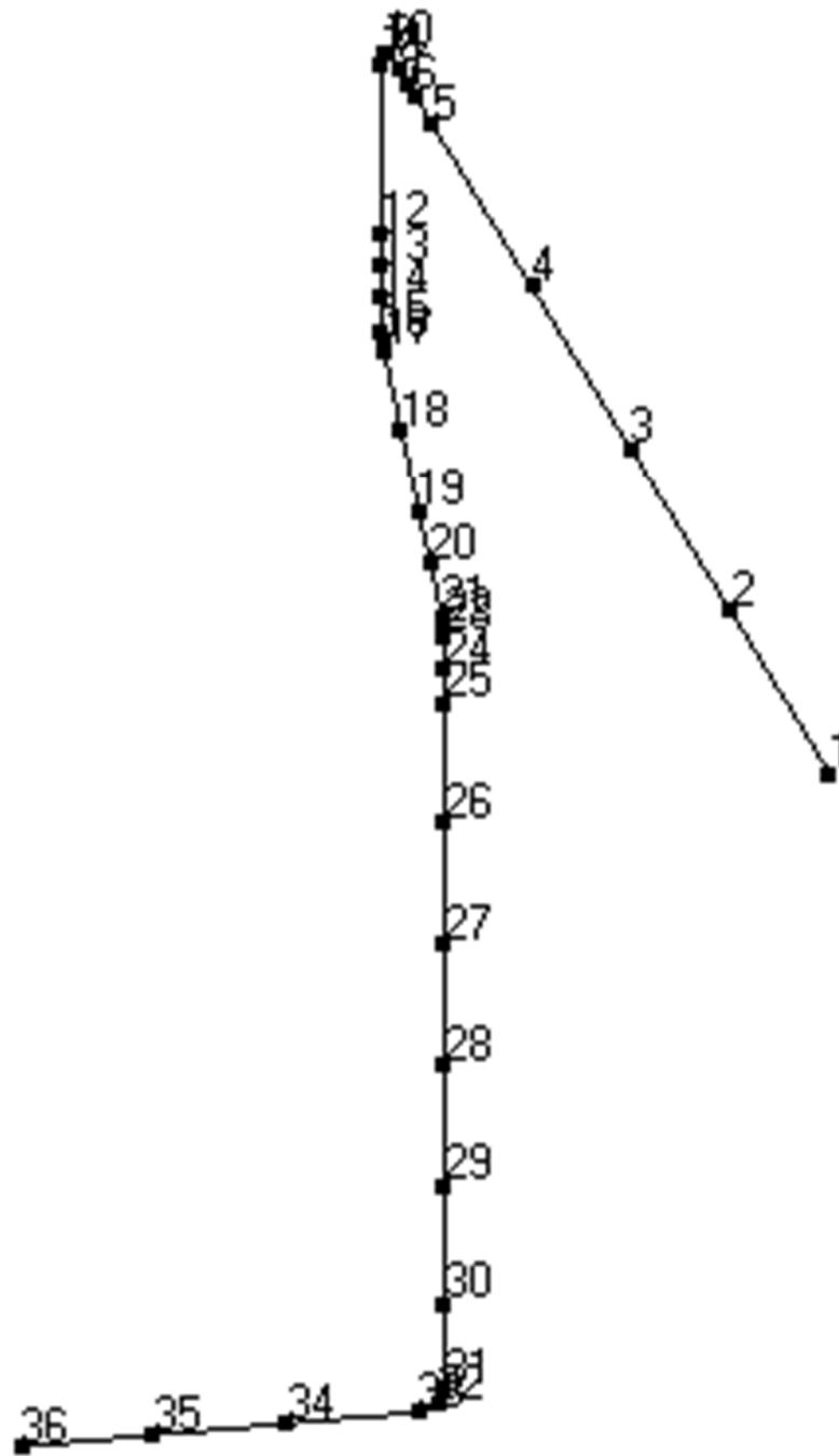
第 3.43 図 貫通部配管 P118 その 2(CV 内)の解析モデル図(節点番号)
