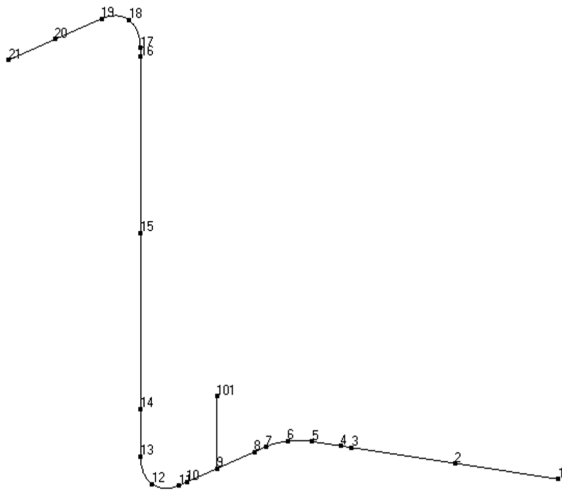
第 3. 141 図 貫通部配管 P120 (CV 外) の解析モデル図 (節点番号)
