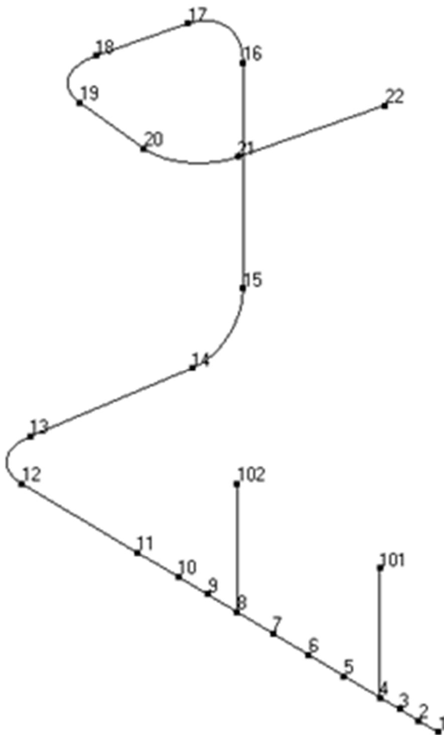
第 3.199 図 貫通部配管 P219 (CV 外) の解析モデル図 (節点番号)
