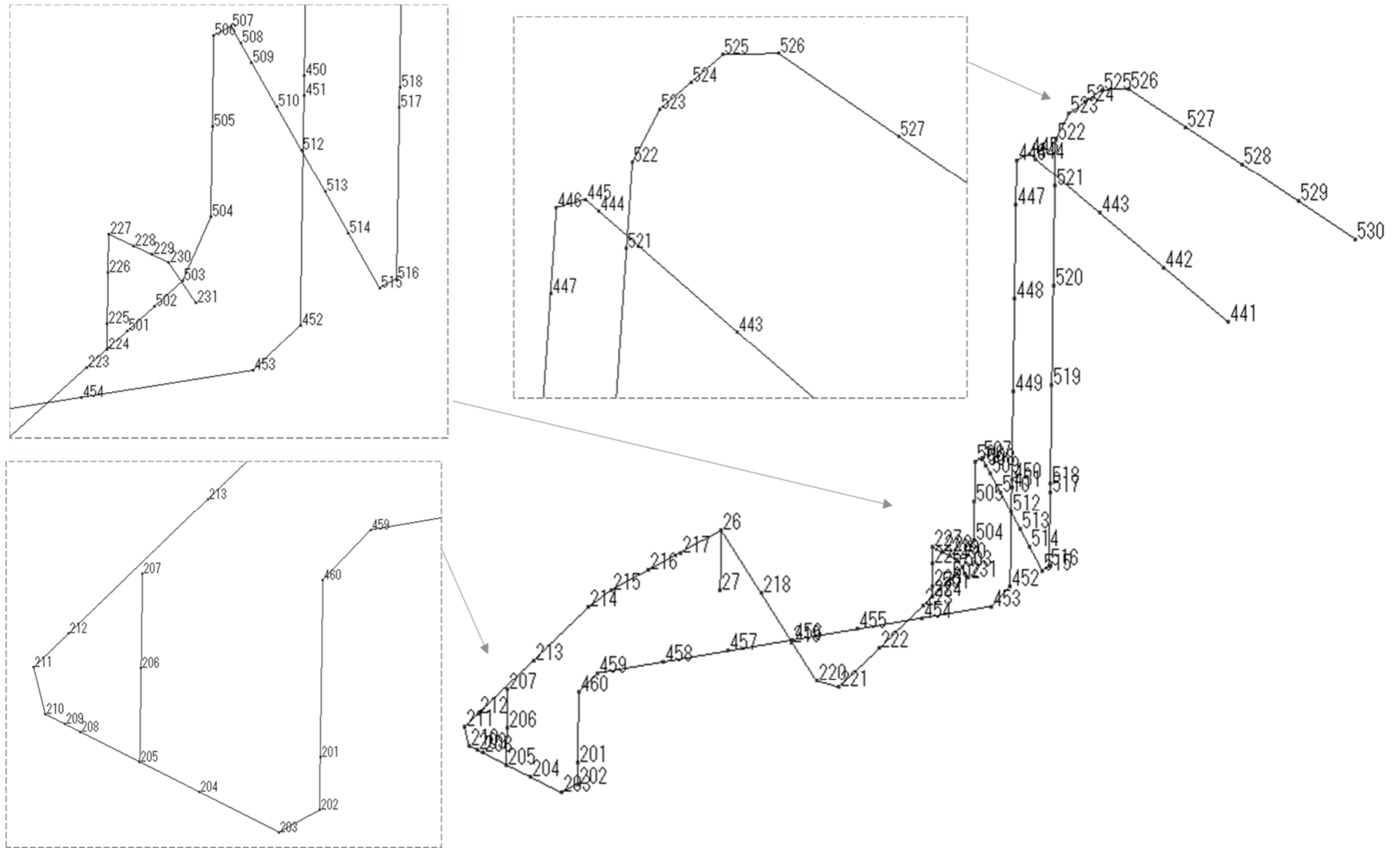
第 3.155 図 貫通部配管 P126(CV 内)の解析モデル図(節点番号)
