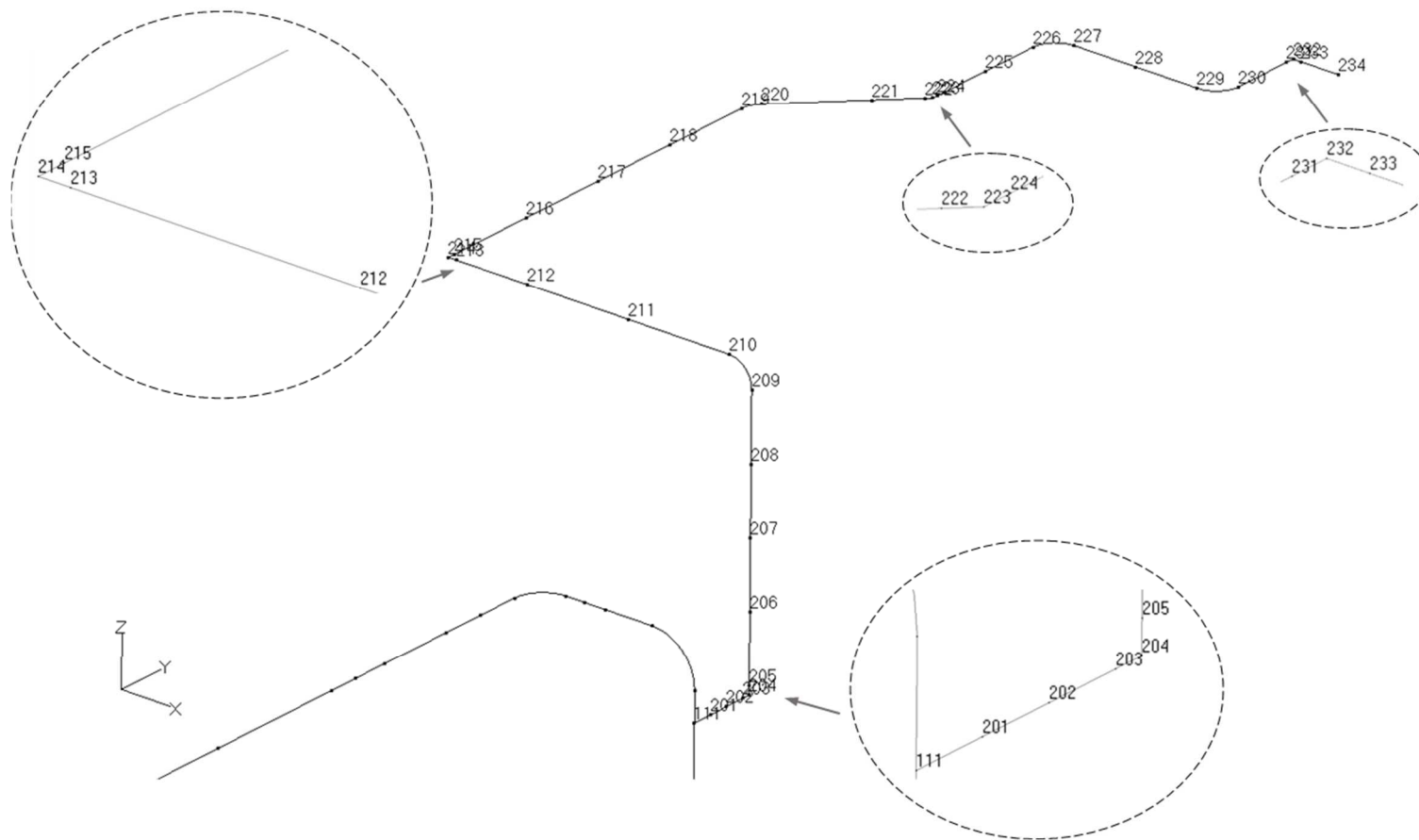
第 3.103 図 貫通部配管 P111 (CV 外) の解析モデル図 (節点番号 3)
