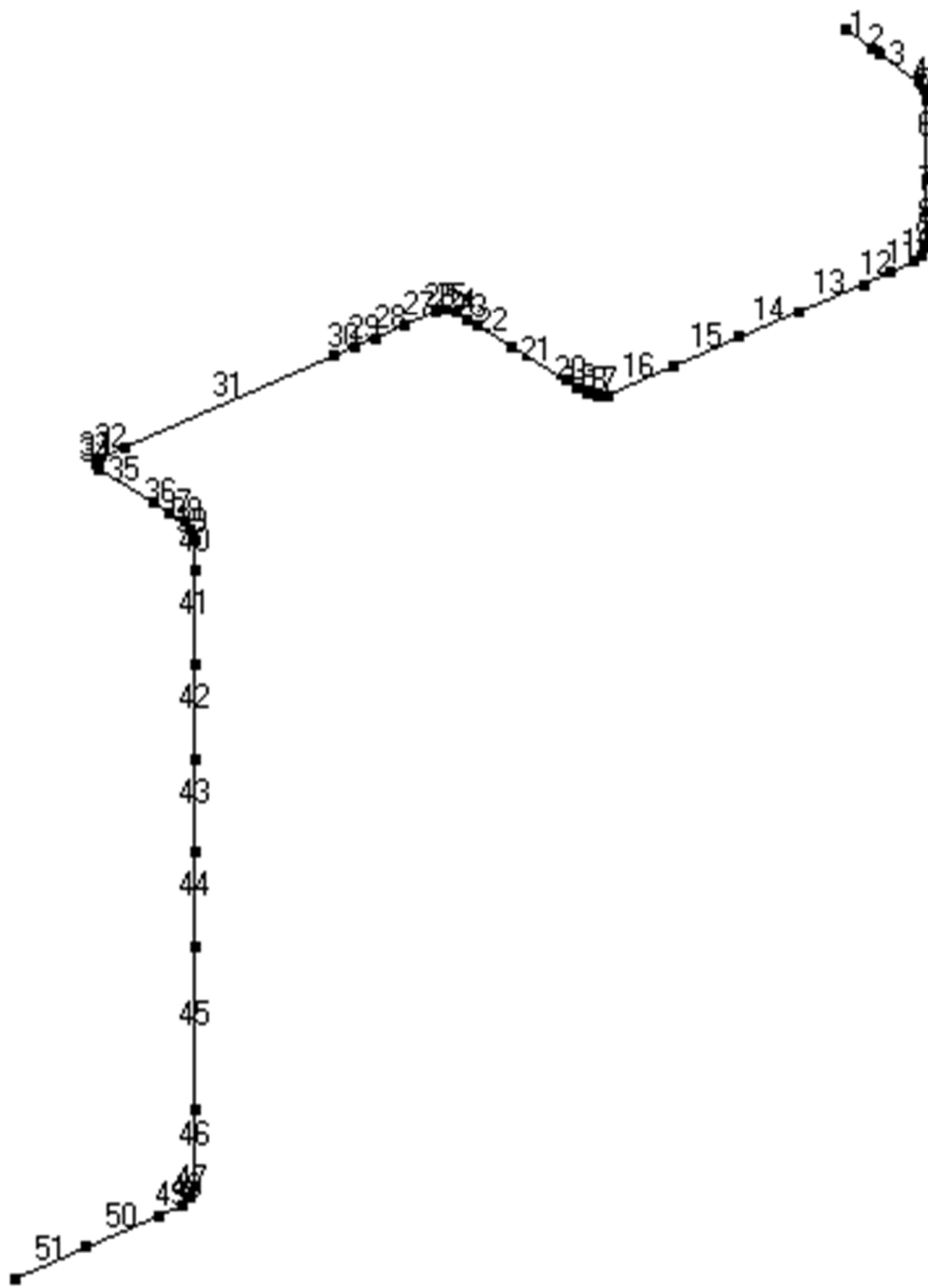
第 3.185 図 貫通部配管 P212 その 1(CV 外)の解析モデル図(要素番号)
