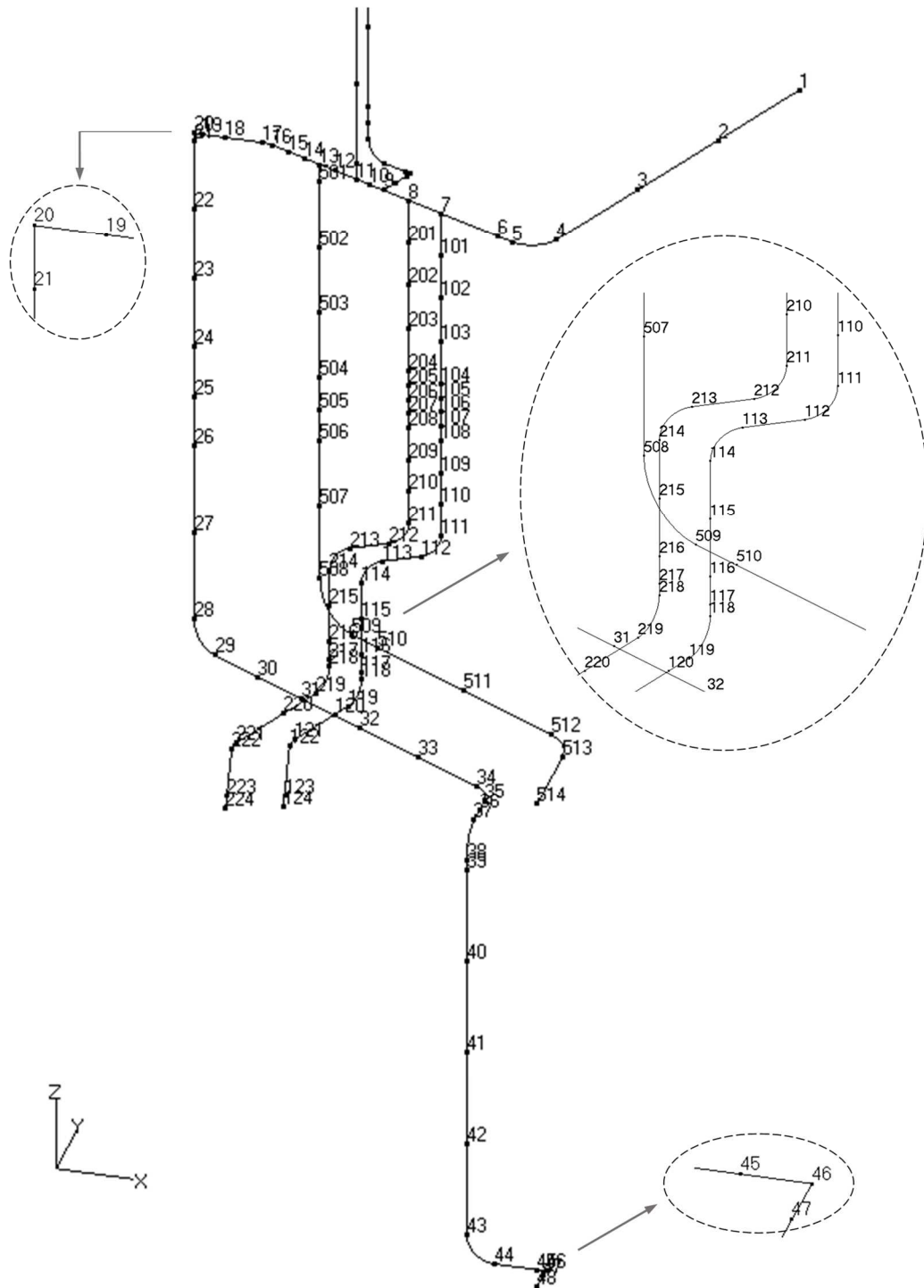
第 3.82 図 貫通部配管 P105(CV 内)の解析モデル図(節点番号 1)
