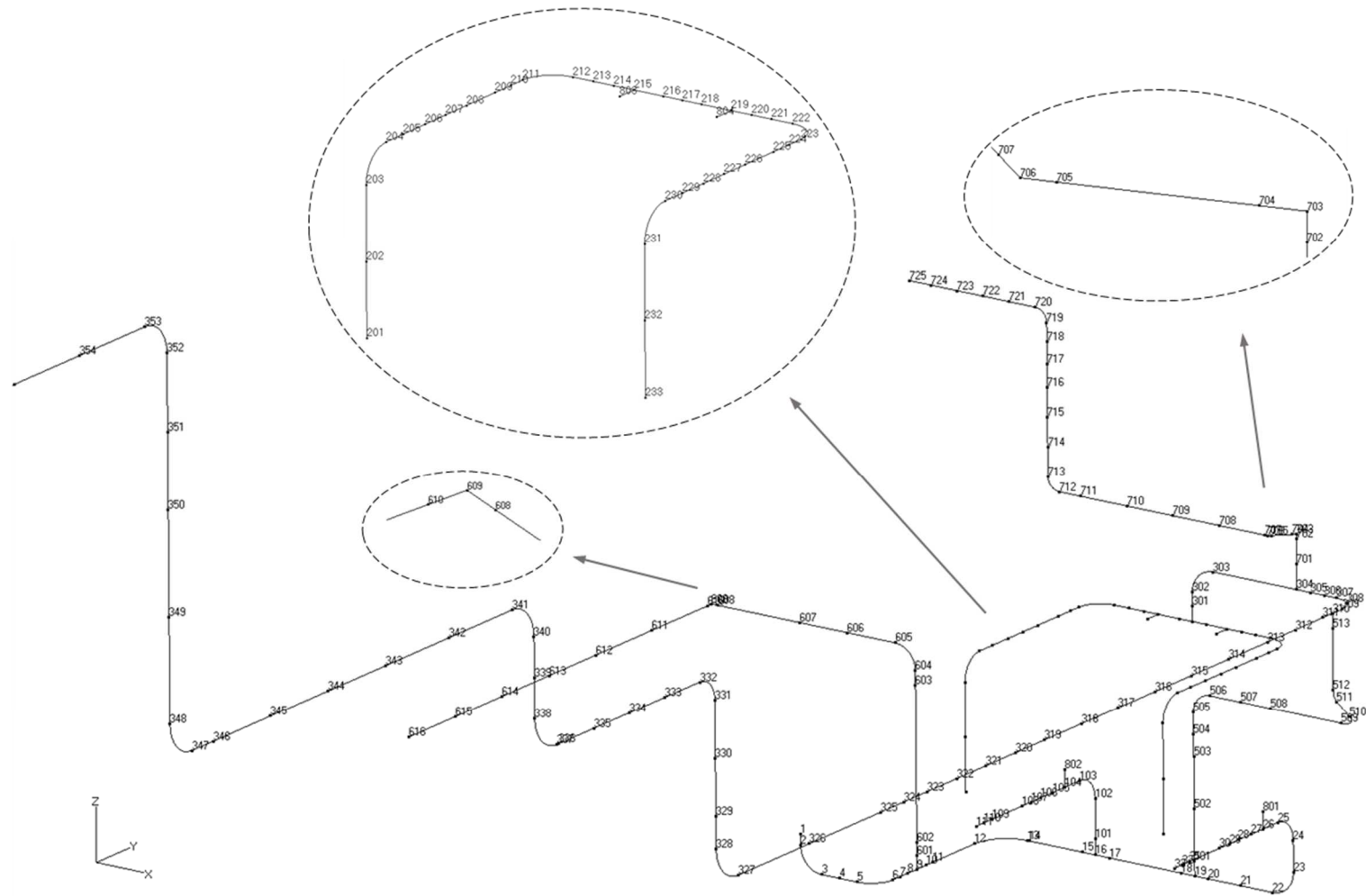
第 3.116 図 貫通部配管 P112 (CV 外) の解析モデル図 (節点番号 1)
