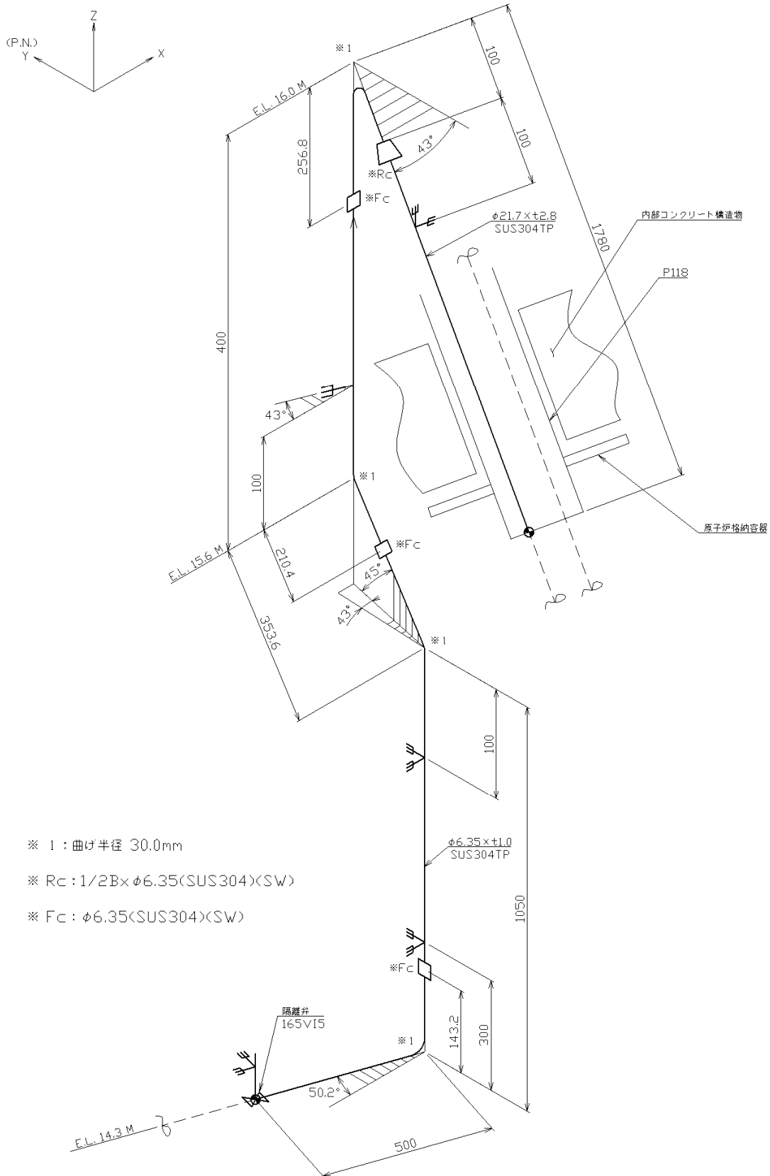
第 3.42 図 貫通部配管 P118 その 2(CV 内)のアイソメ図
