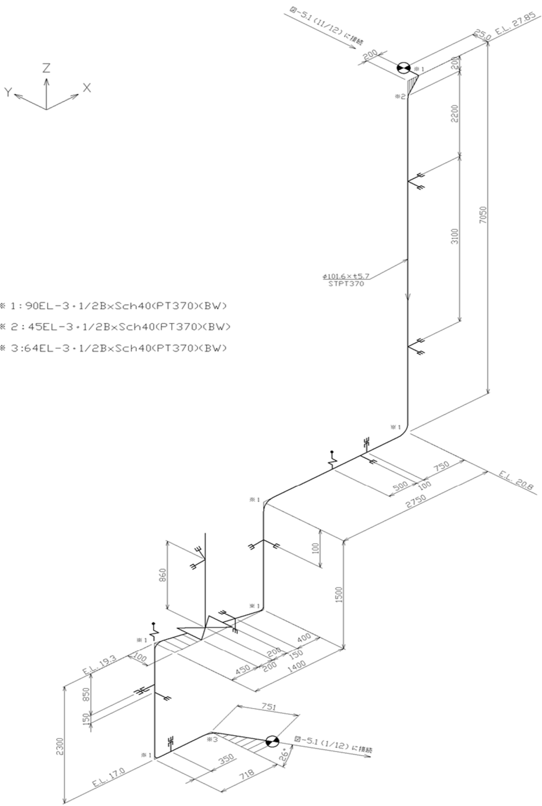
第 3.157 図 貫通部配管 P127 (CV 外) のアイソメ図
