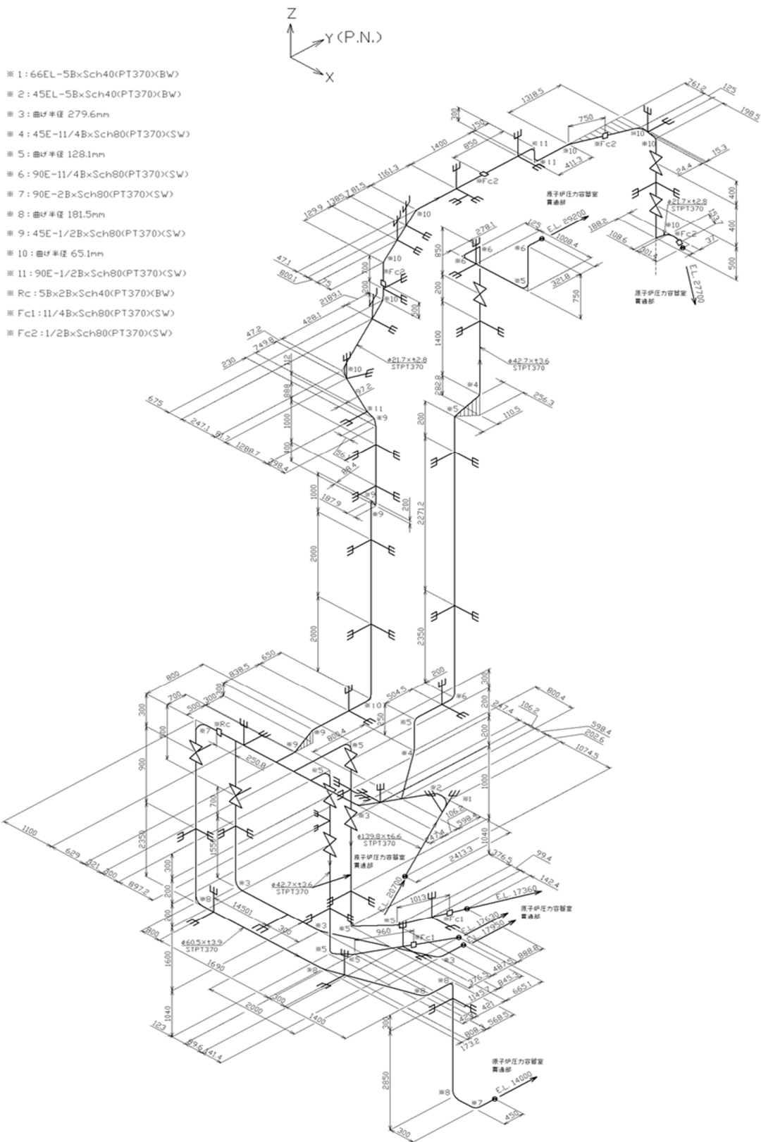
第 3.120 図 貫通部配管 P112(CV 内)のアイソメ図
