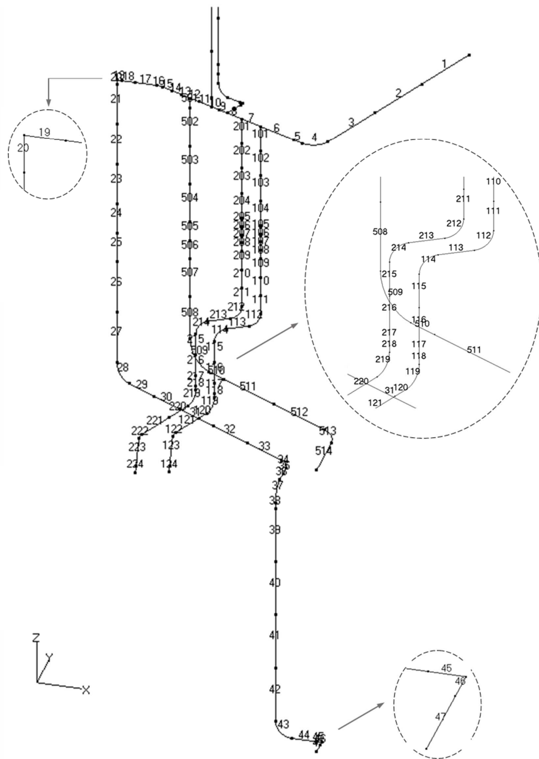
第 3.83 図 貫通部配管 P105(CV 内)の解析モデル図(要素番号 1)
