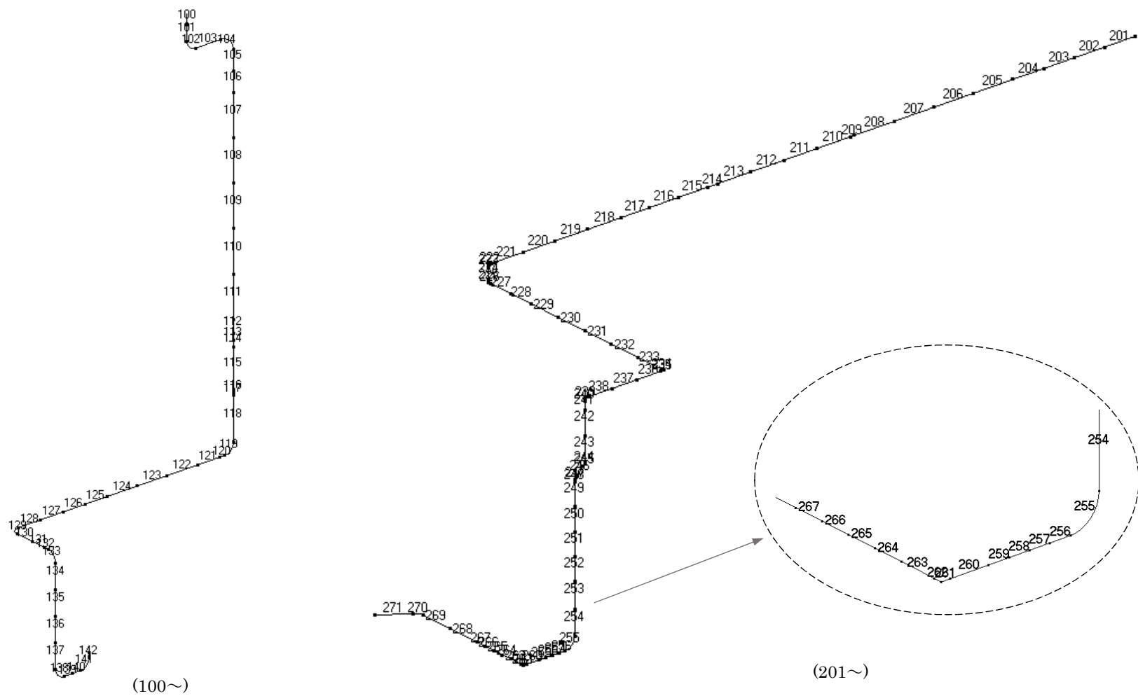
第 3.70 図 貫通部配管 P103(CV 外)の解析モデル図(要素番号 2)
