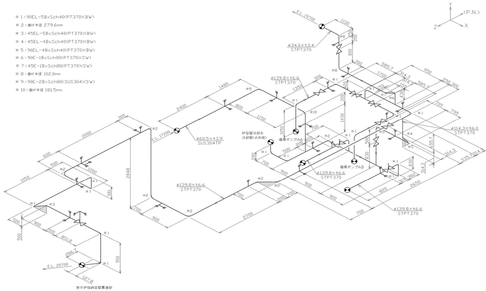
第 3.77 図 貫通部配管 P105(CV 外)のアイソメ図
