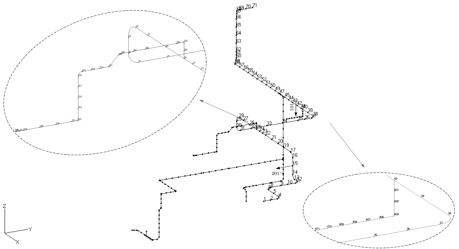
第 3.59 図 貫通部配管 P102(CV 外)の解析モデル図(節点番号 1)
