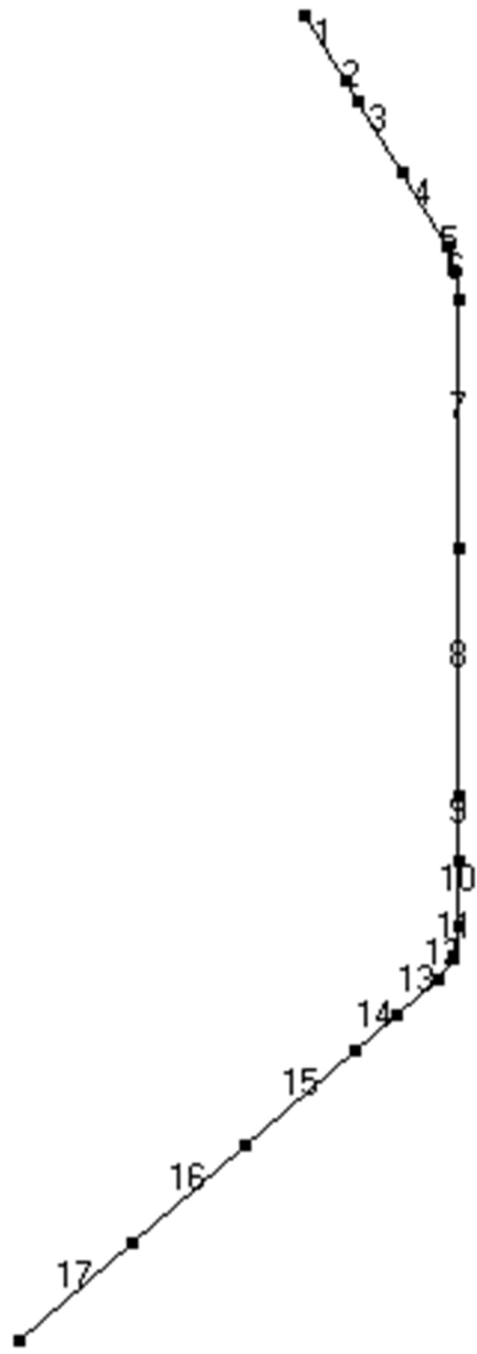
第 3.41 図 貫通部配管 P118 その 2(CV 外)の解析モデル図(要素番号)
