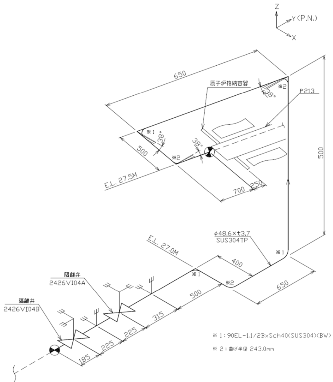
第 3.191 図 貫通部配管 P213 その 2 (CV 外) のアイソメ図
