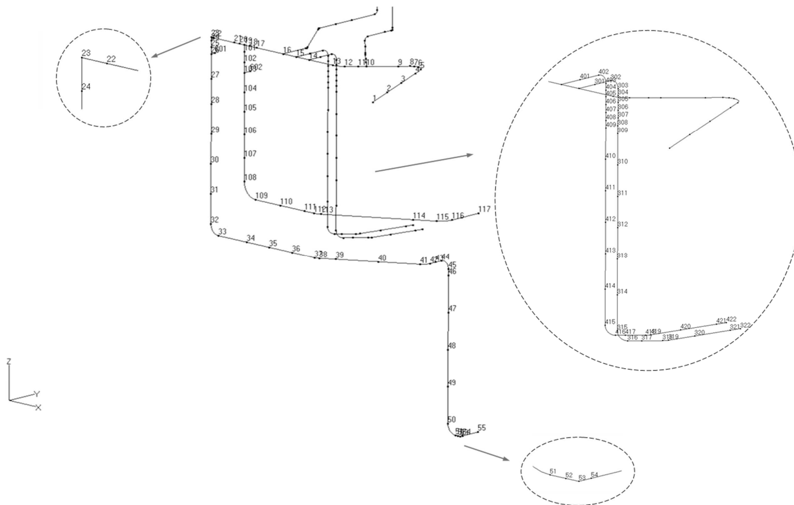
第 3.122 図 貫通部配管 P112 (CV 内) の解析モデル図 (節点番号 1)
