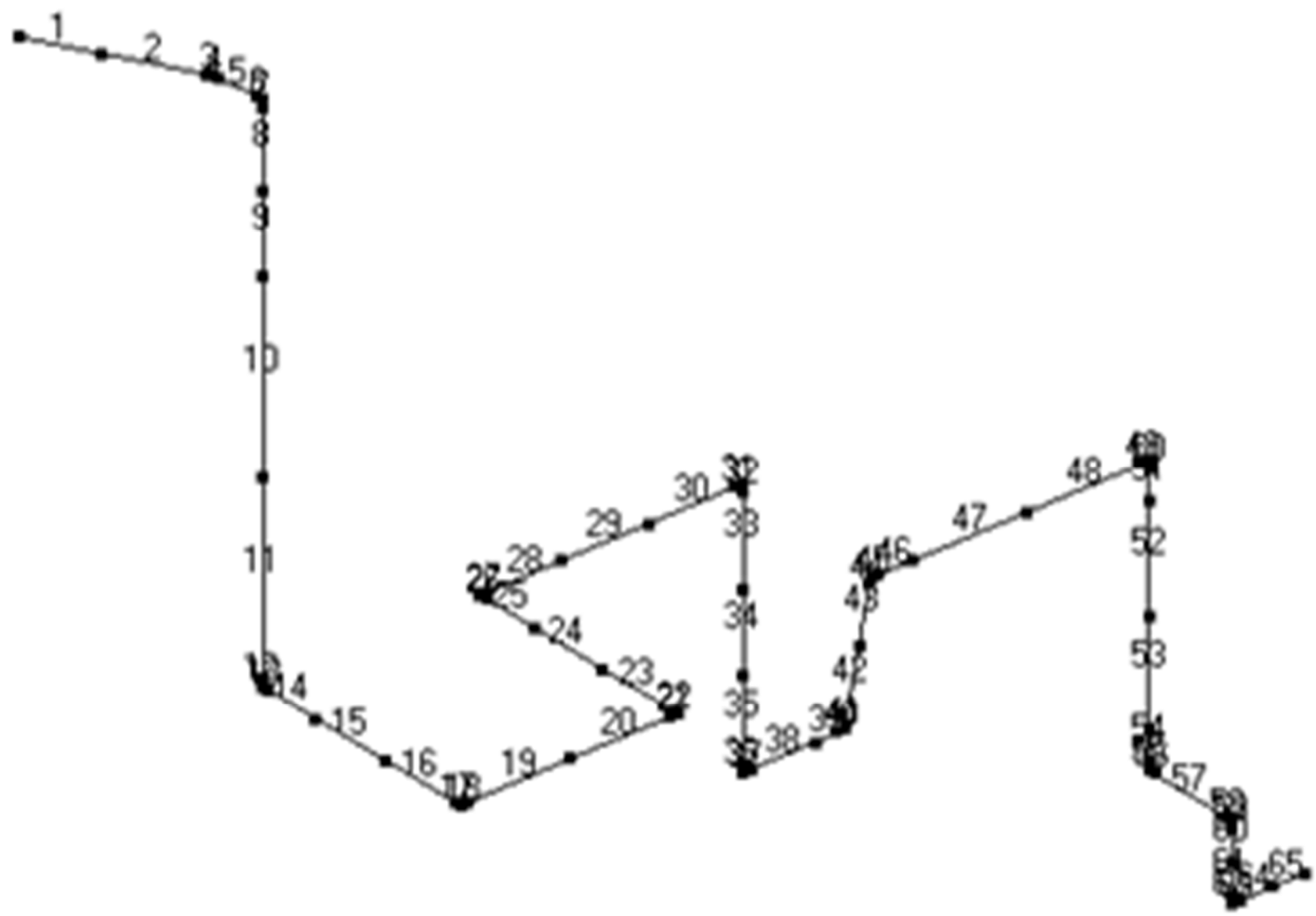
第 3.8 図 貫通部配管 P107 (CV 外) の解析モデル図 (要素番号)
