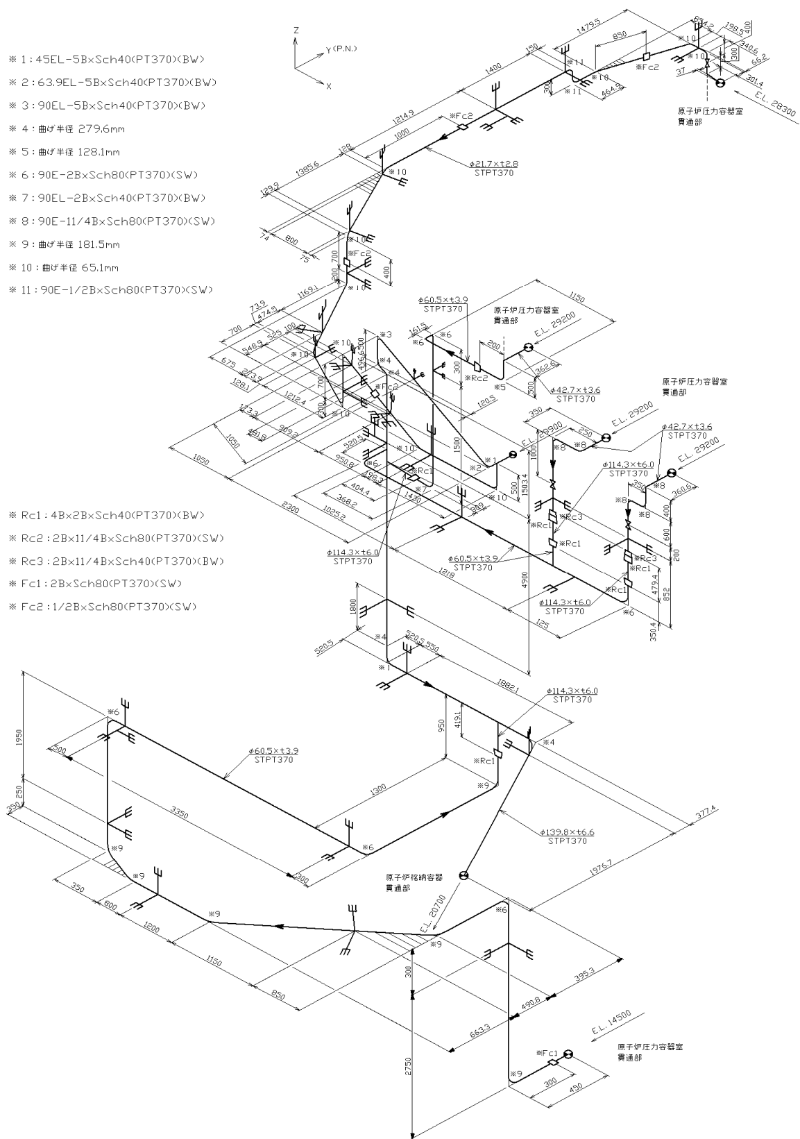
第 3.105 図 貫通部配管 P111(CV 内)のアイソメ図
