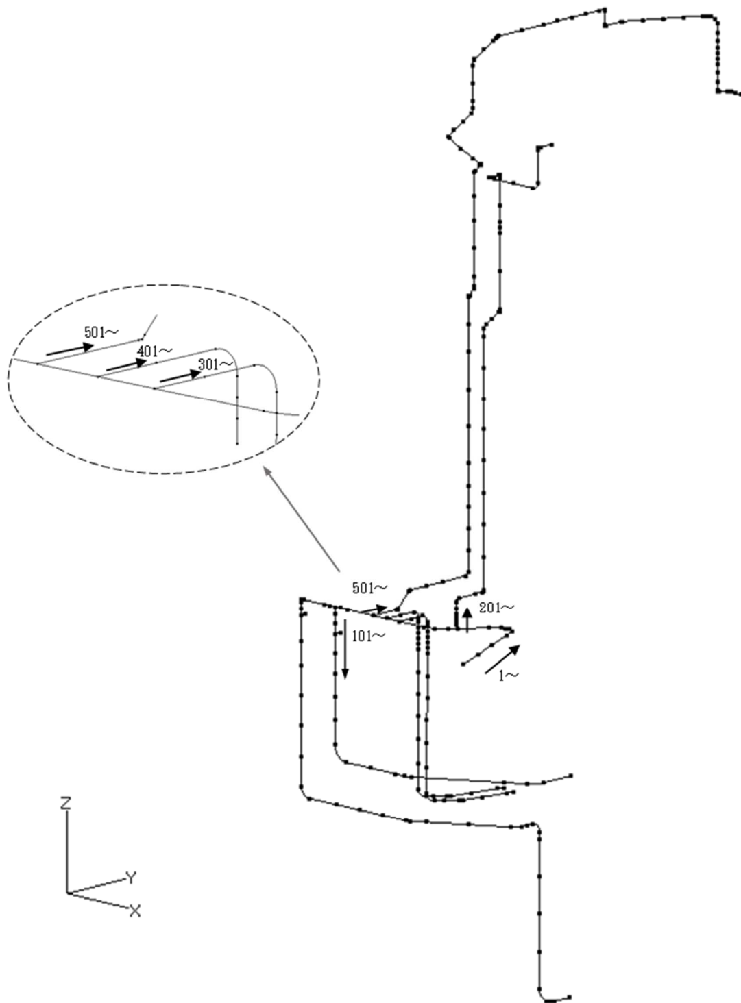
第 3. 121 図 貫通部配管 P112(CV 内)の解析モデル図(全体)
