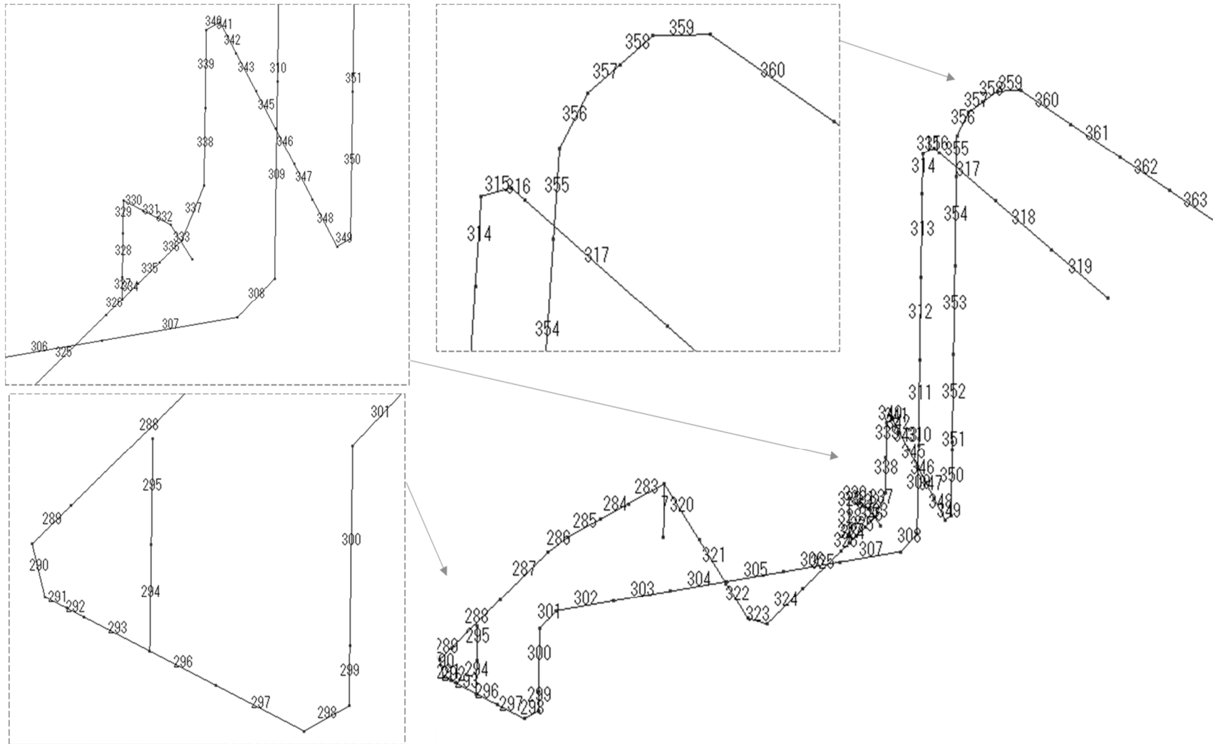
第 3.162 図 貫通部配管 P127(CV 内)の解析モデル図(要素番号)
