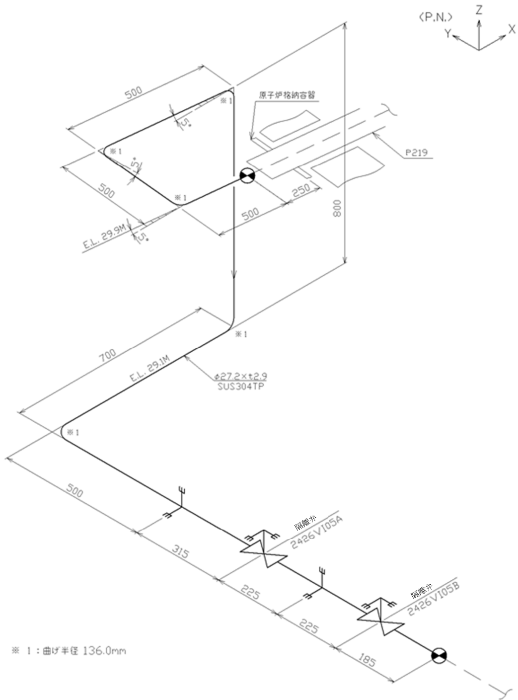
第 3.198 図 貫通部配管 P219 (CV 外) のアイソメ図
