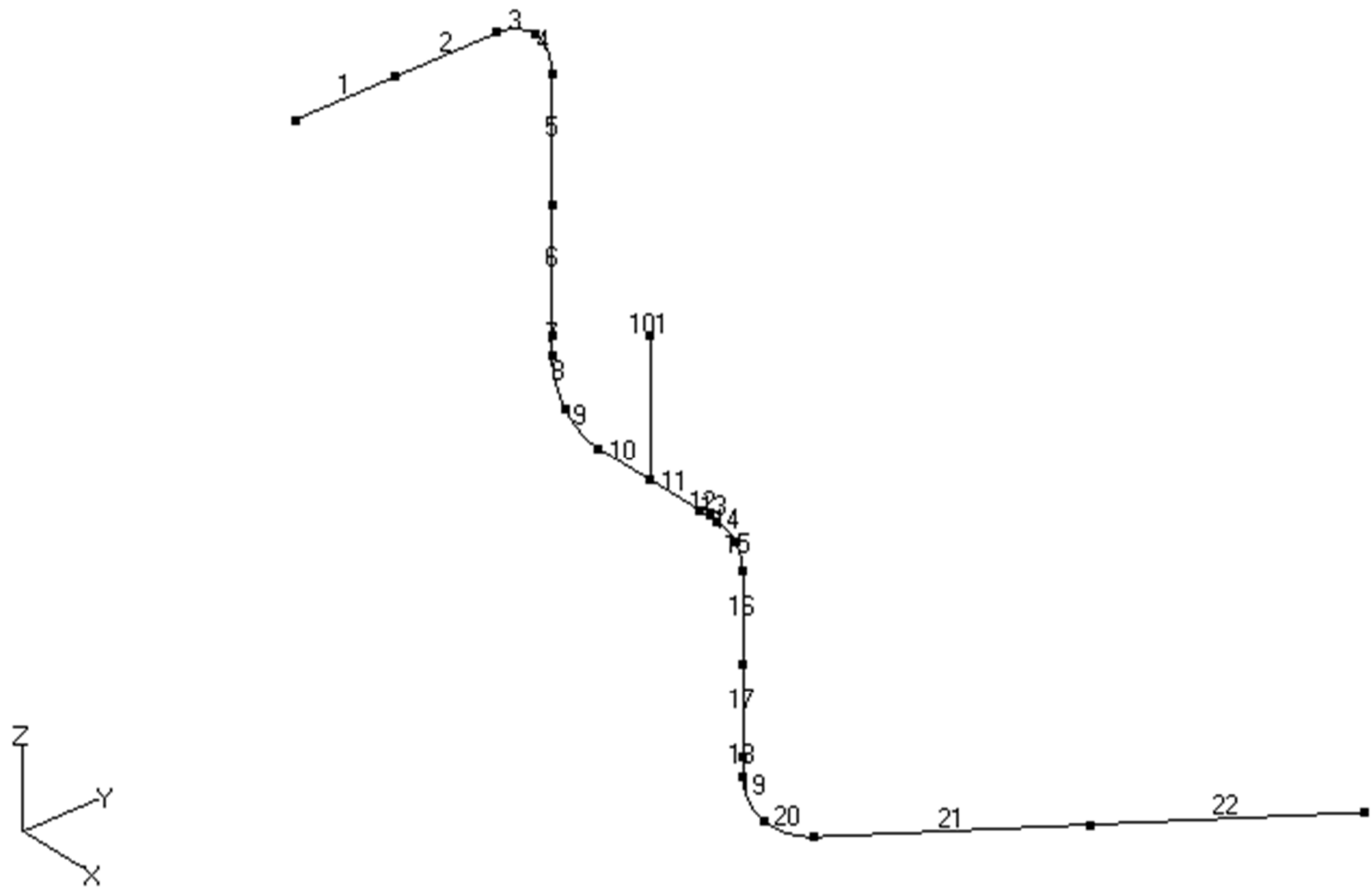
第 3.136 図 貫通部配管 P116(CV 外)の解析モデル図(要素番号)
