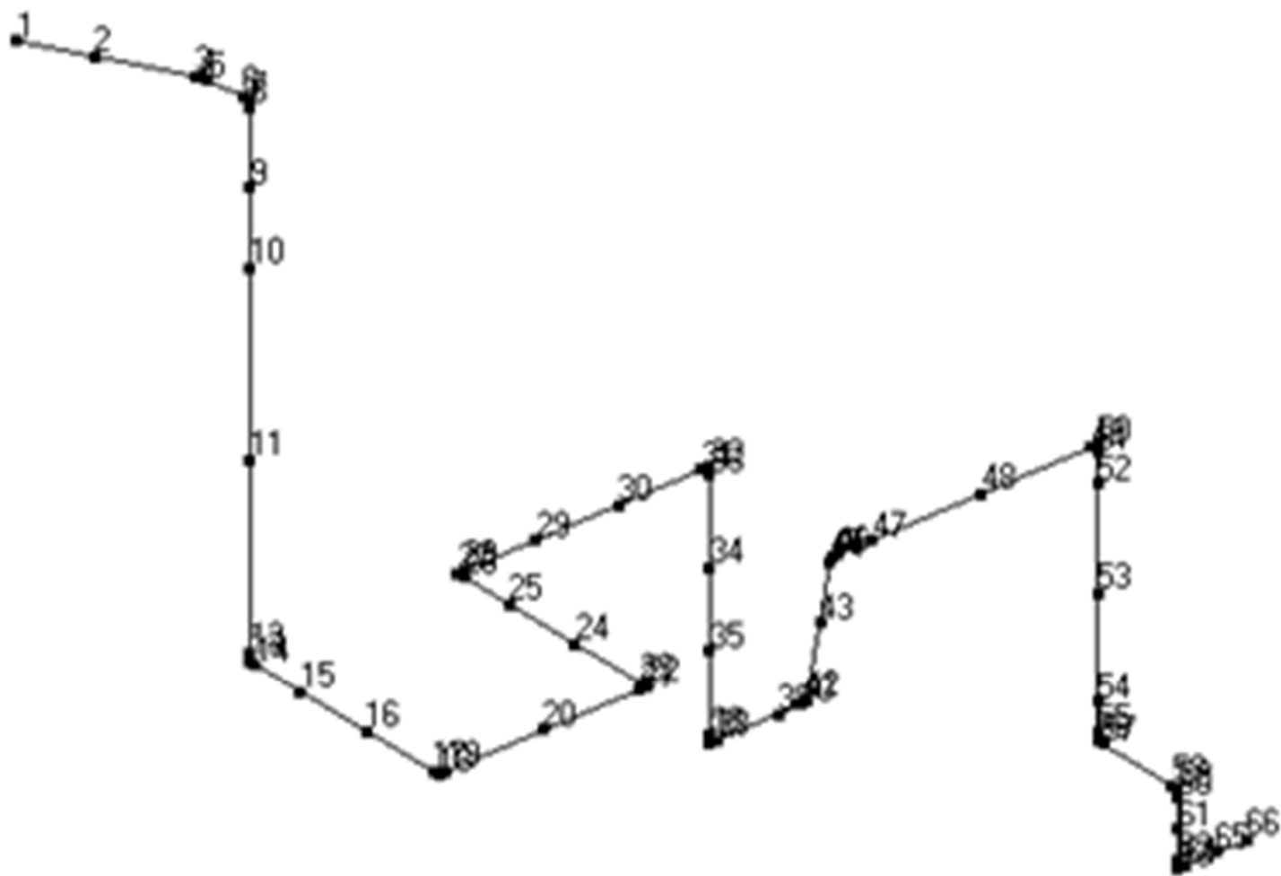
第 3.7 図 貫通部配管 P107 (CV 外) の解析モデル図 (節点番号)
