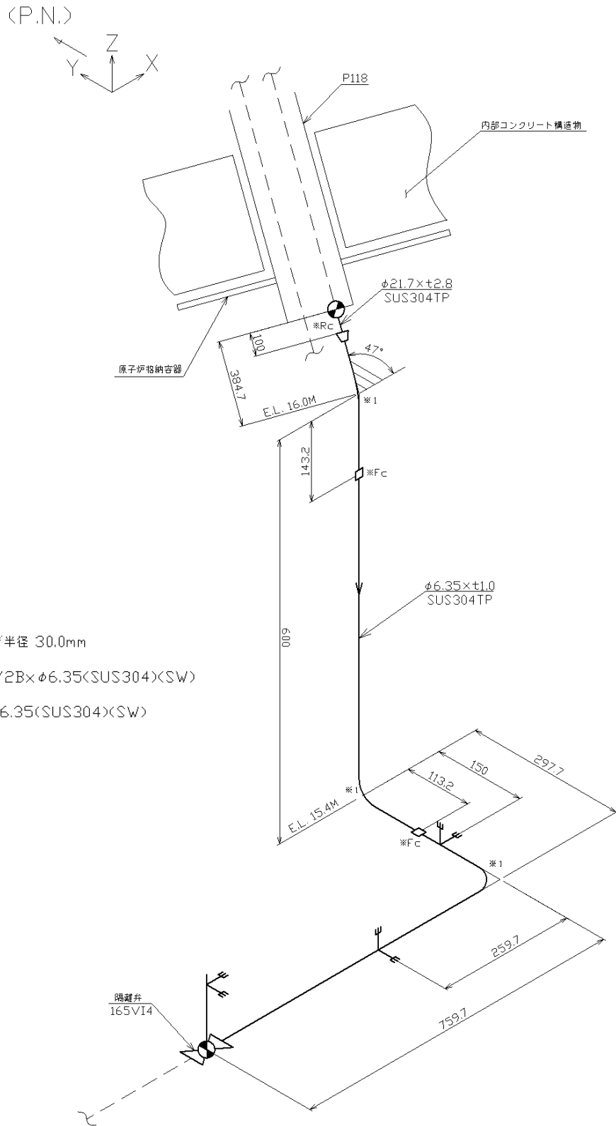
第 3.33 図 貫通部配管 P118 その 1 (CV 外) のアイソメ図
