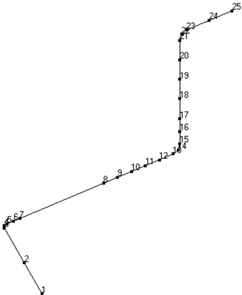
第 3.75 図 貫通部配管 P104 (CV 外) の解析モデル図 (節点番号)
