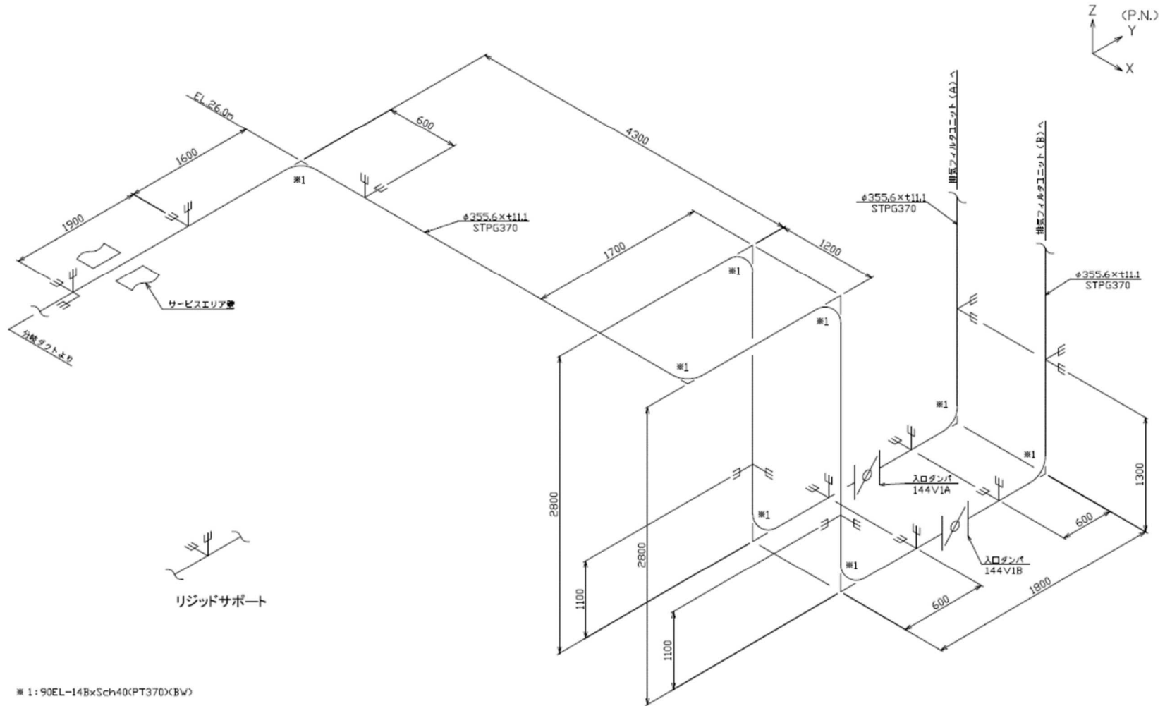
第 3.204 図 非常用空気浄化設備主ダクトのアイソメ図
