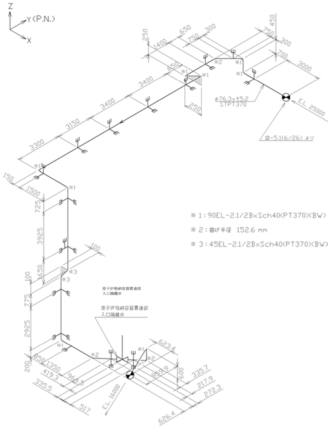
第 3.146 図 貫通部配管 P125 (CV 外) のアイソメ図
