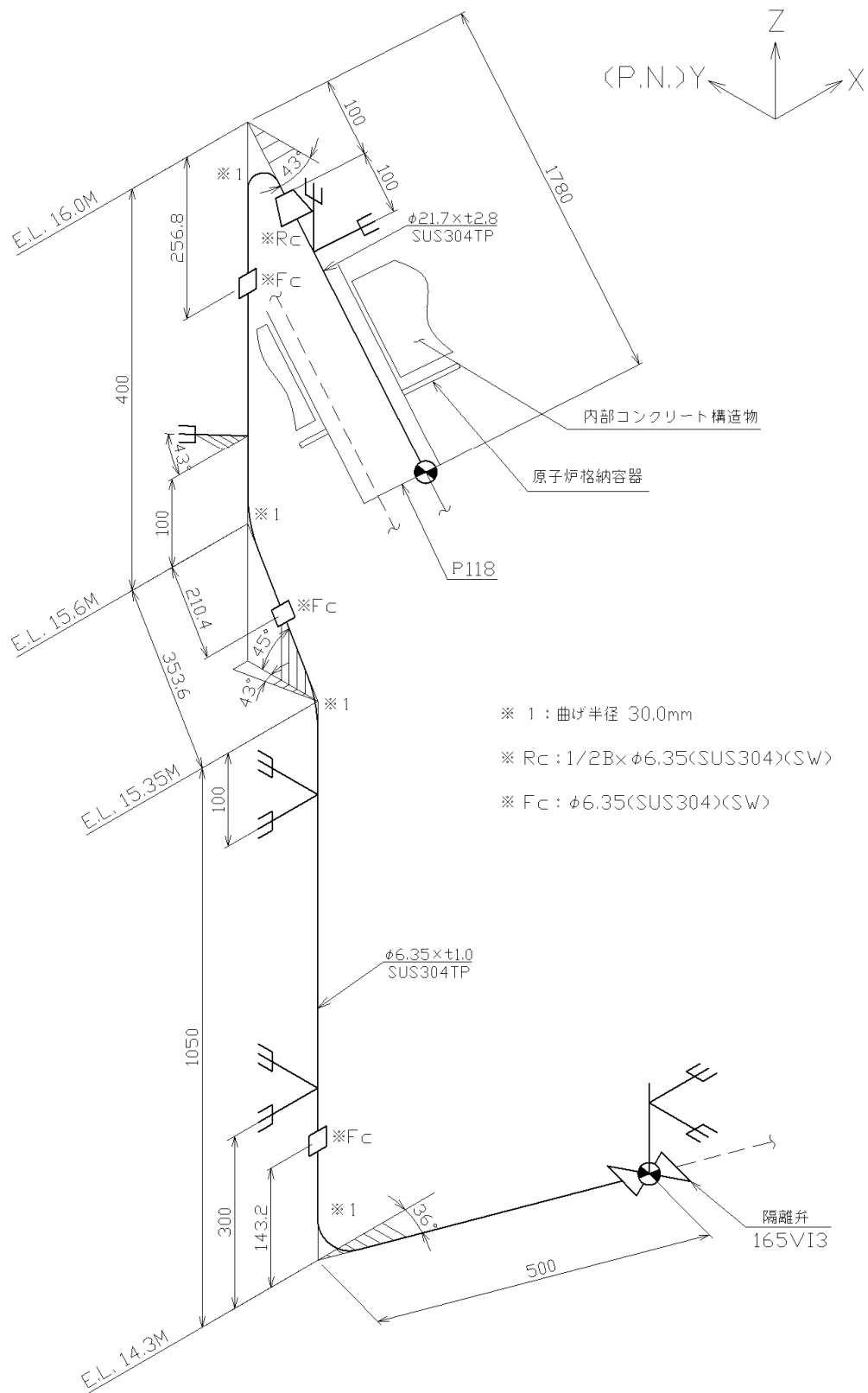
第 3.36 図 貫通部配管 P118 その 1 (CV 内) のアイソメ図
