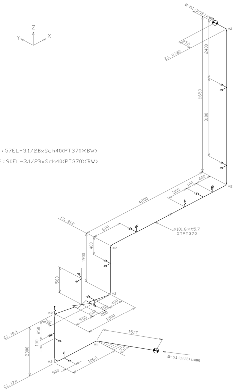
第 3.151 図 貫通部配管 P126 (CV 外) のアイソメ図
