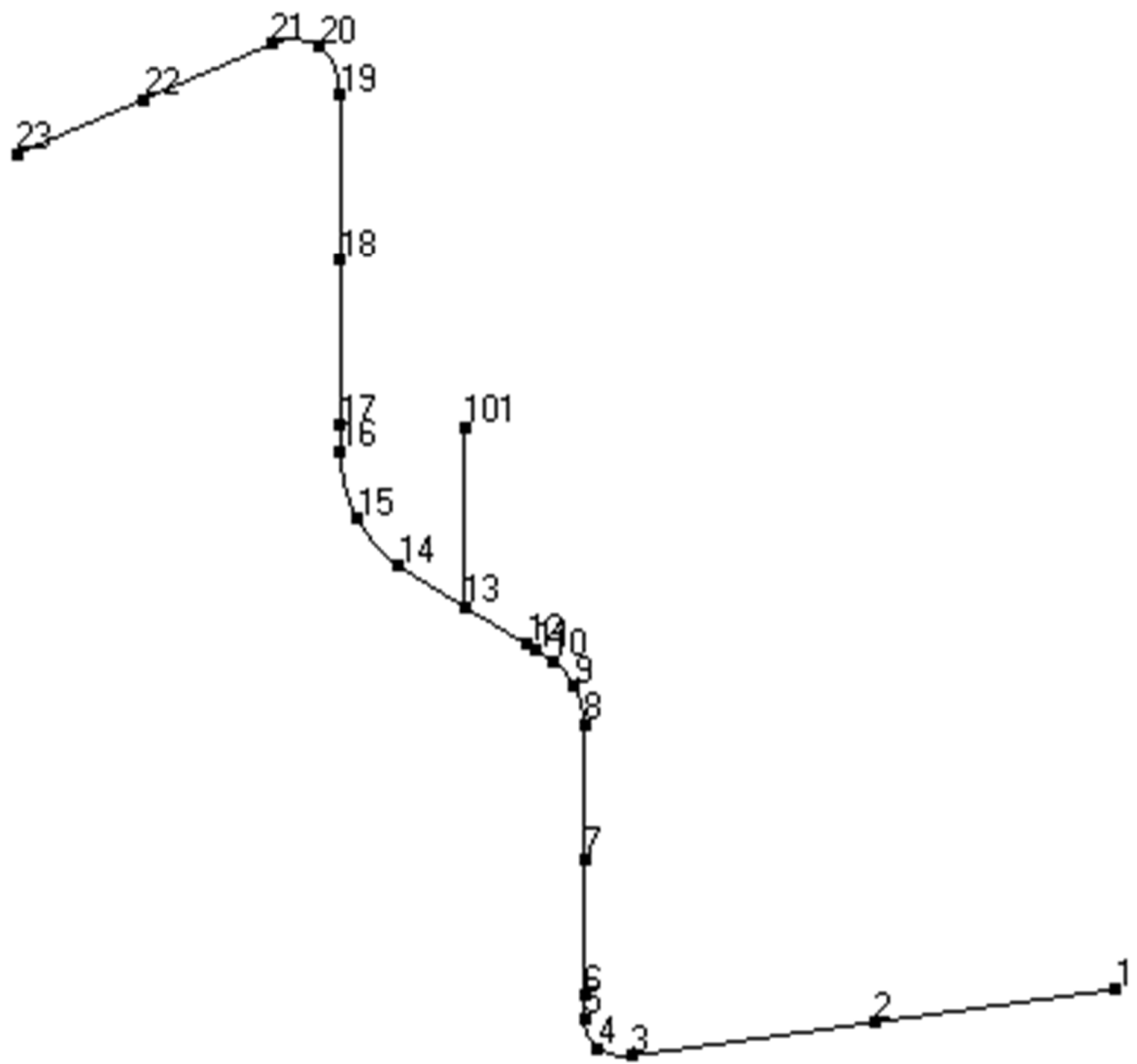
第 3. 132 図 貫通部配管 P115 (CV 外) の解析モデル図 (節点番号)
