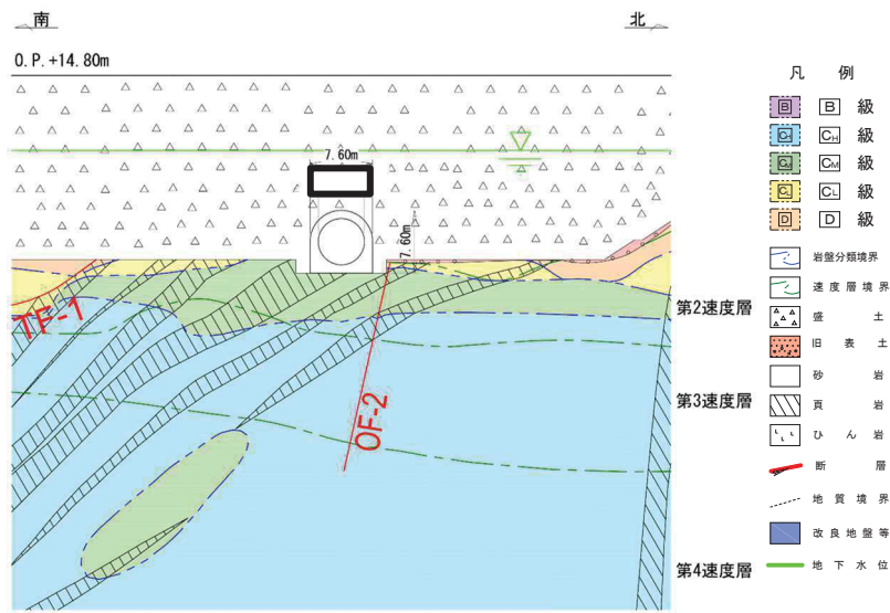
図 4.5-8 排気筒連絡ダクト（土砂部） 評価対象断面図（断面①）
