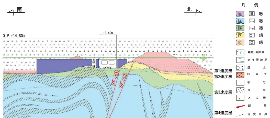
図 4.12-11 取水路（標準部）地質断面図（断面⑥：曲線部）
