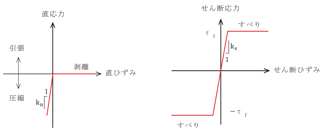
図 7-1 ジョイント要素の力学特性
