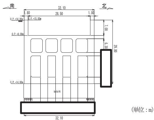
図 4.15-4 第 3 号機海水ポンプ室断面図 (B-B)
