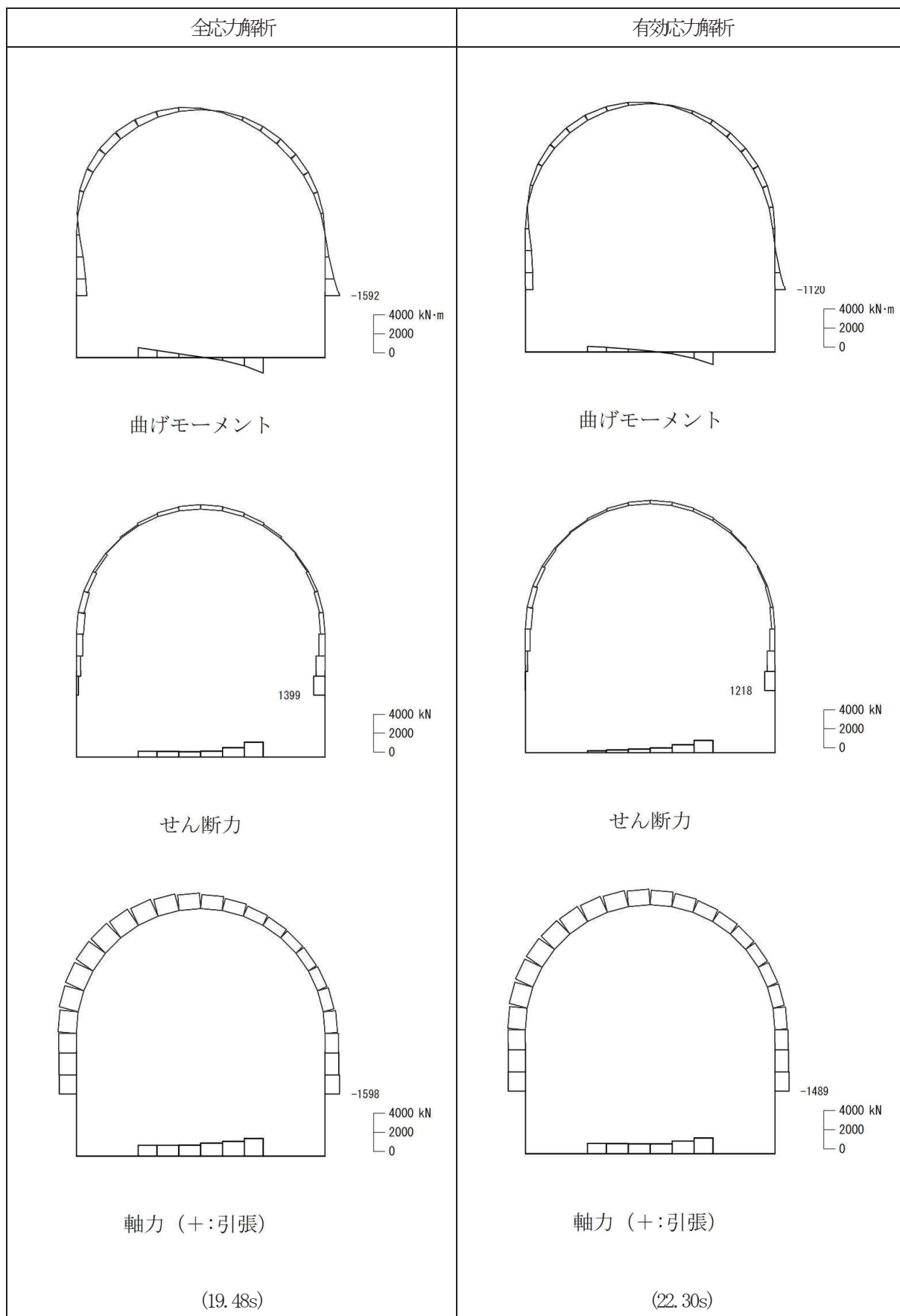
図 3.1-4 断面力図 (S s - F 1 )
