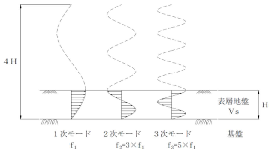
図 9.1-2 せん断振動の固有振動モード
