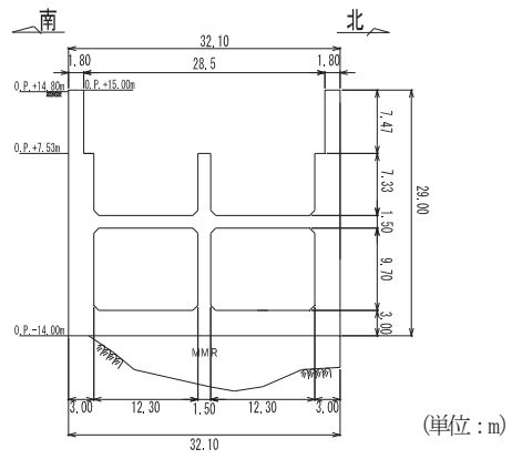
図 4.15-5 第 3 号機海水ポンプ室断面図 (C-C)
