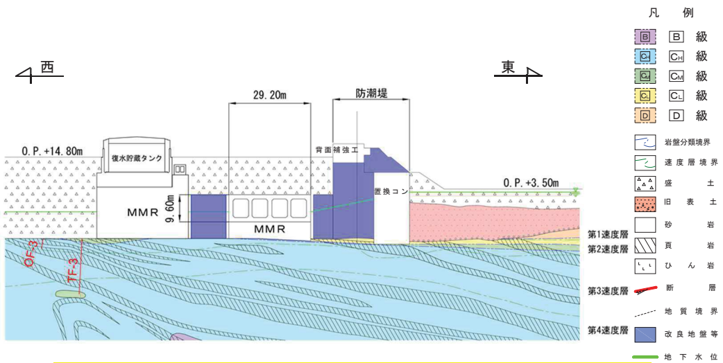
図 4.7-10 取水路（漸拡部）地質断面図（D-D 断面：断面③）
