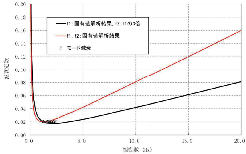
図 9.1-3 Rayleigh 減衰の設定例の比較
