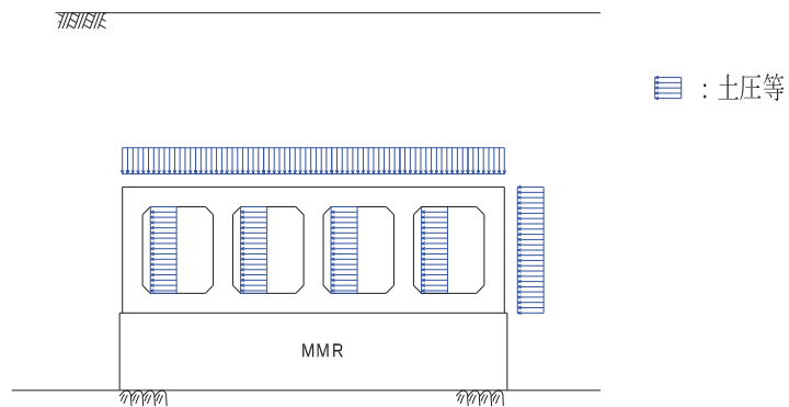
図 4.7-11 荷重イメージ図
