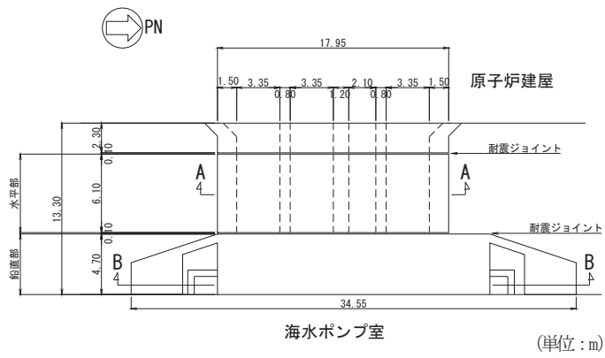
図 4.6-2 原子炉機器冷却海水配管ダクト平面図
