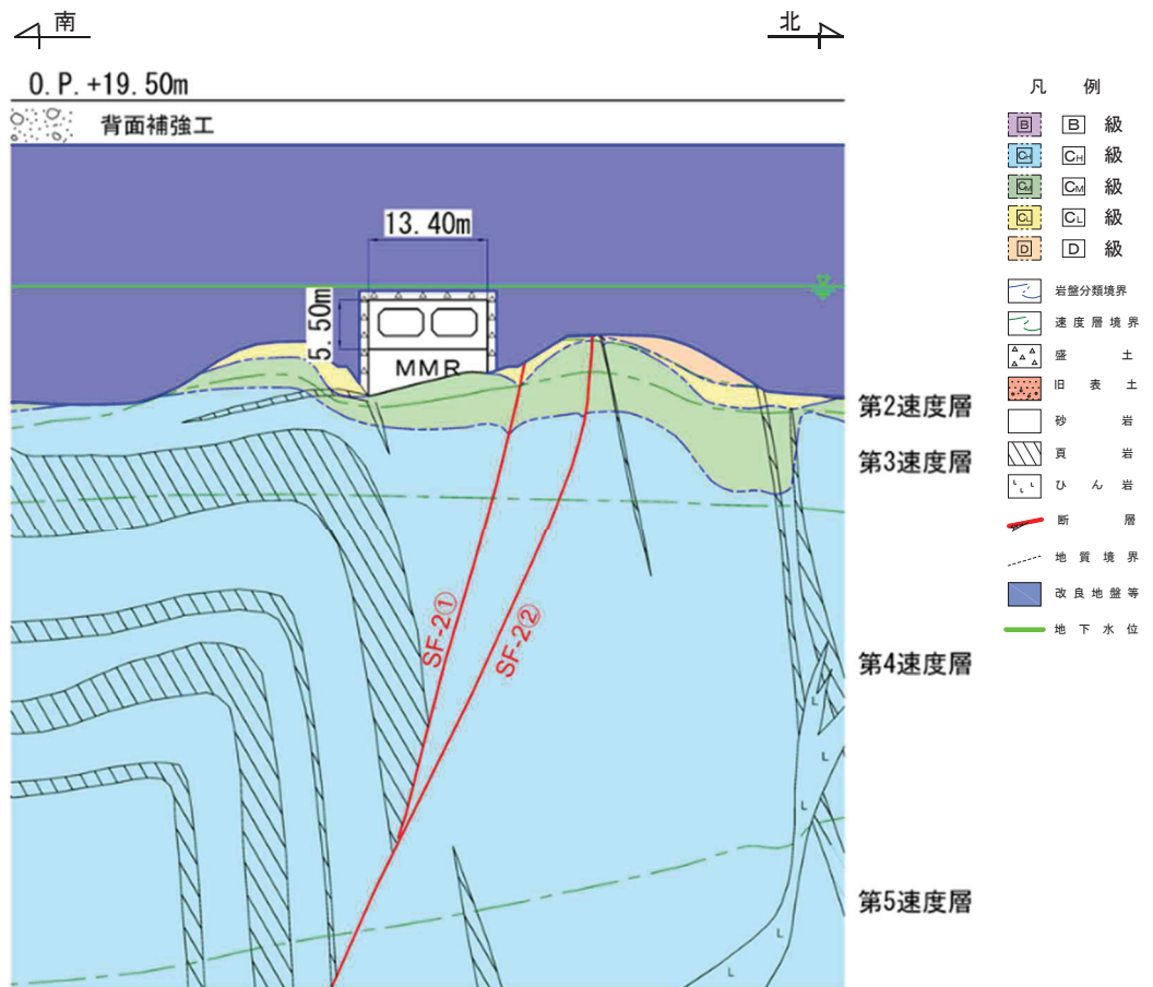
図 4.12-10 取水路（標準部）地質断面図（断面⑤：曲線部）
