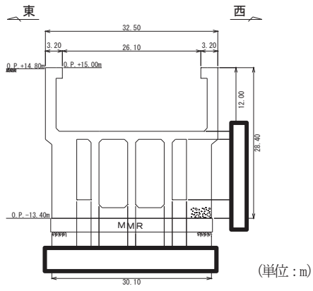
図 4.10-5 海水ポンプ室断面図 (C-C)
