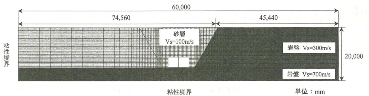
図 2-3 ケース 3 の解析モデル
