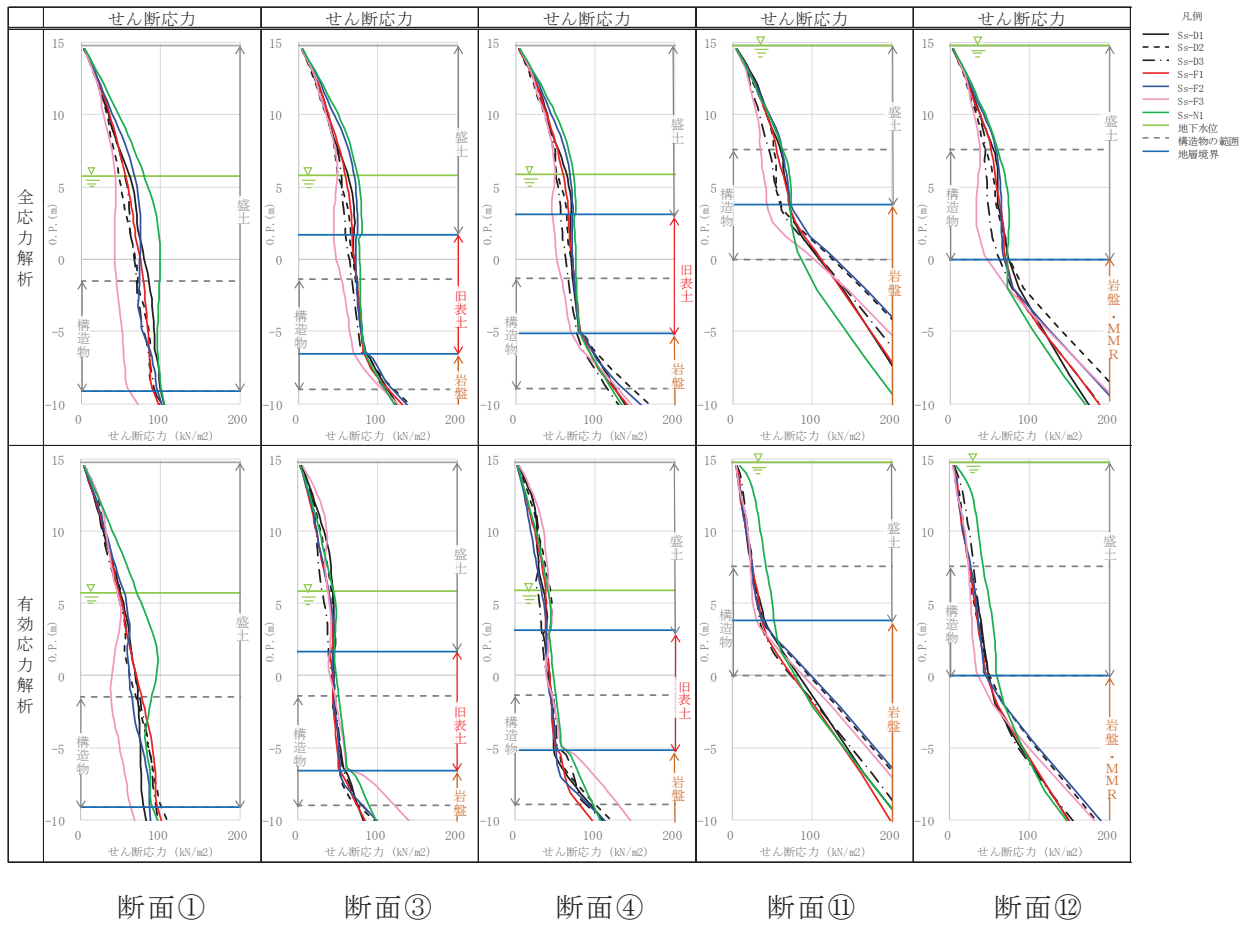
図 1-2 せん断応力分布 (全時刻最大)
