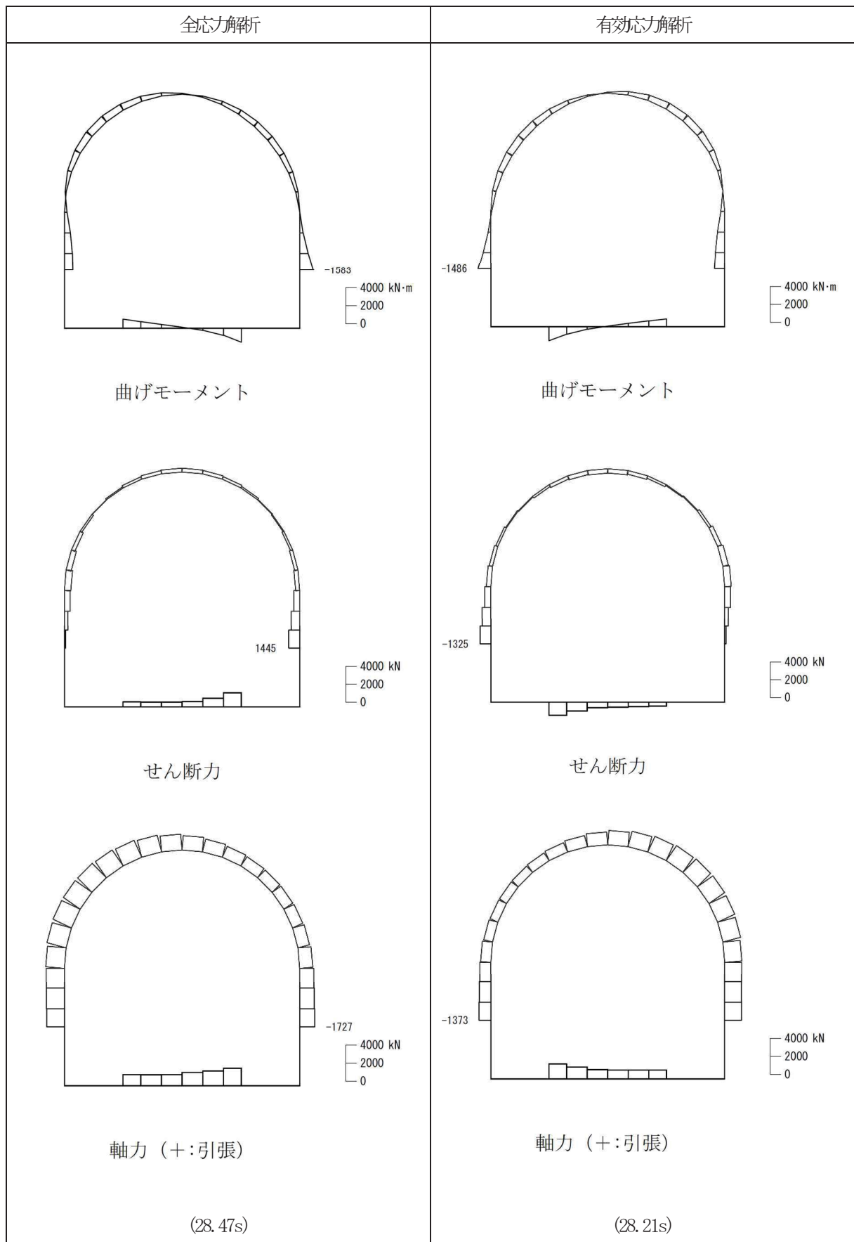
図 3.1-5 断面力図 (S s - F 2)
