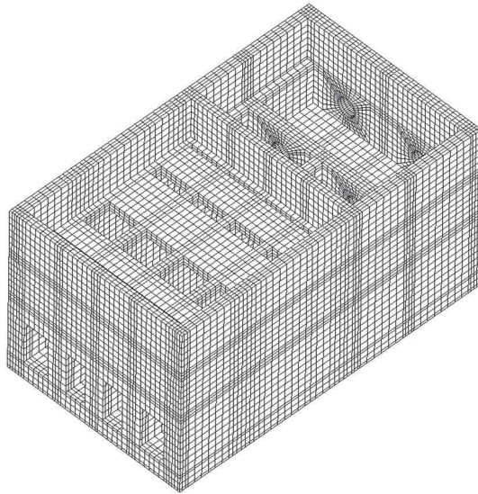
図 4.15-6 第 3 号機海水ポンプ室 三次元モデル図
