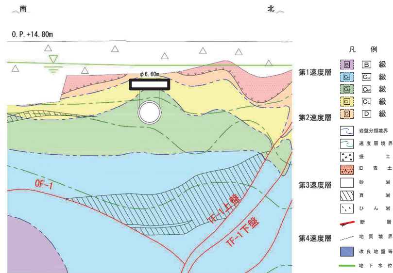
図 4.5-6 排気筒連絡ダクト（土砂部）地質断面図（B-B 断面）
