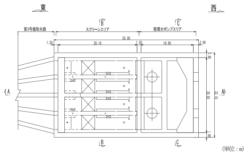
図 4.15-2 第 3 号機海水ポンプ室平面図
