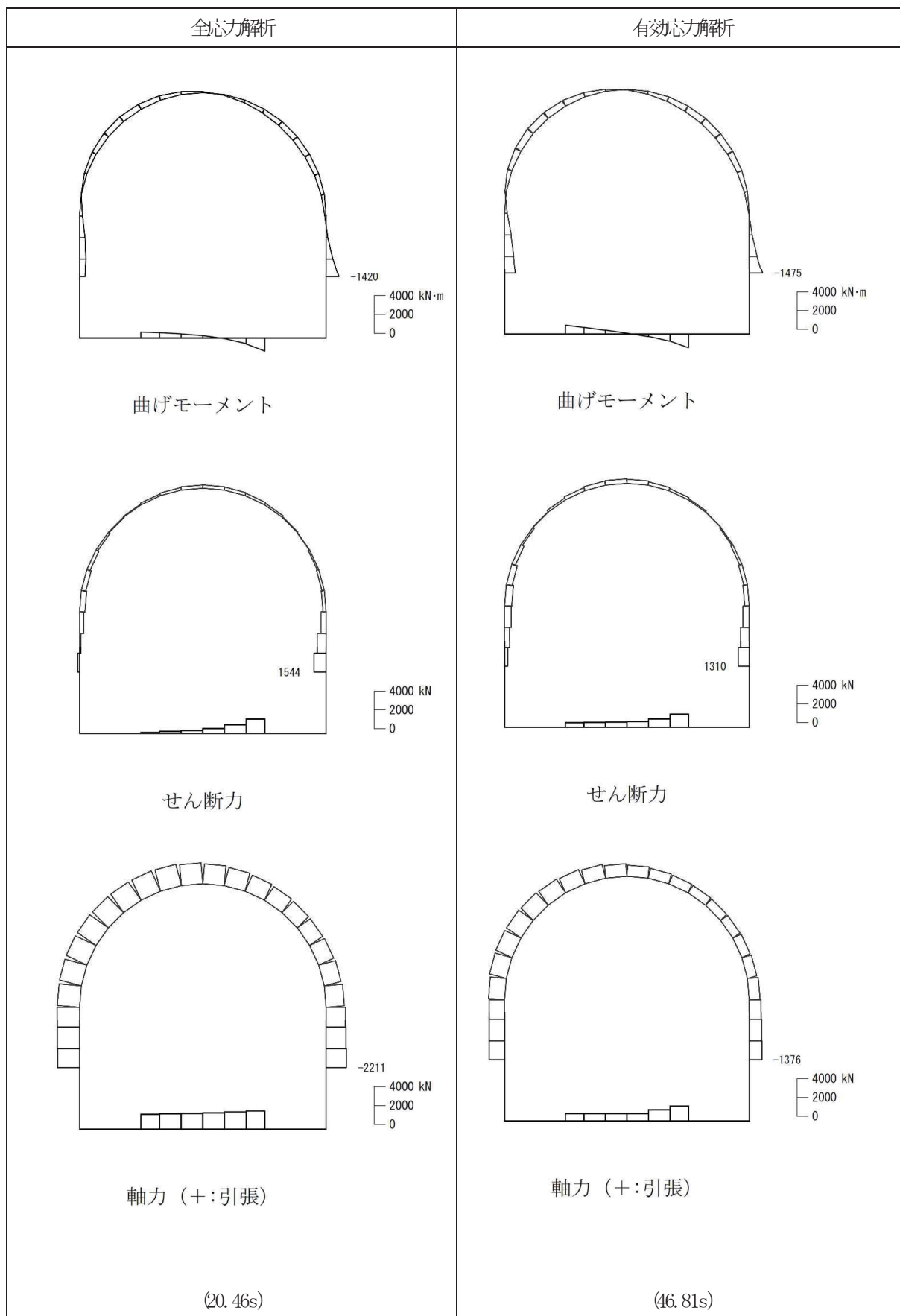
図 3.1-1 断面力図 (S s - D 1)
