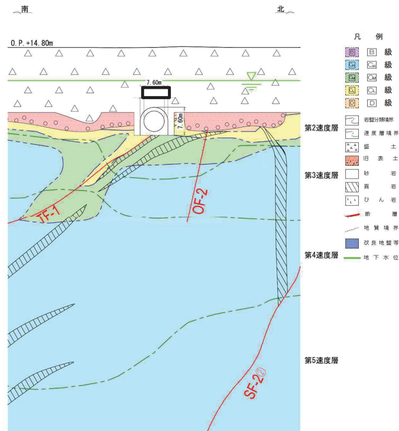
図 4.5-9 排気筒連絡ダクト（土砂部） 評価対象断面図（断面②）
