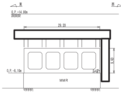
図 4.7-4 取水路 (漸拡部) 断面図 (A-A)
