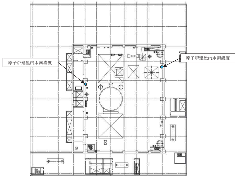
図 2.3.1-1 原子炉建屋内水素濃度検出器配置図 (原子炉建屋地上3階 (原子炉建屋燃料取替床))
