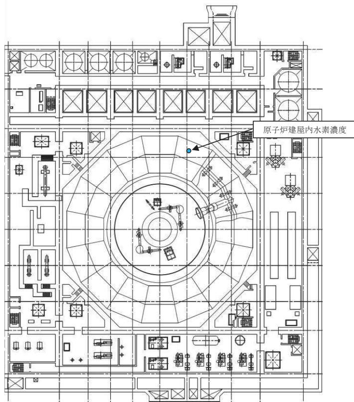
図 2.3.1-4 原子炉建屋内水素濃度検出器配置図 (原子炉建屋地下2階)
