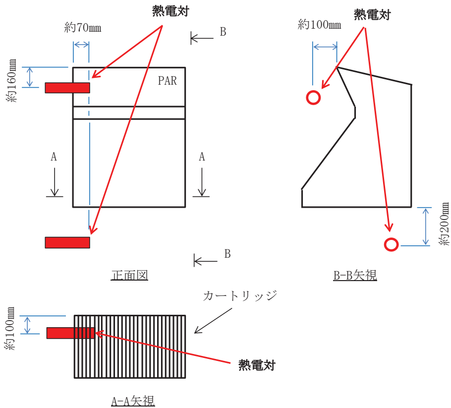
図 4.2.1-2 静的触媒式水素再結合装置動作監視装置の概略構成図
