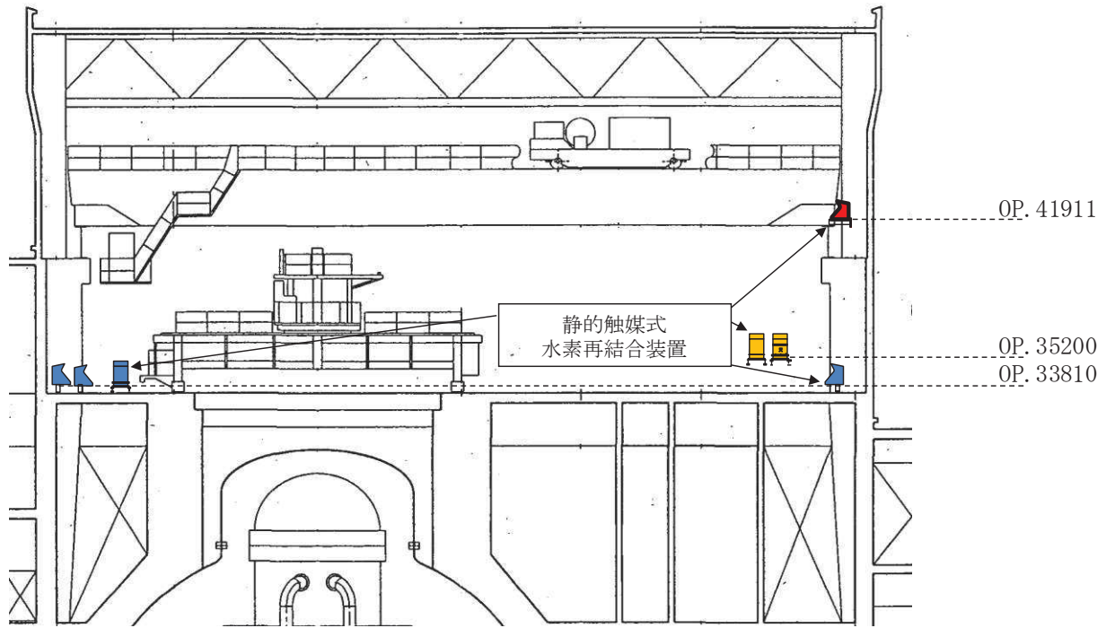
图 4.2.1-1 静的触媒式水素再結合装置概略設置図 (2/2)
