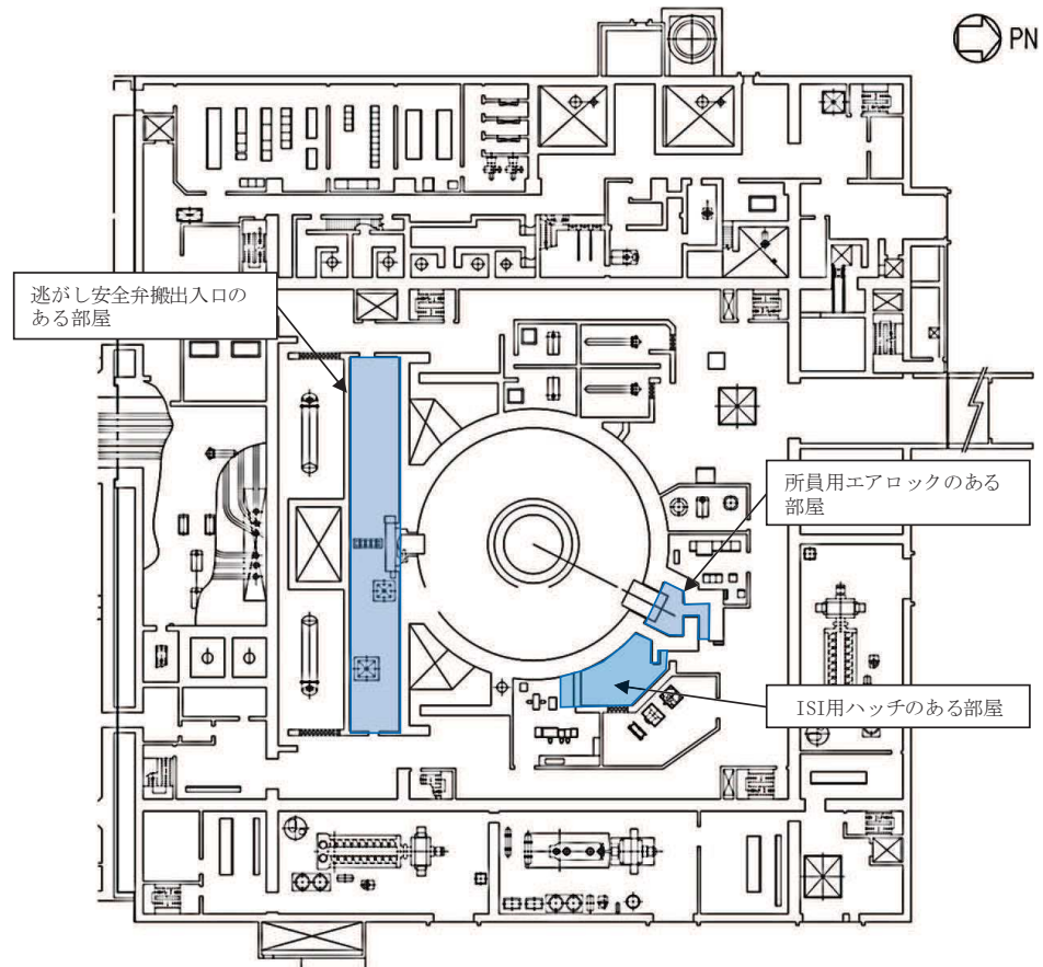
図 2.2.1-9 原子炉建屋原子炉棟地上 1 階
