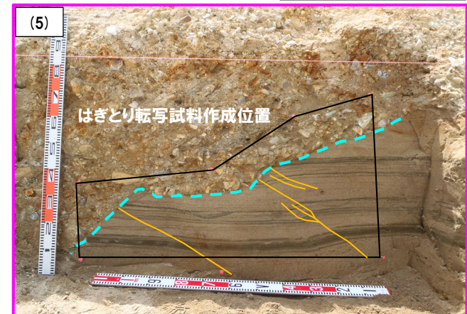
R2.6南側壁面追加はぎとり転写試料採取時露頭 (次頁～P463参照)
