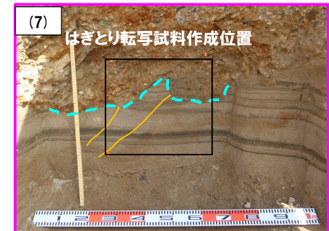
R2.6北側壁面追加はぎとり転写試料採取時壁面 (次頁～P458参照)
