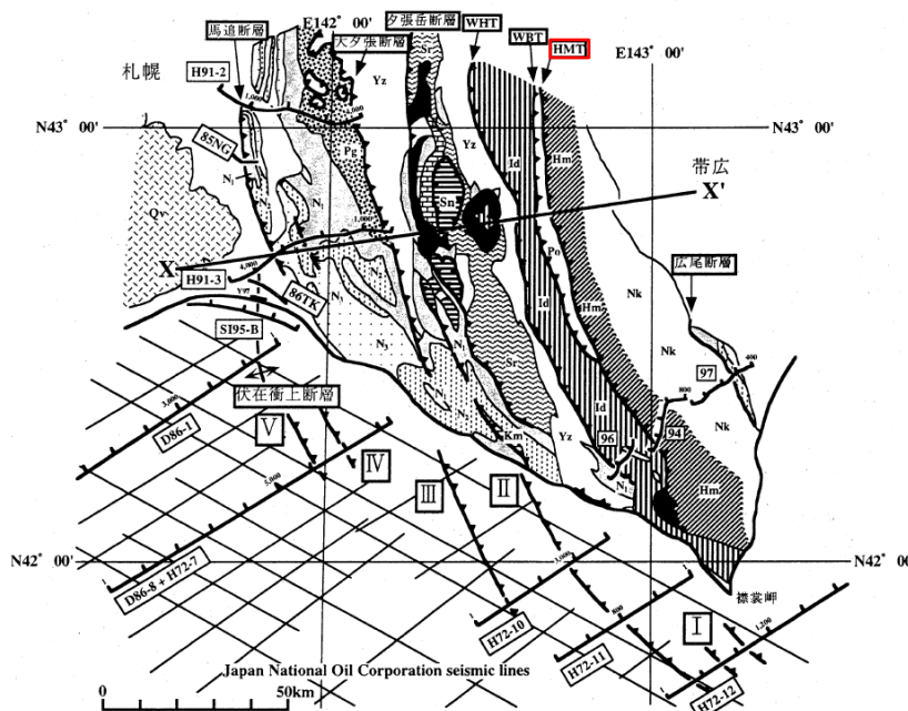
図1 日高衝突帯ならびに前縁褶曲・衝上断層帯の地質概略と主な反射法地震探査測線図。X-X'は図2の断面位置を示す。伊藤ら(1999)を改変。 【地質】主として、地質調査所(1982,1996)による。Nk:中の川層群, Hm:日高変成岩類(主帯), Po:ボロシリ・オフィオライト(西帯), Id:イドンナップ帯, Yz:蝦夷層群, Sr:空知層群, Km:神威古潭変成岩類, Sn:沙流川層-ニセウ層, Pg:古第三系, N1~N3:地質調査所(1982)と同じ。Qv:第四紀火山岩類。HMT:日高主衝上断層, WBT:西縁衝上断層, WHT:日高西部断層群 【測線】94・96・97:日高深部構造反射法探査, 85NG・86TK:浅野ら(1990), Y97:佐藤ら(1998), その他の測線は石油公団(1973,1987,1993,1996)。
