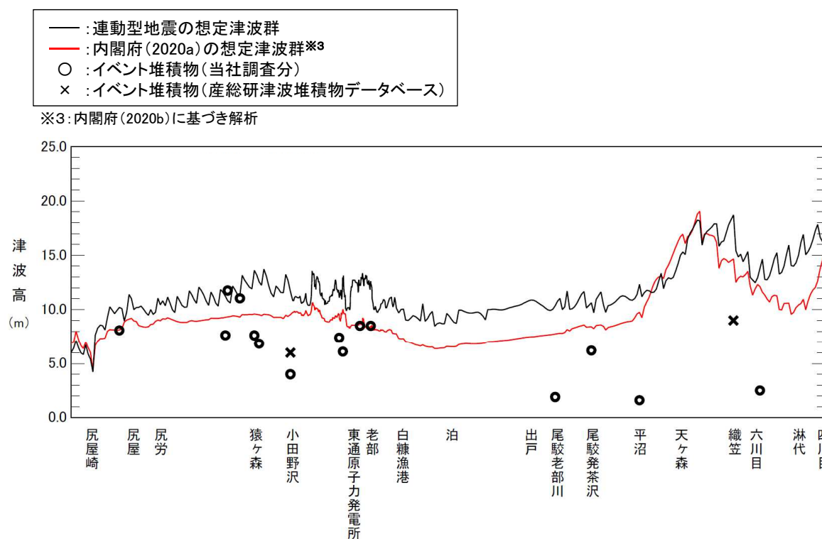
青森県北部太平洋沿岸の汀線位置における 十勝沖・根室沖から岩手県沖北部の連動型地震の想定津波群と 内閣府(2020a)による日本海溝(三陸・日高沖)モデルの想定津波群の比較
