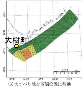
千島海溝沿いの概略パラメータスタディの断層モデル (土木学会(2016)に一部加筆)
