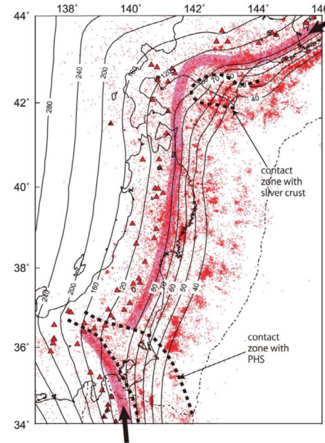
太平洋スラブ地殻内の地震の分布 (長谷川ほか(2012)) 赤点:プレート境界から下方に0~10kmの範囲の地震 ピンク色の網目:上面地震帯 黒線:太平洋スラブ上部境界面の形状 黒点線:太平洋スラブが直上のフィリピン海スラブ及び前弧スリバー地殻と接触している領域
