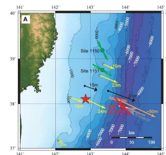
掘削同時検層地点 (Lin et al. (2013))
