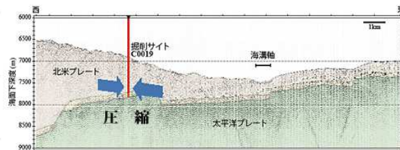
地震前の応力状態
