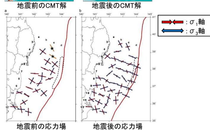
応力テンソルインバージョンから得られた陸のプレートの応力場の変化 (Hasegawa et al. (2012))
