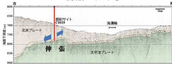
地震後の応力状態
