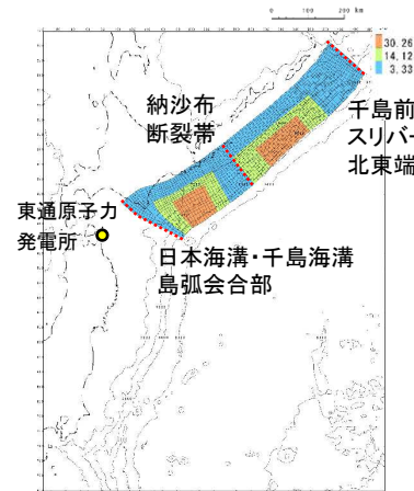
十勝沖・根室沖から千島前弧スリバー北東端の連動型地震
