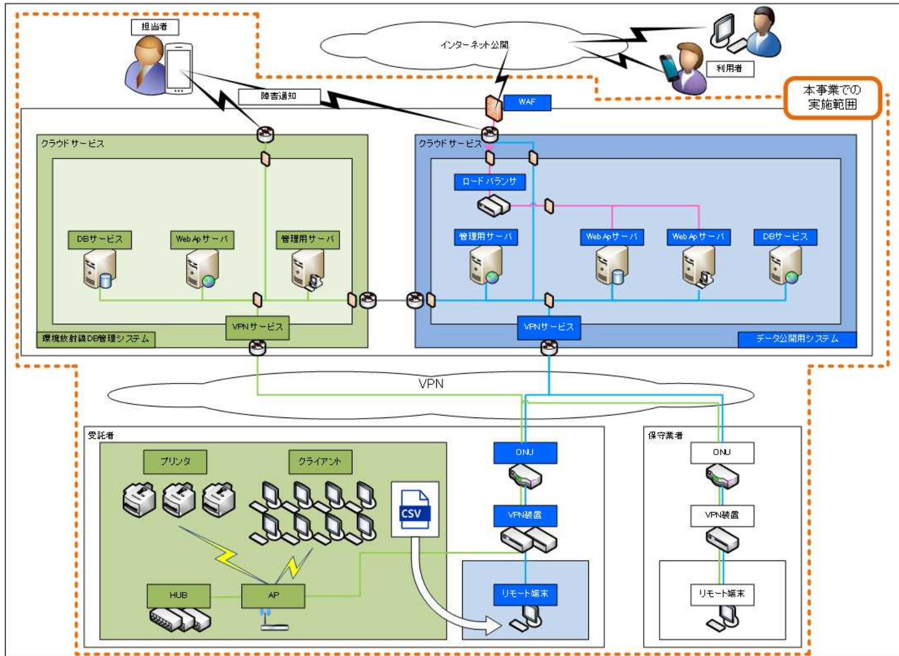
環境放射線データベース管理システム及びデータ公開用システムの構成図
