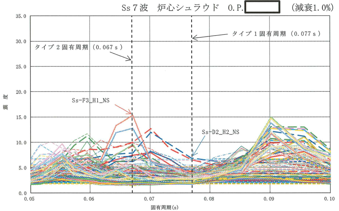
図 2-5 炉心シュラウド支持ロッド固有周期における床応答曲線最大値
