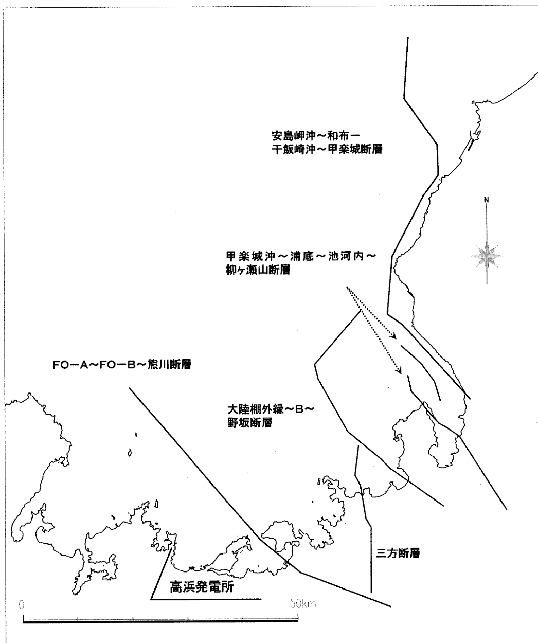
第 3-1 図 敷地周辺の海域における検討対象断層
