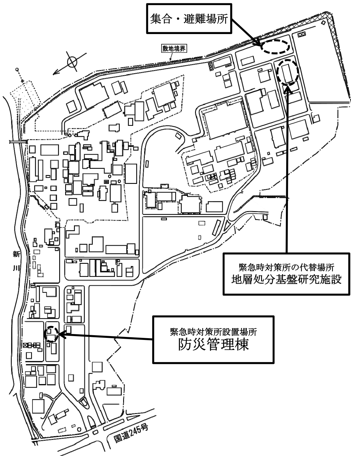
別図－5 サイクル研究所緊急時対策所配置図
