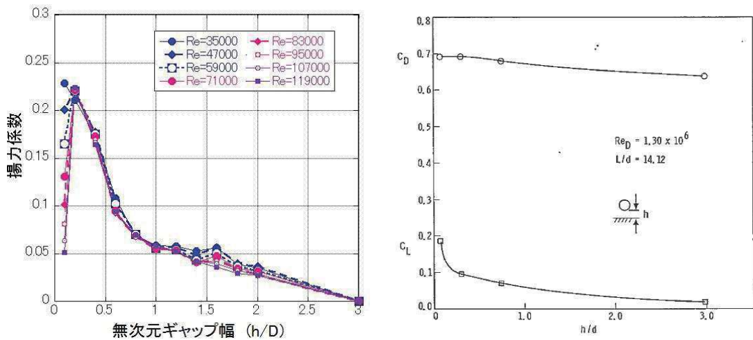
図 19 電力中央研究所の風洞試験 ( Re=3 \times 10^4 \sim 1 \times 10^5 ) (左) と EPRI の風洞試験 (16) ( Re = 1.3 \times 10^6 ) で得られた円柱揚力係数 (右)
