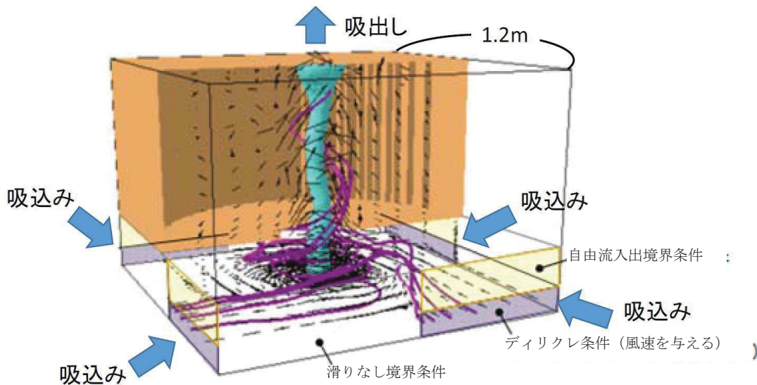
図 8 LES 計算領域内での竜巻状の渦の発生状況
