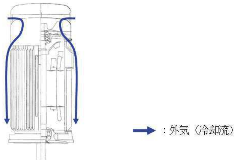
図 1.5-4 高圧炉心スプレイ補機冷却海水ポンプ電動機の冷却方式
