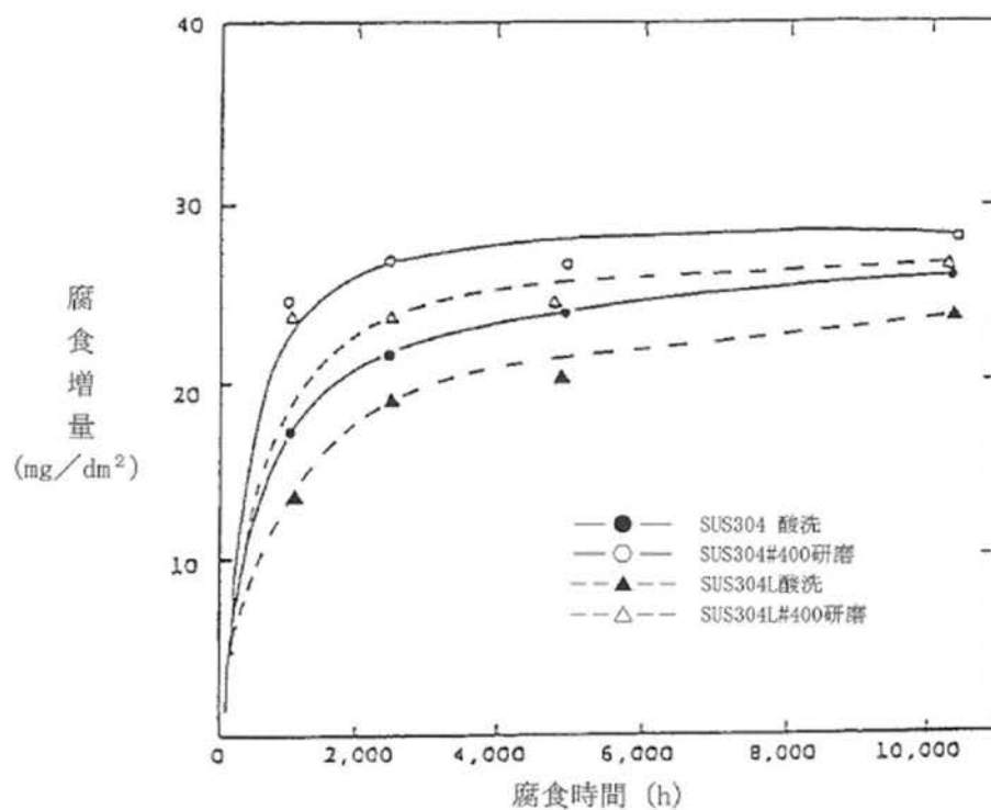
第 8-3 図 SUS304 鋼の高温水中腐食 (試験温度 300^{\circ}\text{C} ) (41)
