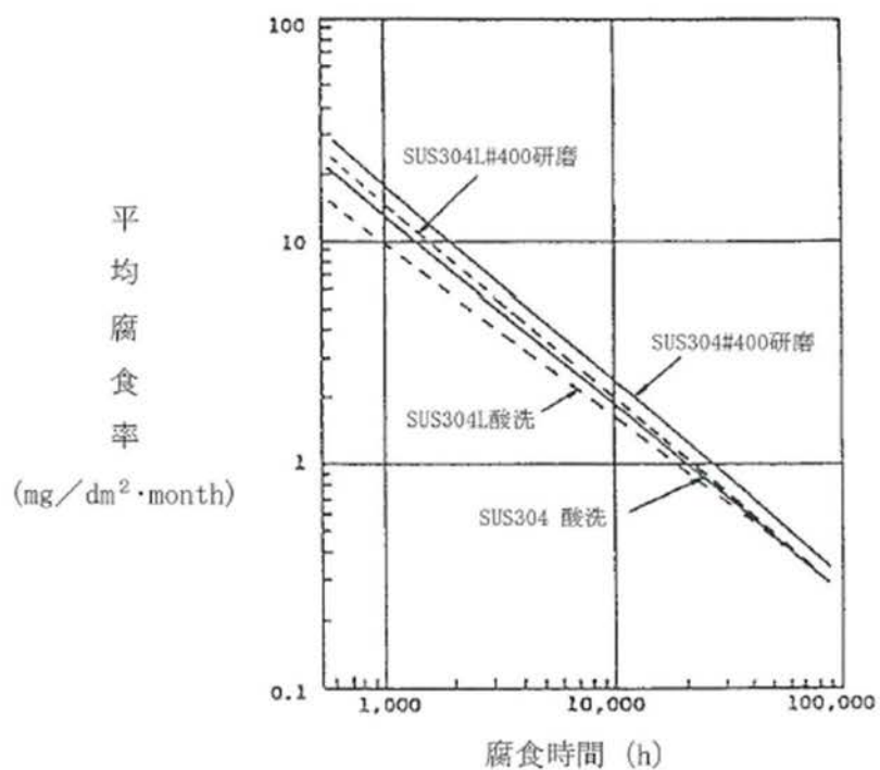
第 8-4 図 SUS304 鋼の溶存酸素を含まない 300^{\circ}\text{C} の 0.92% ホウ酸水中における平均腐食率(41)
