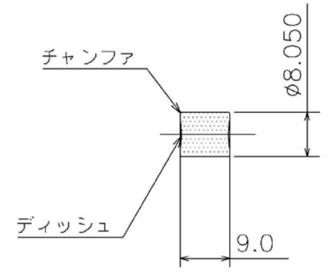
ペレット詳細
