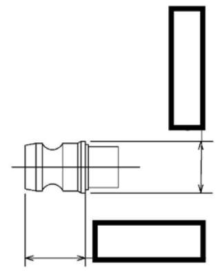
上部端栓詳細
