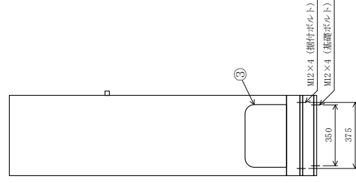
側面図
