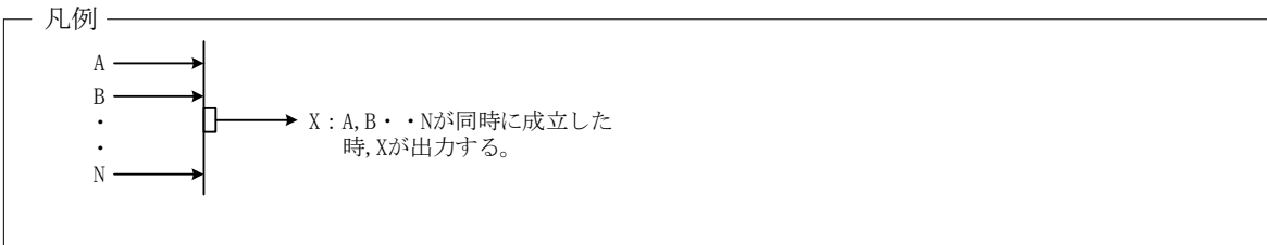
図-1-2-21 UF 6 処理設備（2号一般パージ系コールドトラップ）インターロック （回収側槽類圧力異常上昇によるガス移送停止のインターロック）
