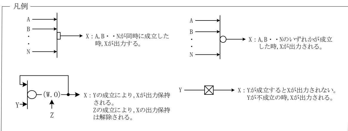
図-1-2-2(3/3) カスケード設備 主要配管 (RE-2A) インターロック (地震発生時のカスケード排気のインターロック)
