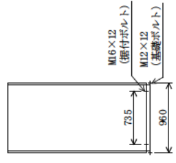
側面図
