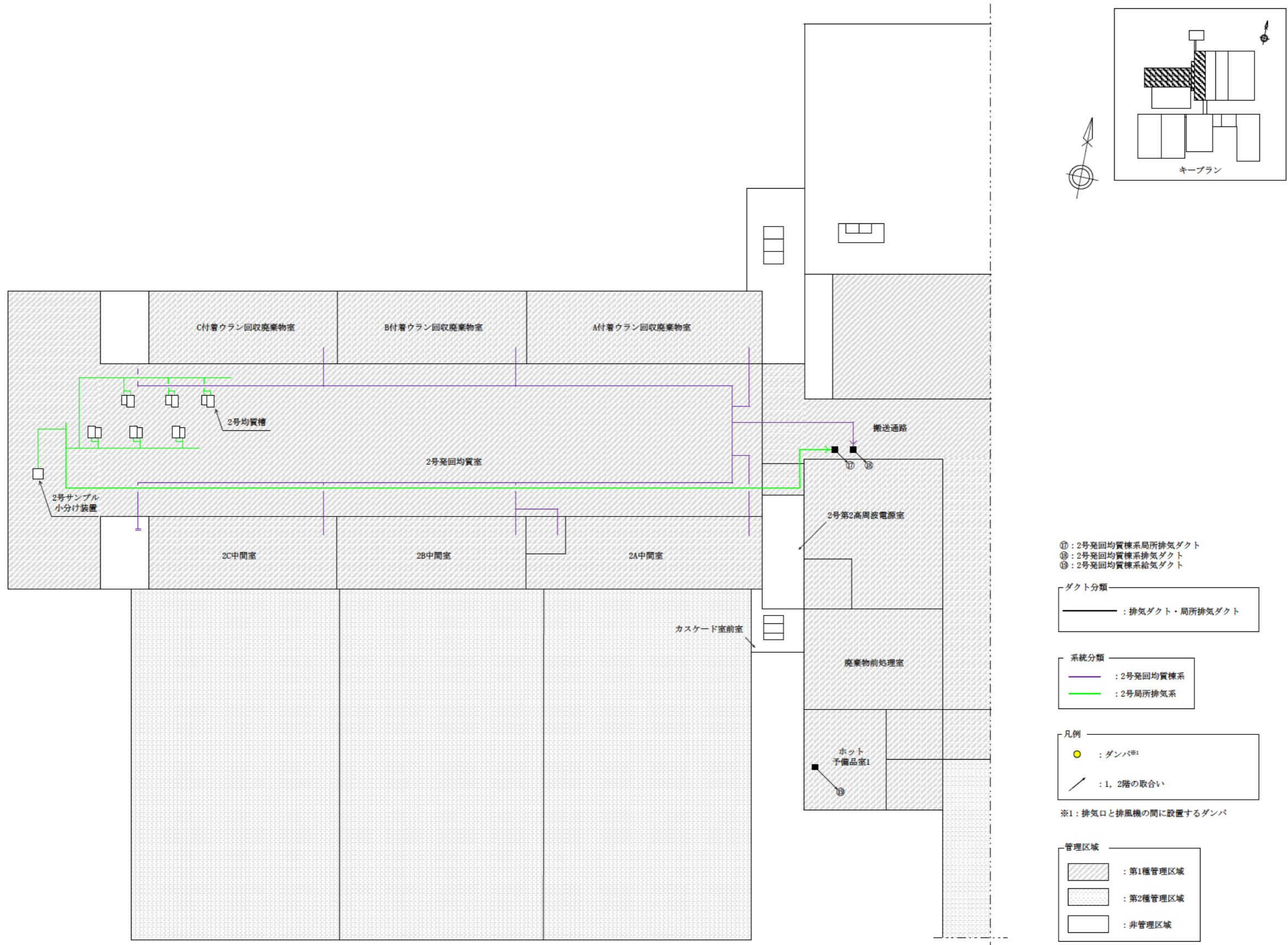
図 1.3.7 気体廃棄物の廃棄設備 系統詳細図 (排気, 局所排気ダクト (1階))
