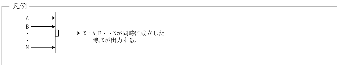
図-1-2-22 UF 6 処理設備（2号一般パージ系コールドトラップ）インターロック （回収側槽類圧力異常上昇によるガス移送停止のインターロック）
