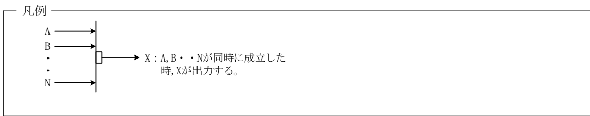
図-1-2-16 UF 6 処理設備（2号廃品回収槽）インターロック （廃品回収槽回収停止による待機槽回収開始インターロック）
