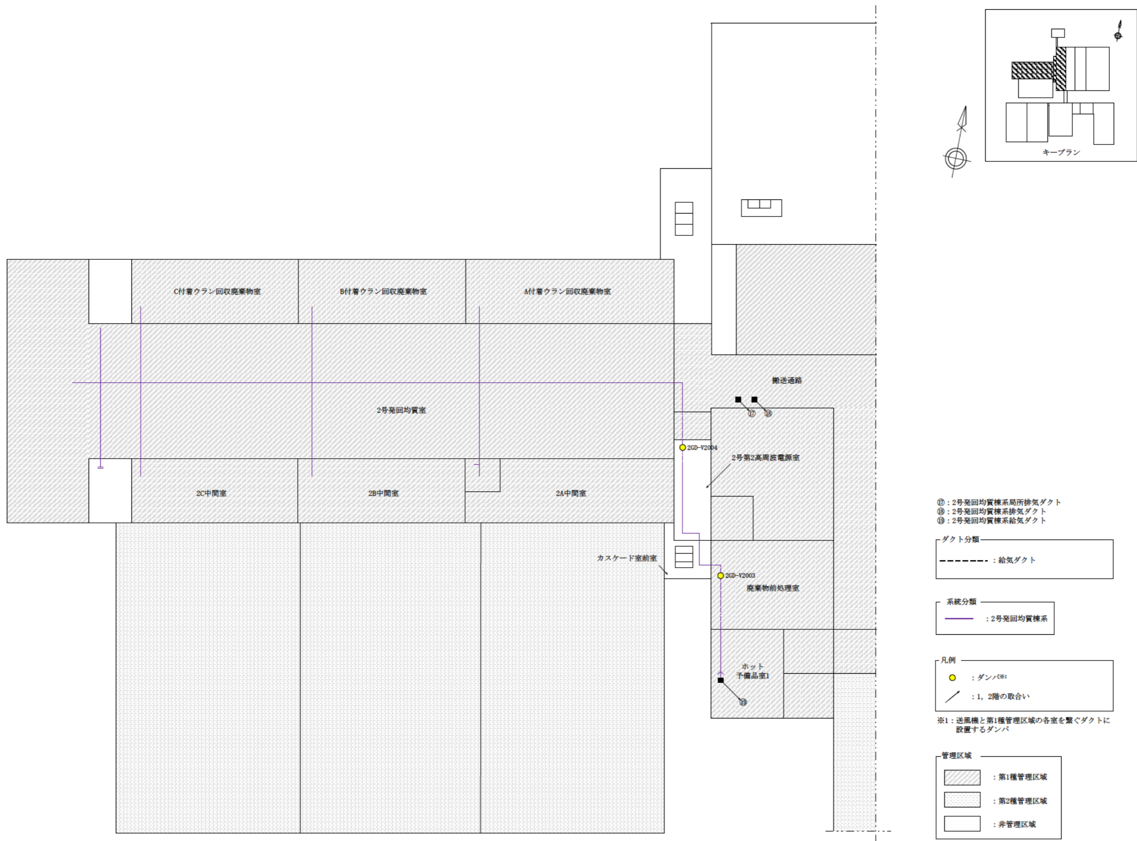
図 1.3.6 気体廃棄物の廃棄設備 系統詳細図 (給気ダクト (1階))
