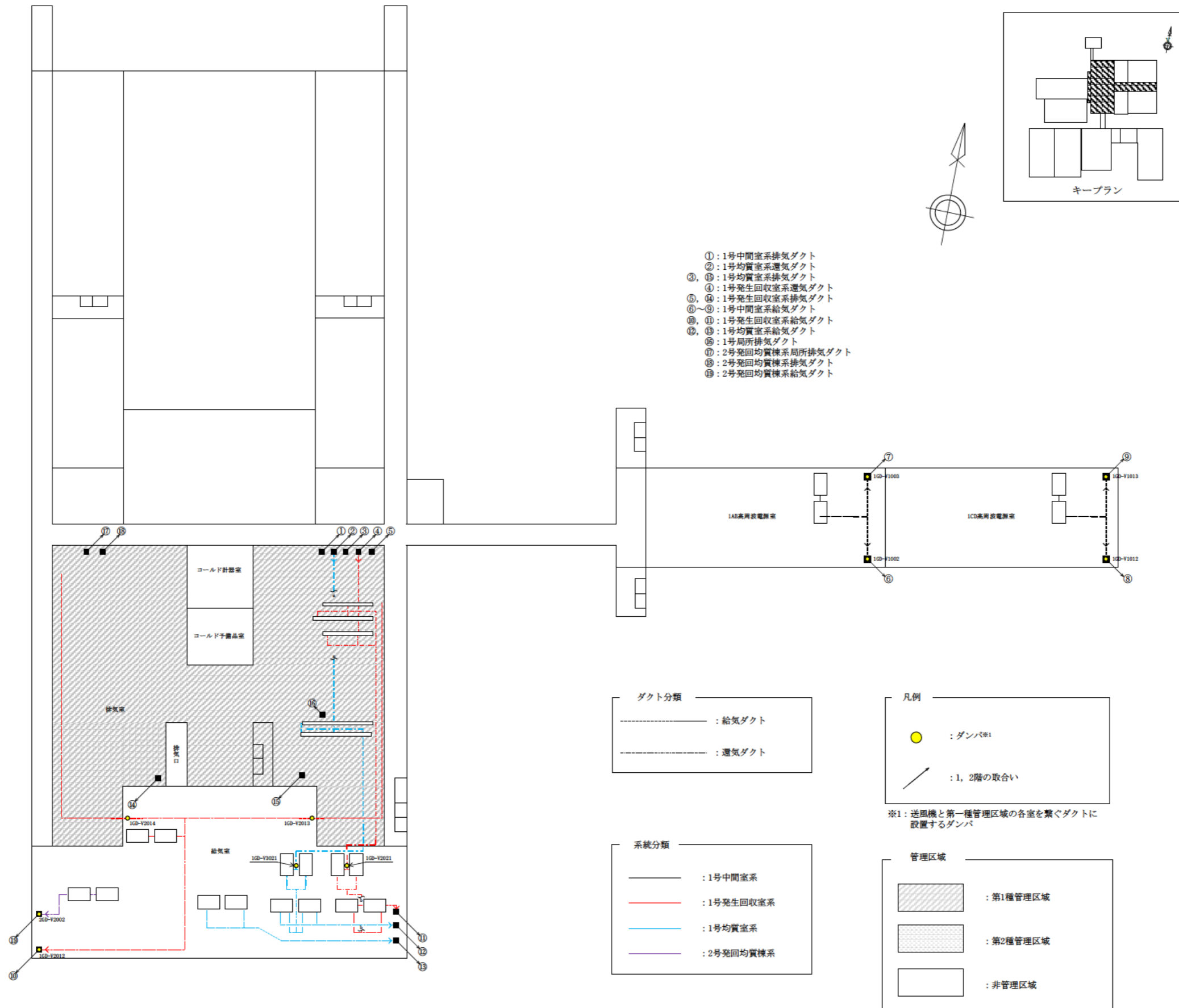
図 1.3.3 気体廃棄物の廃棄設備 系統詳細図 (給気, 還気ダクト (2階))
