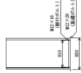
側面図
