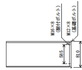
側面図
