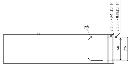
側面図
