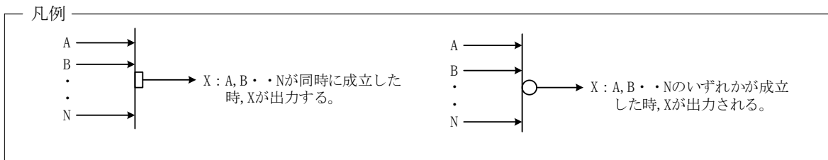
図-1-2-13 UF 6 処理設備 (2A 廃品コールドトラップ) インターロック (廃品ガス移送ヘッダ配管圧力異常上昇によるガス移送停止のインターロック)
