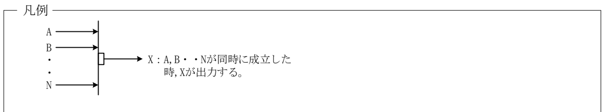
図-2-1-3(2/2) 1号発生回収室系排風機 インターロック (第1種管理区域の排気機能維持)
