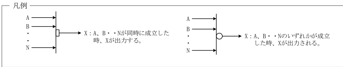
図-1-2-6 UF 6 処理設備（2号製品コールドトラップ） インターロック （圧力異常高又は温度異常高による加熱停止のインターロック）
