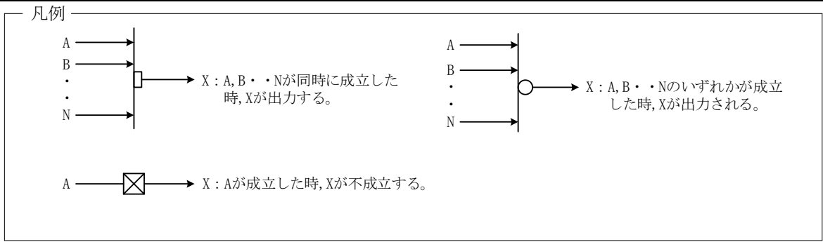
図-1-2-20 UF 6 処理設備 (2号一般ページ系コールドトラップ) インターロック (地震発生時の加熱停止のインターロック)
