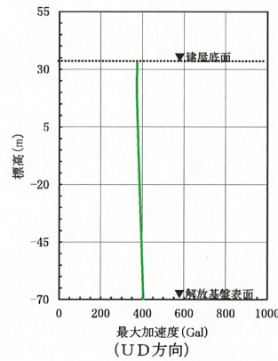
第 6 - 43 図(14) 建屋底面位置における地震動 (S s - B 3, 前処理建屋：中央地盤)
