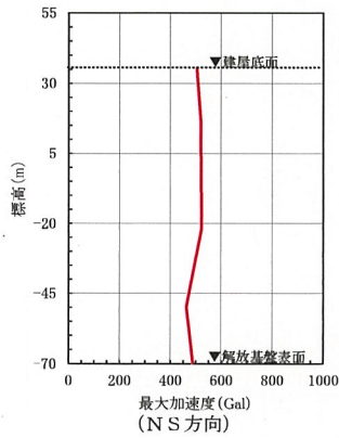
第 6 - 43 図(6) 建屋底面位置における地震動 (S s - B 5, 第 1 ガラス固化体貯蔵建屋：西側地盤)
