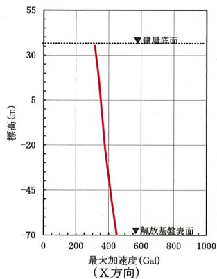
第 6-43 図(8) 建屋底面位置における地震動 (S s - C 2, 第 1 ガラス固化体貯蔵建屋：西側地盤)
