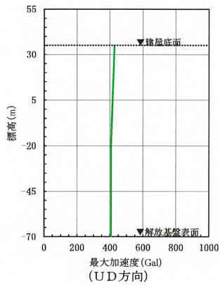
第6-43 図(24) 建屋底面位置における地震動 (S s - B 3, ウラン・プルトニウム混合酸化物貯蔵建屋：東側地盤)
