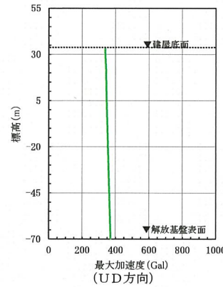
第6-43 図(16) 建屋底面位置における地震動 (S s - B 5, 前処理建屋: 中央地盤)
