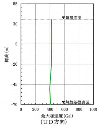
第6-43 図(4) 建屋底面位置における地震動 (S s - B 3, 第1 ガラス固化体貯蔵建屋: 西側地盤)
