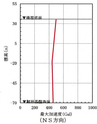
第6-43 図(23) 建屋底面位置における地震動 (S s - B 2, ウラン・プルトニウム混合酸化物貯蔵建屋: 東側地盤)
