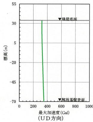
第 6 - 43 図(13) 建屋底面位置における地震動 (S s - B 2, 前処理建屋: 中央地盤)
