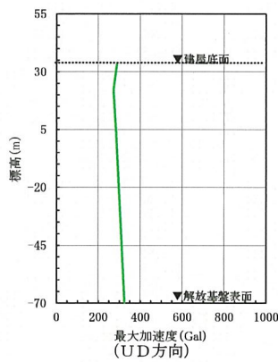
第6-43 図(15) 建屋底面位置における地震動 (S s - B 4, 前処理建屋: 中央地盤)
