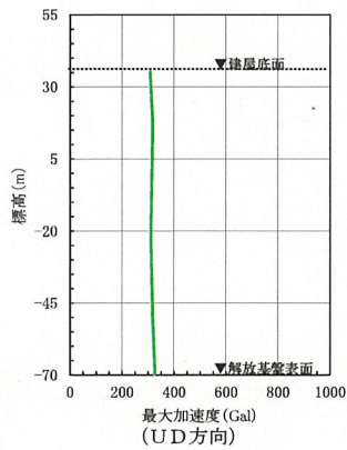
第 6-43 図(5) 建屋底面位置における地震動 (S s -B4, 第 1 ガラス固化体貯蔵建屋: 西側地盤)
