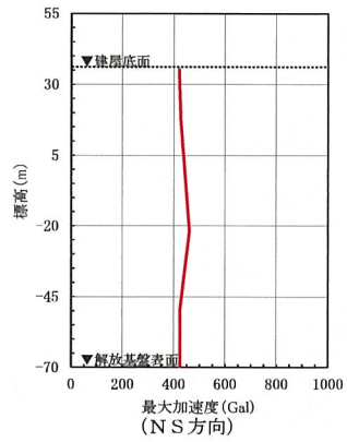
第6-43図(2) 建屋底面位置における地震動 (S s - B 1, 第1ガラス固化体貯蔵建屋: 西側地盤)
