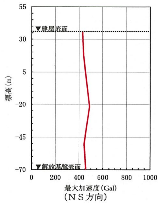
第 6 - 43 図(3) 建屋底面位置における地震動 (S s - B 2, 第 1 ガラス固化体貯蔵建屋: 西側地盤)
