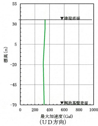
第6-43 図(25) 建屋底面位置における地震動 (S s - B 4, ウラン・プルトニウム混合酸化物貯蔵建屋: 東側地盤)
