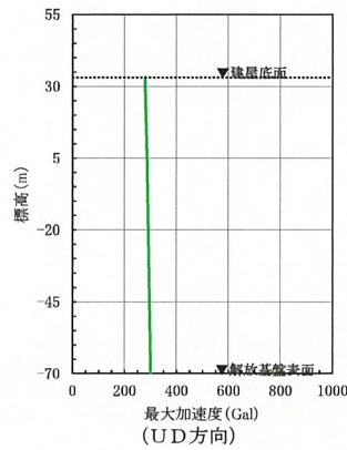
第 6 - 43 図(19) 建屋底面位置における地震動 (S s - C 3, 前処理建屋：中央地盤)
