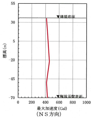
第 6 - 43 図(9) 建屋底面位置における地震動 (S s - C 3, 第 1 ガラス固化体貯蔵建屋 : 西側地盤)
