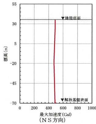
第 6 - 43 図(26) 建屋底面位置における地震動 (S s - B 5, ウラン・プルトニウム混合酸化物貯蔵建屋: 東側地盤)
