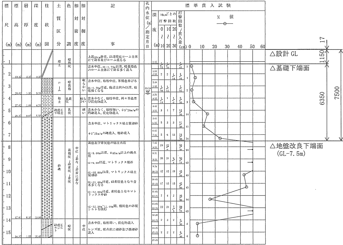
ボーリング柱状図 No. 2 による平均 N 値
