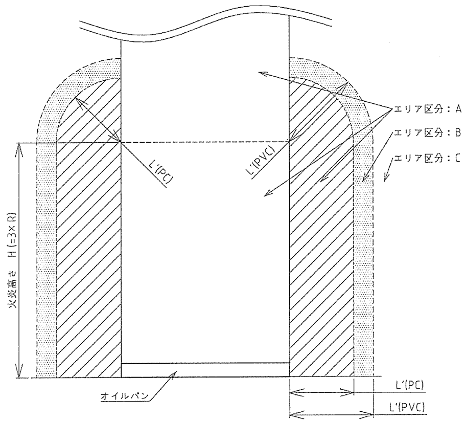
側面図
