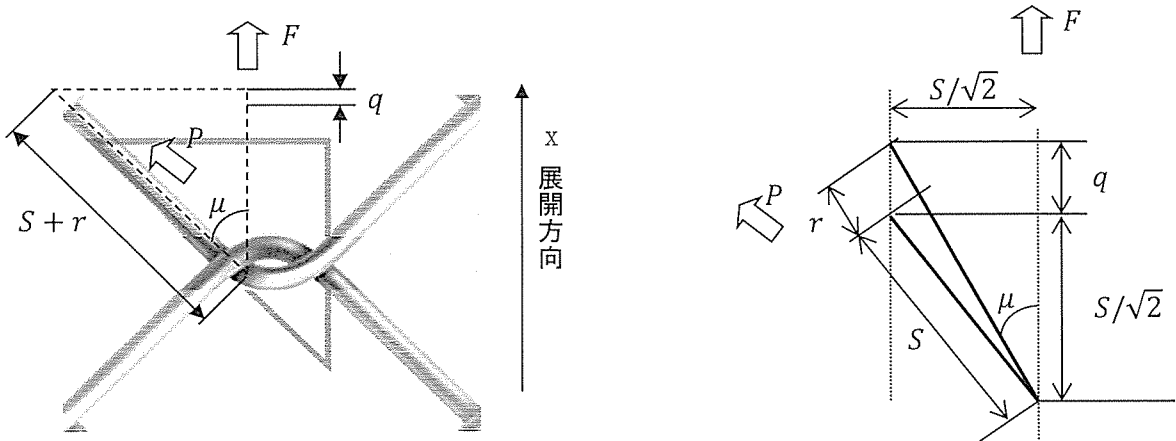
添説建 7.4.1-4 図 1 交点の変形模式図
