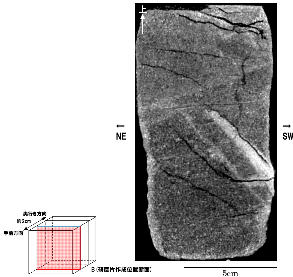
X線CT画像(傾斜方向断面, 解釈線なし) (断面(B):研磨片作成位置断面, P162~P163断面再掲)
