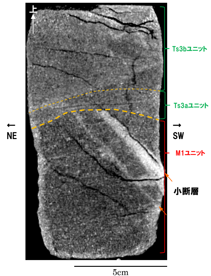
X線CT画像(傾斜方向断面, 解釈線あり) (断面(B):研磨片作成位置断面, P162~P163断面再掲)
