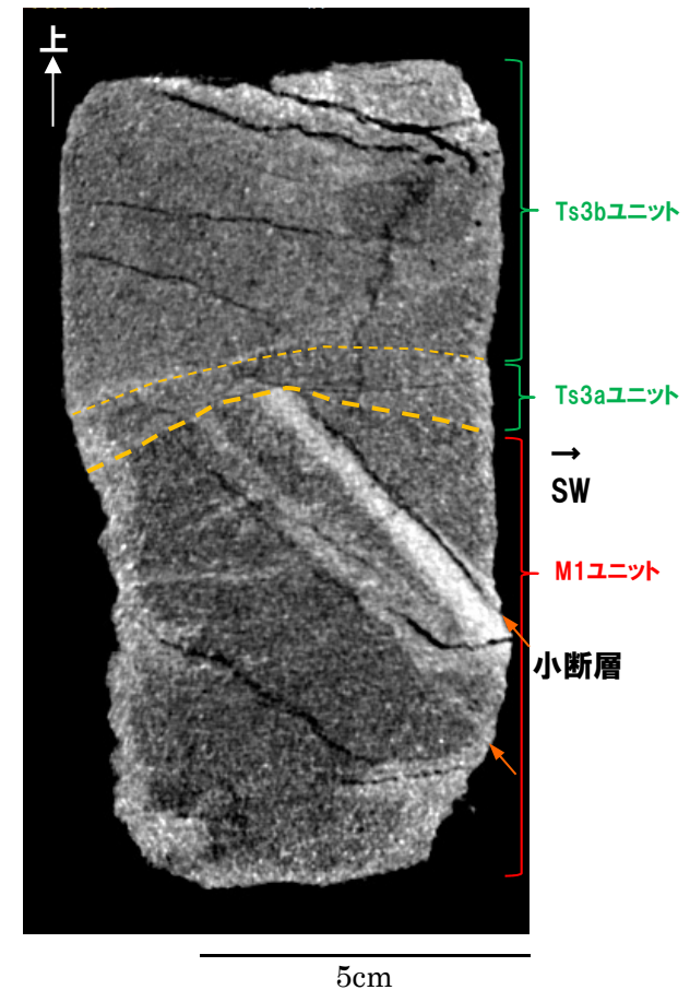
X線CT画像(傾斜方向断面, 解釈線あり) (断面(A): 研磨片作成位置断面から手前方向に約5mmの位置)
