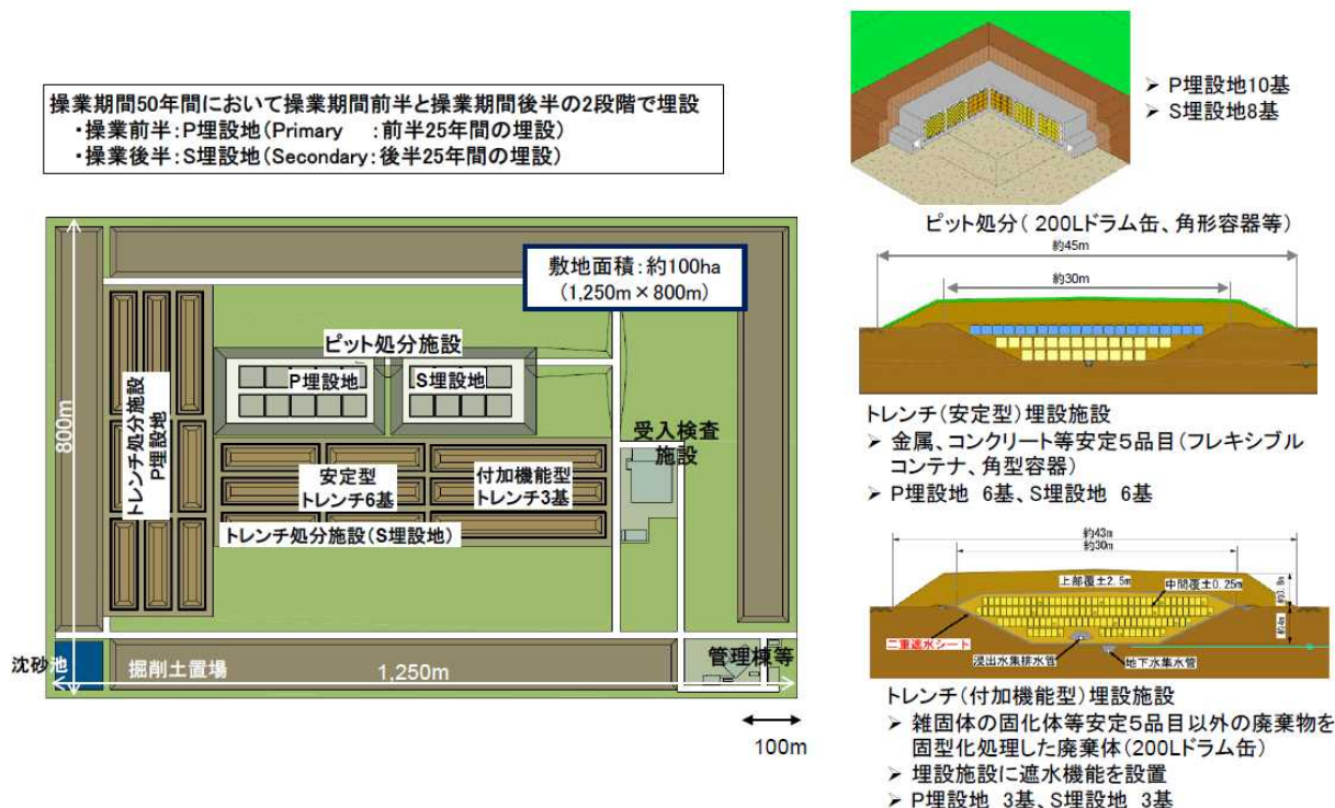
図 4 埋設施設の概要 ([8]より抜粋)
