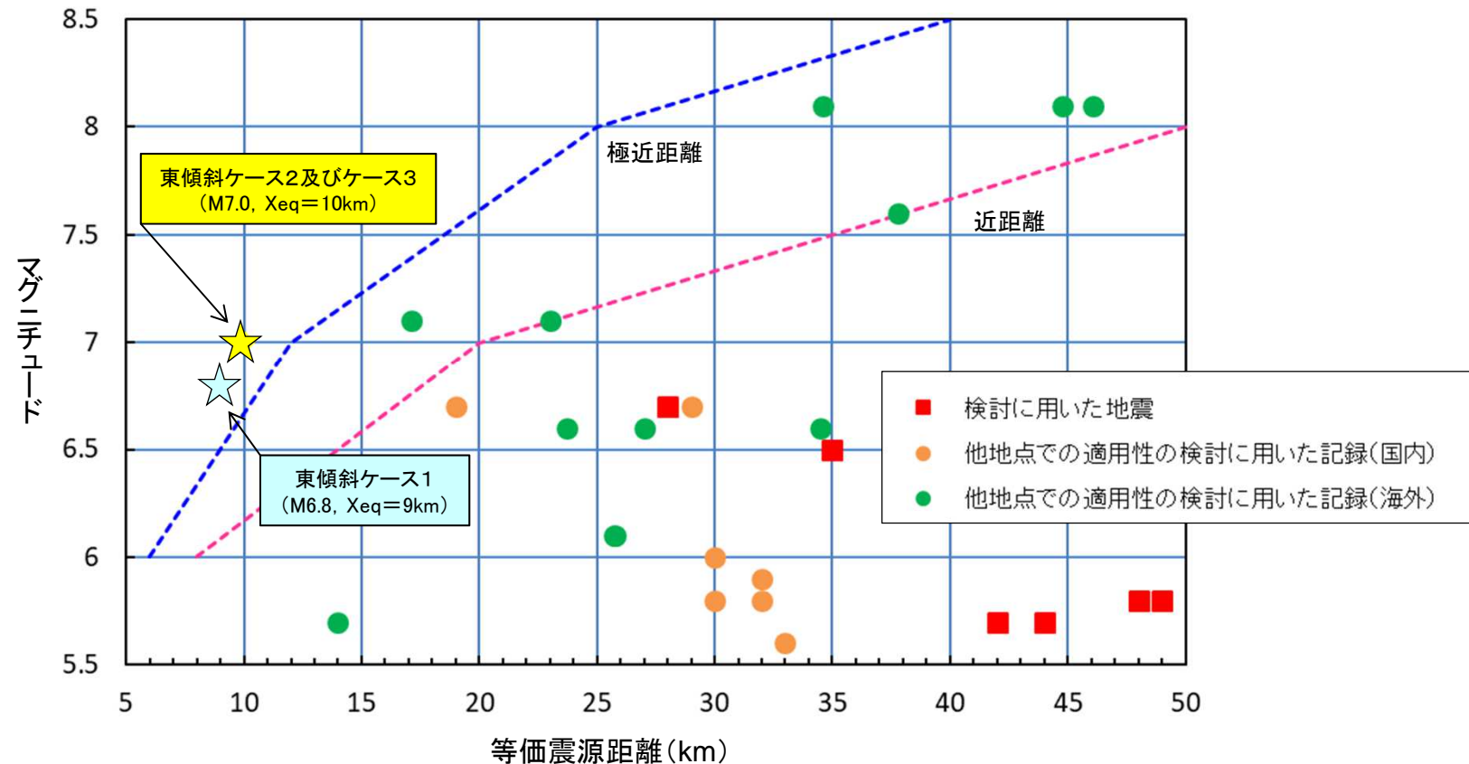
Noda et al.(2002)のデータ範囲と横浜断層(東傾斜)による地震との関係
