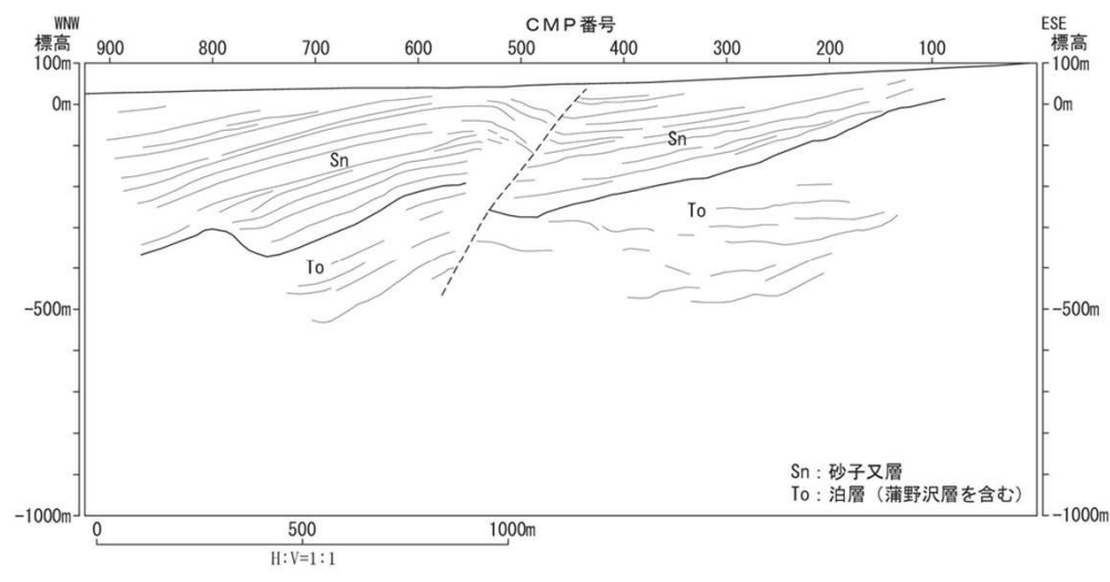
鶏沢測線の深度断面とその解釈
