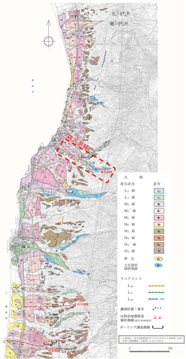
横浜断層周辺の空中写真判読図
