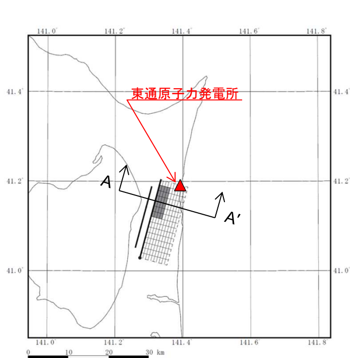
断層配置図
