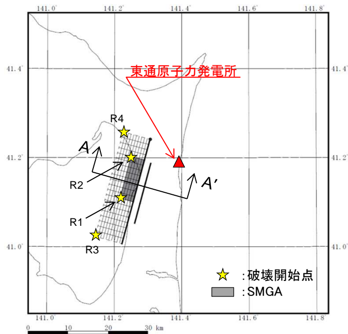
断層配置図
