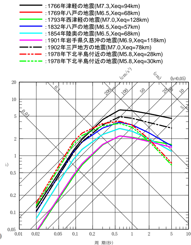
主な被害地震の応答スペクトル [Noda et al.(2002)による]
