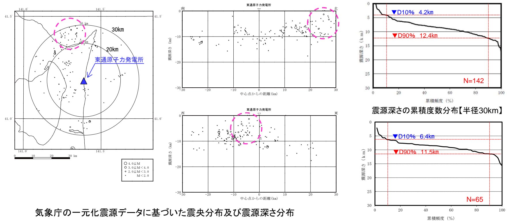
震源深さの累積度数分布【半径20km】
