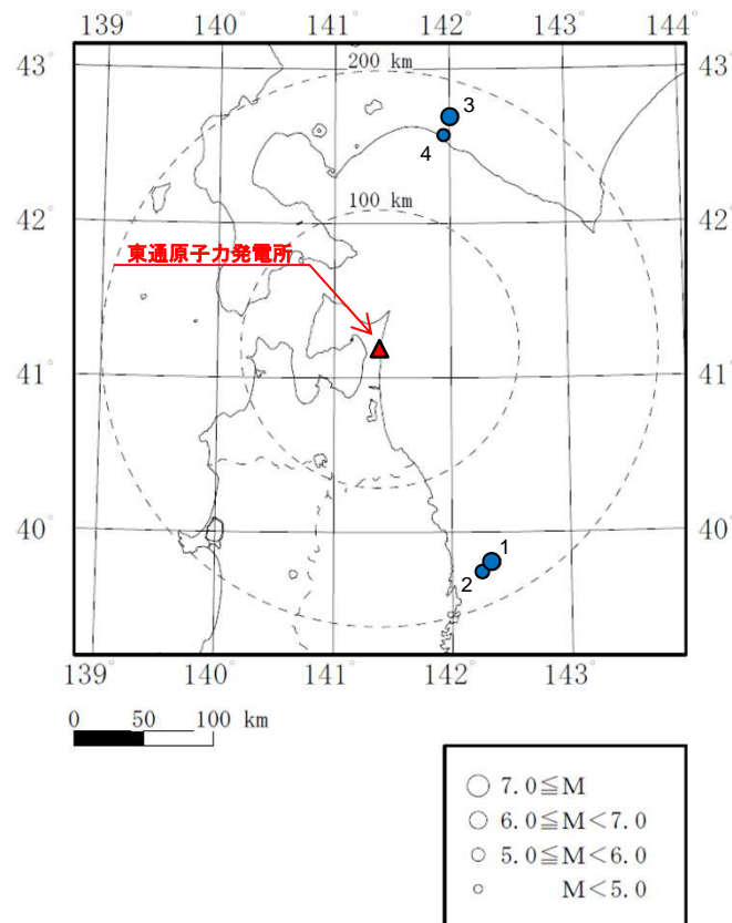
検討に用いた内陸地殻内地震の震央分布
