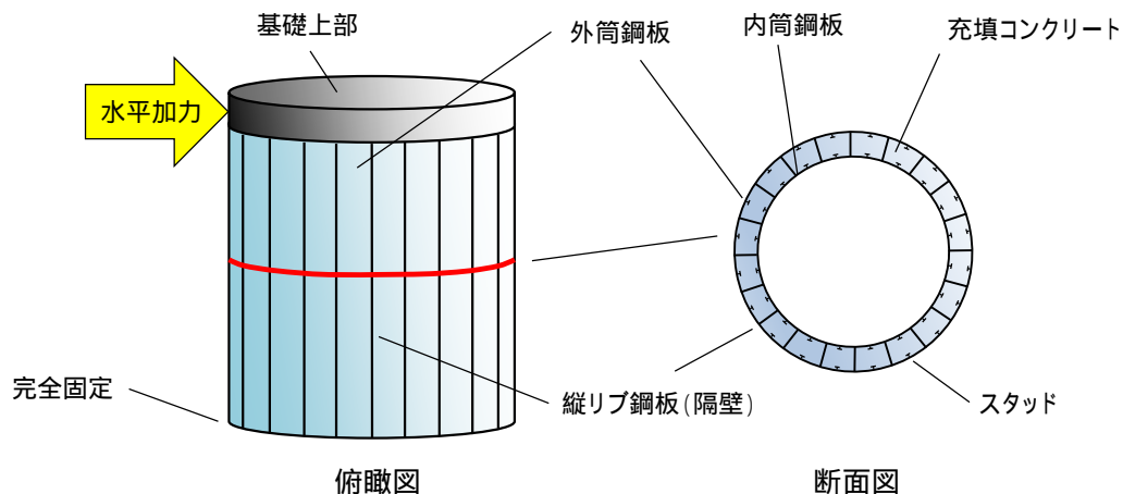
図1 鋼コンクリート合成構造製の基礎構造物のイメージ
