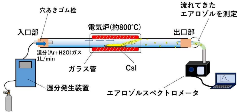
図1 蒸気凝縮法によるエアロゾル生成試験装置の構成例
