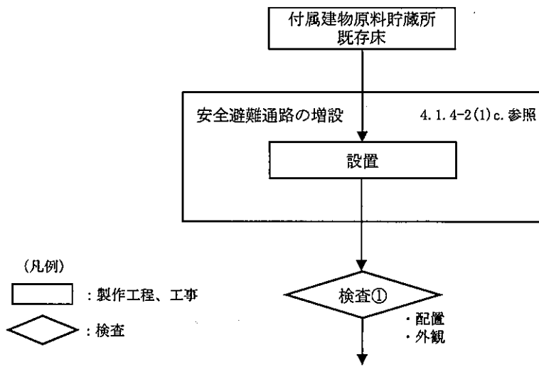
(図へ1-1 工事の手順フロー図へ)
