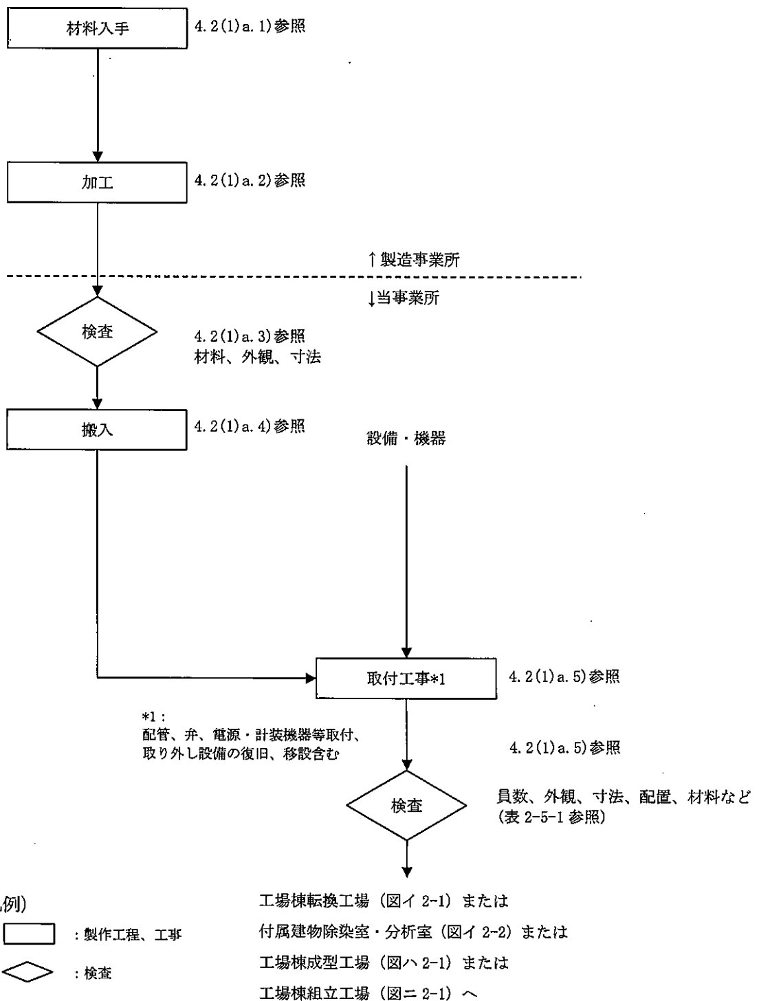
図へ 2-3-1 工事の手順フロー図 (改造する設備・機器)
