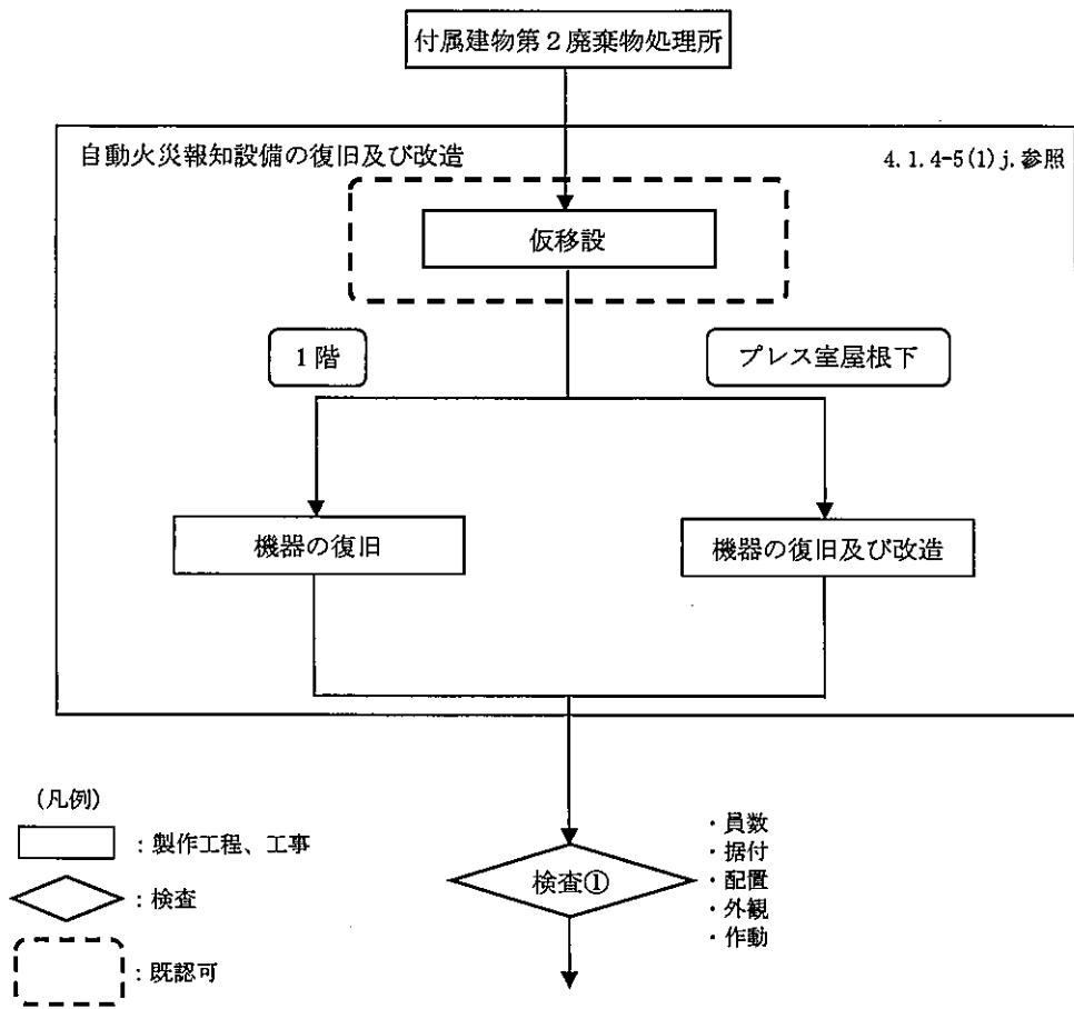
(図ト 1-2 工事の手順フロー図へ)
