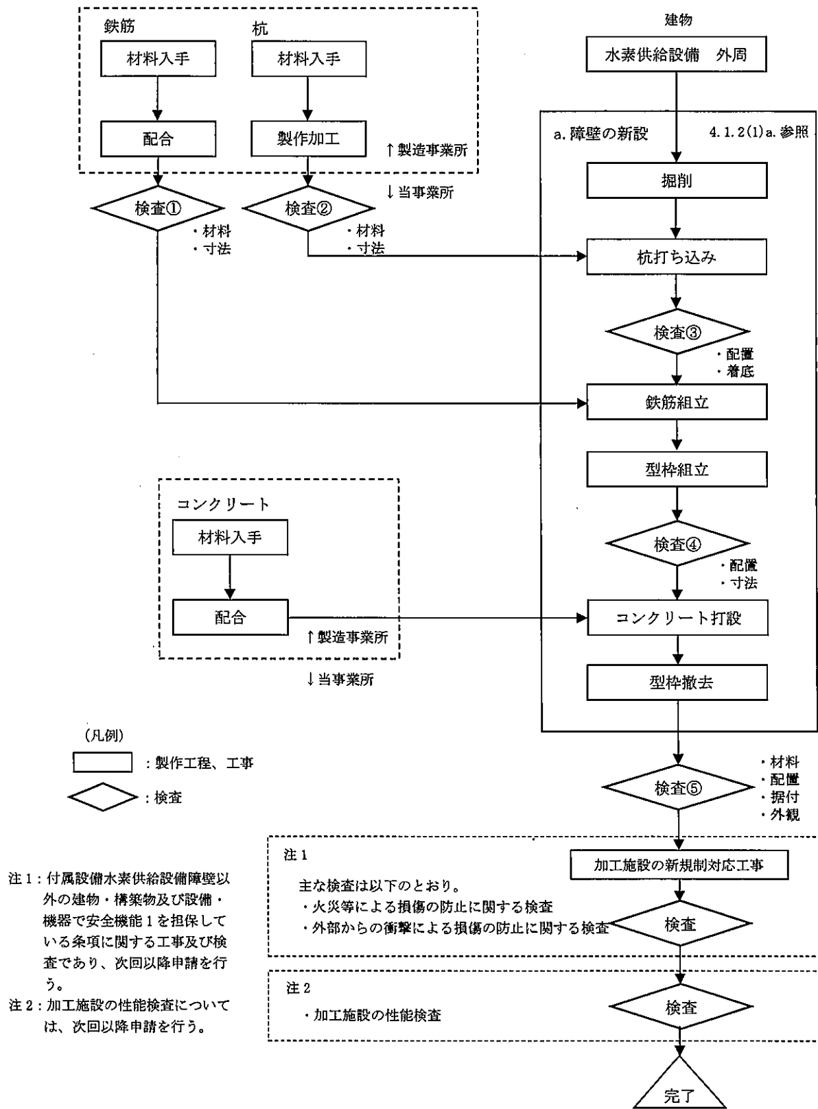
図リ 2-1 障壁の新設の手順フロー図
