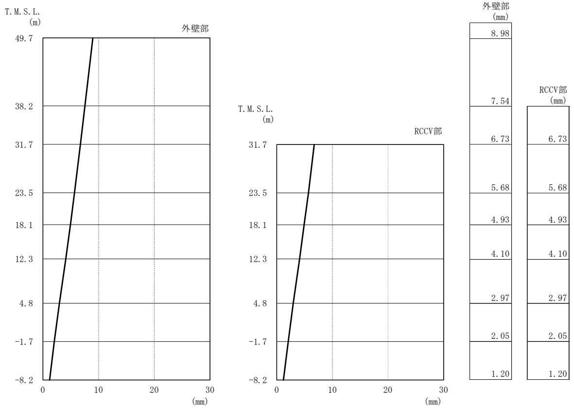
図4-7 最大応答変位 (EW方向)
