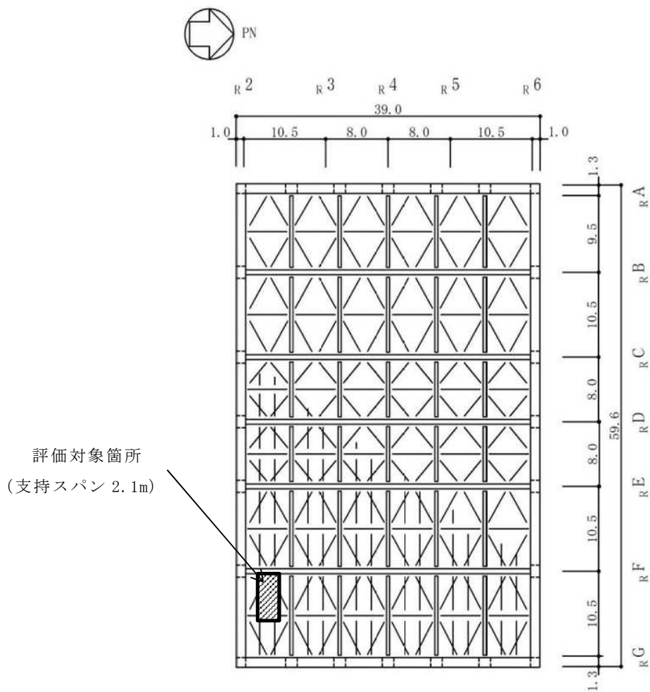
図 4-1 評価対象箇所（屋根スラブ，T. M. S. L. 49.7m）
