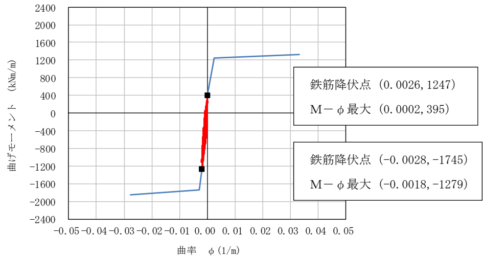
図 4-85 B-B断面のM- \phi 曲線を用いた貯水機能の確認
