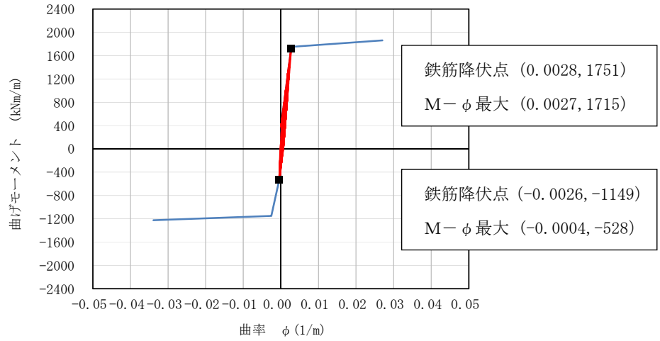
図 3-85 B-B断面のM- \phi 曲線を用いた貯水機能の確認 (左側壁下部, 解析ケース④, 地震動 Ss-1-1) *
