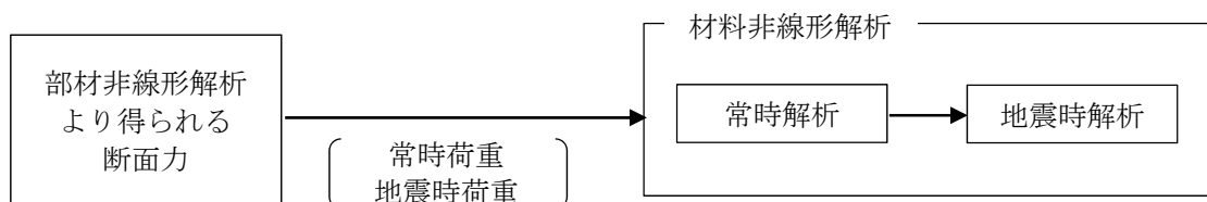
図 4-105 荷重の作用手順
