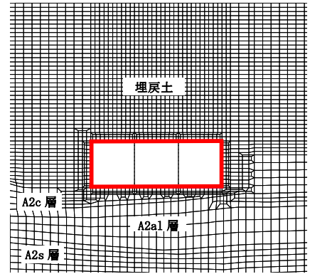
(B-B断面)
