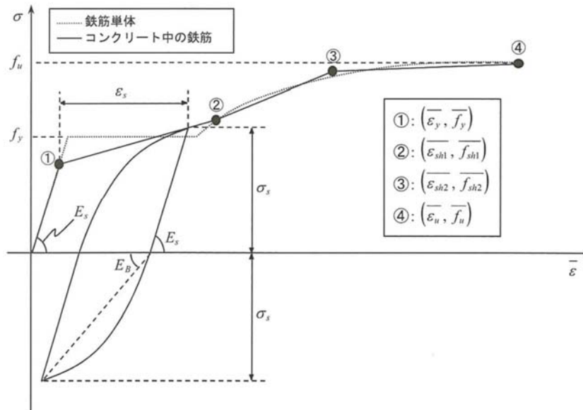
図 4-102 ひずみ硬化域までモデル化した鉄筋の平均応力ー平均ひずみ関係
