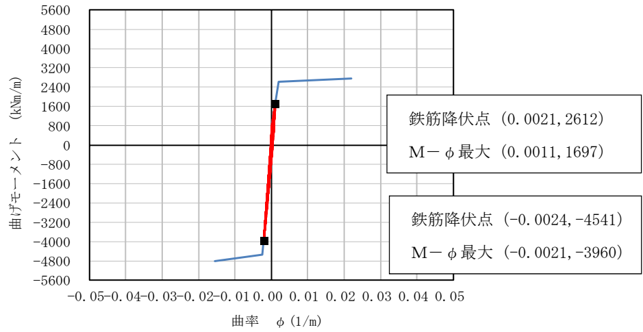
図 3-87 C-C断面のM-φ曲線を用いた貯水機能の確認
