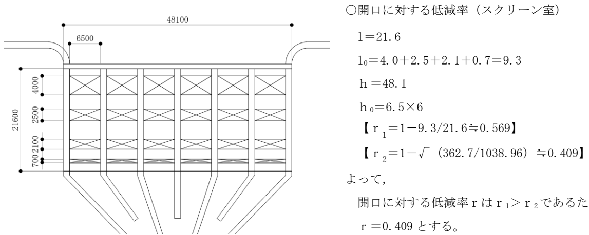
図 1-16 部材奥行幅の低減率の算定結果
