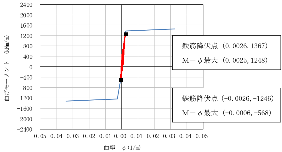
図 3-86 B-B断面のM- \phi 曲線を用いた貯水機能の確認 (頂版, 解析ケース④, 地震動 Ss-1-1) *
