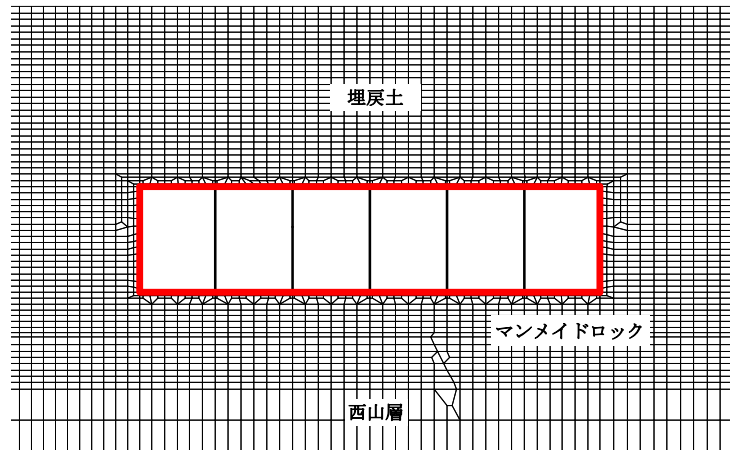
(C-C断面)
