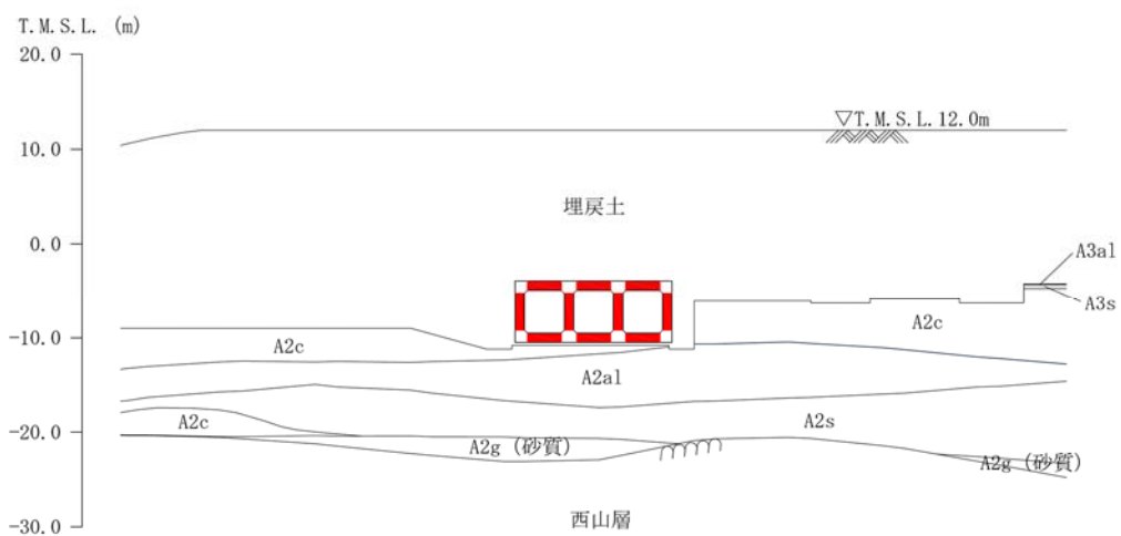
図 3-13 通水機能を要求する範囲 (A-A断面)
