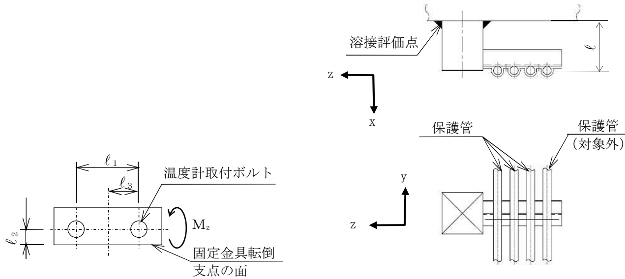
固定金具と取付ボルト部詳細
