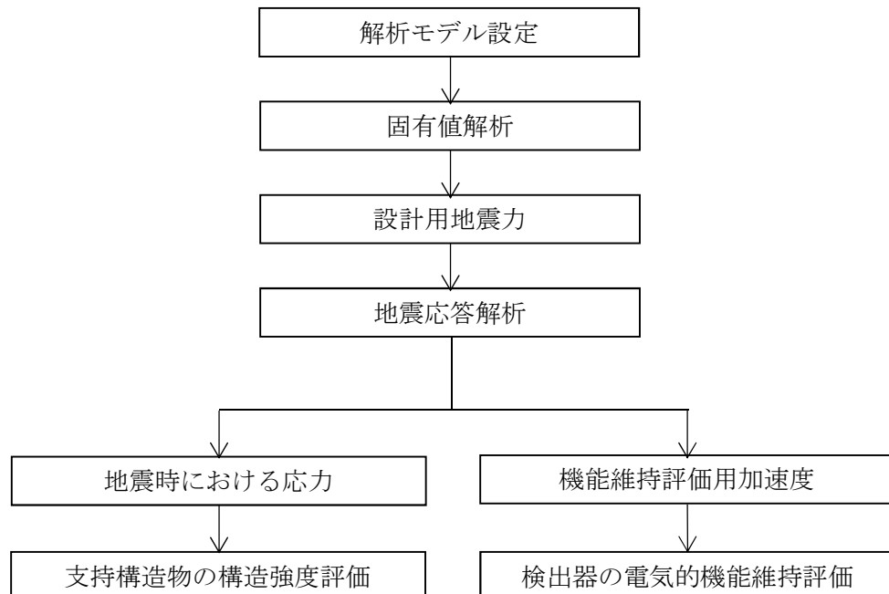
図2-1 サブプレッションチェンバプール水温度の耐震評価フロー
