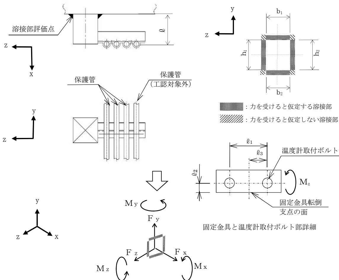
図5-1 計算モデル（溶接部，温度計取付ボルト）
