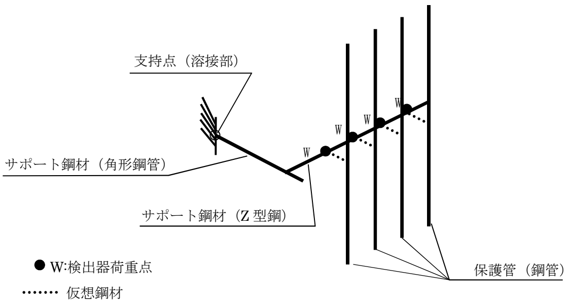
図4-1 解析モデル
