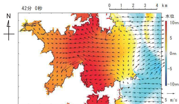
押し波時の流況（地震発生 42 分後）
