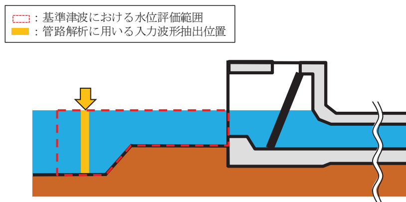
図 1.4-26 取水口前面における水位抽出位置（概念図）
