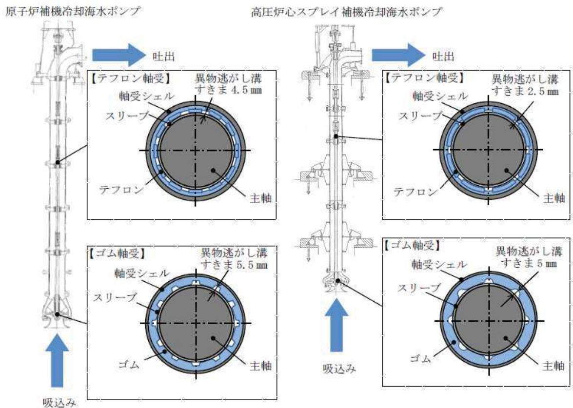
図 3.1.1-6 非常用海水ポンプ軸受配置図
