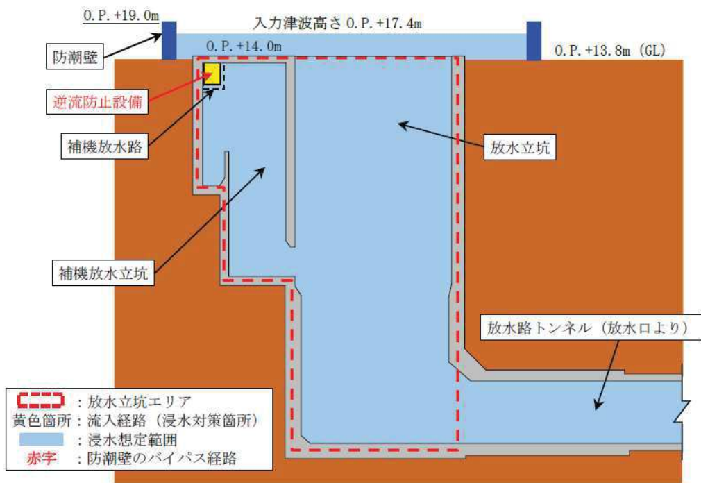
図 3-14 第 2 号機 放水立坑 浸水対策配置図 (A-A 断面図)
