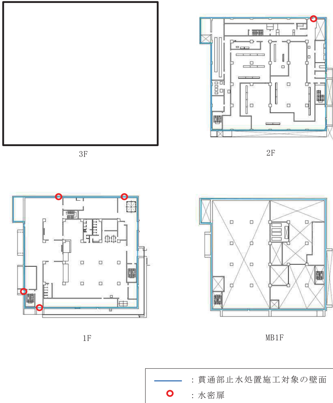
図 3-35 貫通部止水処置及び水密扉の位置図 (4/5) (制御建屋)
