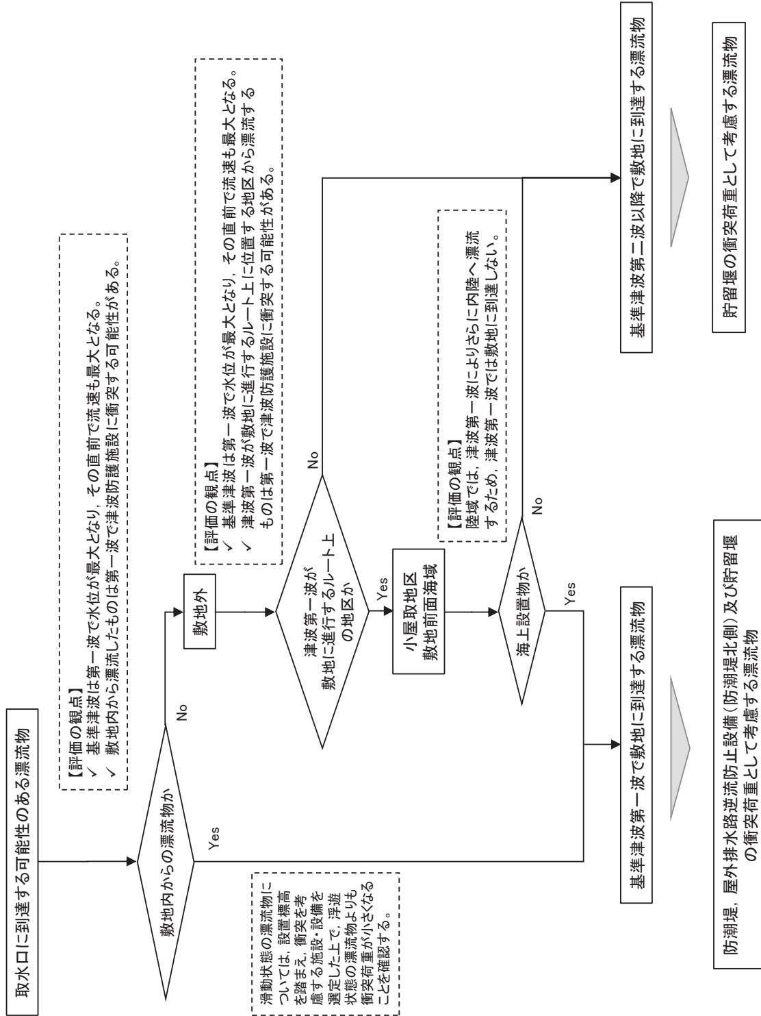
図 3-37 津波防護施設の機能に対する影響評価フロー
