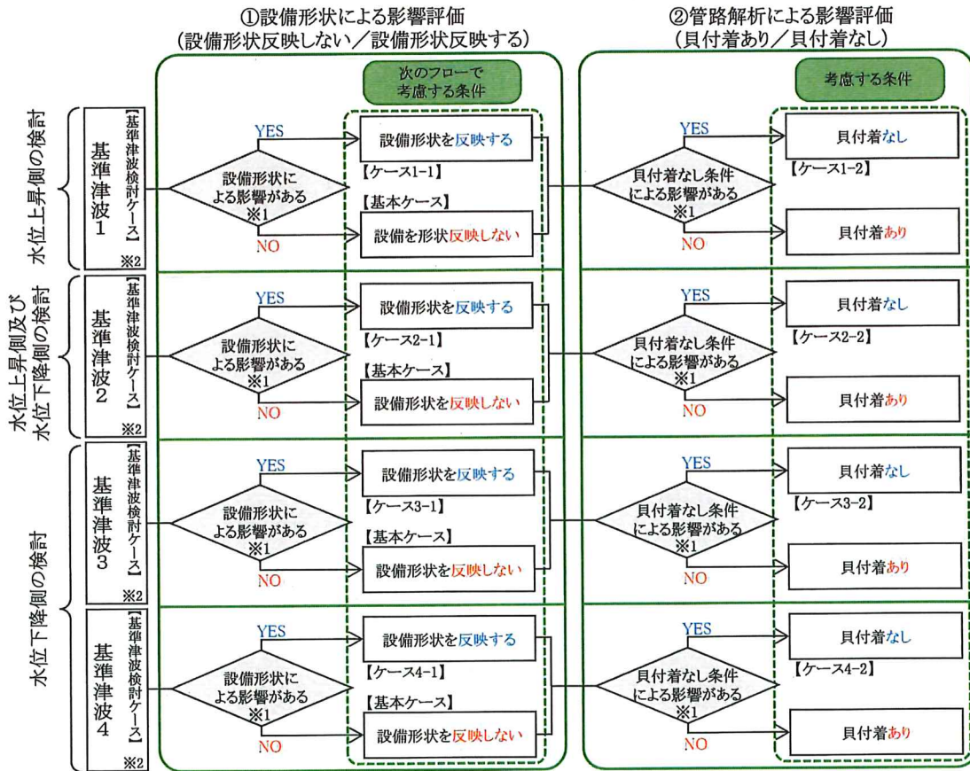
第4-3図 影響評価検討フロー
