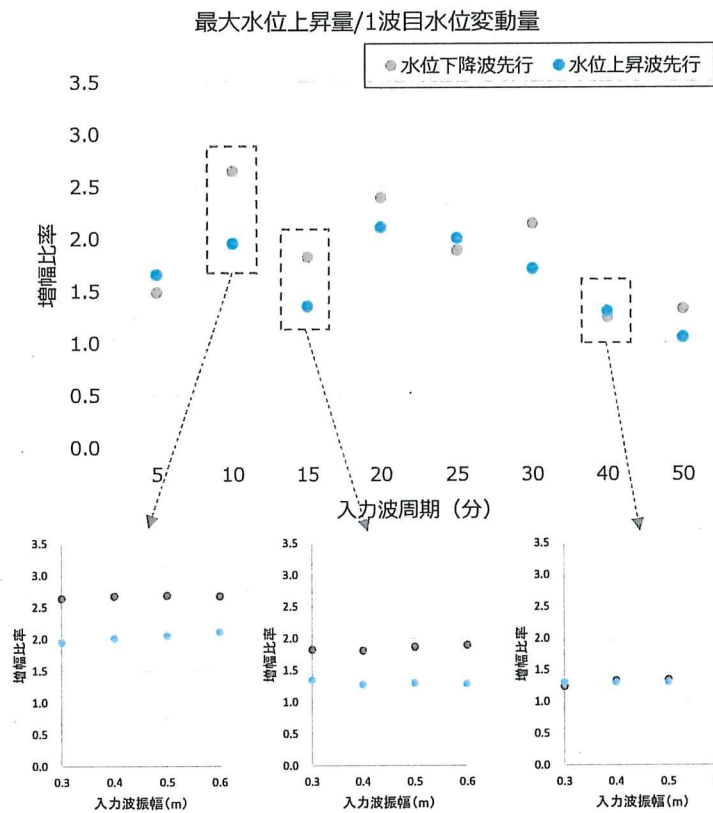
第3-19図 正弦波によるパラメータスタディ結果 (取水口前面)
