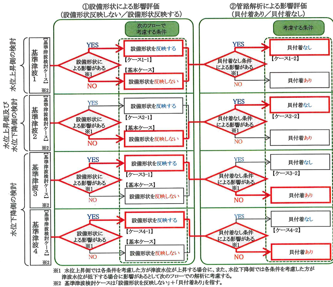
第4-6図 管路解析による影響評価結果
