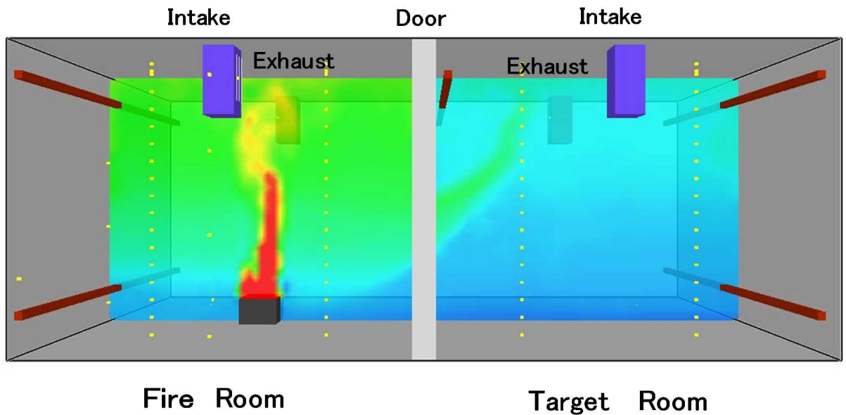
図 4.1-4 本試験（その1）の解析結果の温度分布出力例
