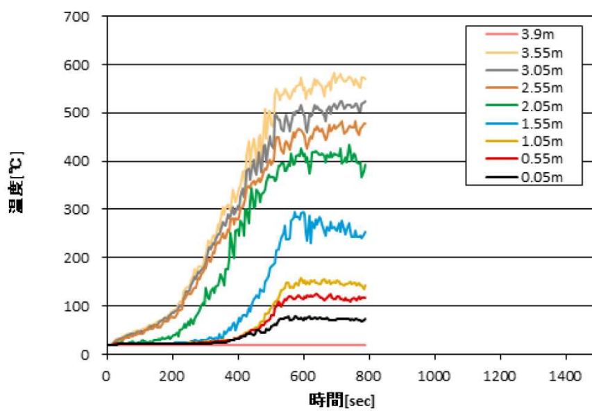
図 4.1-6 本試験（その1）の解析結果の過渡変化例
