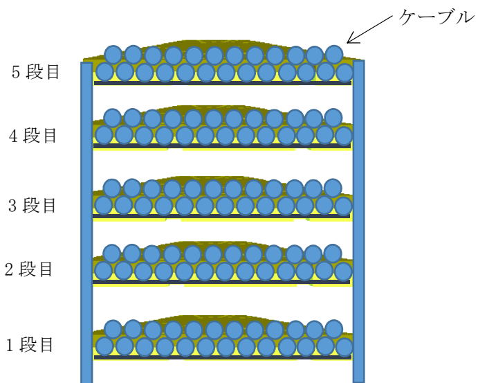
ケーブル部詳細配置
