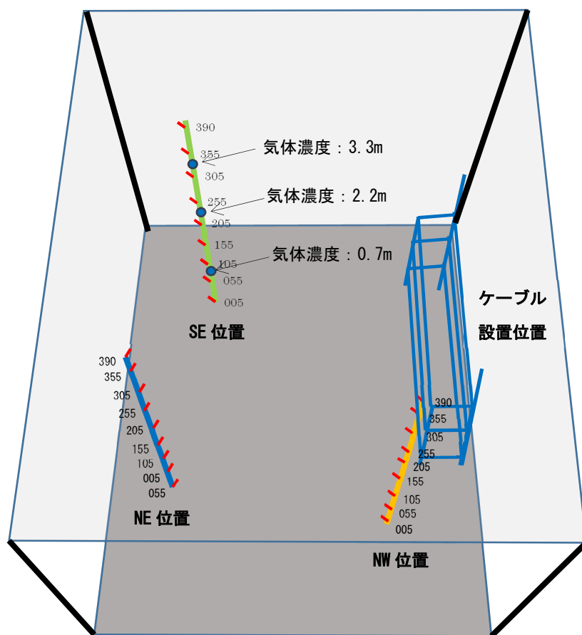
図 4.1-5 本試験（その1）の解析結果の過渡変化出力位置
