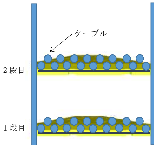
ケーブル部詳細配置
