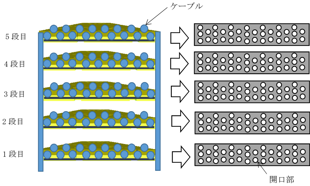
図 4.2-2 サポート試験（その2）のケーブルトレイ部及びケーブル部のモデル化例
