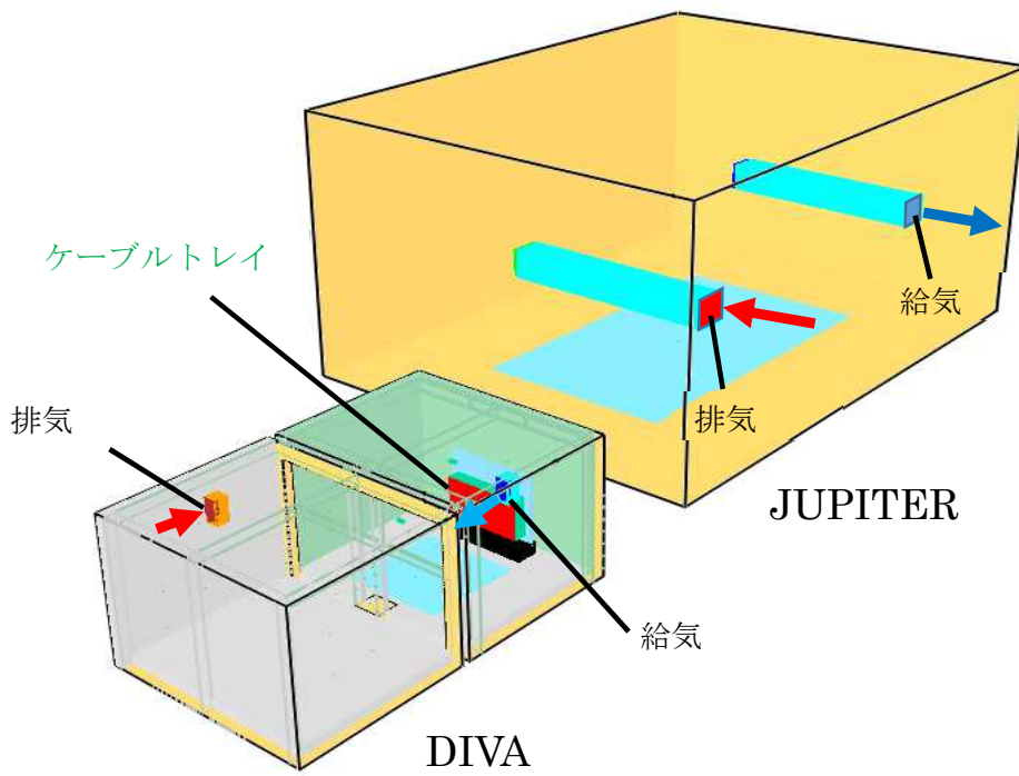
試験体の全体構成図
