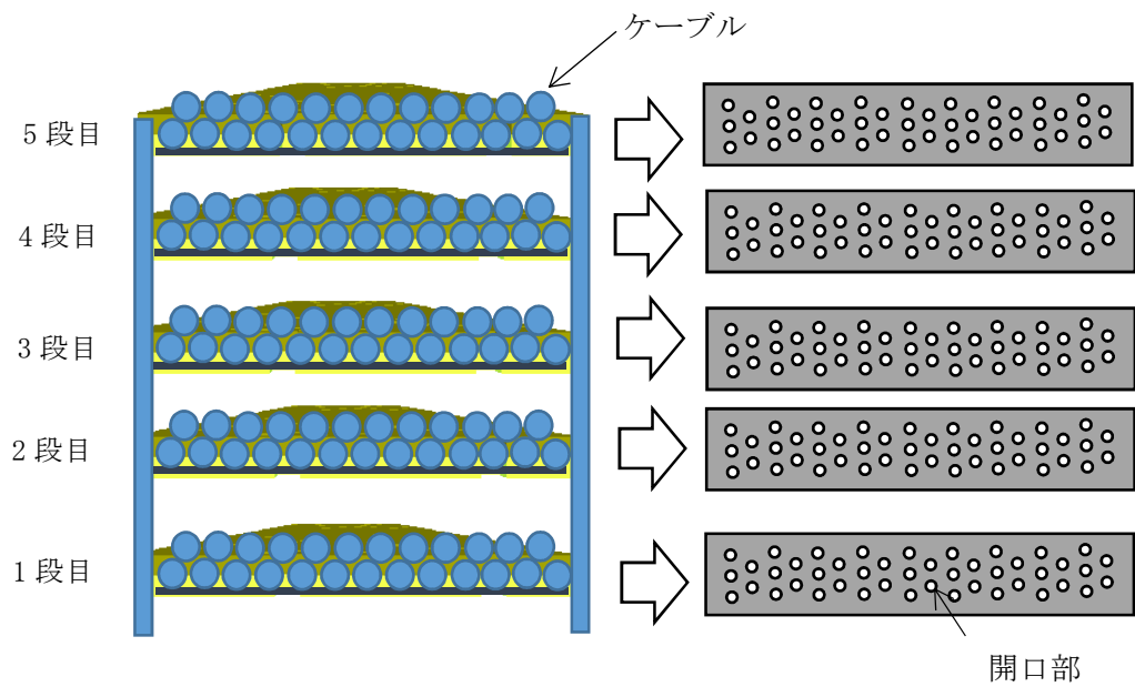
図 4.1-2 サポート試験（その1）のケーブルトレイ部及びケーブル部のモデル化例
