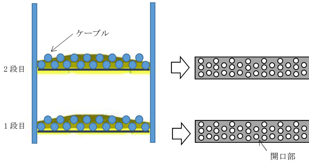
図 4.3-2 サポート試験（その3）のケーブルトレイ部及びケーブル部のモデル化例
