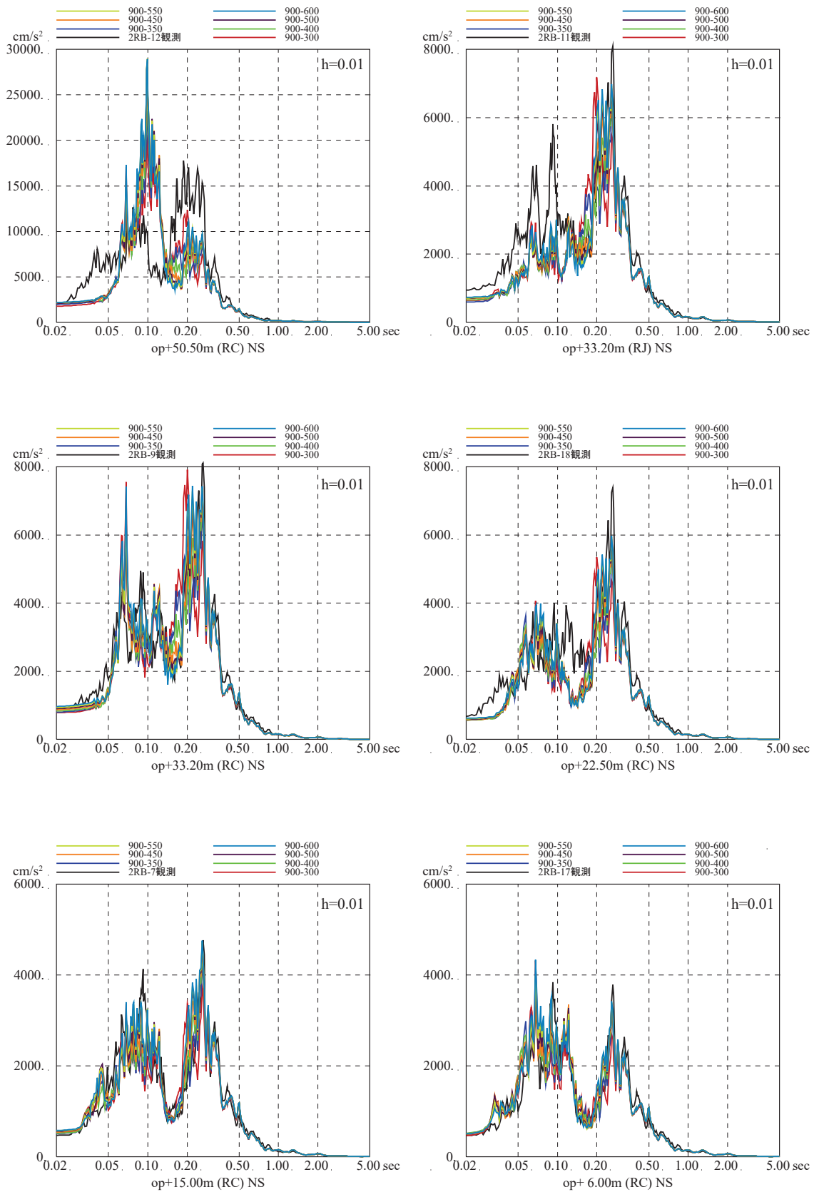
図 3-2 (7) 表層地盤上部の地盤物性の検討結果 (はざとり波入力のシミュレーション解析の床応答スペクトルの比較)
