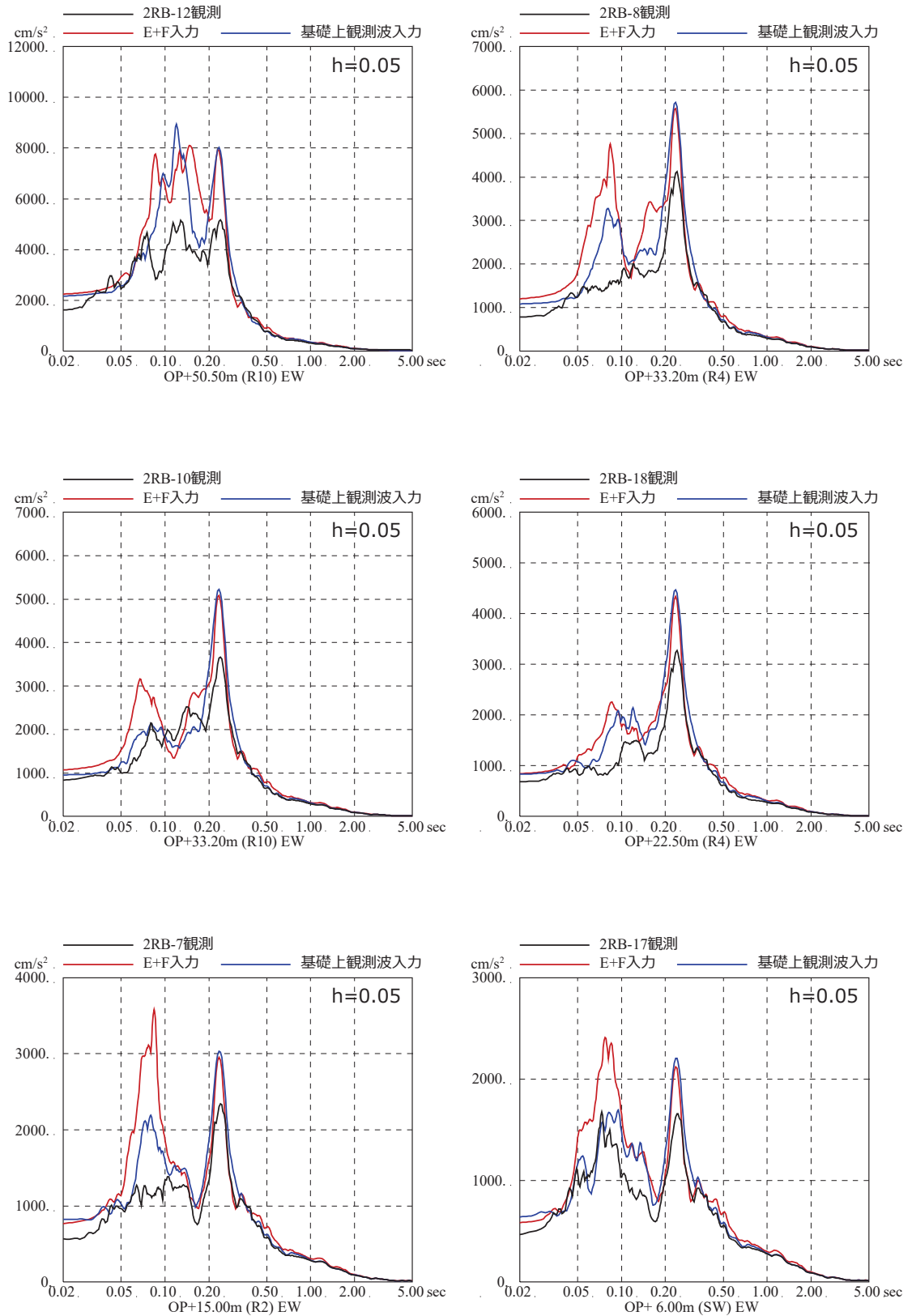
図4-31 3.11地震のはざとり波を入力に用いた場合と 基礎版上観測記録を用いた場合のシミュレーション解析結果の比較 (原子炉建屋, EW方向)
