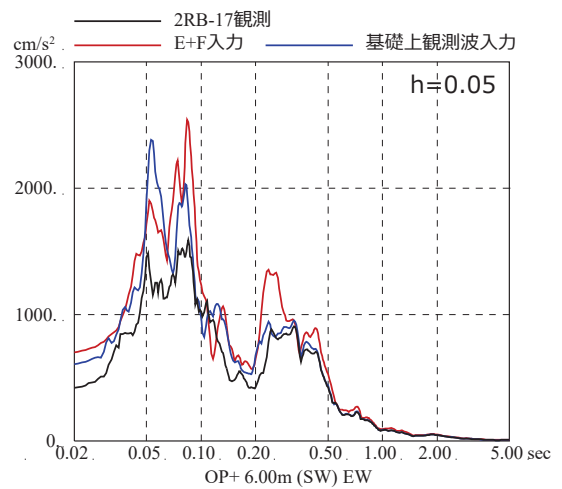
図 3-9 4.7 地震のはざとり波を入力に用いた場合と 基礎版上観測記録を用いたシミュレーション解析結果の比較 (原子炉建屋, EW 方向, 減衰 5%) ※地震計位置は, 付録 1 参照
