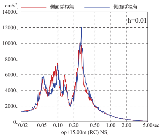
図 3-15 基準地震動 S s -D 2 を用いた側面地盤ばねの有無による地震応答解析結果の比較 (原子炉建屋, NS 方向, 減衰 1%)
