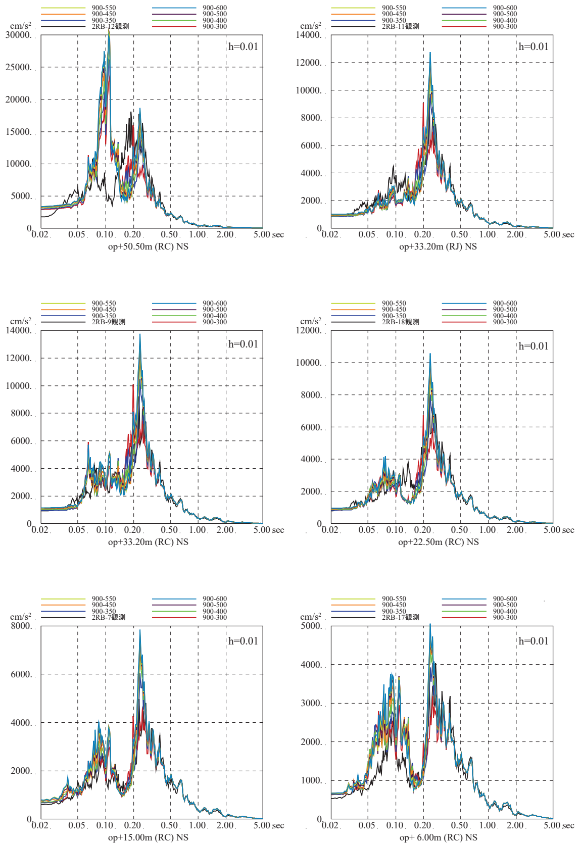
図 3-2 (3) 表層地盤上部の地盤物性の検討結果 (はざとり波入力のシミュレーション解析の床応答スペクトルの比較)
