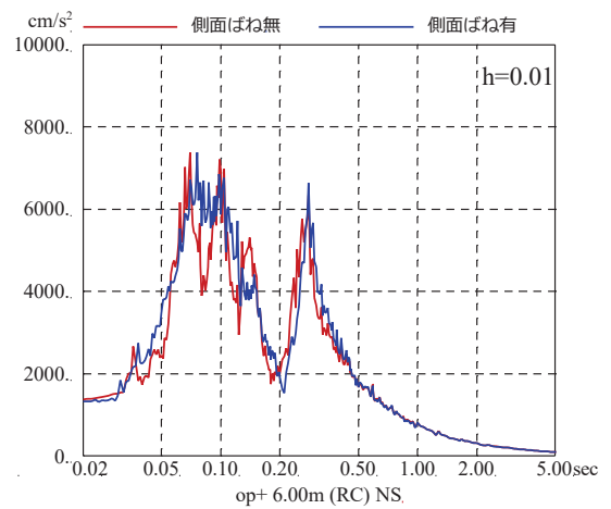
図 3-15 基準地震動 S s -D 2 を用いた側面地盤ばねの有無による地震応答解析結果の比較 (原子炉建屋, NS 方向, 減衰 1%)
