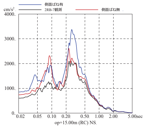
図 4-38 3.11 地震のはざとり波を用いた側面地盤ばねの有無による シミュレーション解析結果の比較 (原子炉建屋, NS 方向)
