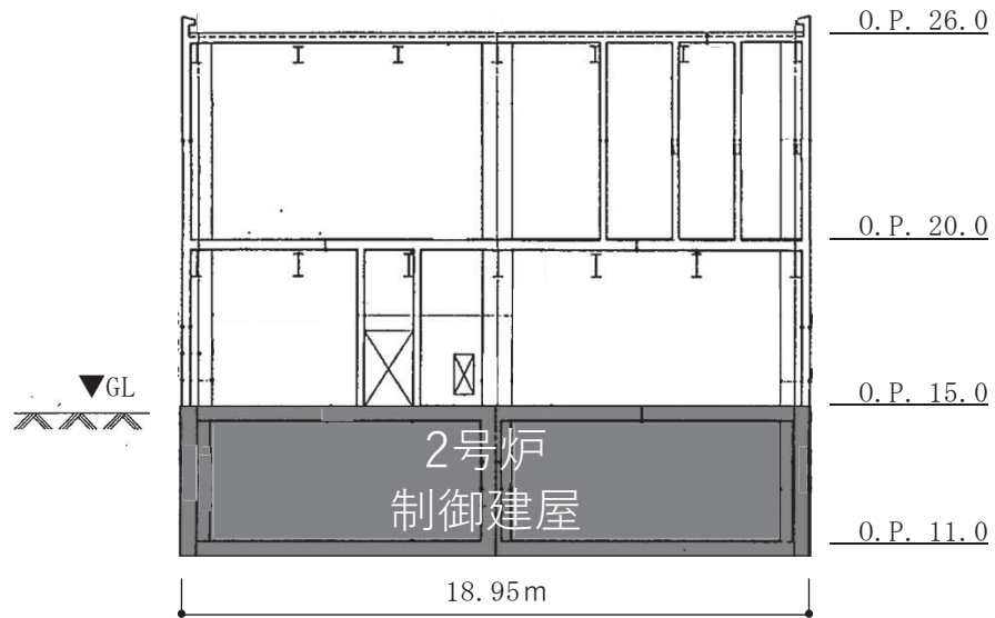
付録 2-13 図 補助ボイラー建屋（北面）の地盤の接地状況
