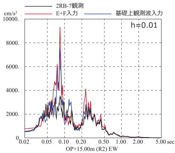
図 3-10 4.7 地震のはぎとり波を入力に用いた場合と 基礎版上観測記録を用いたシミュレーション解析結果の比較 (原子炉建屋, EW 方向, 減衰 1%) ※地震計位置は, 付録 1 参照
