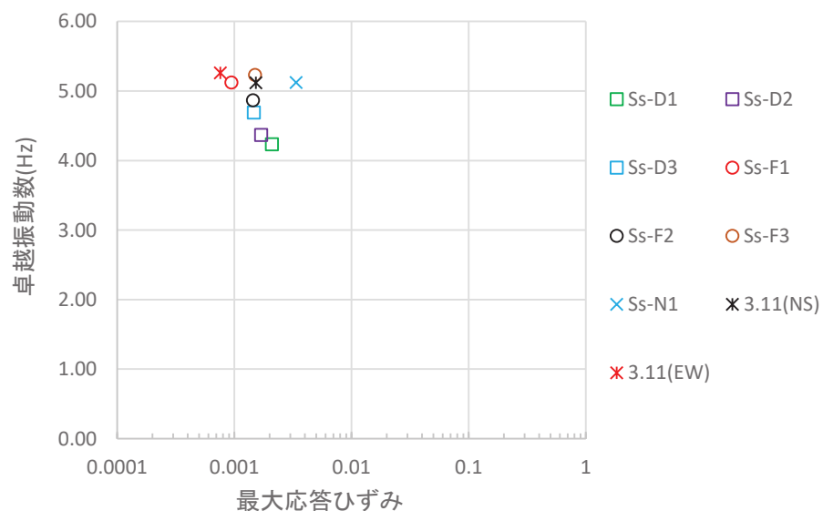
図 4-50 地盤の最大応答ひずみと表層地盤の卓越振動数の関係
