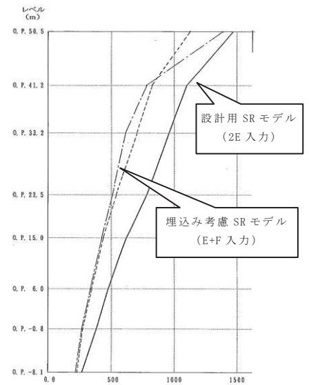
図4-7 解析結果の比較 (最大応答加速度)
