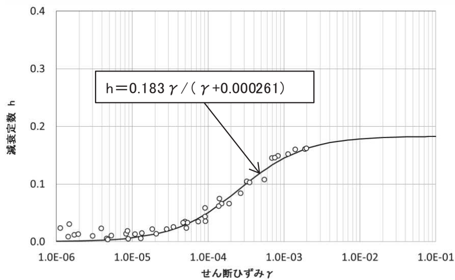
図-4 h - γ 曲線
