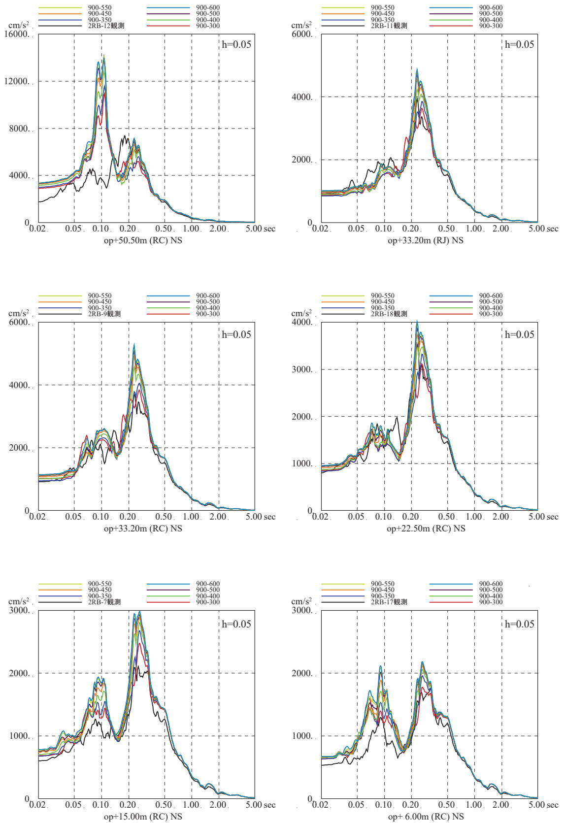
図 3-2 (1) 表層地盤上部の地盤物性の検討結果 (はぎとり波入力のシミュレーション解析の床応答スペクトルの比較)
