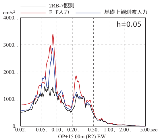
図 3-9 4.7 地震のはざとり波を入力に用いた場合と 基礎版上観測記録を用いたシミュレーション解析結果の比較 (原子炉建屋, EW 方向, 減衰 5%) ※地震計位置は, 付録 1 参照
