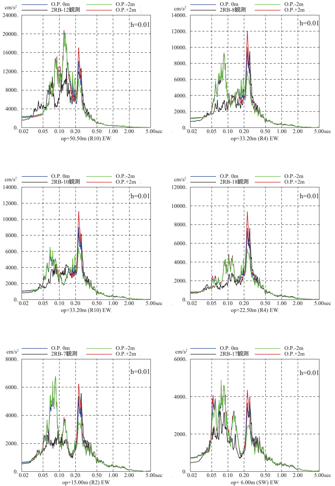
図 3-2 (4) 表層地盤の層境界に関する検討結果 (床応答スペクトルの比較) (3.11 地震, EW 方向, 減衰 1%)
