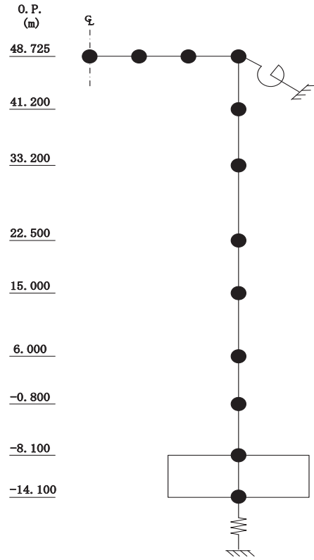
図 4-25 最大応答軸力 (弾性設計用地震動 S d, 鉛直方向)
