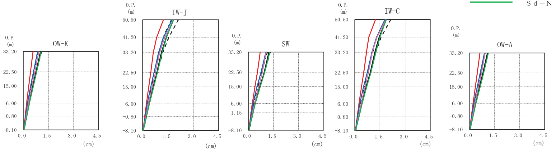
图 4-16 最大応答変位 (弾性設計用地震動 S d, NS 方向)
