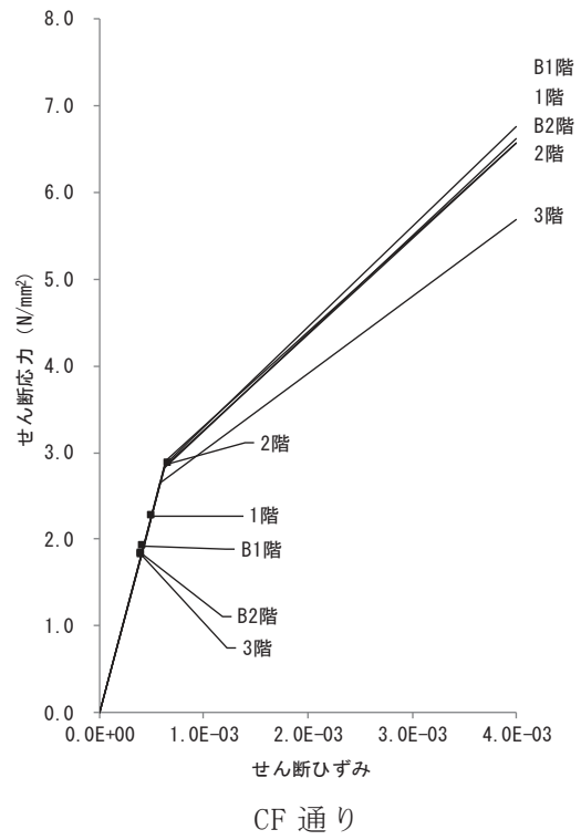
図 2-26(1) せん断スケルトンカーブ上の最大応答値(4.7地震, NS方向)
