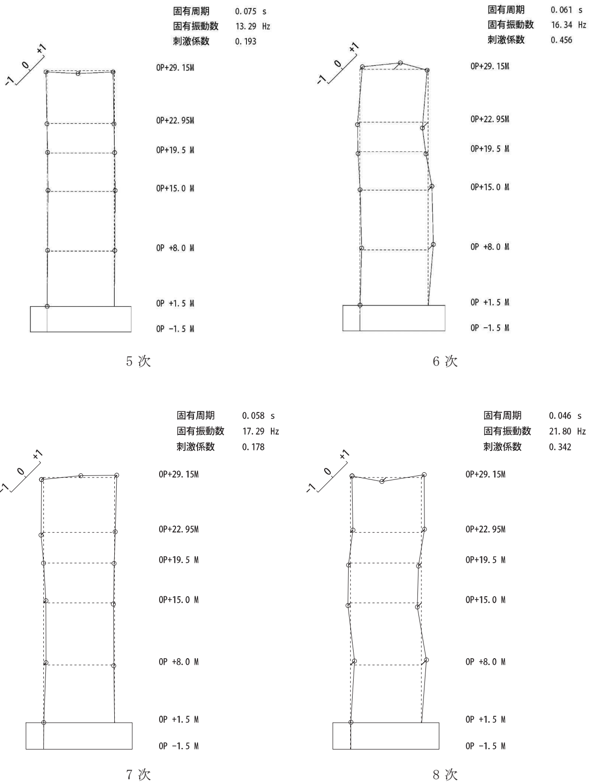
図 4-11(2) 刺激関数図 (ケース 5) (EW 方向 5 次~8 次)
