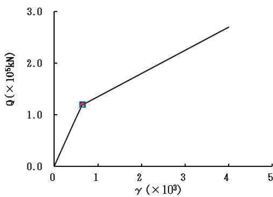
図 2-31 (2) せん断スケルトンカーブ上の最大応答値 (S s - D 2, NS 方向) (2/2)
