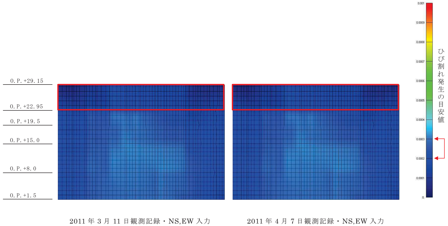
図 17 (2) 制御建屋の面内せん断ひずみコンター図 (耐震壁 3階 C1 通り)
