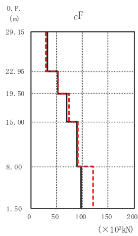
図 2-3 (2) 最大応答せん断力 (基準地震動 S s, NS 方向) (2/3)
