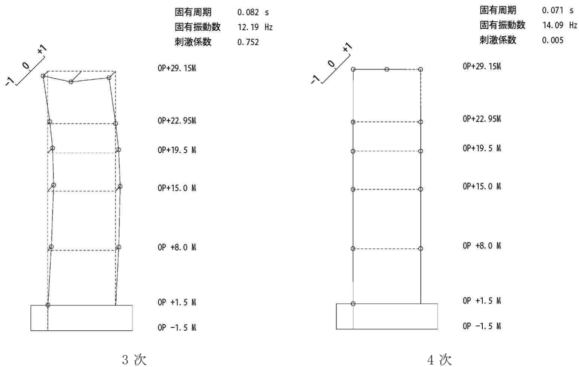
図 4-5(1) 刺激関数図 (ケース 2) (EW 方向 1 次~4 次)
