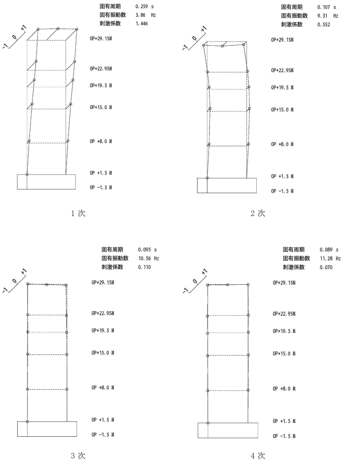
図 4-2(1) 刺激関数図 (ケース 4) (NS 方向 1 次~4 次)
