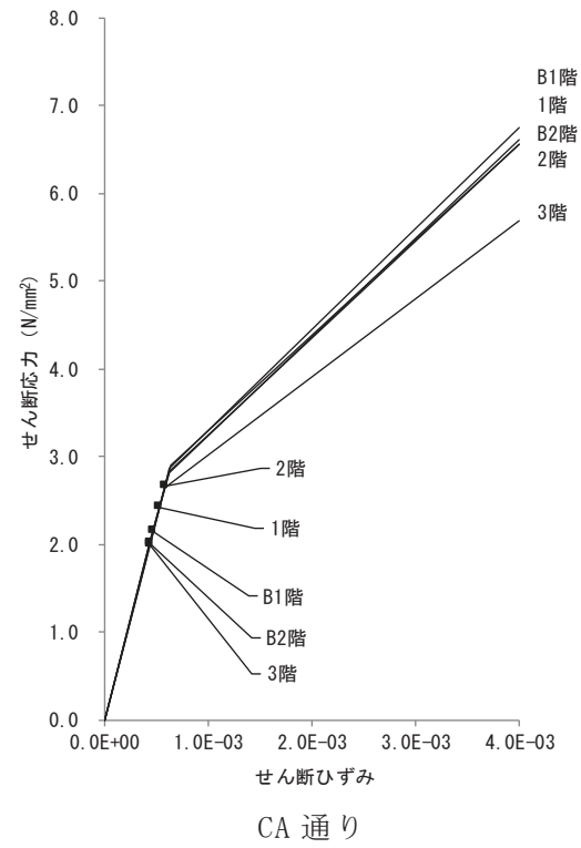
図 2-25(1) せん断スケルトンカーブ上の最大応答値(3.11地震, NS方向)
