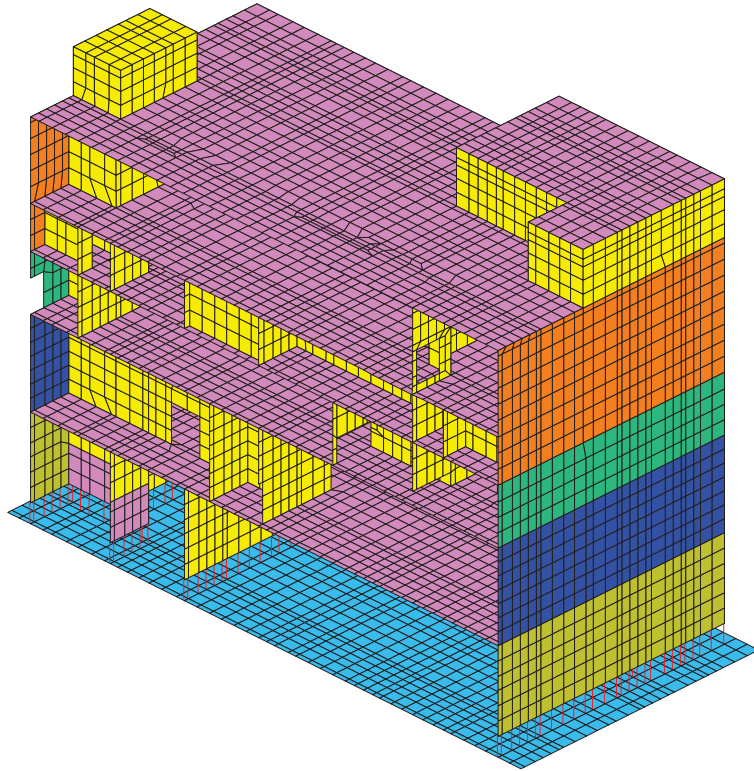
図2-1 3次元FEMモデル断面図
