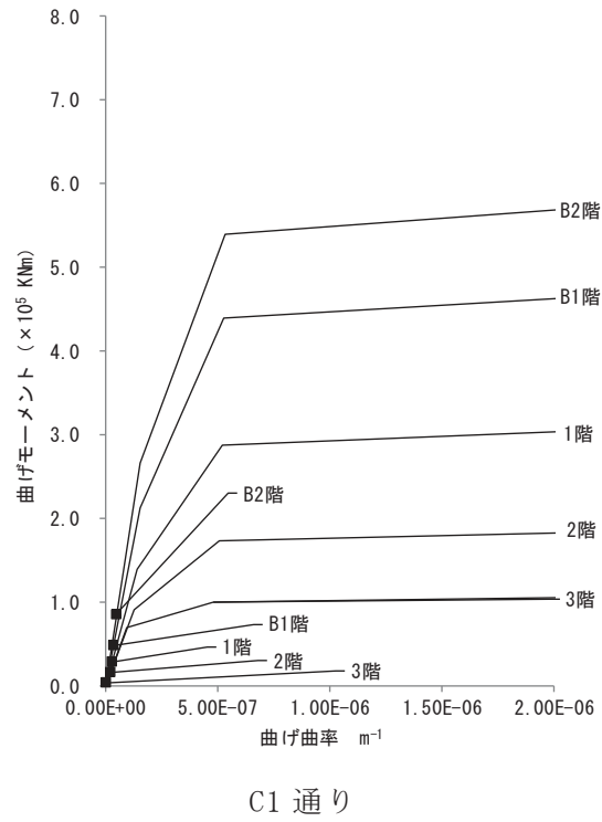
図 2-27(2) 曲げスケルトンカーブ上の最大応答値(3.11 地震, EW 方向)
