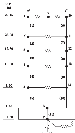
図 2-15 (2) せん断スケルトンカーブ上の最大応答値 (S s - D 2, EW 方向) (2/2)
