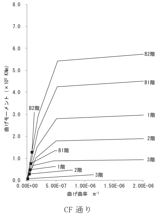
図 2-27(1) 曲げスケルトンカーブ上の最大応答値(3.11 地震, NS 方向)
