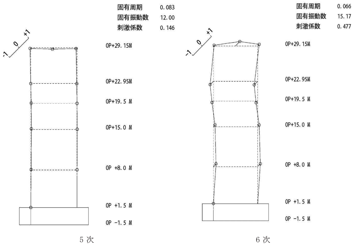
図 4-10(2) 刺激関数図 (ケース 5) (NS 方向 5 次及び 6 次)
