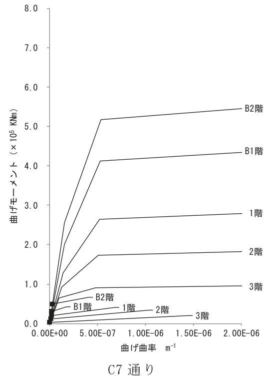
図 2-28(2) 曲げスケルトンカーブ上の最大応答値(4.7地震, EW方向)
