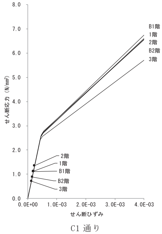
図 2-26(2) せん断スケルトンカーブ上の最大応答値(4.7地震, EW方向)
