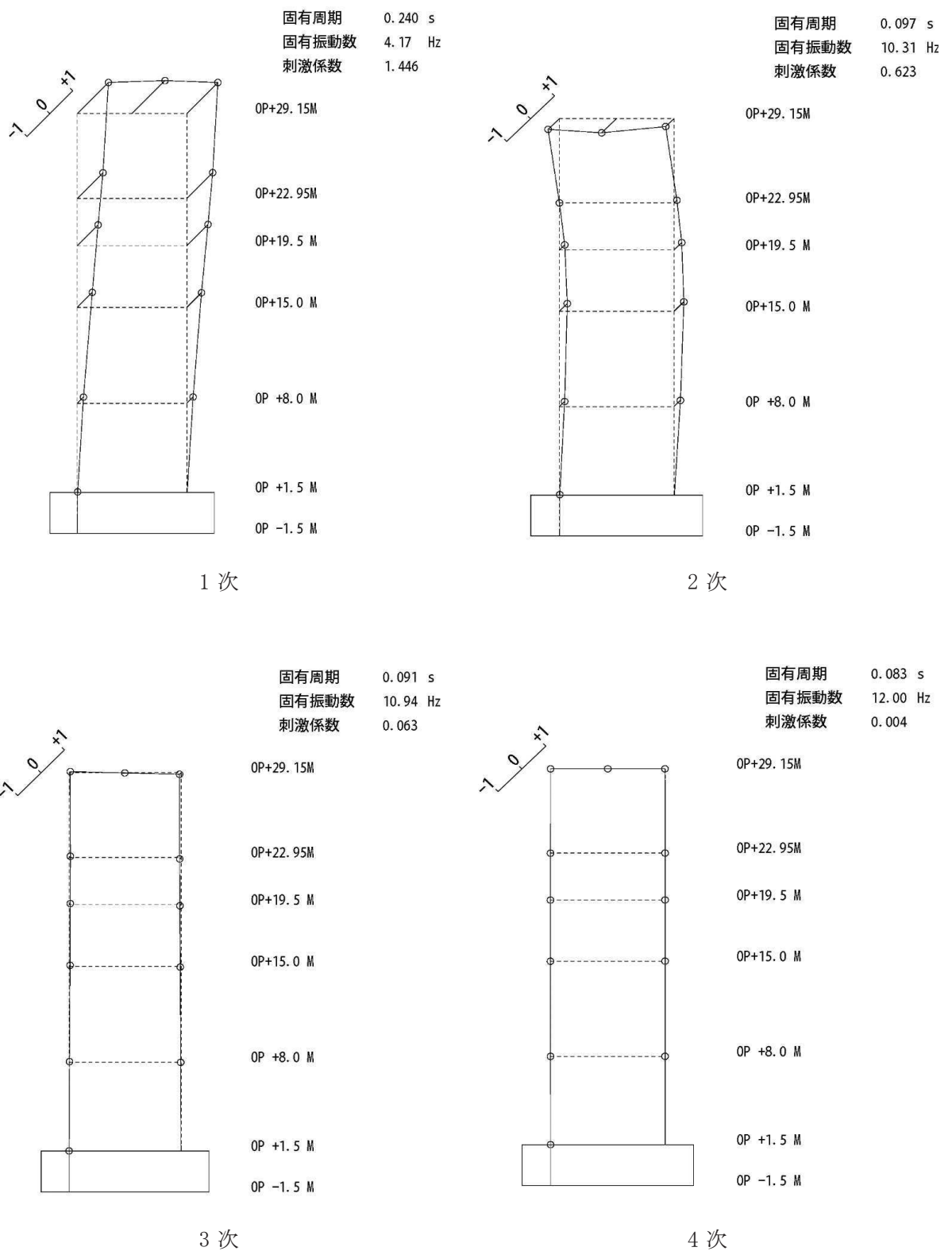
図 4-13(1) 刺激関数図 (ケース 6) (EW 方向 1 次~4 次)
