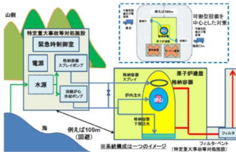
図1-5 特定重大事故等対処施設の概要 (7)
