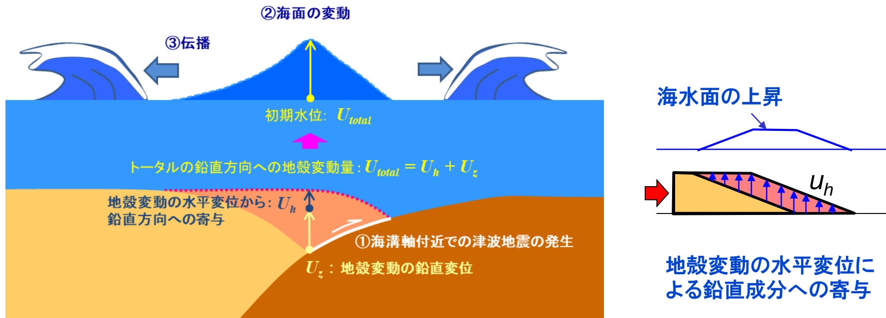
図1 津波初期水位設定のイメージ
