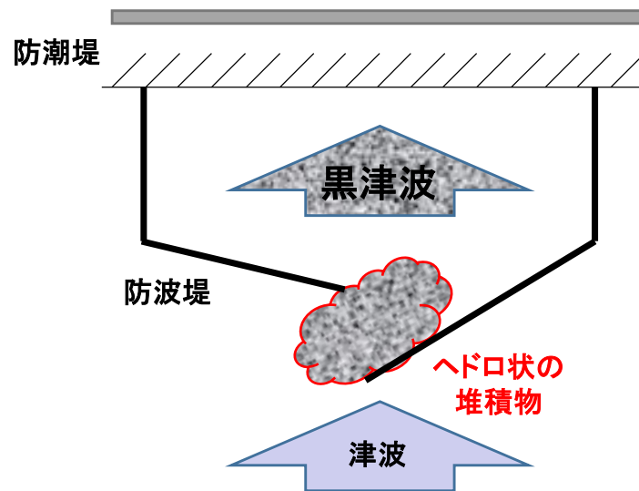
図2-1 狭窄部による黒津波発生 の概念図
