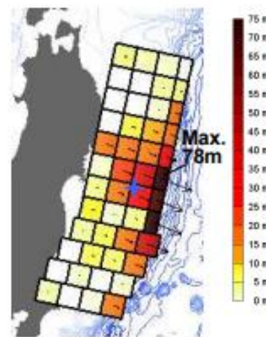
図6 初期水位の設定方法を改良した手法ですべり量分布の推定
