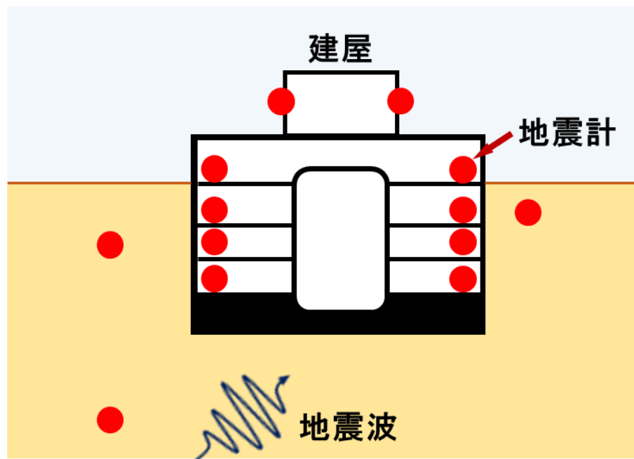
図1-2 建屋及び地盤における地震観測の概要図
