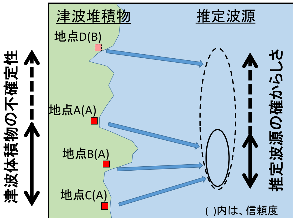
図12 津波堆積物の分布と推定波源の拡がりの相関関係のイメージ
