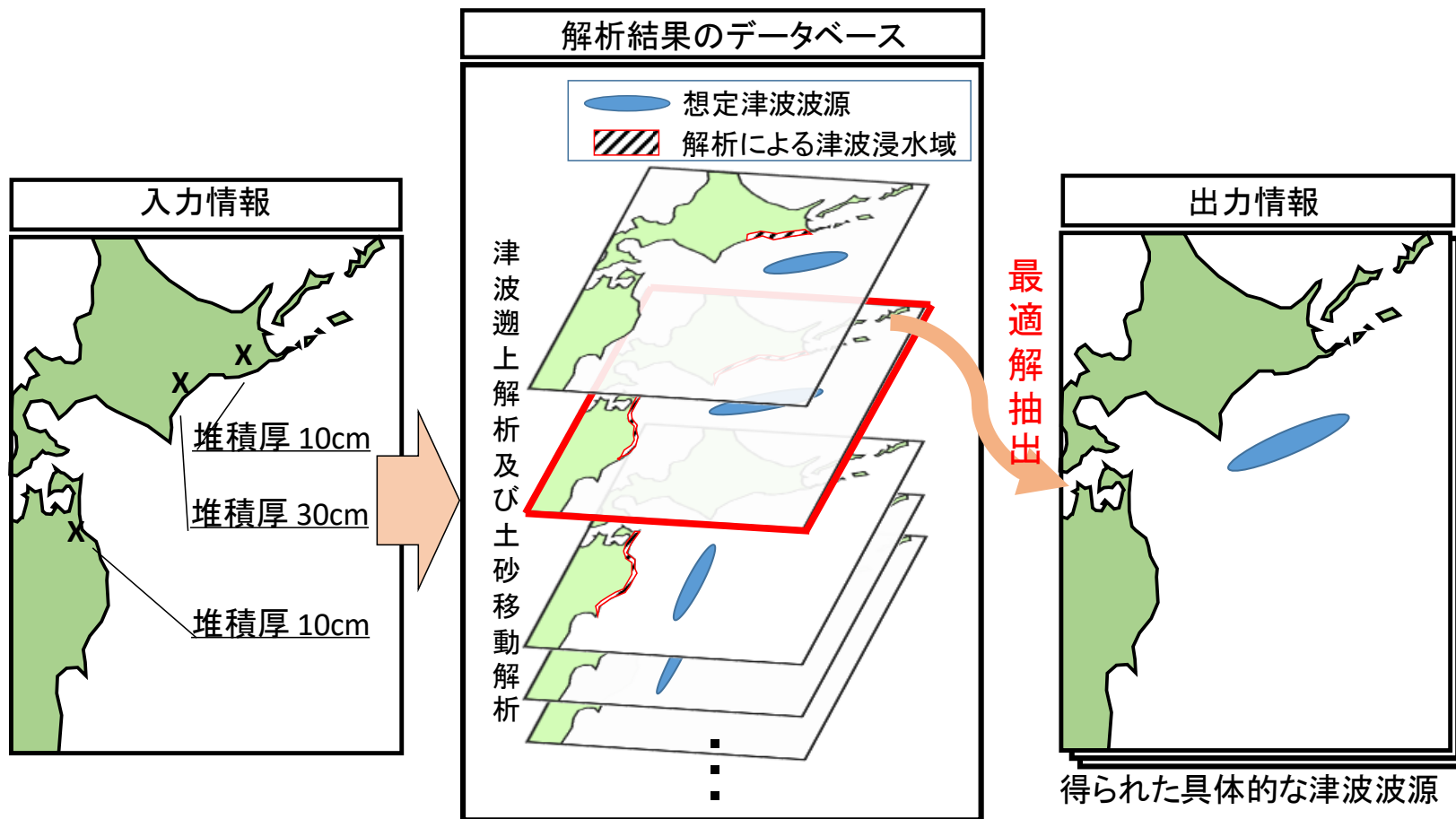
図11 1611年慶長三陸地震津波の波源推定方法のイメージ
