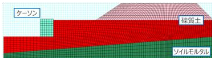
有効応力解析モデル
