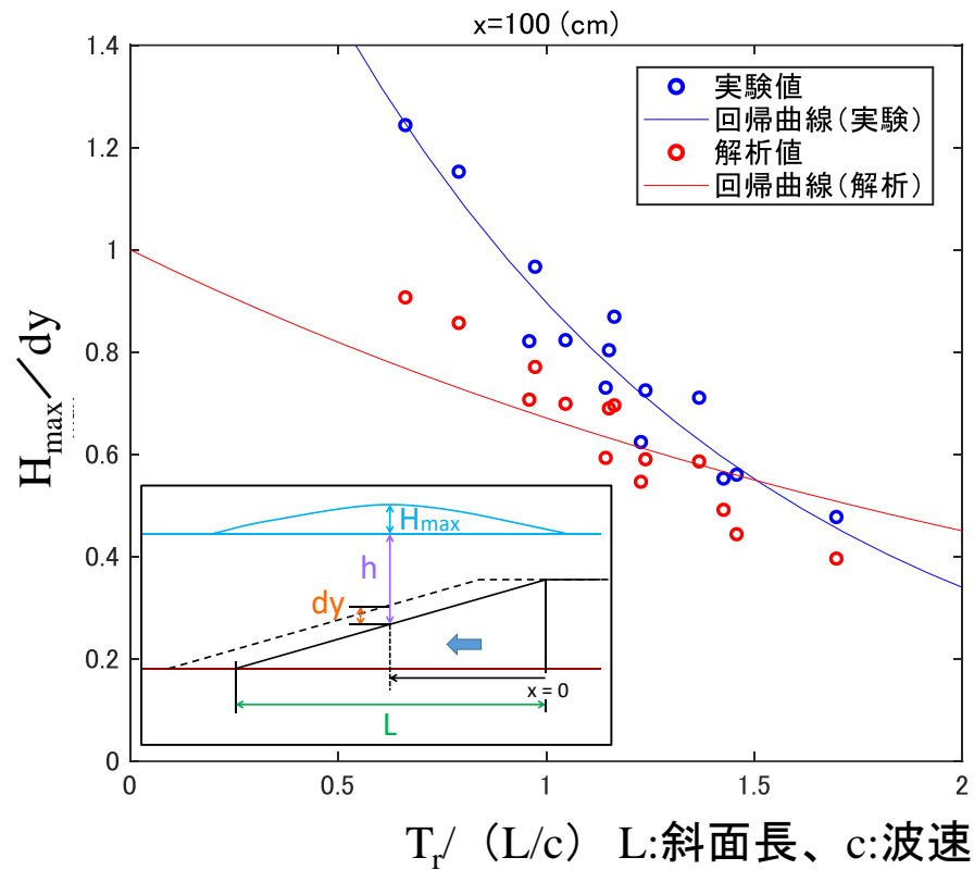
図4 最大水位 H_{max} と底面高さの増分 dy の比と無次元ライズタイム( T_r/(L/c) )の関係
