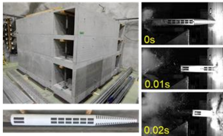
図3-1 構築物への衝突実験の一例
