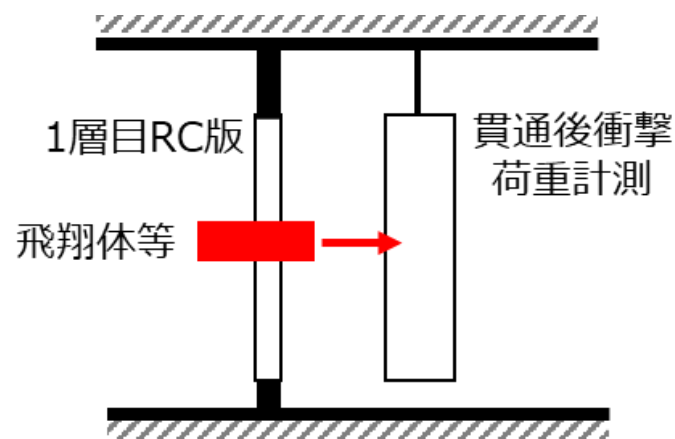
図3-3 多層版衝突実験の概念図 (既往研究の例)
