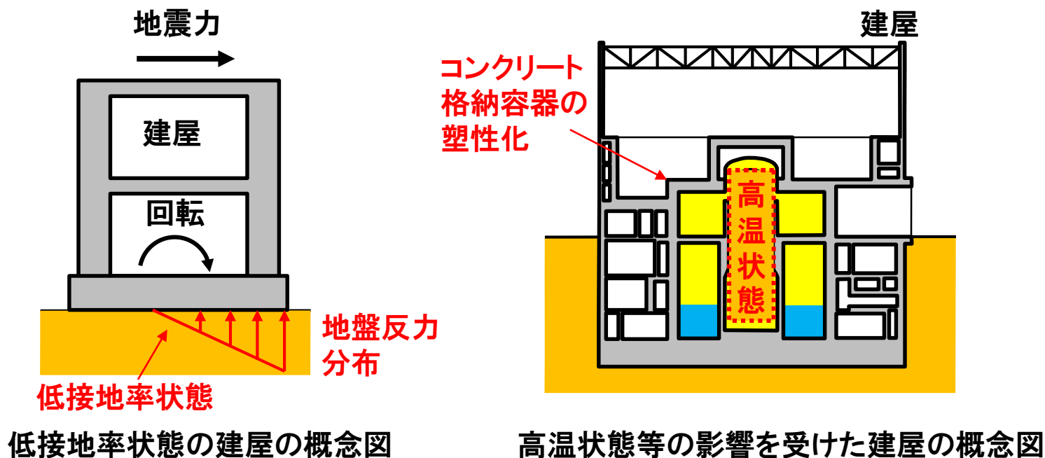
図1-1 低接地率状態の建屋及び高温状態等の影響を受けた建屋の概念図
