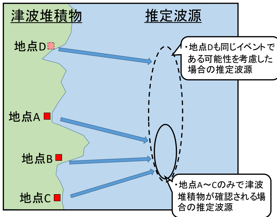
図8 津波堆積物を用いた津波波源推定のイメージ
