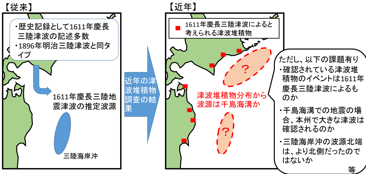
図7 1611年慶長三陸津波の津波波源に関する知見の整理
