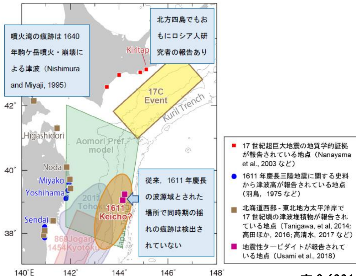
図9 1611年慶長三陸地震津波に係る津波堆積物報告地点
