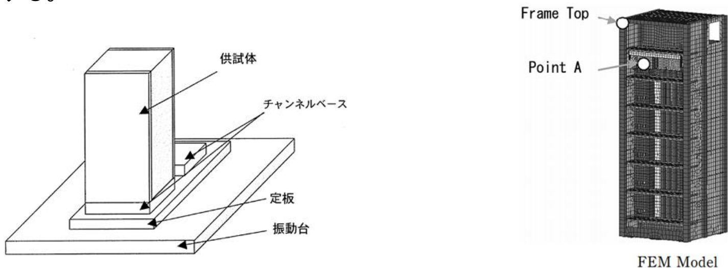
図3-5 衝撃振動試験のイメージと電気品の解析モデルの一例
