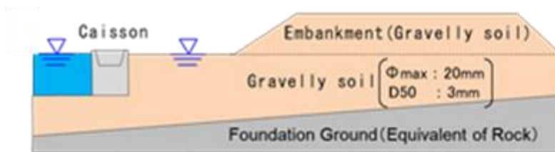
遠心模型実験モデル
