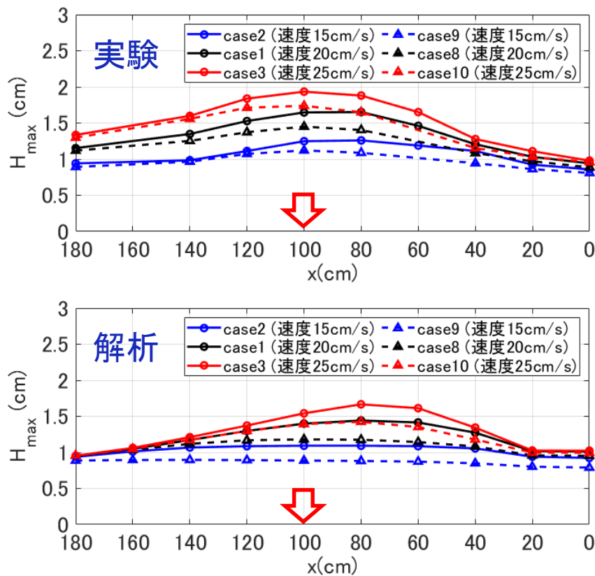
図3 速度を変化させたときの各地点での最大水位
