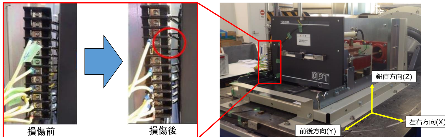
図3-4 ガタ系を有する設備の衝撃振動試験とその損傷事例
