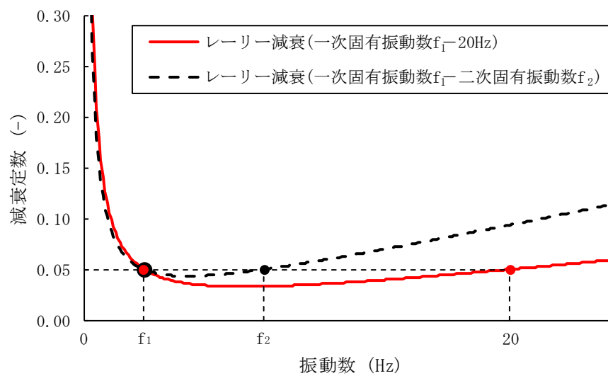
図 2-2 レーリー減衰の設定の概念図
