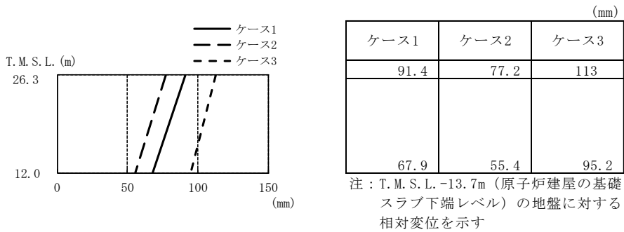
図 4-5 最大応答変位 (Ss-1, NS 方向)
