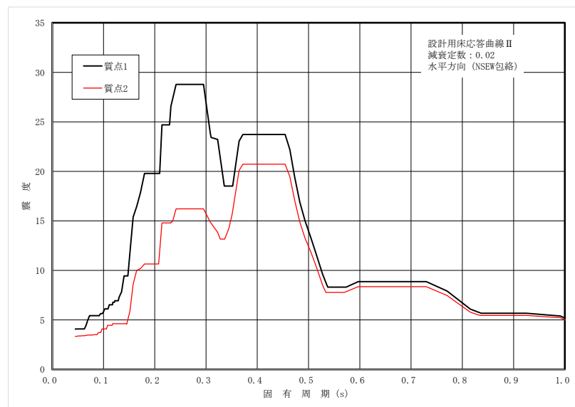
(d) 設計用床応答曲線 II (h=0.02)
