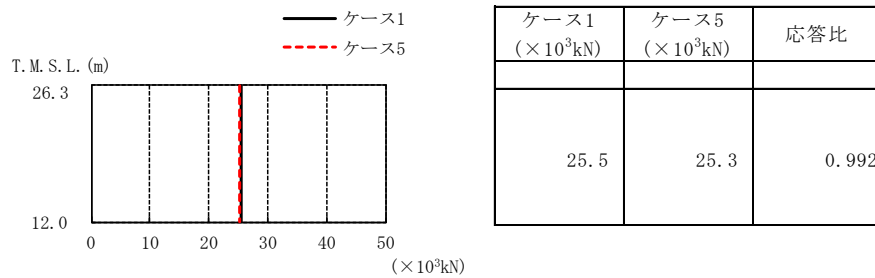
図3-4 最大応答せん断力 (Ss-1, NS方向)
