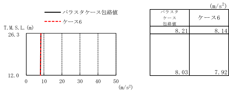
図3-22 最大応答加速度（バラストケース包絡値との比較，鉛直方向）
