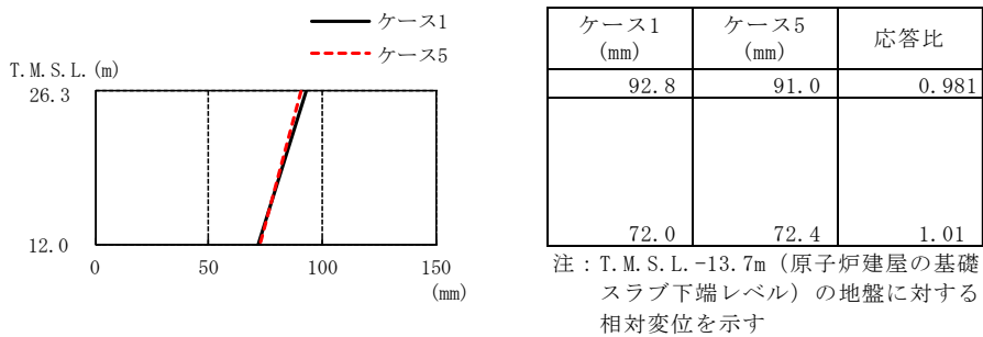
図3-7 最大応答変位 (Ss-1, EW方向)
