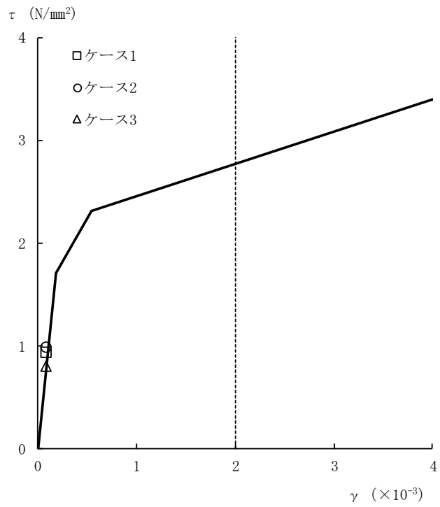
図2-15 τ - γ 関係と最大応答値 (Ss-1, EW方向)
