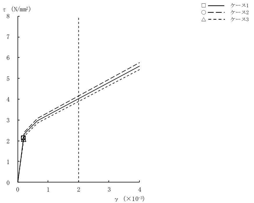
図2-16 \tau - \gamma 関係と最大応答値 (Ss-1, EW方向, B3F) (8/9)
