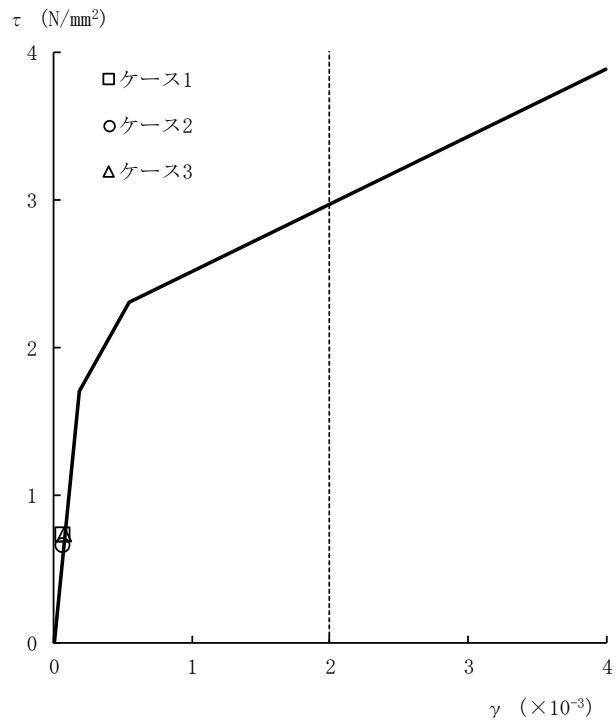
図2-14 τ - γ 関係と最大応答値 (Ss-8, NS方向)
