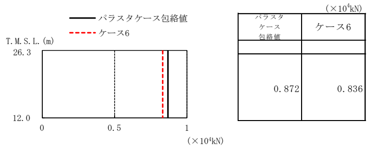
図3-24 最大応答軸力（バラストケース包絡値との比較，鉛直方向）
