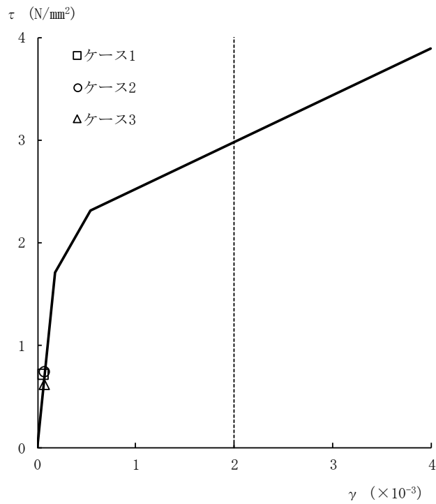
図2-13 τ - γ 関係と最大応答値 (Ss-2, NS方向)
