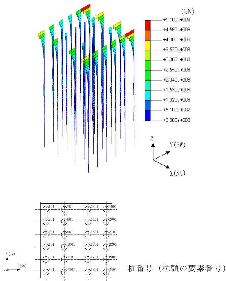
図 4-1 杭の最大応答せん断力 (基本ケース, Ss-1, EW 方向)
