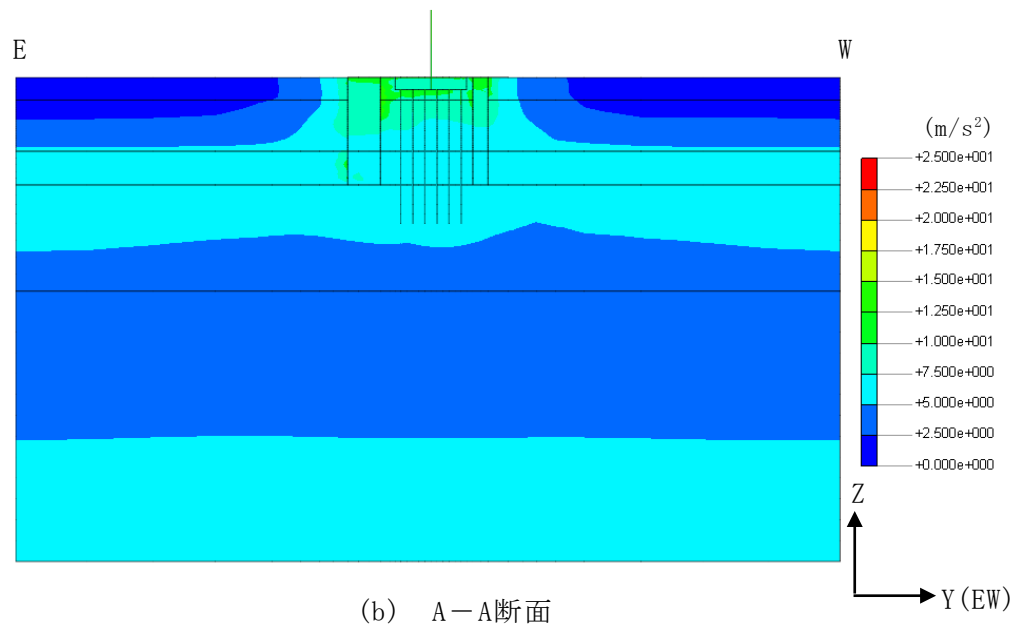
図4-2 地盤の最大応答加速度 (Ss-1, EW方向)
