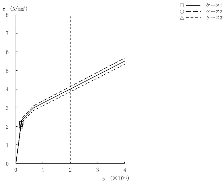
図2-15 \tau - \gamma 関係と最大応答値 (Ss-8, NS方向, B3F) (8/9)
