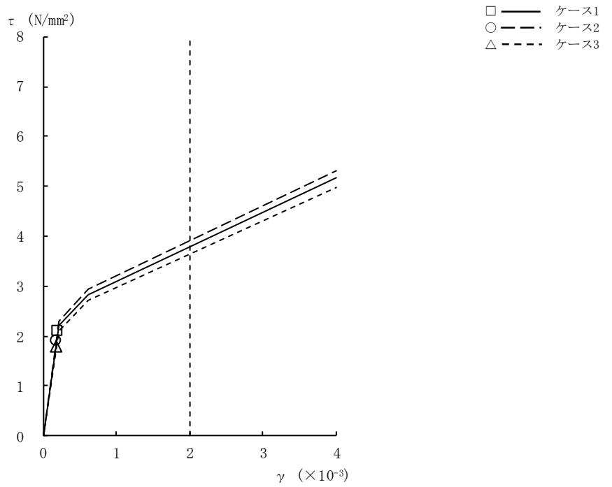
図2-17 \tau - \gamma 関係と最大応答値 (Ss-2, EW方向, B1F) (6/9)
