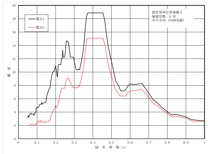
(c) 設計用床応答曲線 I (h=0.02)
