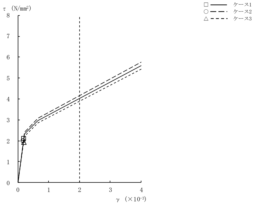
図2-19 \tau - \gamma 関係と最大応答値 (Ss-8, EW方向, B3F) (8/9)
