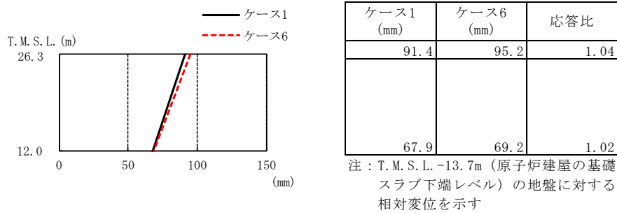
図3-2 最大応答変位 (Ss-1, NS方向)
