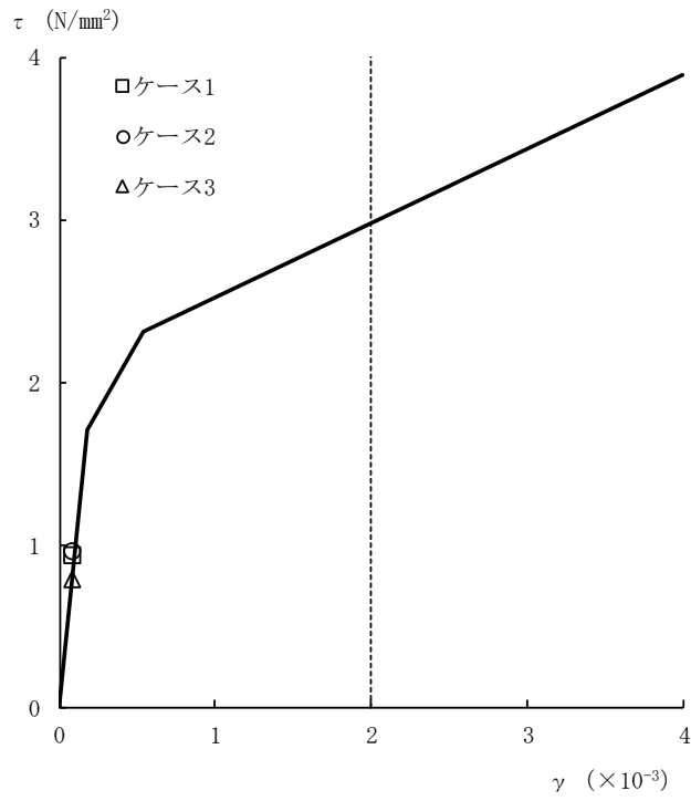
図2-12 τ - γ 関係と最大応答値 (Ss-1, NS方向)
