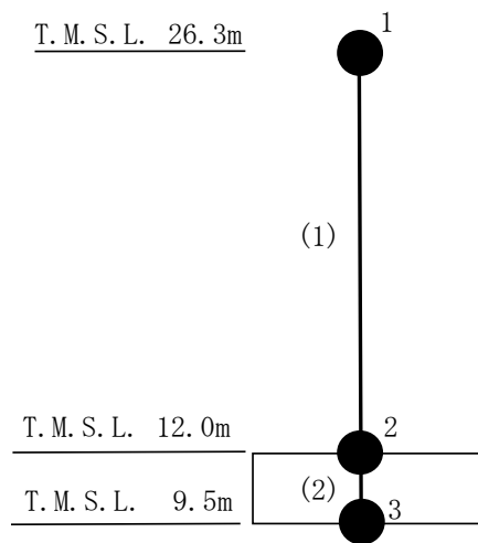
図 4-2 遮蔽壁及び基礎スラブの地震応答解析モデル
