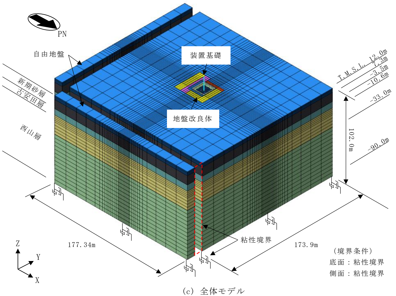
図 4-1 地震応答解析モデル
