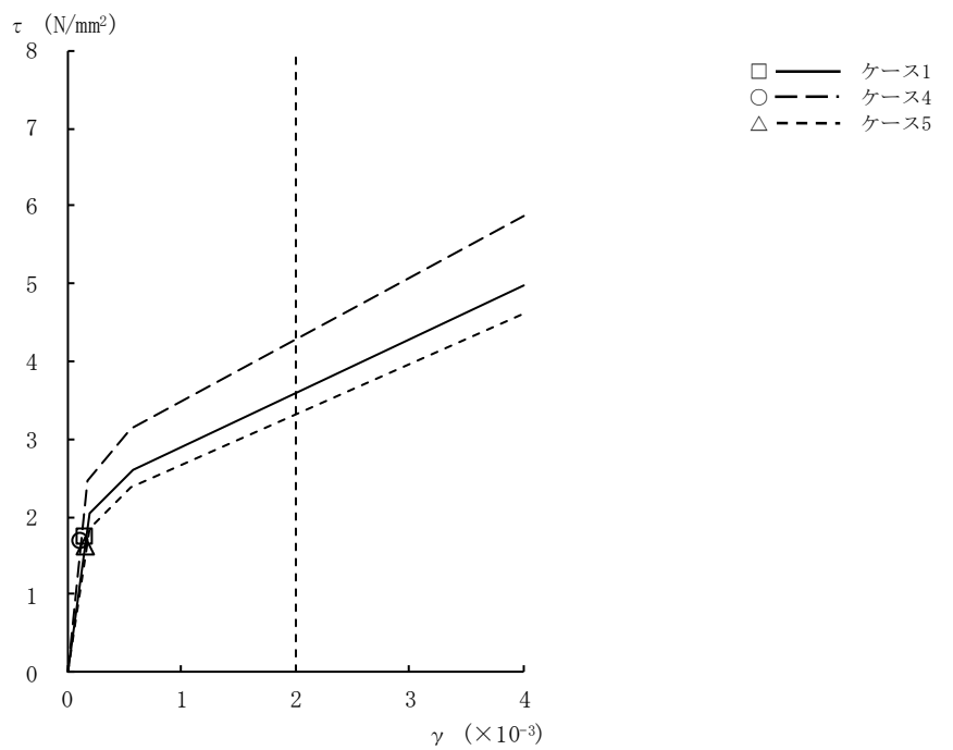
図2-35 τ - γ 関係と最大応答値 (Ss-1, EW方向, 2F) (4/9)
