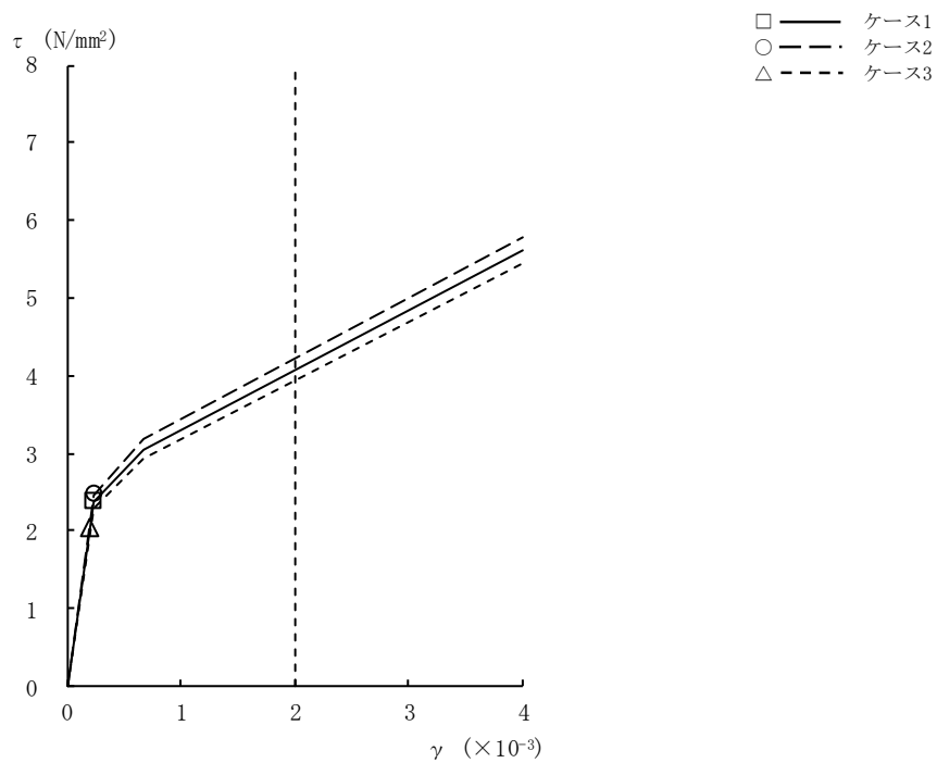
図2-17 τ - γ 関係と最大応答値 (Ss-2, EW方向, B4F) (9/9)
