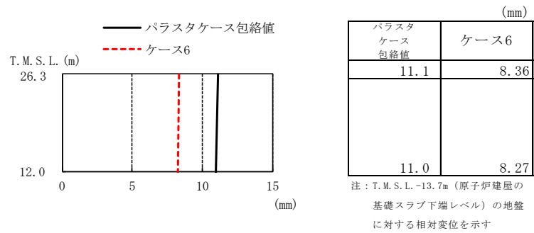
図3-23 最大応答変位（バラストケース包絡値との比較，鉛直方向）
