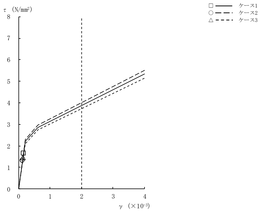
図2-13 \tau - \gamma 関係と最大応答値 (Ss-2, NS方向, B1F) (6/9)
