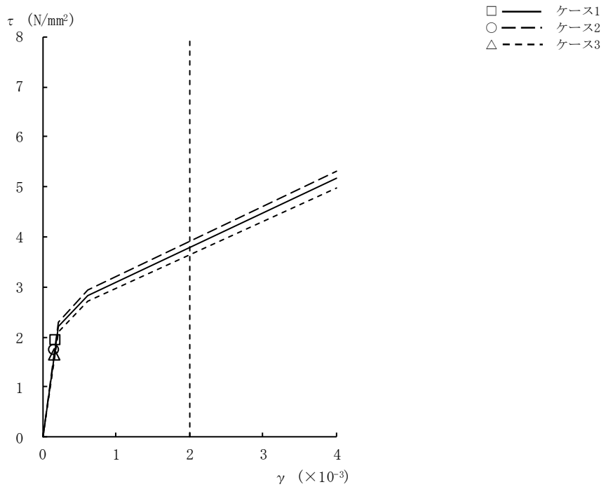
図2-16 \tau - \gamma 関係と最大応答値 (Ss-1, EW方向, B1F) (6/9)
