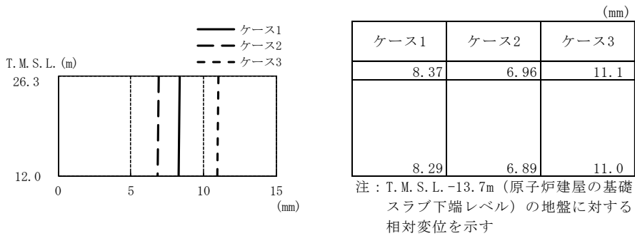
図 4-13 最大応答変位 (S S -1, 鉛直方向)
