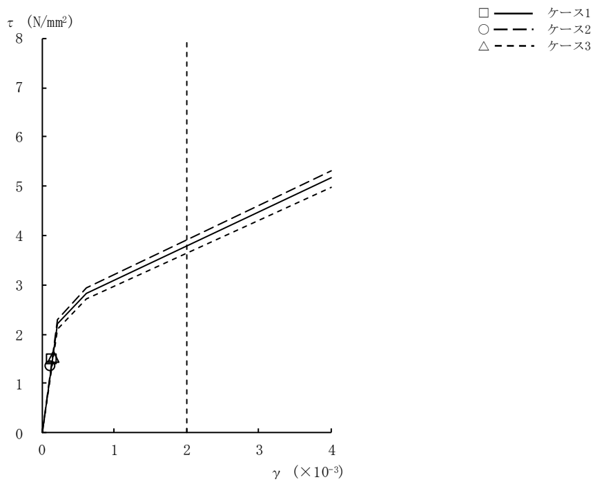
図2-18 \tau - \gamma 関係と最大応答値 (Ss-3, EW方向, B1F) (6/9)
