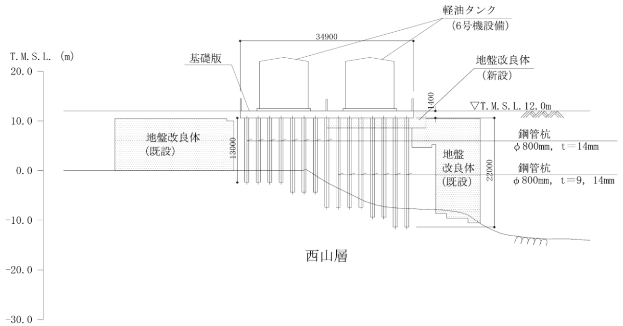
図 4-41 (2) 軽油タンク基礎 (6号機設備) の断面図 (B-B断面)
