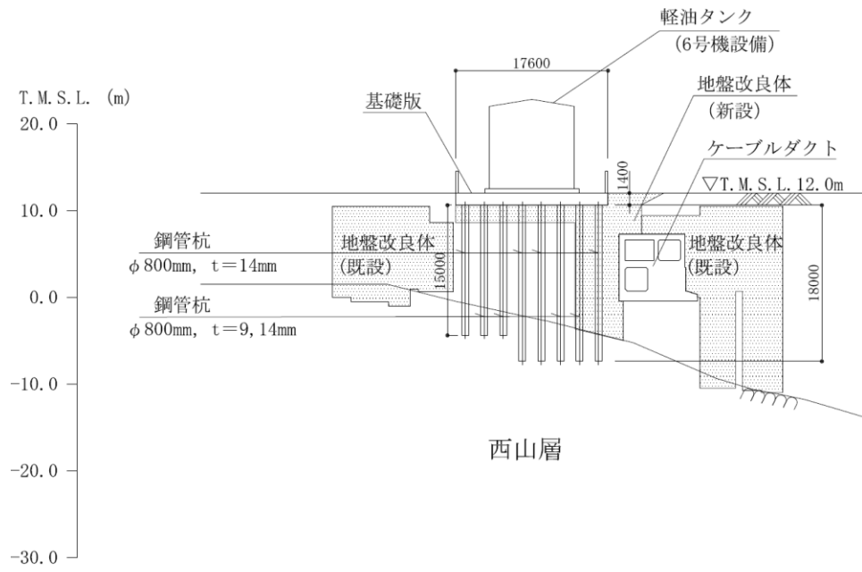
図 4-41 (1) 軽油タンク基礎 (6号機設備) の断面図 (A-A断面)
