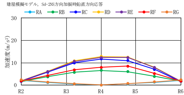
(d) 建屋模擬モデル Sd-2
