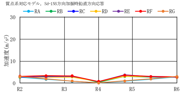
(a) 質点系対応モデル Sd-1
