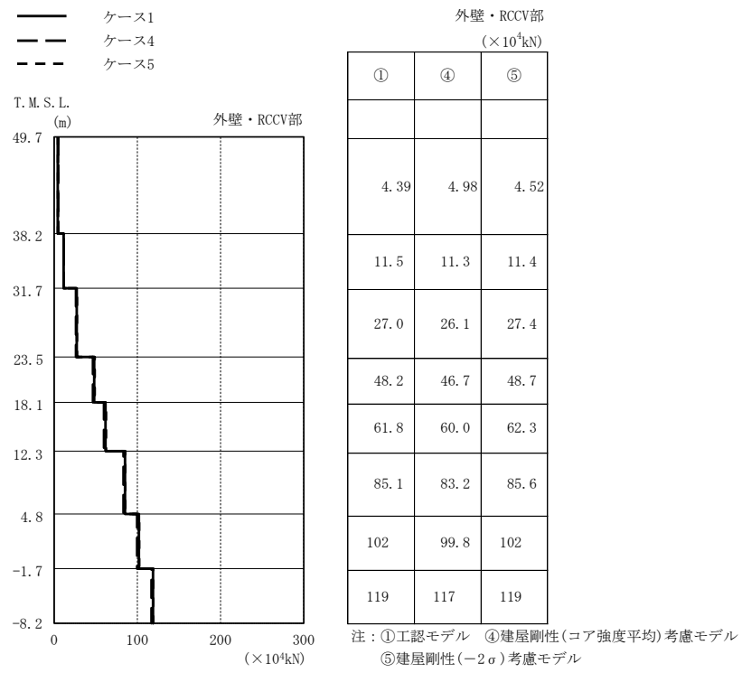
図4-38 最大応答軸力 (Ss-1, 鉛直方向)
