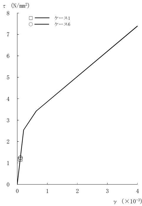
図2-122 τ - γ 関係と最大応答値 (Sd-3, EW方向, B1F) (6/8)
