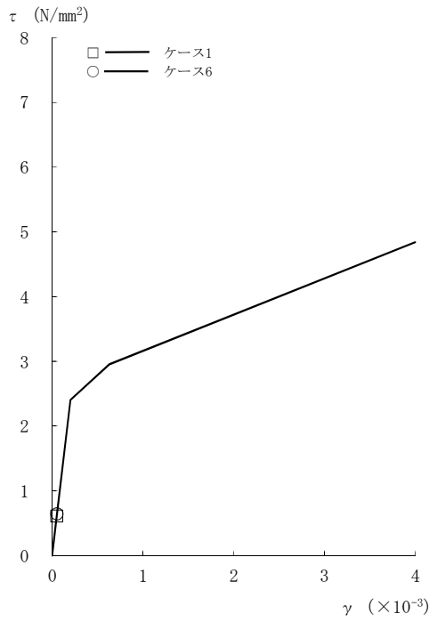
図2-118 τ - γ 関係と最大応答値 (Sd-3, NS方向, 3F) (3/8)
