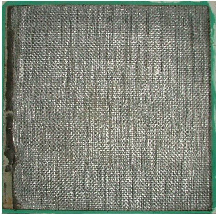
図 3-44 スケール影響試験後の供試体状況 ケース 2-4 (保護層表面)
