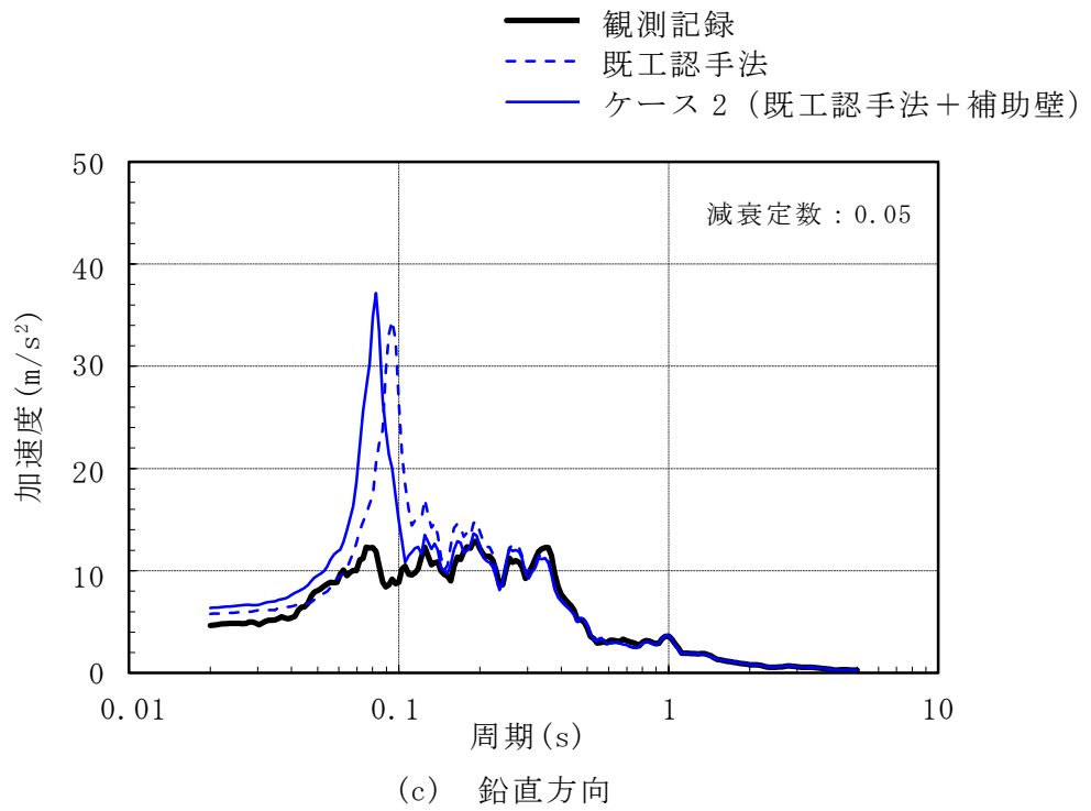
図3-7 加速度応答スペクトルの比較 (T. M. S. L. 23.5m) (ケース2) (2/2)
