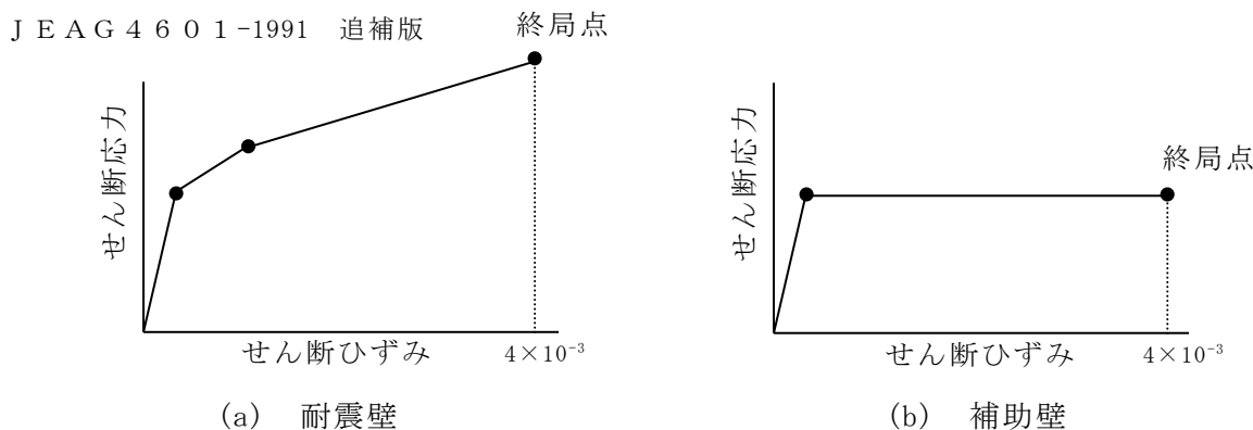
図3-1 せん断に関するスケルトン曲線の概念図
