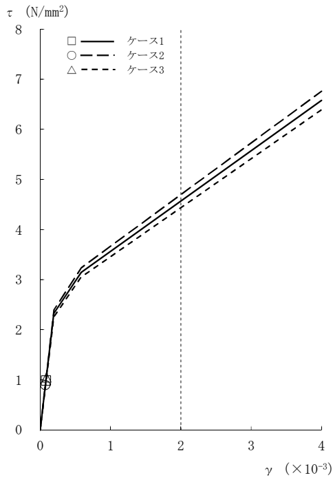
図2-25 \tau - \gamma 関係と最大応答値 (Ss-8, EW方向, CRF) (1/8)
