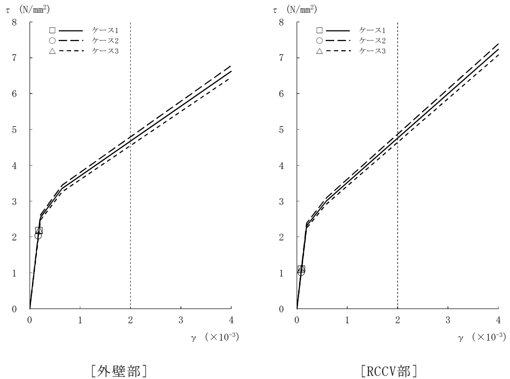
図2-19 \tau - \gamma 関係と最大応答値 (Ss-2, NS方向, 2F) (4/8)
