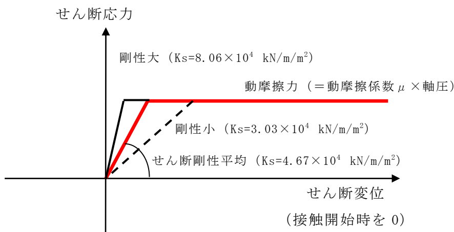
図 6 せん断剛性をばらつかせた場合のせん断ばねの特性
