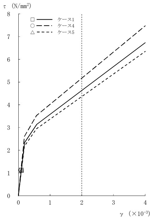
図2-66 τ - γ 関係と最大応答値 (Ss-8, EW方向, 4F) (2/8)
