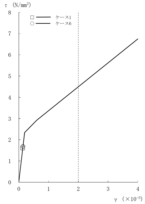
図2-103 τ - γ 関係と最大応答値 (Ss-8, NS方向, 1F) (5/8)
