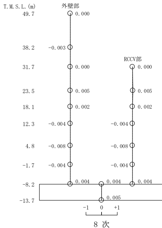
図4-3 刺激関数図 (ケース2) (NS方向, S s -1) (2/2)
