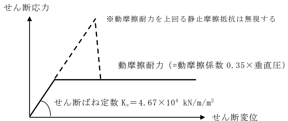
図 3-50 2次元 FEM 解析モデルで用いる地下外壁と地盤間の摩擦特性
