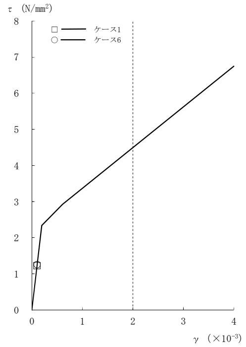
図2-102 τ - γ 関係と最大応答値 (Ss-3, NS方向, 1F) (5/8)
