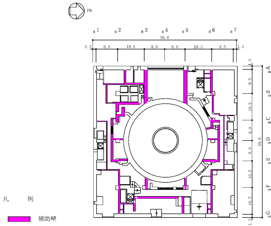
図 2-2 補助壁の考慮範囲 (1F, T. M. S. L. 12.3m) (単位 : m) (4/6)
