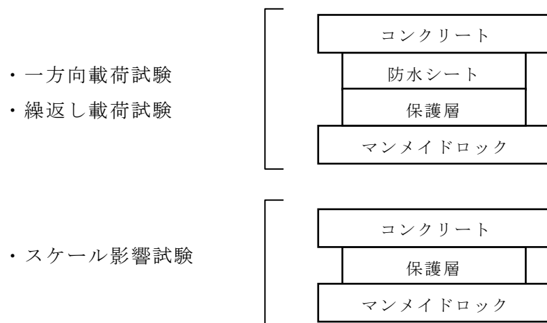
図 3-5 各試験に用いる供試体
