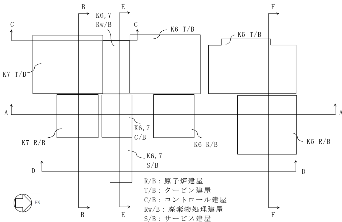
図 2-1 配置図
