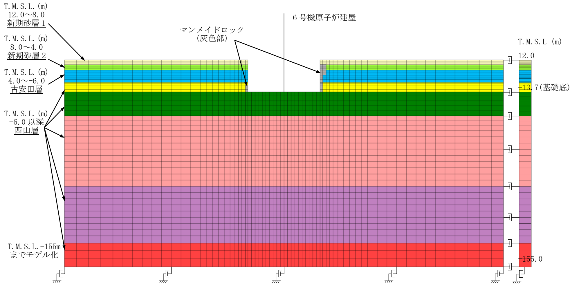
図 4-5 地盤メッシュ図 (EW 方向)
