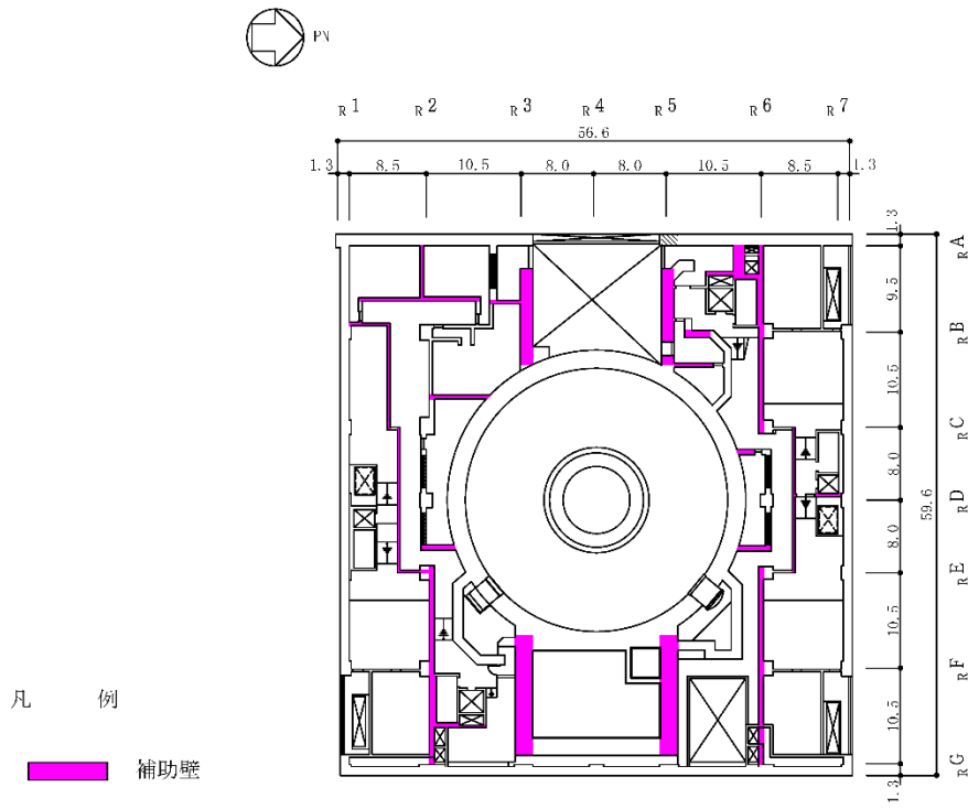
図2-2 補助壁の考慮範囲 (2F, T.M.S.L. 18.1m) (単位:m) (5/6)
