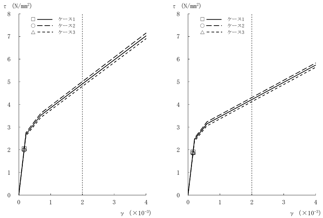
図2-19 \tau - \gamma 関係と最大応答値 (Ss-2, NS方向, B3F) (8/8)
