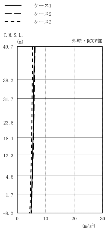
図2-9 最大応答加速度（基準地震動 S s，鉛直方向）（1/2）
