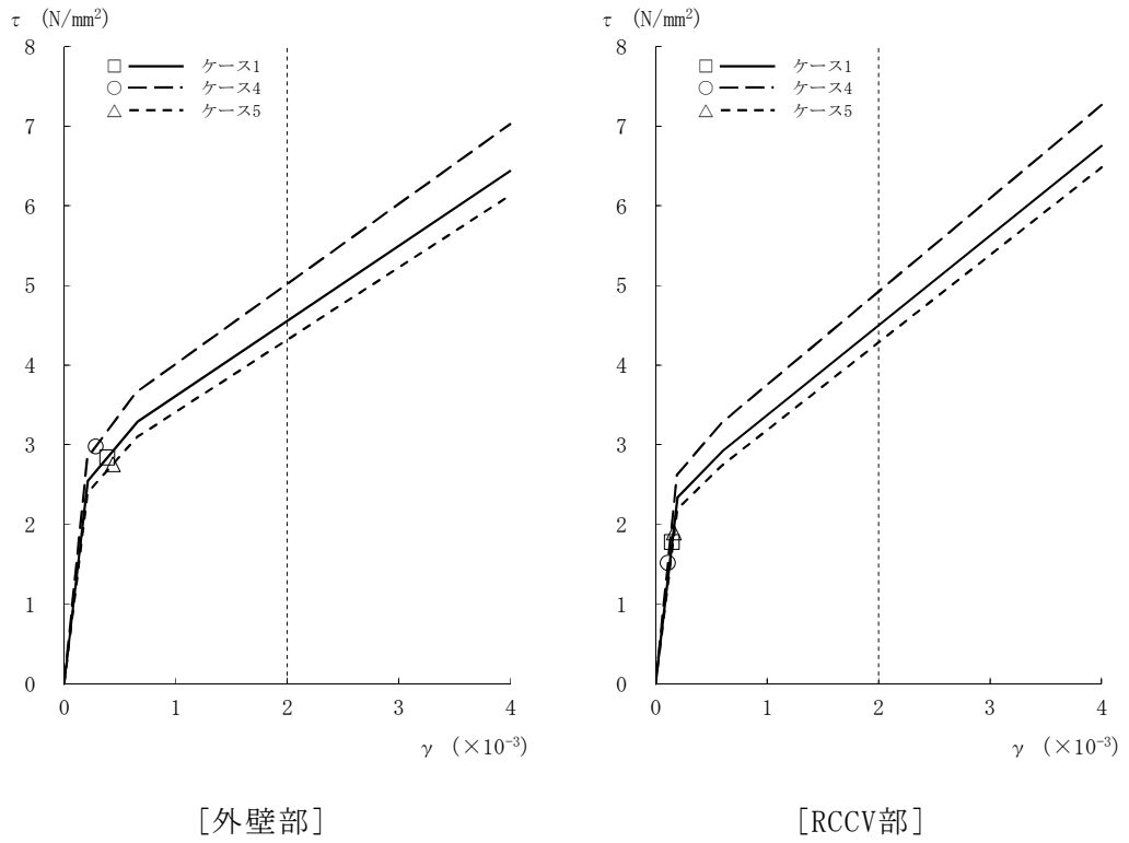
図2-59 τ - γ 関係と最大応答値 (Ss-1, NS方向, 1F) (5/8)
