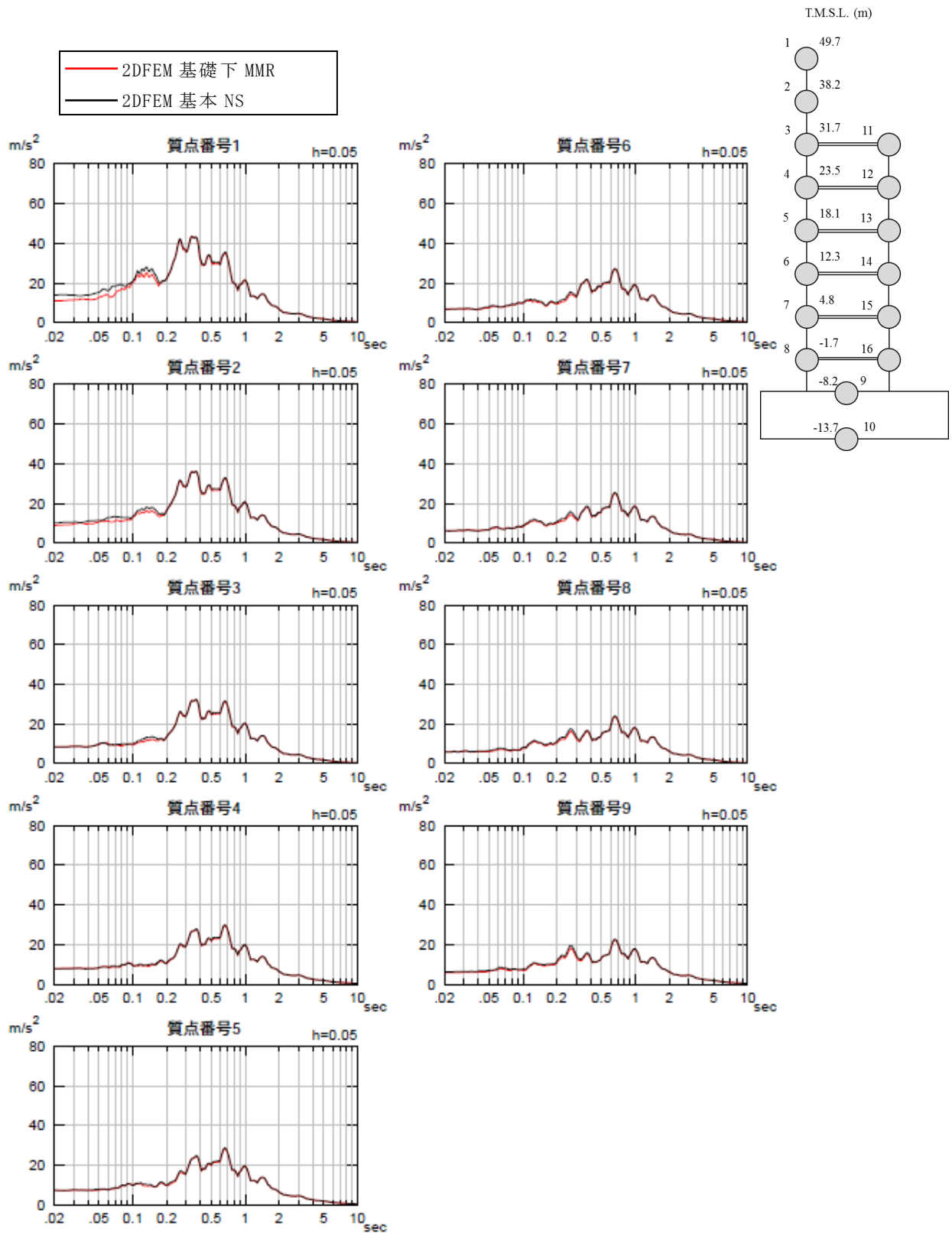
図3 床応答スペクトルの比較 (基本モデルと6号機基礎下マンメイドロックモデル) (NS方向) h=5%
