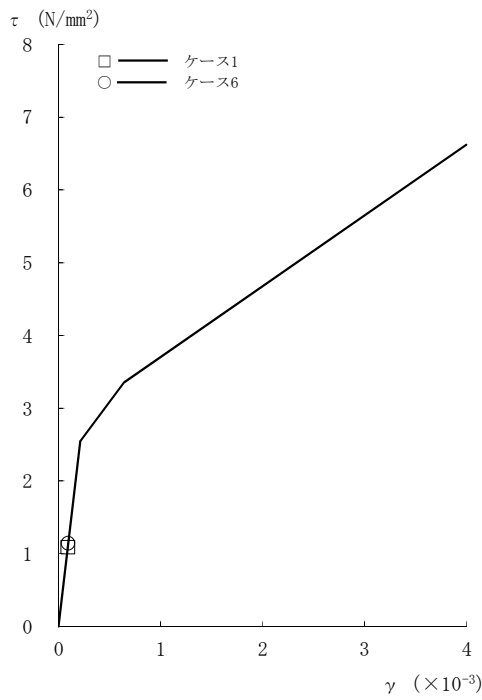
図2-118 τ - γ 関係と最大応答値 (Sd-3, NS方向, 2F) (4/8)
