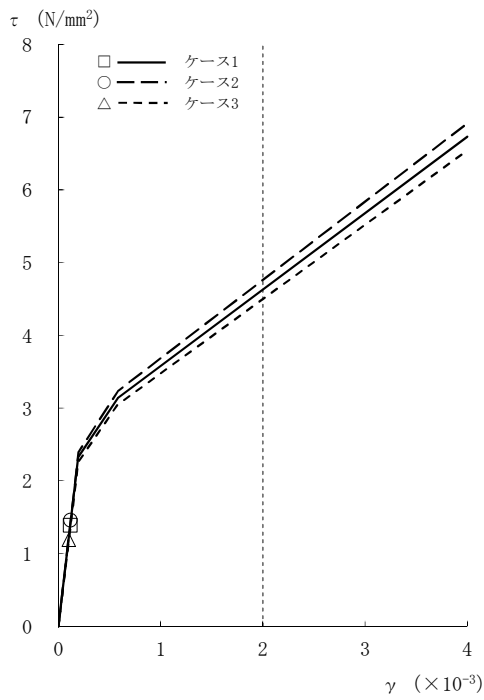
図2-22 \tau - \gamma 関係と最大応答値 (Ss-1, EW方向, 4F) (2/8)
