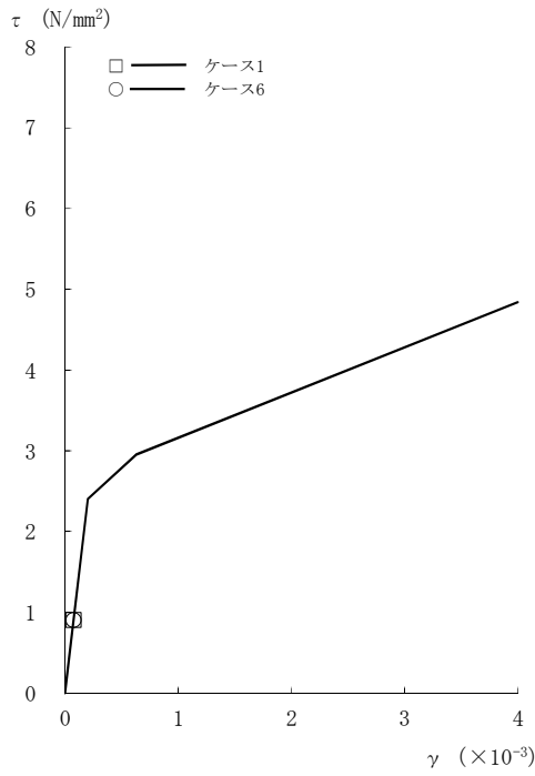
図2-116 τ - γ 関係と最大応答値 (Sd-1, NS方向, 3F) (3/8)
