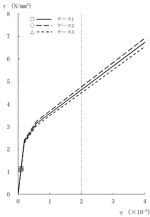
図2-25 \tau - \gamma 関係と最大応答値 (Ss-8, EW方向, 4F) (2/8)
