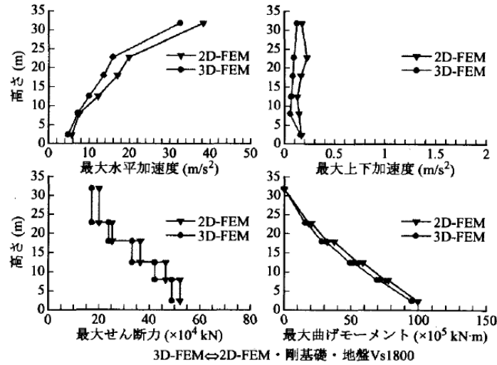
3D-FEM⇔2D-FEM・剛基礎・地盤 V_s1800 図6 解析次元の違いによる建屋最大応答値の比較
