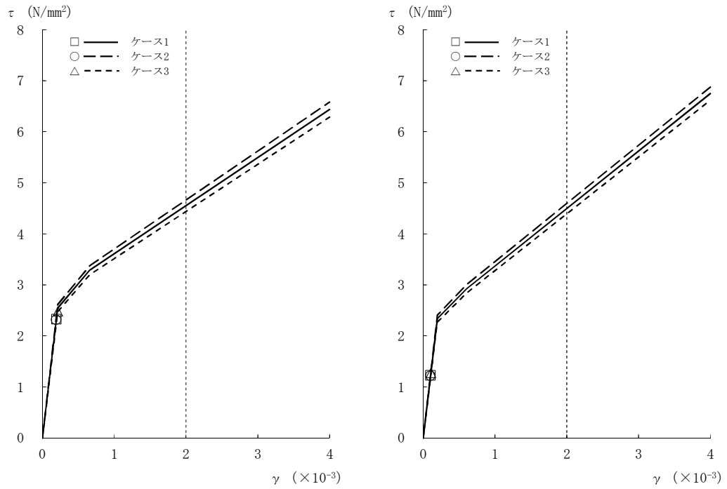
図2-20 \tau - \gamma 関係と最大応答値 (Ss-3, NS方向, 1F) (5/8)
