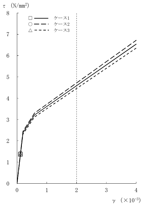
図2-19 τ - γ 関係と最大応答値 (Ss-2, NS方向, 4F) (2/8)
