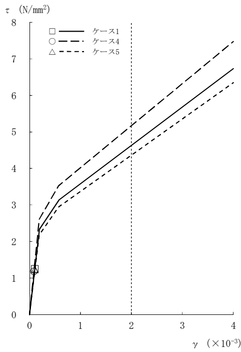
図2-64 \tau - \gamma 関係と最大応答値 (Ss-2, EW方向, 4F) (2/8)
