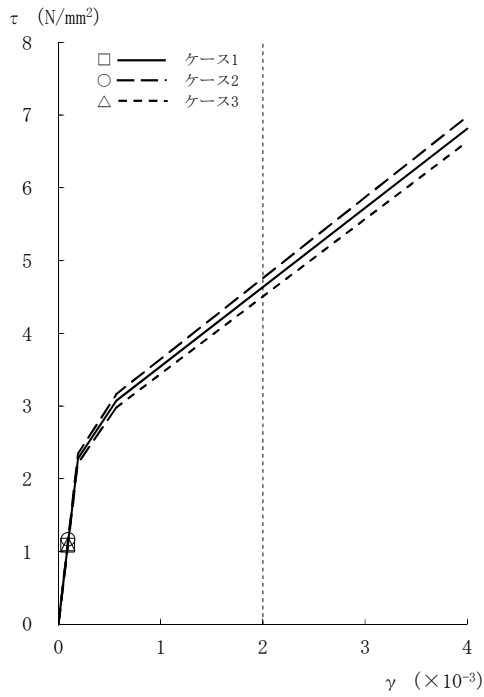
図2-19 τ - γ 関係と最大応答値 (Ss-2, NS方向, CRF) (1/8)
