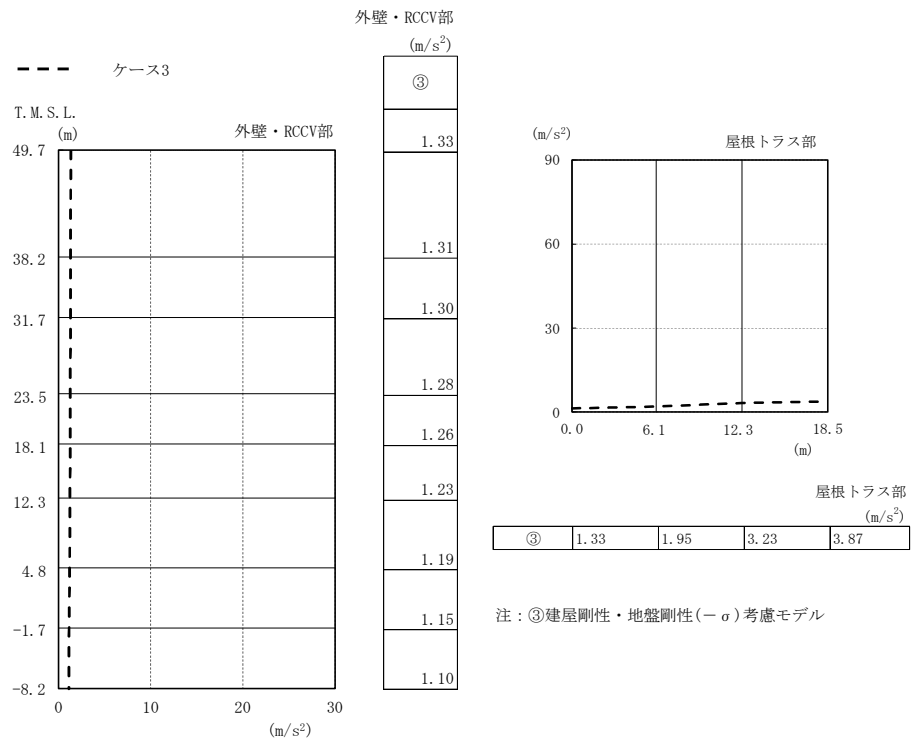
図2-12 最大応答加速度 (基準地震動 S s , NS方向, 誘発上下動)
