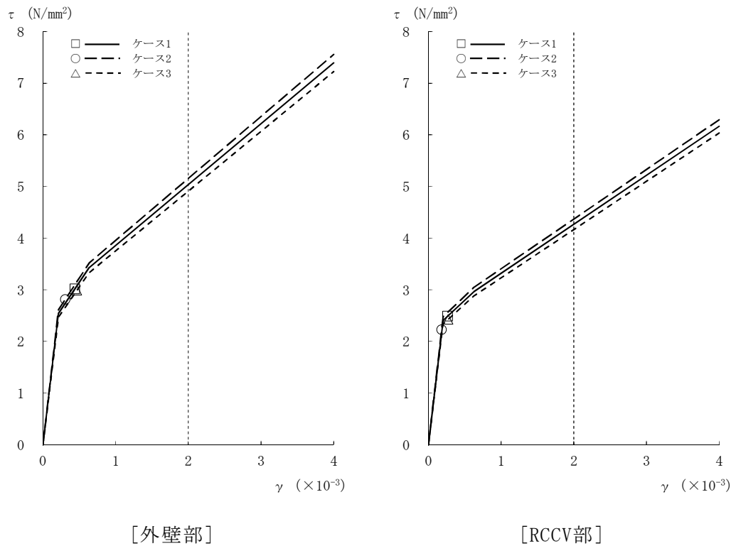
図2-23 \tau - \gamma 関係と最大応答値 (Ss-2, EW方向, B1F) (6/8)
