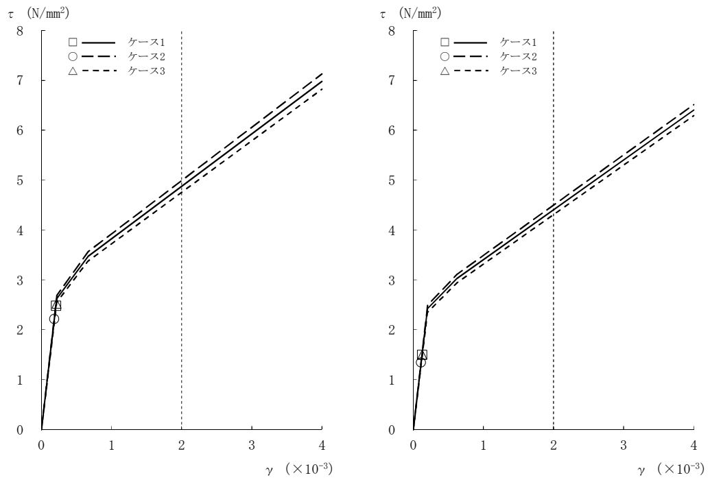
図2-19 τ - γ 関係と最大応答値 (Ss-2, NS方向, B1F) (6/8)
