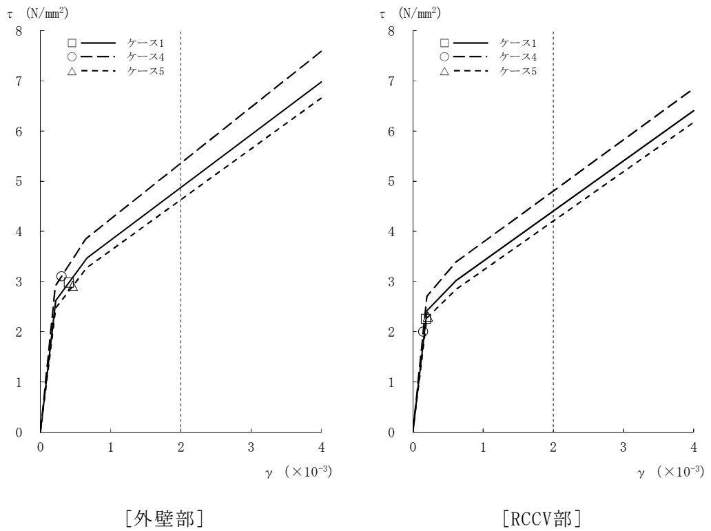
図2-59 τ - γ 関係と最大応答値 (Ss-1, NS方向, B1F) (6/8)
