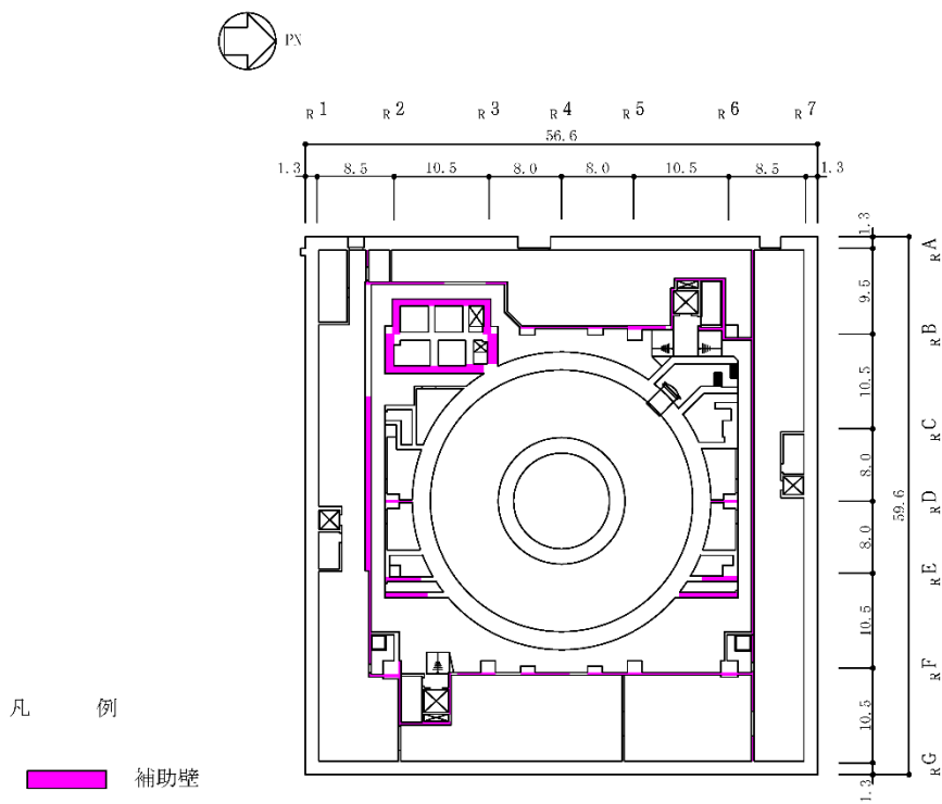
図 2-2 補助壁の考慮範囲 (B1F, T. M. S. L. 4.8m) (単位 : m) (3/6)
