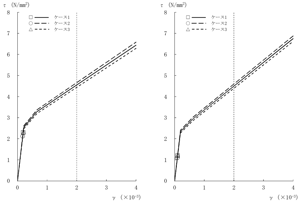
図2-19 τ - γ 関係と最大応答値 (Ss-2, NS方向, 1F) (5/8)
