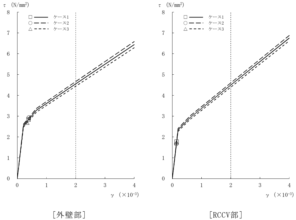
図2-18 \tau - \gamma 関係と最大応答値 (Ss-1, NS方向, 1F) (5/8)
