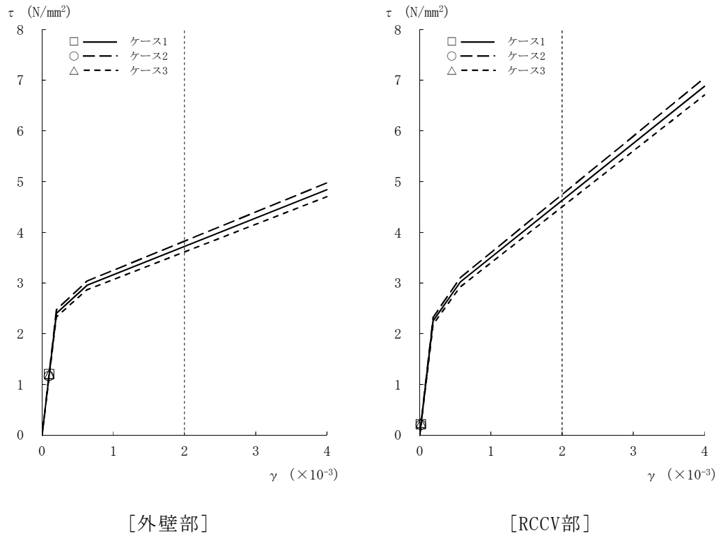
図2-19 \tau - \gamma 関係と最大応答値 (Ss-2, NS方向, 3F) (3/8)
