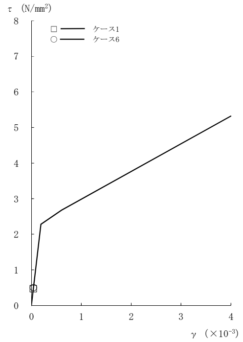
図2-122 τ - γ 関係と最大応答値 (Sd-3, EW方向, 1F) (5/8)
