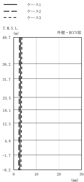
図2-10 最大応答変位 (基準地震動 S s , 鉛直方向) (2/2)
