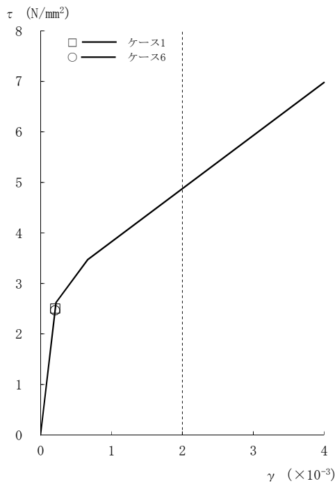
図2-102 τ - γ 関係と最大応答値 (Ss-3, NS方向, B1F) (6/8)
