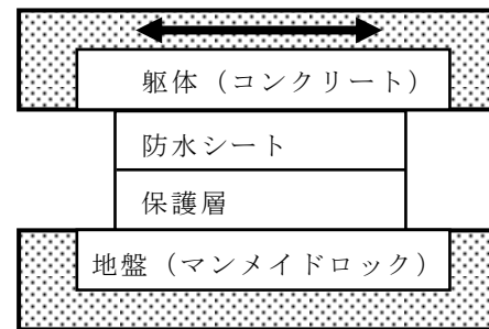
図 3-4 供試体（標準）
