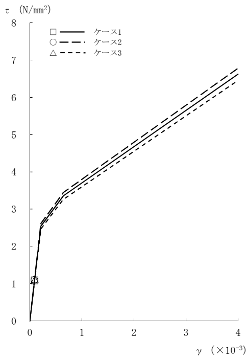
図2-39 \tau - \gamma 関係と最大応答値 (Sd-3, NS方向, 2F) (4/8)
