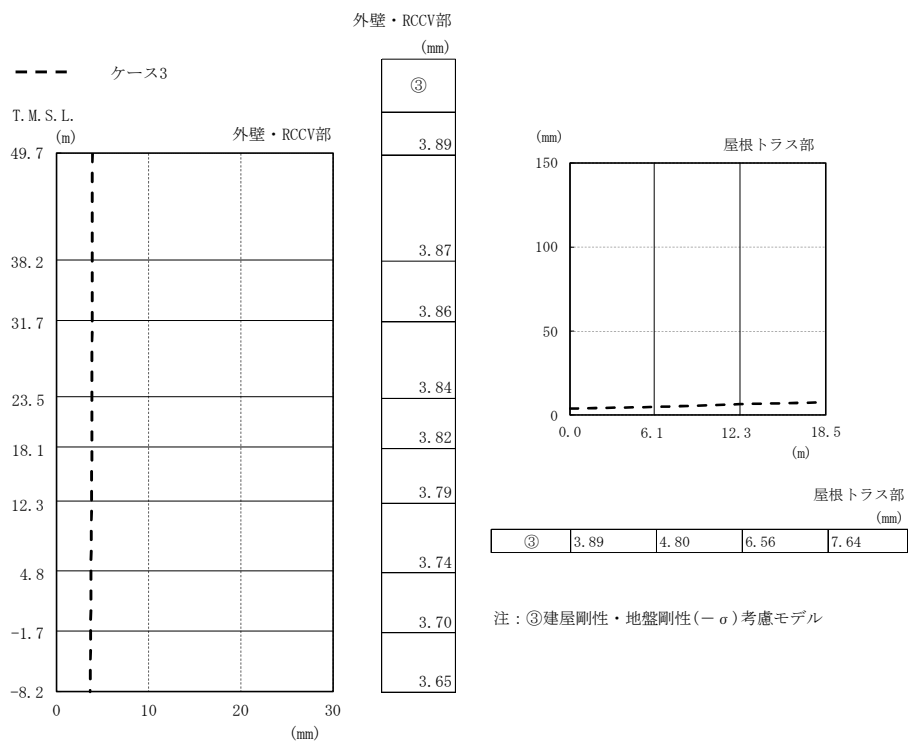
図2-13 最大応答変位 (基準地震動 S s , NS方向, 誘発上下動)
