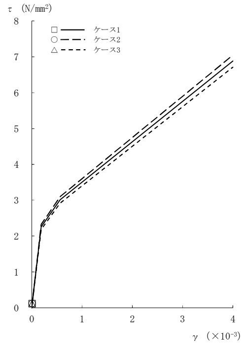
図2-39 \tau - \gamma 関係と最大応答値 (Sd-3, NS方向, 3F) (3/8)
