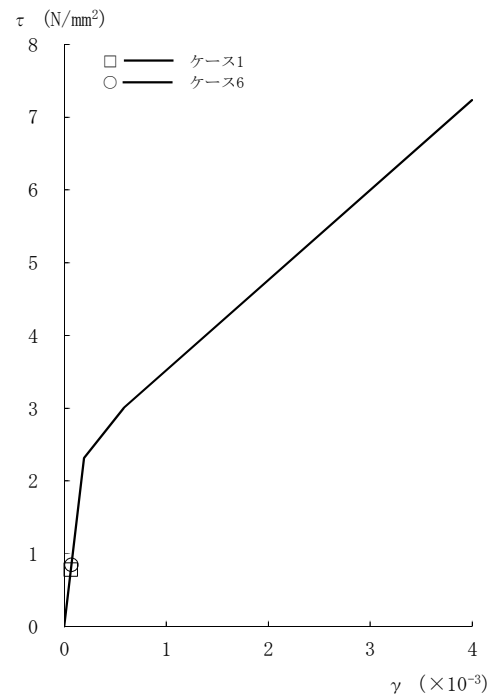
図2-116 τ - γ 関係と最大応答値 (Sd-1, NS方向, 2F) (4/8)
