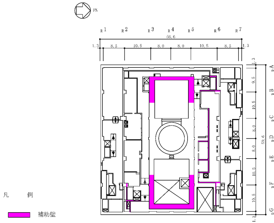
図2-2 補助壁の考慮範囲 (3F, T.M.S.L. 23.5m) (単位:m) (6/6)
