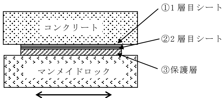
図 3-12 一方向荷重及び繰返し荷重試験供試体
