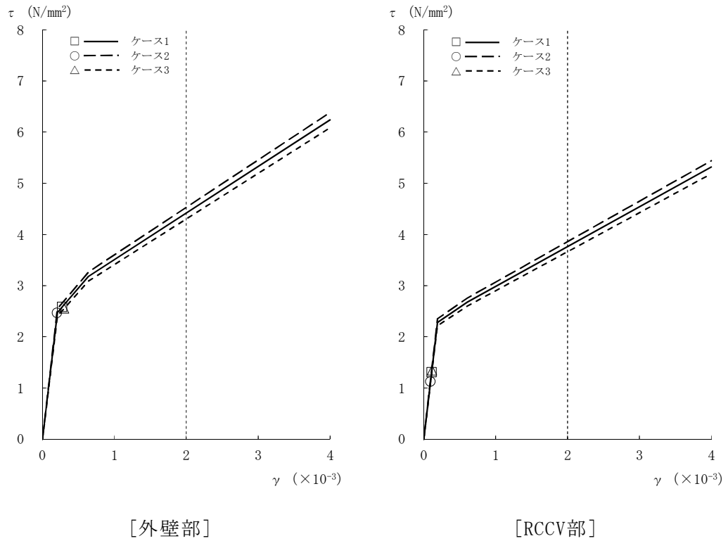
図2-23 \tau - \gamma 関係と最大応答値 (Ss-2, EW方向, 1F) (5/8)
