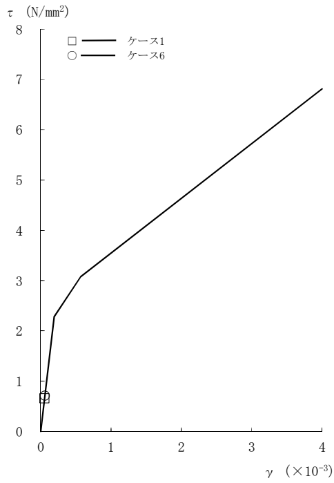
図2-119 \tau - \gamma 関係と最大応答値 (Sd-8, NS方向, CRF) (1/8)
