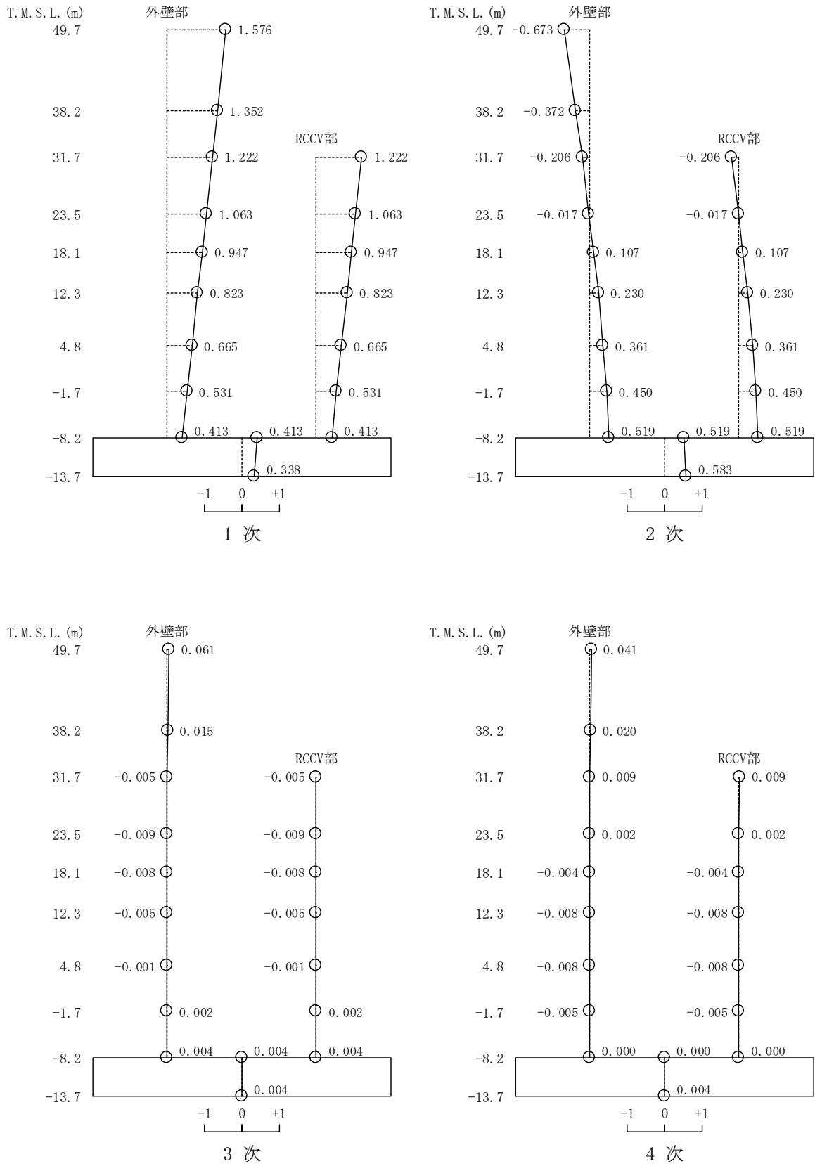
図 4-22 刺激関数図 (ケース 4) (NS方向, S s -1) (1/2)
