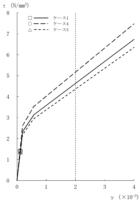
図2-63 \tau - \gamma 関係と最大応答値 (Ss-1, EW方向, 4F) (2/8)
