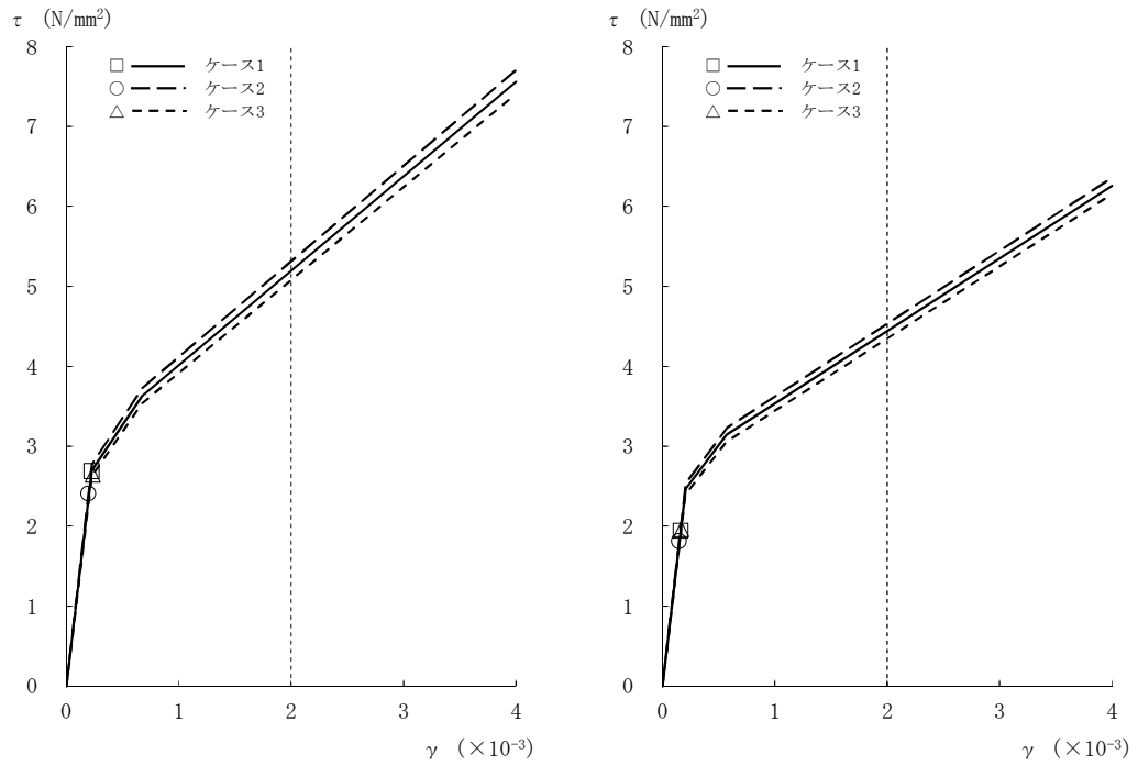
図2-19 \tau - \gamma 関係と最大応答値 (Ss-2, NS方向, B2F) (7/8)
