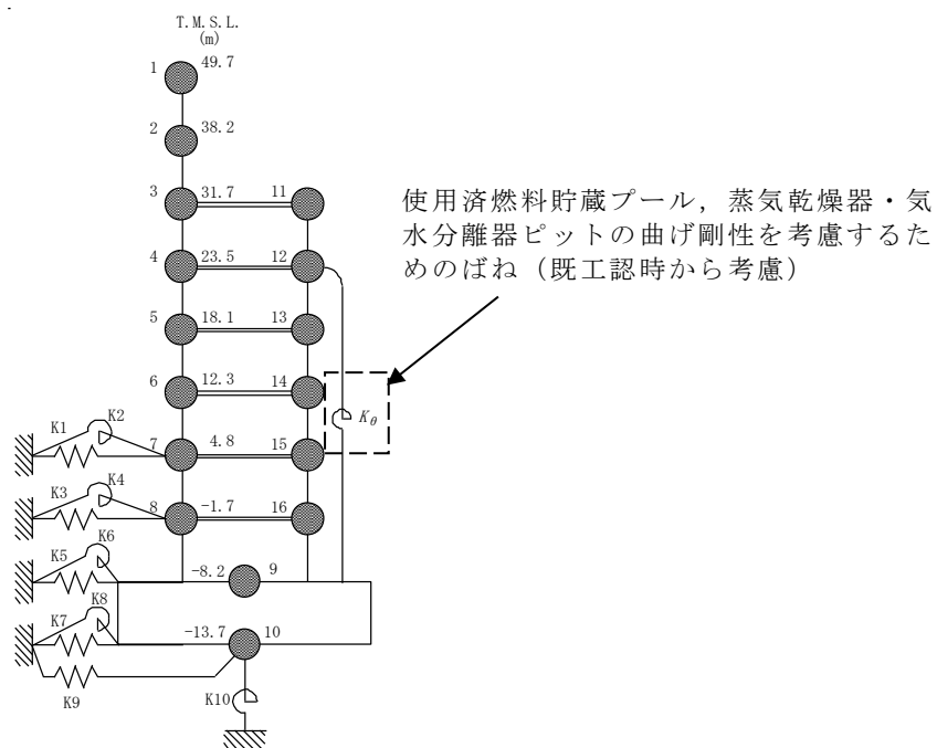
図3-3 今回工認の原子炉建屋の地震応答解析モデル (EW方向)
