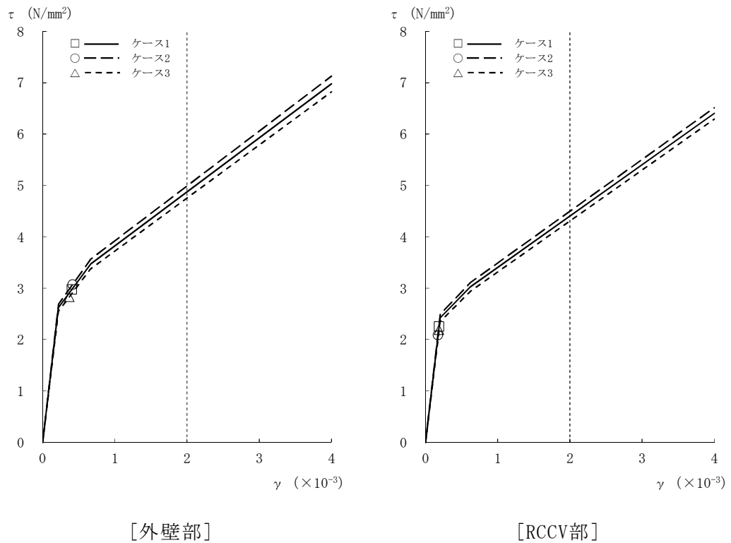
図2-18 \tau - \gamma 関係と最大応答値 (Ss-1, NS方向, B1F) (6/8)
