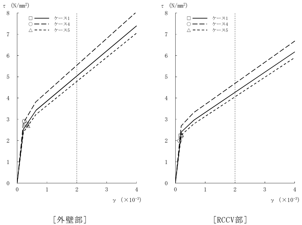
図2-66 \tau - \gamma 関係と最大応答値 (Ss-8, EW方向, B1F) (6/8)
