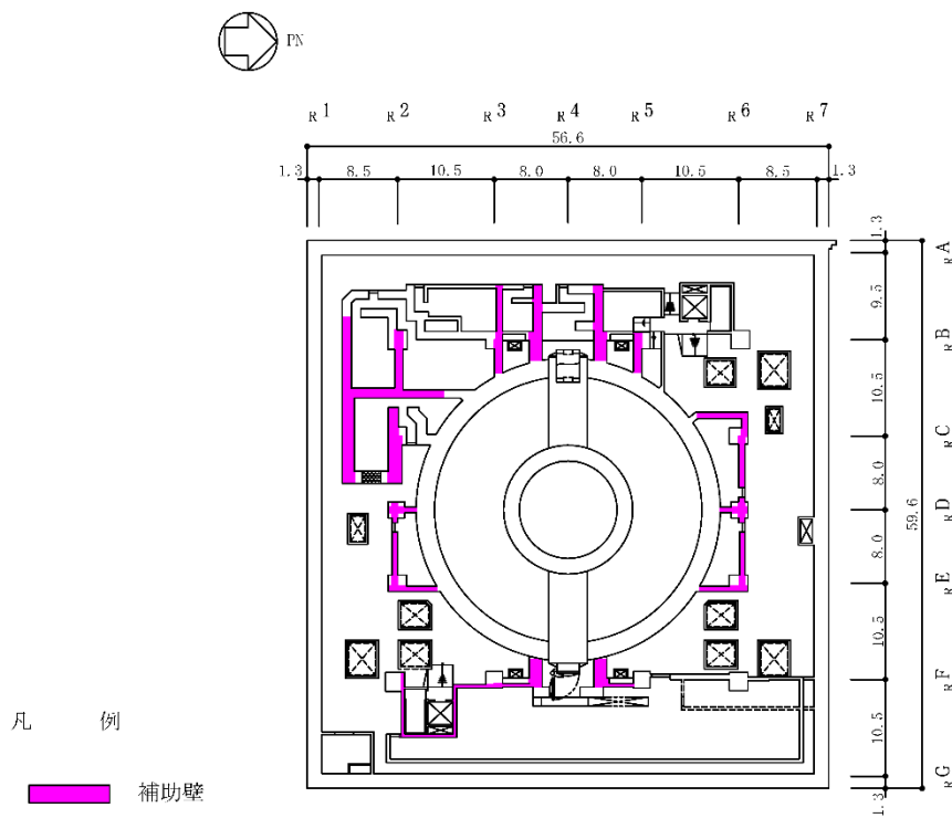
図 2-2 補助壁の考慮範囲 (B2F, T. M. S. L. - 1.7m) (単位 : m) (2/6)
