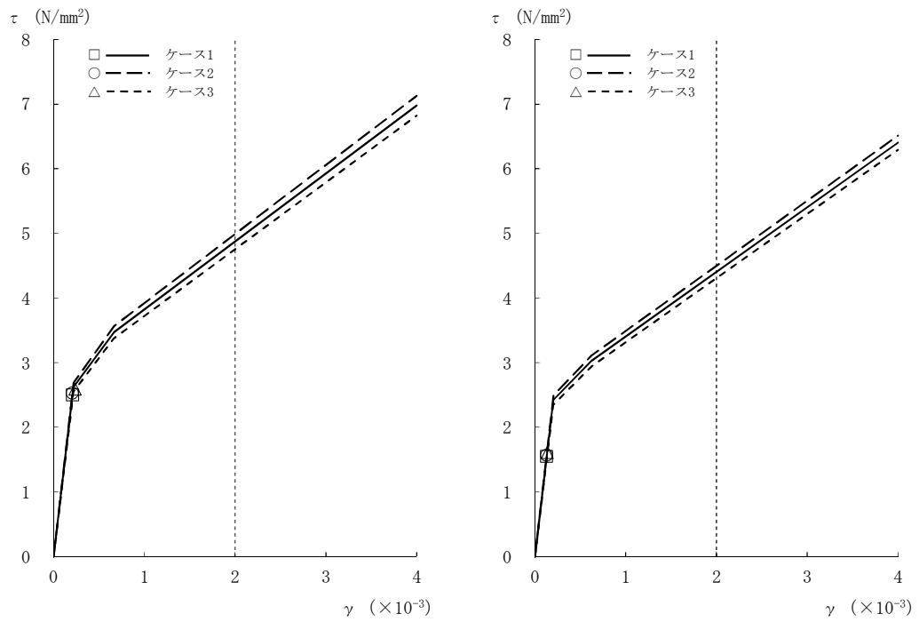
図2-20 \tau - \gamma 関係と最大応答値 (Ss-3, NS方向, B1F) (6/8)
