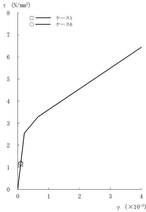
図2-118 τ - γ 関係と最大応答値 (Sd-3, NS方向, 1F) (5/8)
