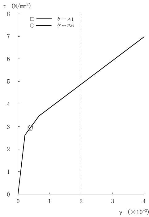
図2-103 τ - γ 関係と最大応答値 (Ss-8, NS方向, B1F) (6/8)
