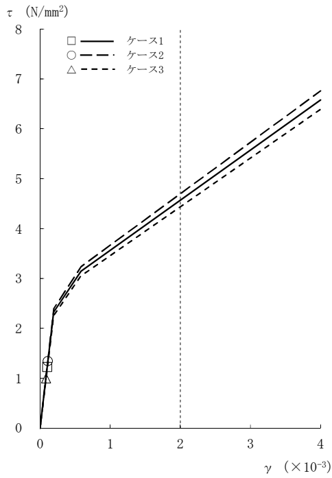
図2-22 \tau - \gamma 関係と最大応答値 (Ss-1, EW方向, CRF) (1/8)
