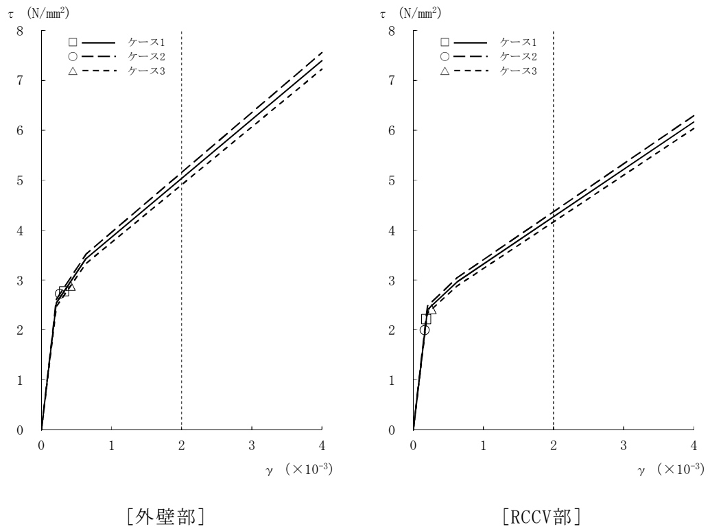
図2-25 \tau - \gamma 関係と最大応答値 (Ss-8, EW方向, B1F) (6/8)
