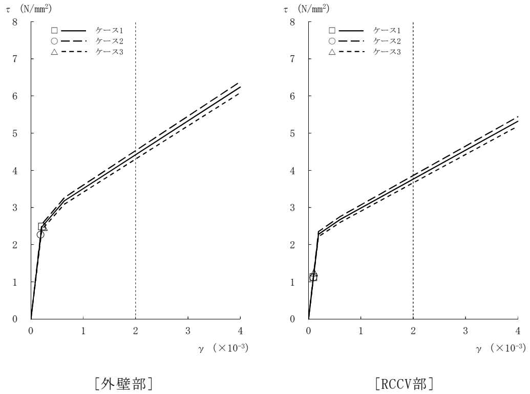
図2-25 \tau - \gamma 関係と最大応答値 (Ss-8, EW方向, 1F) (5/8)
