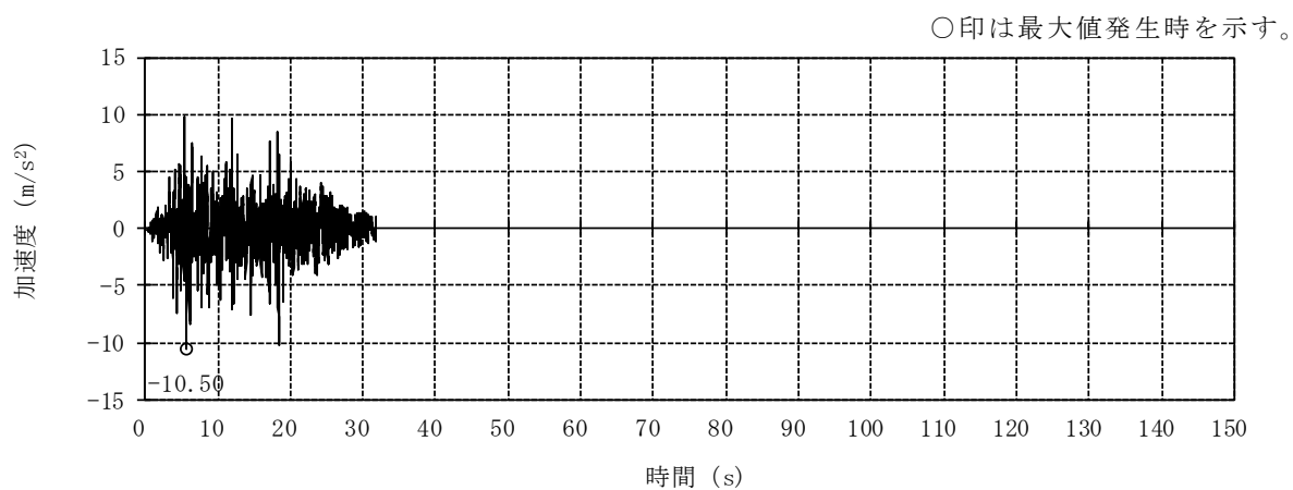
図 5-6 基準地震動 S S -1H の加速度波形 (解放基盤表面)
