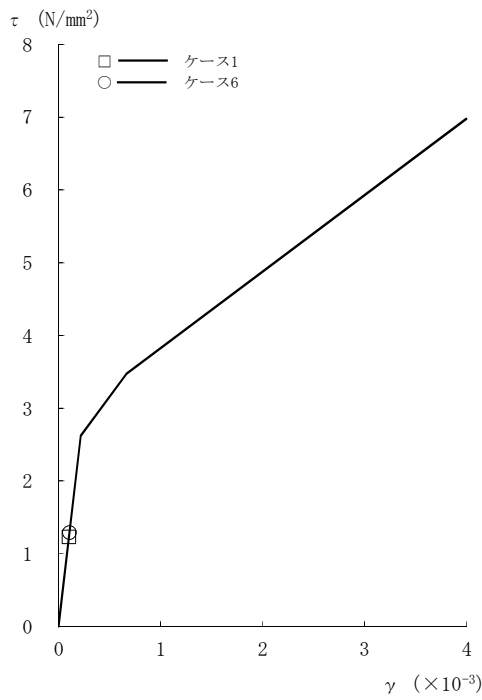
図2-118 τ - γ 関係と最大応答値 (Sd-3, NS方向, B1F) (6/8)
