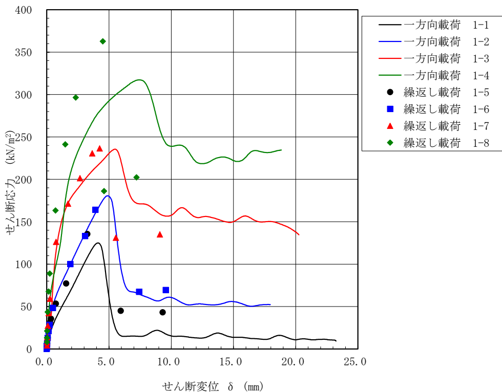
図 3-32 一方向載荷及び繰返し載荷試験によるせん断応力ーせん断変位関係
