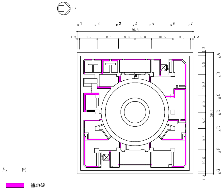
図 2-2 補助壁の考慮範囲 (B3F, T. M. S. L. - 8.2m) (単位 : m) (1/6)
