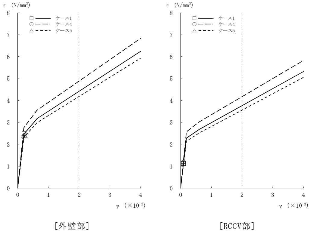
図2-66 \tau - \gamma 関係と最大応答値 (Ss-8, EW方向, 1F) (5/8)
