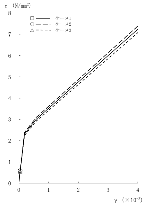
図2-39 \tau - \gamma 関係と最大応答値 (Sd-3, NS方向, 2F) (4/8)
