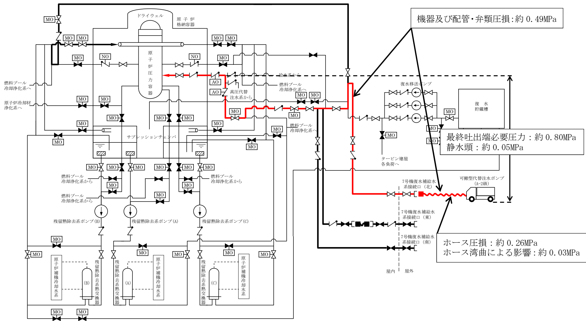
図 4-10 低圧代替注水系及び代替格納容器スプレィ冷却系の同時使用 原子炉圧力容器への注水及び原子炉格納容器内へのスプレィを同時に実施する場合 【施設区分：原子炉冷却系統施設，原子炉格納施設】
