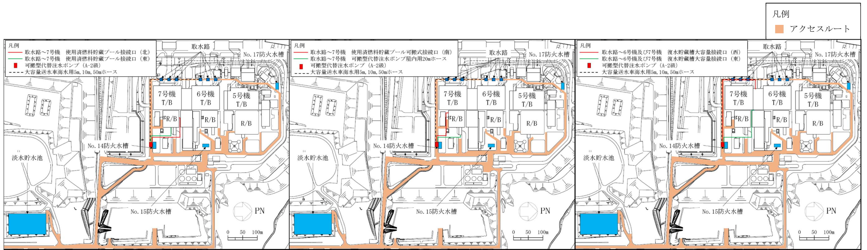
図 1-7 可搬型代替注水ポンプ屋外用 20m ホース 敷設ルート(7)
