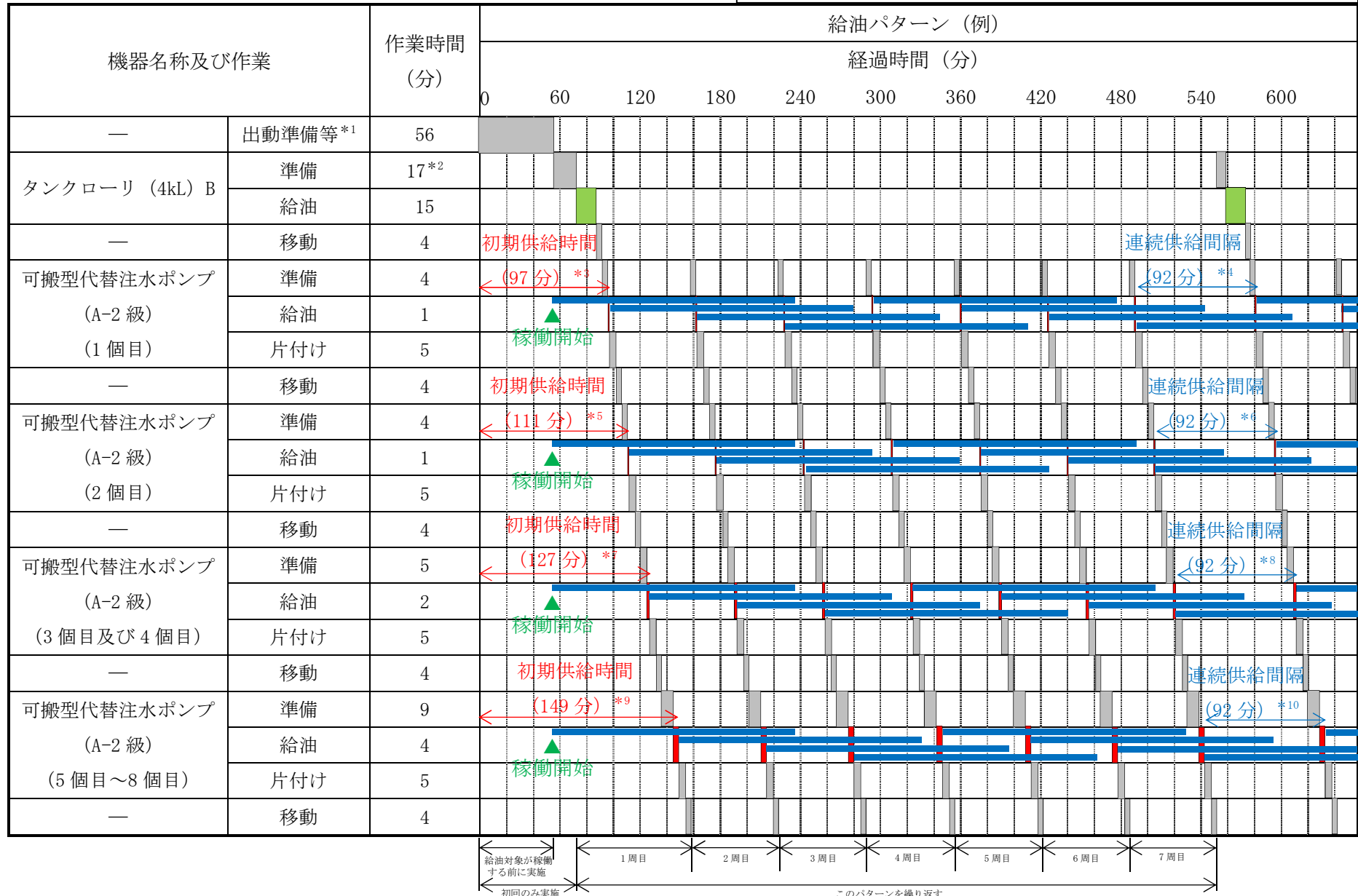
図 4-5 タンクローリ（4kL）B 給油作業 時系列
