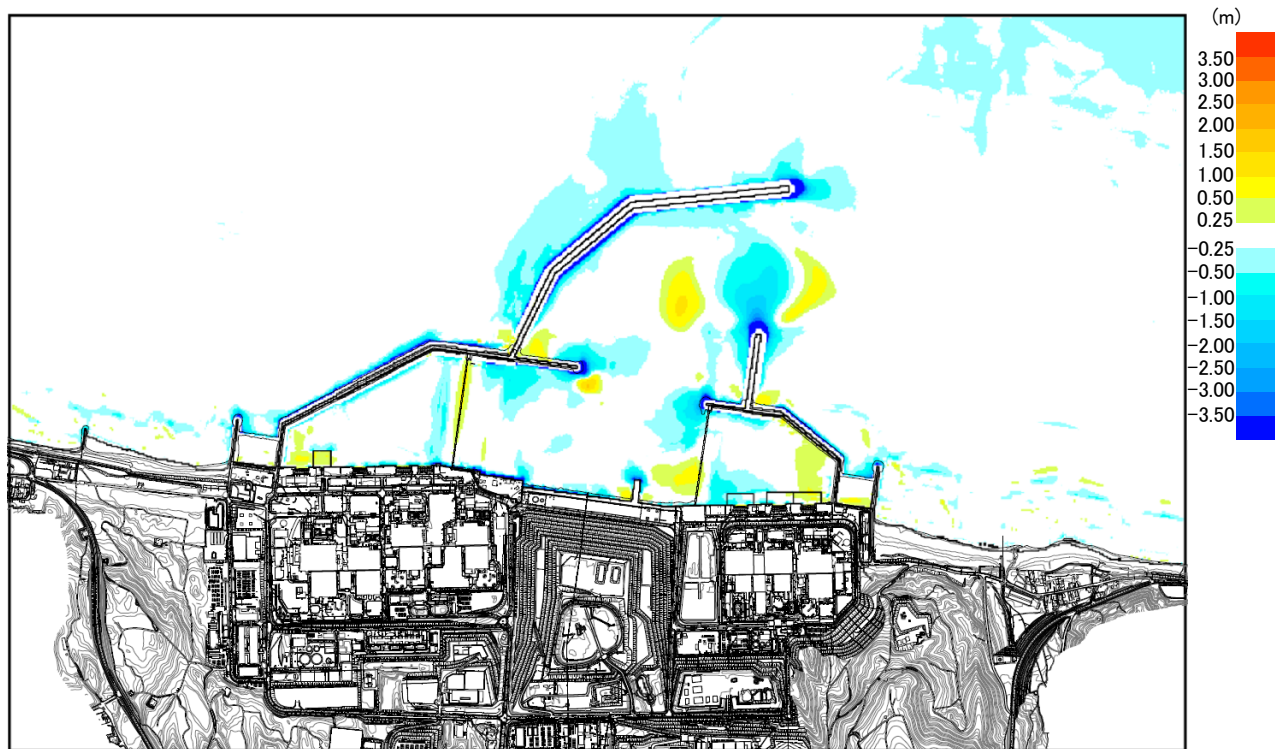
图 3.1-4(3) 堆積侵食分布図 D10 相当 (0.1mm)
