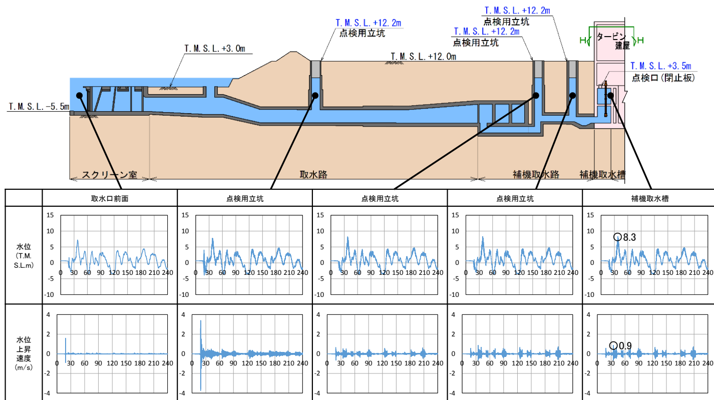
図 3.2-参 1-5 7号機補機取水槽（上昇側）において考慮する入力津波 各位置での水位時刻歴と流速（水位上昇速度）時刻歴
