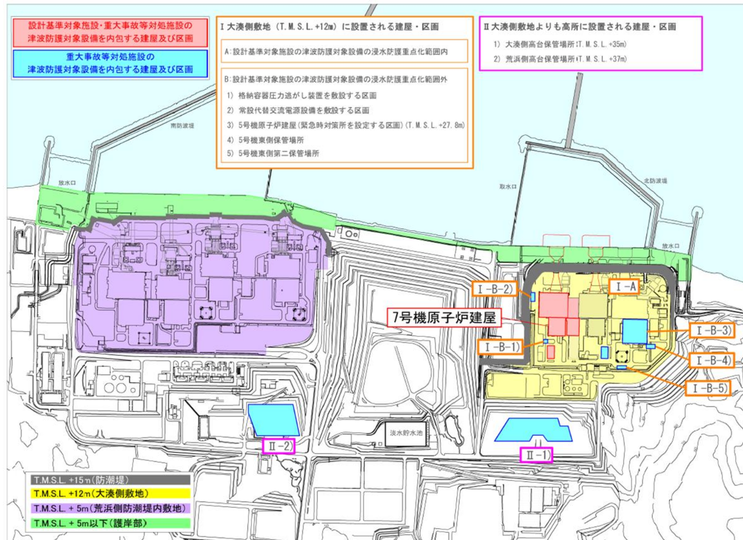
図 2.1-5 重大事故等対処施設の津波防護対象設備を設置する範囲
