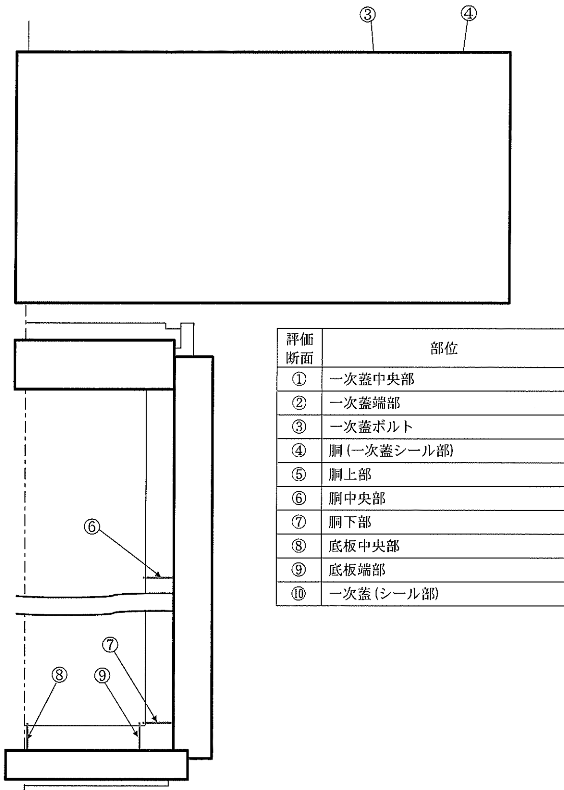
図 2.6.1-1 密封容器の応力評価位置
