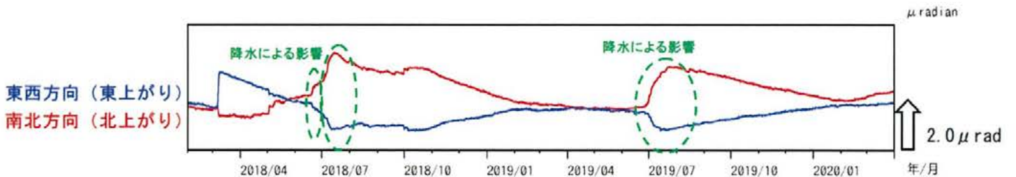
図 高千穂河原傾斜計
