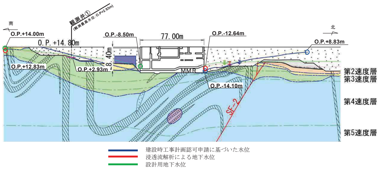
図 6-4 海水ポンプ室の設計用地下水位（縦断） （本文-図 3. 3-13(1)に観測井①を投影）
