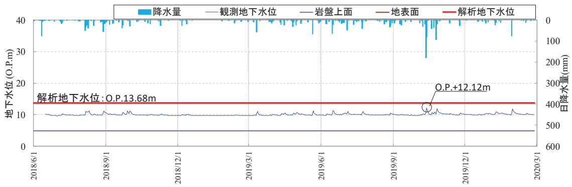
図 6-9(7) 地下水位観測記録と解析水位の関係 (観測井⑦)
