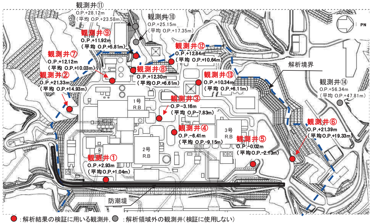
図 6-2 検証に用いる観測井位置図
