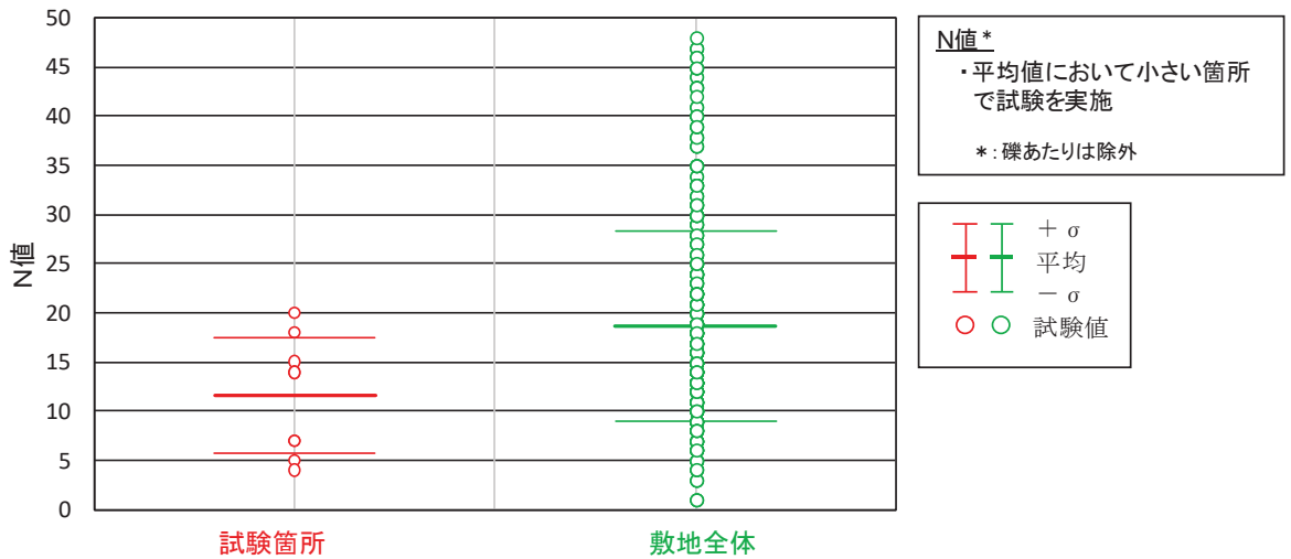
図 4.2-11 液状化強度試験位置の基本物性の比較 (盛土)
