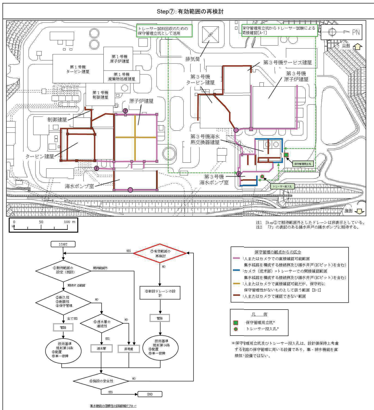
図 2-4-9 有効範囲の再検討での整理結果 (Step⑦)
