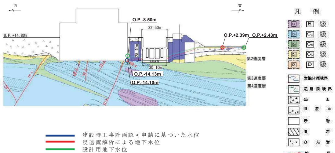
図 3.3-13(1) 海水ポンプ室の設計用地下水水位（縦断）
