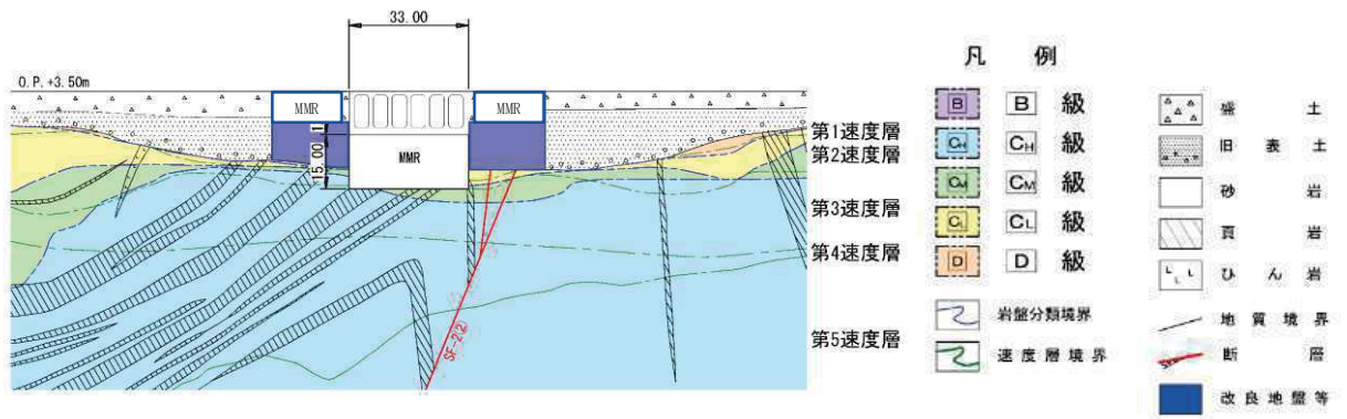
図 2-3 地盤改良体の配置図（取水口，A-A 断面）
