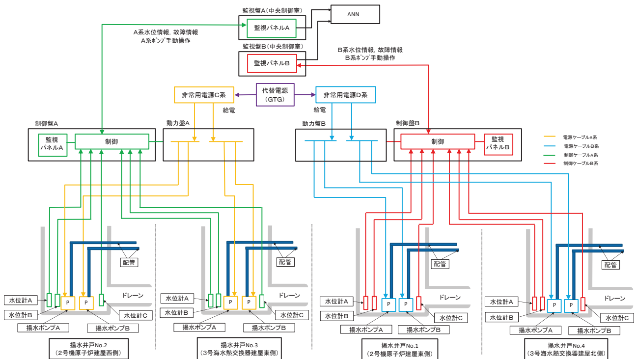
図 3-1-3 系統構成図
