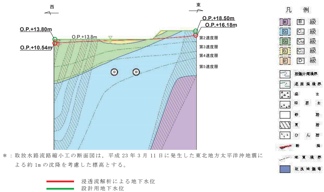
図 3.3-20(1) 取放水路流路縮小工の設計用地下水位 (1号機取水路)
