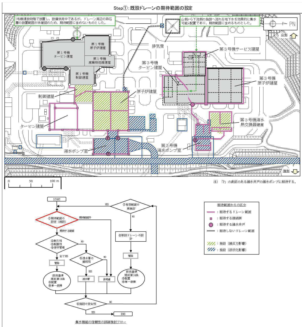
図 2-4-4 既設ドレーンの期待範囲の設定 (Step①)
