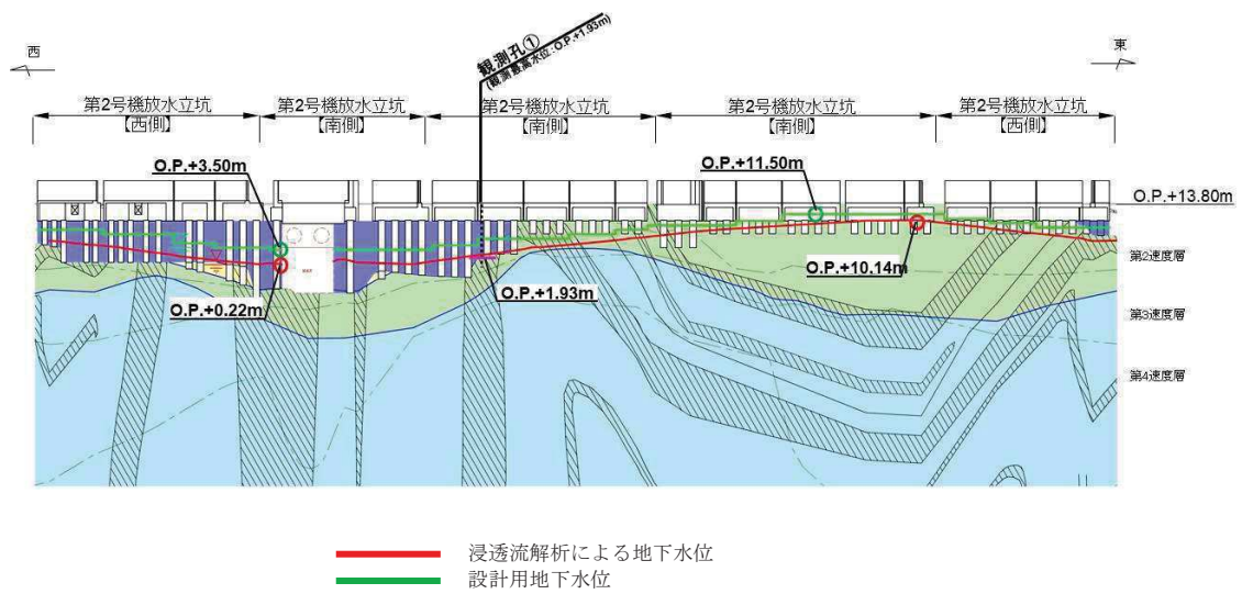
図 6-5 防潮壁の設計用地下水位（2号機放水立坑） （本文-図 3. 3-19(2)に観測井①を投影）
