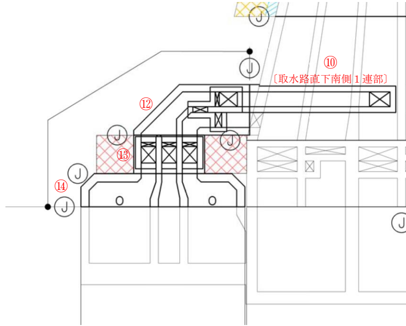
(a) 補機冷却用海水取水路（南側）
