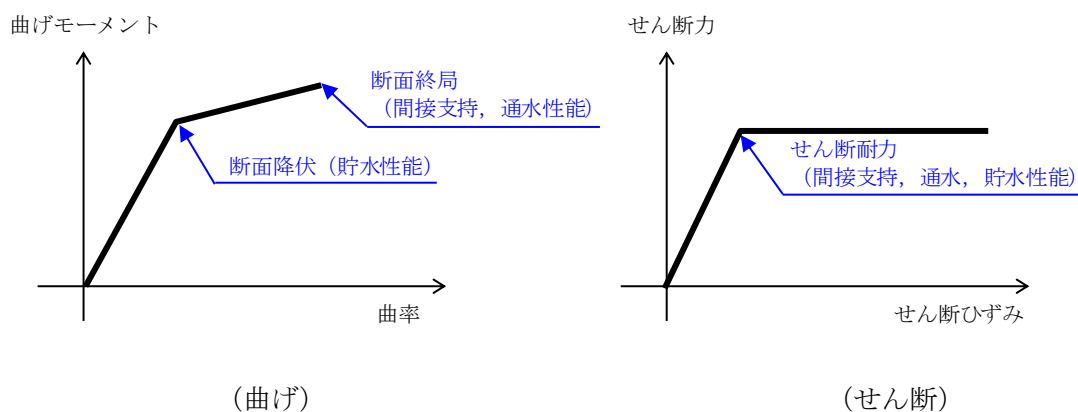
図 2-1 各要求性能と許容限界の関係の概念
