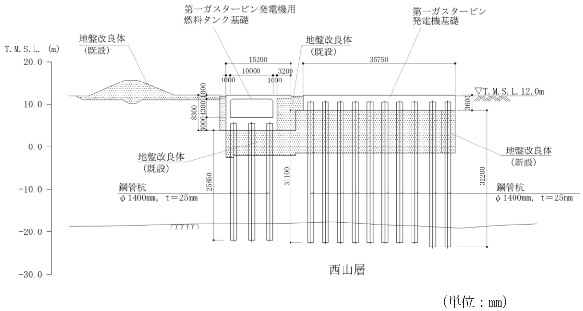
図 4-29 (3) 常設代替交流電源設備基礎断面図 (C-C 断面)
