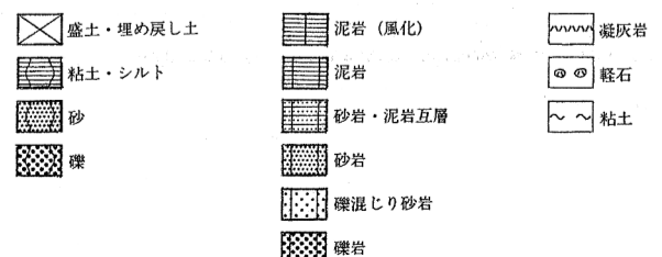
図-2(10) 6号機及び7号機の地質柱状図(7-5孔) ※図中赤破線は標高-155mの位置を示す。
