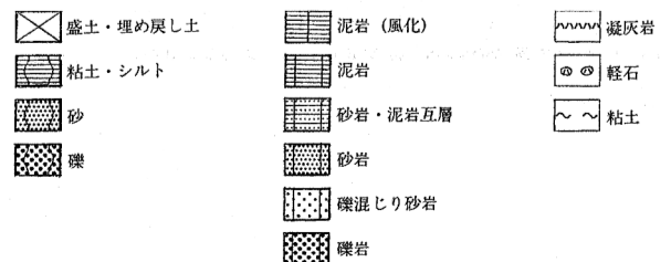
図-2(7) 6号機及び7号機の地質柱状図(7-2孔) ※图中赤破線は標高-155mの位置を示す。
